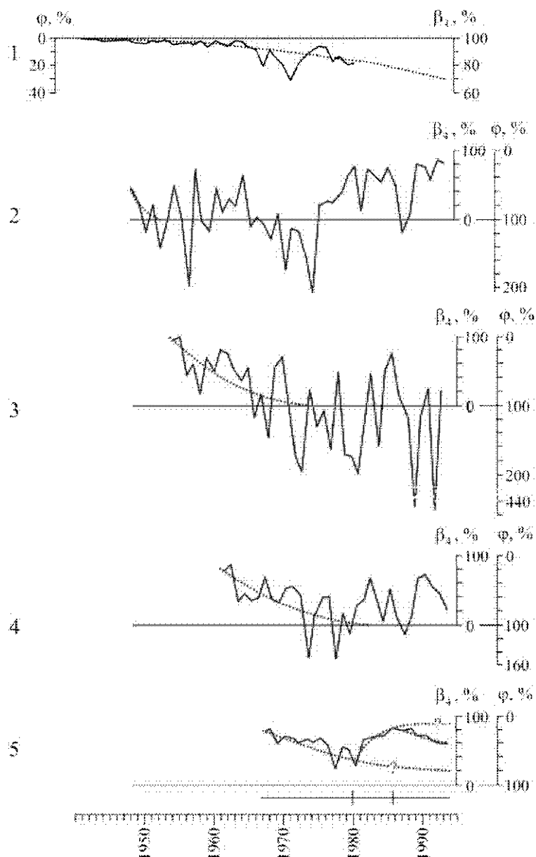
Рис. 2. Годовые значения наносодерживающей способности \beta_4 и коэффициента \phi отдельных водохранилищ за время их функционирования до 1995 г. Водохранилища: 1 – Роженув, 2 – Чхув, 3 – Гочалковце, 4 – Дембе, 5 – Влоцлавек. В случае водохранилища Влоцлавек обозначены периоды: перед началом извлечения осадков (до 1982 г), с извлеченными осадками (1982-1987 гг) и после окончания (с 1988 г).
