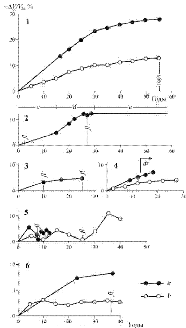
Рис. 4. Ход сокращения объема -\Delta V/V_0 отдельных водохранилищ, охарактеризованный на основе: a — повторной нивелировки чаши, b — баланса транспорта наносов. Водохранилища: 1 Рожпув, 2 Поромбка, 3 Тресна, 4 Влоцлавек, 5 Чхув, 6 Гочатковце. На горизонтальной оси обозначены годы функционирования водохранилища от заполнения до 1995 г. fl — частичный или полный спуск (промывка) водохранилища (flushing), dr — начало извлечения осадков из водохранилища Влоцлавек (dregging). Для водохранилища Поромбка обозначены периоды: c — перед установкой турбин, частичное заполнение (до 1953 г.), d — до заполнения водохранилища Тресна (1953-1966), e — после заполнения водохранилища Тресна (с 1967 г.).
