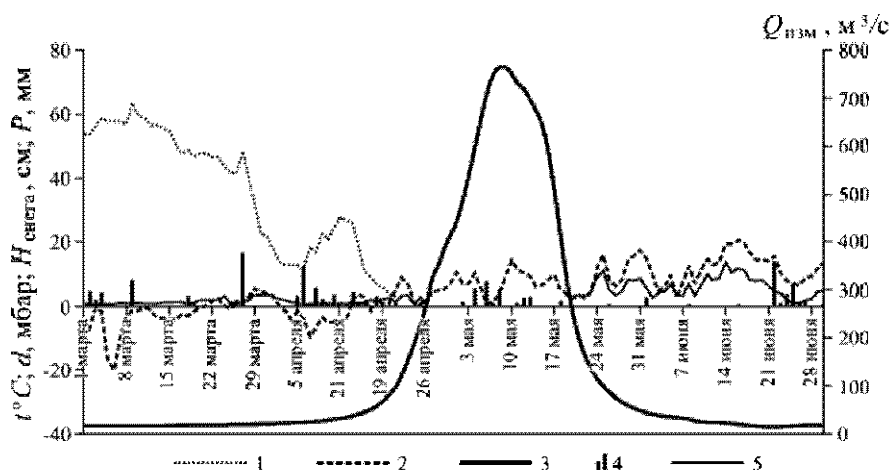
Рис.3. Колебания гидрометеорологических элементов во время половодья и гидрограф стока р. Лузы (г.п. Объячсво): 1- высота снежного покрова; 2 – влажность; 3 – измеренный расход воды; 4- осадки; 5- средняя температура воздуха.
