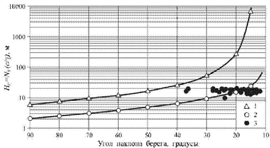
Рис. 1. Связь критической высоты берегов и крутизны откосов для грунтов: 1 - в сухом состоянии; 2 - в состоянии увлажнения; 3 - берегов Волги и Терека
