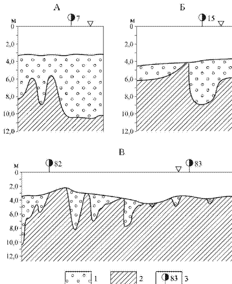
Рис. 1. Геологическое строение порогов Енисея (продольные разрезы гребней): А – аккумулятивное (Ладейский); Б – эрозионно-аккумулятивное (Верх. Палудинский); В – эрозионное (Атамановские камни). 1 – галечный аллювий; 2 – скальные коренные породы; 3 – километраж по судовому ходу. Горизонтальный масштаб разрезов – 1:10000.
