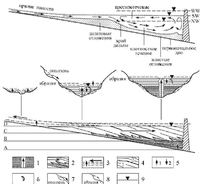
Рис. 1. Гидролого-морфологическая схема водохранилища: 1 – осадки пылевато-илистые и направление нарастания; 2 – осадки дельтовые и направление нарастания; 3 – материал, накопленный на полностью обмелевшем водохранилище и направление нарастания; 4 – граничная величина заполнения чаши осадками в момент перехода от первой ко второй фазе заиления; 5 – направления заиления водохранилища (1- заиление положительное, 2 – заиление отрицательное); 6 – взвешивание осадков в результате волнения; 7 – принос материала оползней; 8 – принос материала абразии берегов; 9 – уровень воды в водохранилище (NW – низкий, SW – средний, WW – высокий). Зоны по глубине, заполняемые: А – осадками пылевато-илистыми, В – песчано-пылеватыми, С – преимущественно песчаными, D – осадки, перекрывающие вновь формирующееся русло и пойму на территории полностью заиленного водохранилища.
