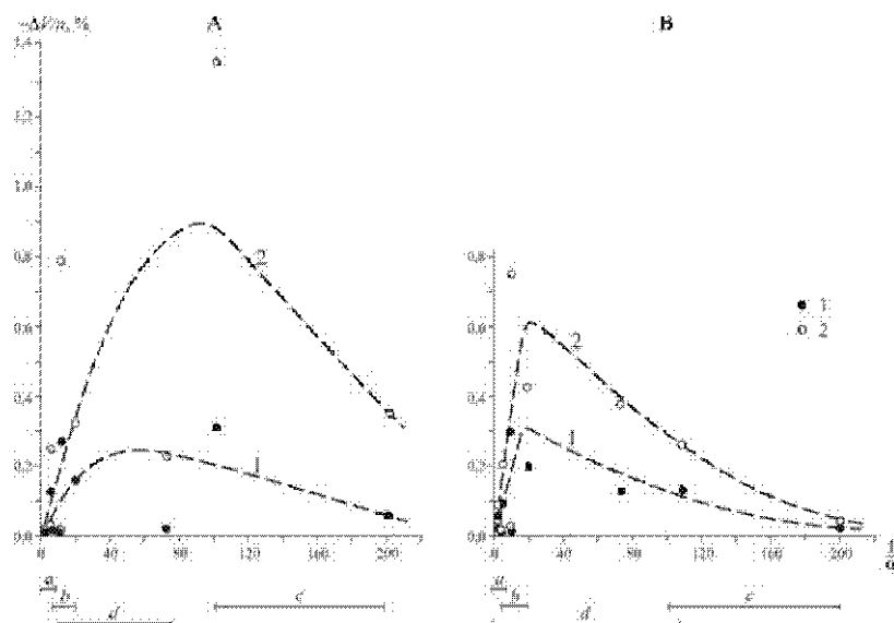
Рис. 5. Связь между средним годовым сокращением объема водохранилища -\Delta V/n и кратностью водообмена в течение года 1/a , охарактеризованная на основе: 1 – баланса паводков, 2 – повторной нивелировки чаши. Периоды функционирования водохранилищ: А – первые 5-20 лет, В – первые 21-30 лет. Категории водохранилищ: а – глубокие на верхних участках карпатских долин, б – глубокие на средних участках карпатских долин, с – мелкие в карпатских долинах (выравнивающие), d – широкие и мелкие на низменности.
