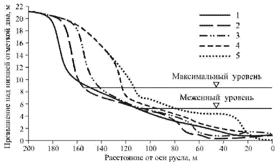
Рис. 2. Поперечные профили левого берега р. Волги в пос. Волжском (3 км от ворот Рыбинского шлюза) в годы: 1 - 1970; 2 - 1987; 3 - 1992; 4 - 1997; 5 - 1999
