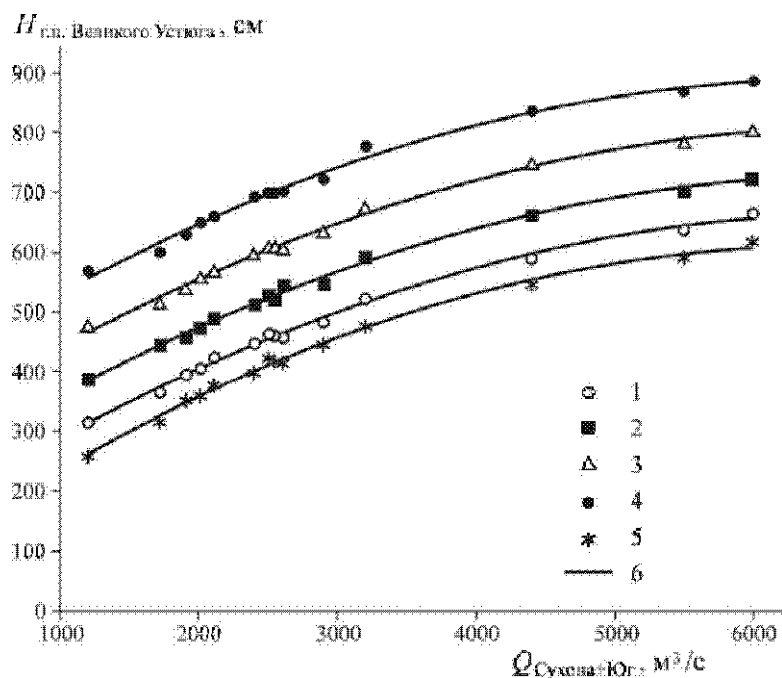
Рис. 6. Изменение уровня воды у г. Великого Устюга при различной высоте заторного повышения уровней в районе о-ва Коневецкие пески и изменение расхода воды в Малой Северной Двине.
