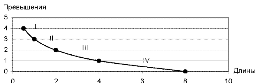
Рис. 2. Идеализированный продольный профиль сопряженных разнорядковых русел в бассейне 4-го порядка (длины и относительные превышения даны в условных единицах; за единицу превышения принято превышение истока над устьем тальвега I порядка, за единицу длины взята длина водотока I-го порядка модального бассейна).
