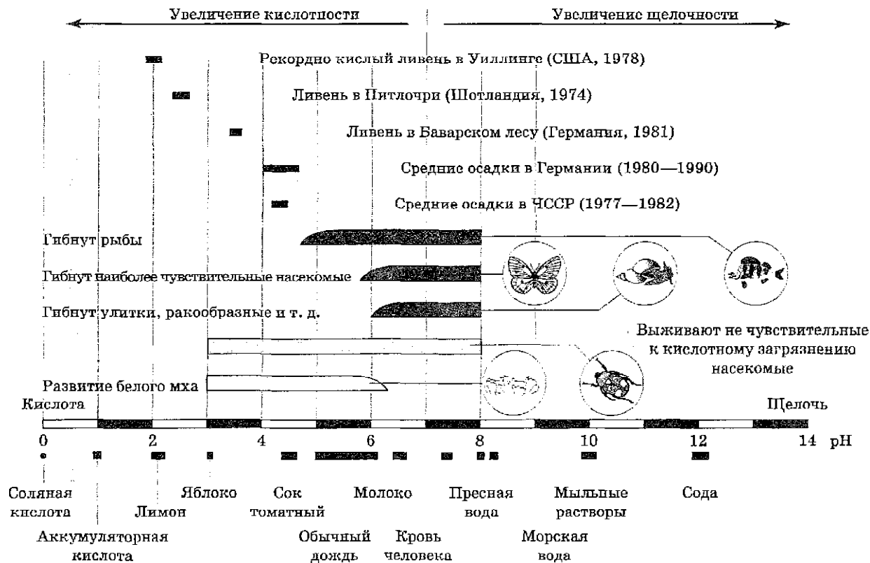
Рис. 9.7. Ориентировочная кислотность дождевой воды, воды и различных веществ, выраженная в единицах pH
