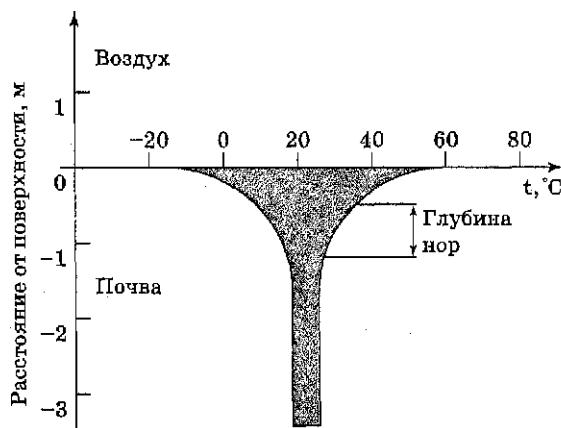
Рис. 3.3. Уменьшение годового колебания температуры почвы с глубиной
