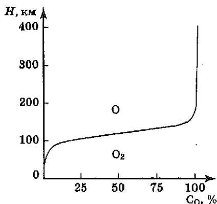
Рис. 7.6. Распределение кислорода в молекулярной и атомарной формах по высоте атмосферы (по Ю. И. Скурлатову, Г. Г. Дуже, А. Мизити)
