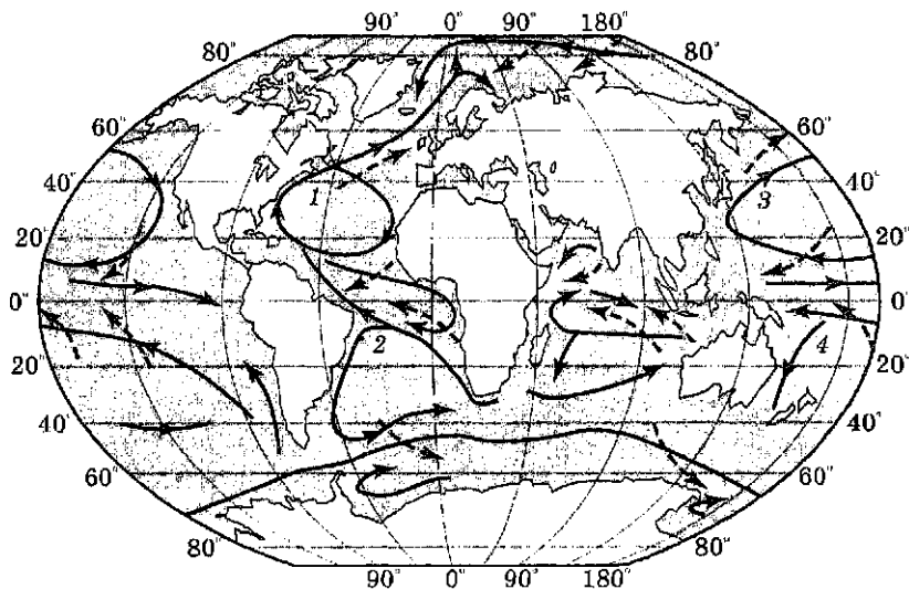
Рис. 7.16. Главные течения Мирового океана
