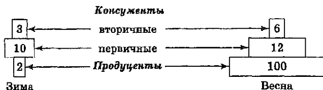
Рис. 5.6. Сезонные изменения в пирамидах биомассы озера (на примере одного из озер Италии): цифры — биомасса в граммах сухого вещества, приходящегося на 1 \text{ м}^3
