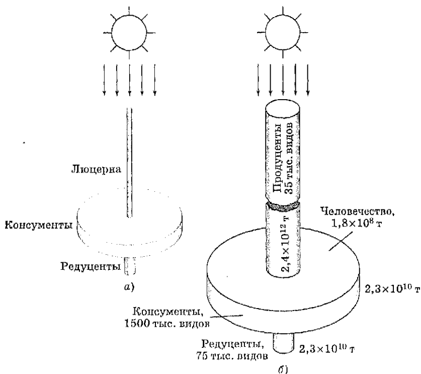
Рис. 5.16. «Волчок жизни» (по Н. Реймерсу): а — для упрощенной модельной экосистемы Ю. Одума: люцерна — теллятина — мальчик (с включением других консументов и редуцентов); б — для биоценоза Земли в целом
