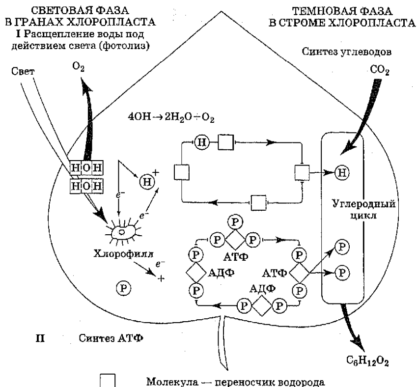
Рис. 2.2. Процесс фотосинтеза (по С. Г. Мамонтову)
