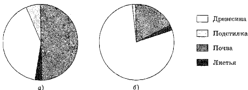
Рис. 6.10. Распределение органического углерода в частях экосистем северного (а) и тропического (б) лесов (по Ю. Одуму)
