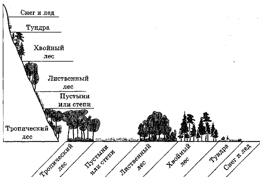
Рис. 3.6. Вертикальная и широтная зональности растительности
