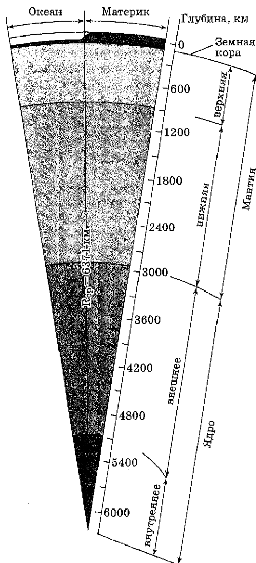
Рис. 7.1. Внутреннее строение Земли
