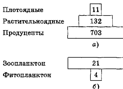
Рис. 5.5. Пирамиды биомасс биоценозов кораллового рифа (а) и пролива Ла-Манш (б): цифры — биомасса в граммах сухого вещества, приходящегося на 1 м²
