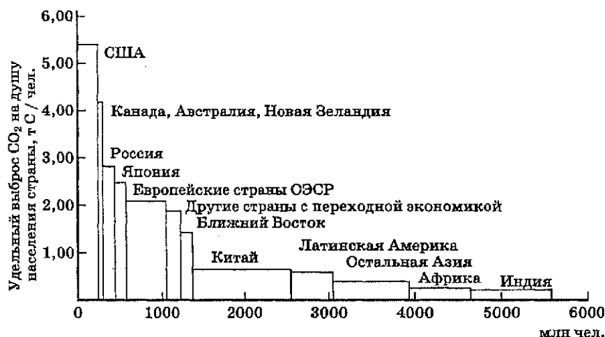
Рис. 9.6. Распределение по странам и группам стран удельного (на душу населения) выброса CO 2 в пересчете на углерод
