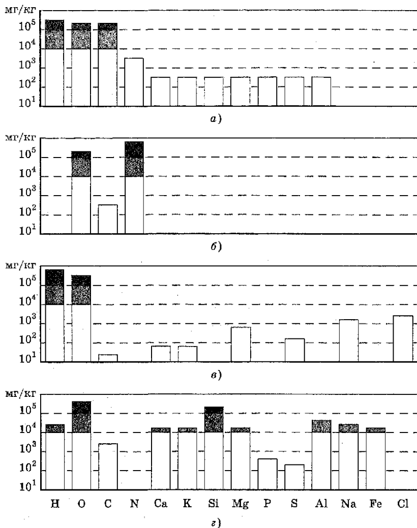
Рис. 2.1. Распространенность химических элементов в живом веществе (а), атмосфере (б), гидросфере, литосфере (в) (по В. Лархеру)
