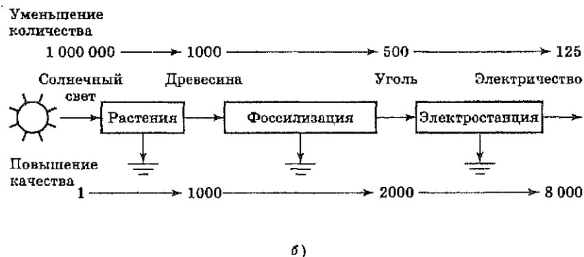
Рис. 6.9. Схема повышения качества и снижения количества энергии, идущей от Солнца, при ее преобразовании в пищевой цепи (а) и цепи получения электроэнергии (б) (по Г. Одуму, Э. Одуму, Ю. Одуму).
