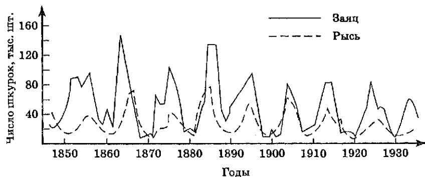
Рис. 5.12. Равновесие популяций в системе «хищник—жертва» на примере «рысь—заяц» по результатам наблюдений за количеством шкурок, добытых компанией Гудзонова залива (по Мак-Луличу)
