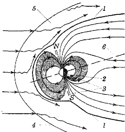
Рис. 7.24. Строение магнитосферы Земли: 1 — магнитопауза; 2 — Земля; 3 — радиационный пояс; 4 — фронт ударной волны; 5 — переходная область; 6 — плоскость геомагнитного экватора
