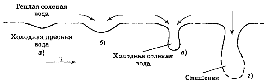
Рис. 7.15. Рост солевых пальцев в расслоенной воде по стадиям (а — в) развития процесса
