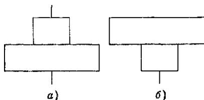
Рис. 5.4. Нарушенная (а) и перевернутая (б) пирамиды численности
