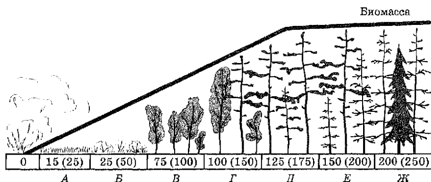
Рис. 6.7. Фазы типичной наземной сукцессии (по Н. Ф. Реймерсу): А —вейниковский луг; Б — зарастание кустарниками; В — березовый или осиновый лес; Г — смешанный лес; Д — сосновый лес; Е — сосново-кедровый лес; Ж — кедрово-пихтовый лес
