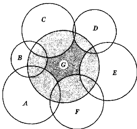
Рис. 5.15. Схема сокращения фундаментальной ниши вида G (покрытая точками и заштрихованная области) до его реализованной ниши (заштрихованная область) в результате диффузной конкуренции с видами A , B , C , D и F (по П. Джиллету )
