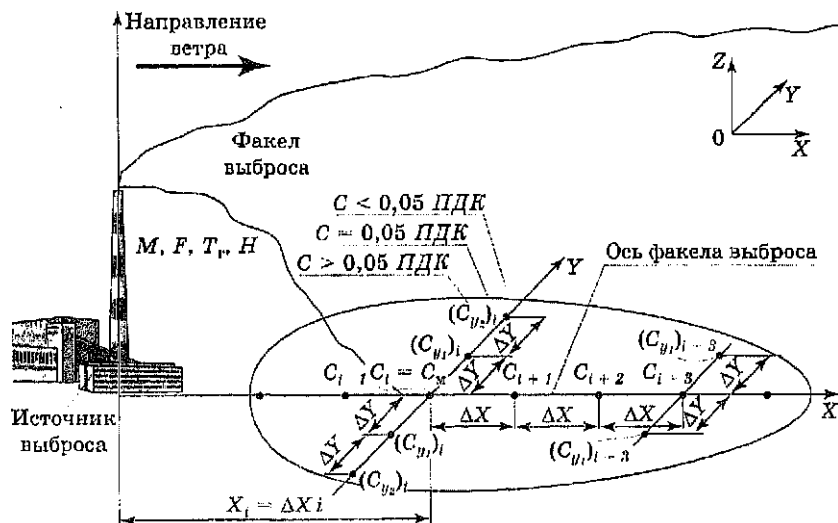
Рис. 10.13. Схема размещения расчетных точек при определении приземной концентрации вредного вещества в атмосфере под факелом выброса одиночного точечного источника
