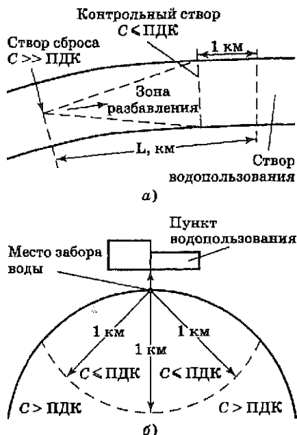
Рис. 10.16. Схемы расположения контрольного створа в водотоке (а) и контрольной зоны в непроточном водоеме (б) при нормировании содержания загрязняющих веществ в воде (по Г. В. Стадницкому и А. И. Родионову)
