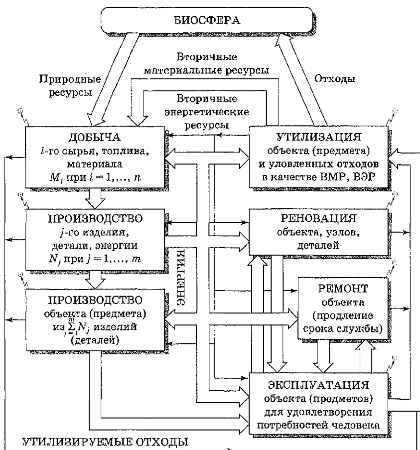
Рис. 9.1. Схема использования природных ресурсов при удовлетворении потребностей общества (по Н. И. Николайкину): \nearrow — неудовленное при очистке вещество и низкопотенциальная энергия, рассеивающиеся в окружающей среде
