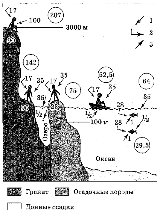
Рис. 3.5. Дозы получаемого радиоактивного облучения, мрад/г. (по Н. Ф. Реймерсу): 1 — космические лучи; 2 — внутренние \alpha -лучи и излучение ^{40}\text{K} , содержащегося в живых организмах; 3 — излучение местных внешних источников
