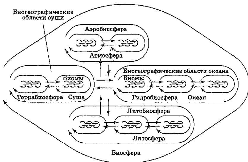
Рис. 6.3. Принципиальная схема круговорота веществ (по Н. Ф. Реймерсу)
