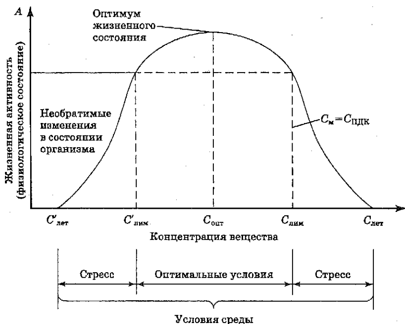
Рис. 3.12. Интерпретация закона толерантности на примере воздействия на организм концентрации некоего вещества как экологического фактора: C_{лет} , C_{лим} , C_{опт} , C_{лим} , C_{лет} — концентрации летальная, лимитирующая, оптимальная, максимальная и предельно допустимая
