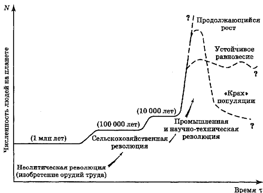
Рис. 4.8. Увеличение поддерживающей емкости среды для популяции человека (по Т. Миллеру), масштаб по осям условный
