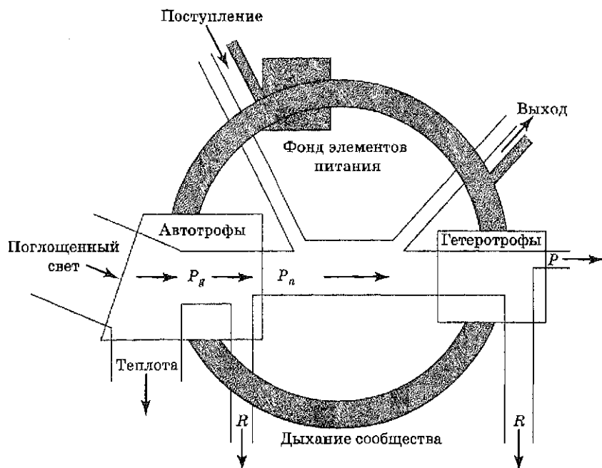
Рис. 7.25. Схема биогеохимического круговорота (заштрихованное кольцо), совмещенная со схемой однонаправленного потока энергии (по Ю. Одуму): P_g — валовая продукция; P_n — чистая первичная продукция, которая может быть потреблена гетеротрофами в данной экосистеме либо экспортирована, например, для нужд человека; R — дыхание; P — вторичная продукция
