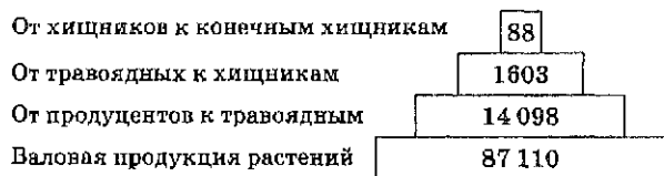
Рис. 5.7. Пирамида энергии: цифры — количество энергии, \text{кДж} \cdot \text{м}^{-2} \cdot \text{г}^{-1}
