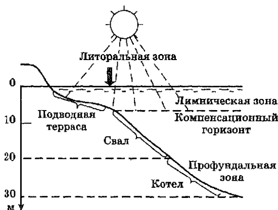
Рис. 6.12. Главные зоны в экосистеме непроточного континентального водоема (по Ю. Одуму); глубины указаны ориентировочно
