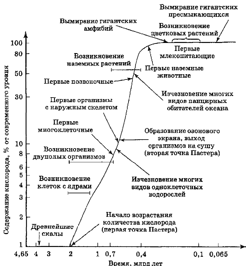
Рис. 7.28. Схема эволюции состава атмосферы и биосферы (по Ю. Одуму с дополнениями)
