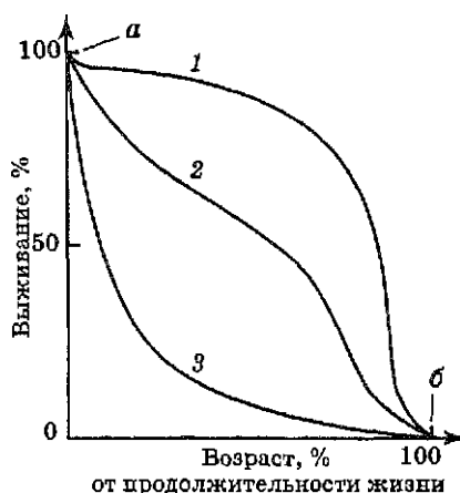
Рис. 4.4. Кривые выживания: 1 — человек или крупные млекопитающие; 2 — гидра или чернохвостый олень; 3 — устрица или рыба
