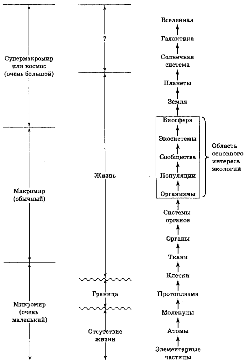
Рис. 1.1. Уровни организации материи (по Т. Миллеру)
