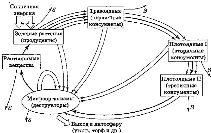
Рис. 6.2. Схема большого биосферного круговорота (по В. А. Радкевичу): S — энтропия
