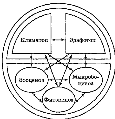
Рис. 6.1. Структурная схема биogeоценоза (по В. Н. Сукачеву)
