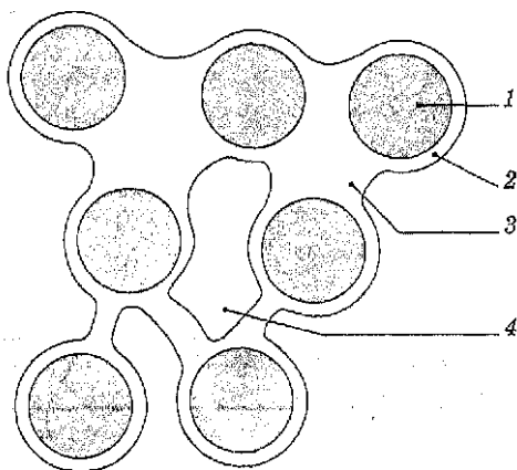
Рис. 3.10. Типы почвенной воды, доступной корням растений (по И. Грину, У. Стауту, Д. Тейлору): 1 — частицы почвы; 2 — гигроскопическая вода; 3 — капиллярная вода; 4 — воздух или гравитационная вода
