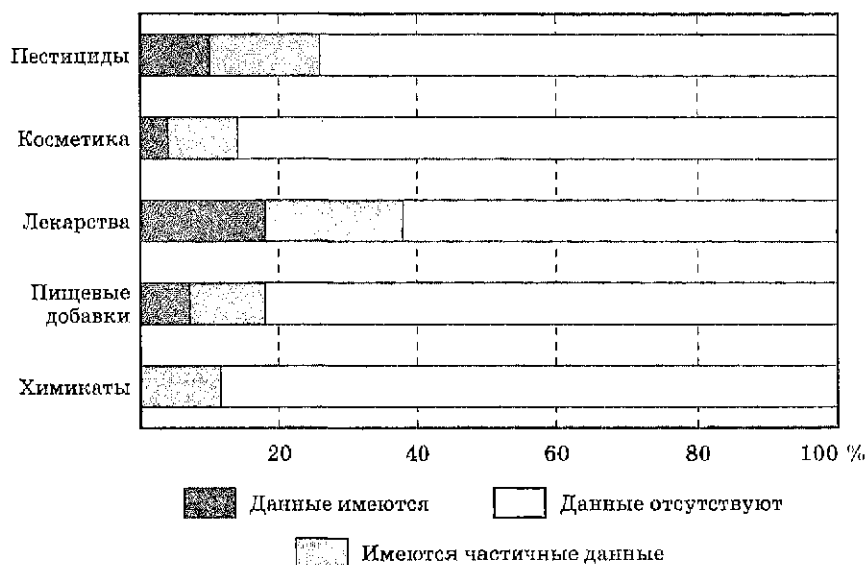
Рис. 8.7. Данные о токсичности по группам химических веществ по данным UNEP на 1991 г.
