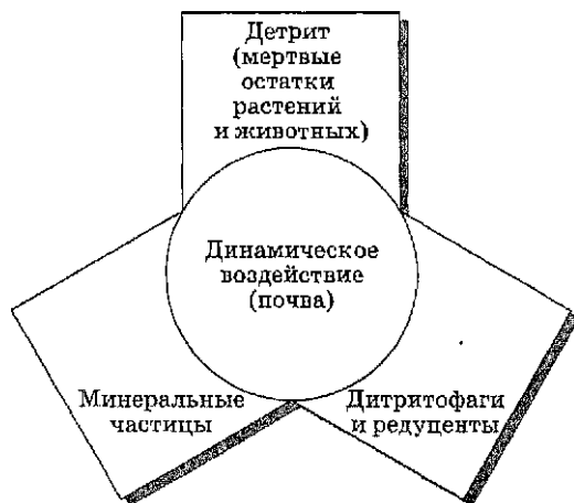
Рис. 3.8. Схема преобразования минерального вещества в почву
