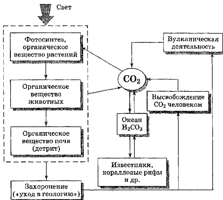
Рис. 6.4. Структурная схема круговорота углерода
