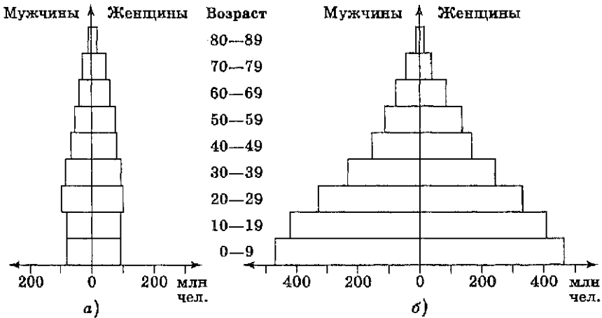
Рис. 8.3. Половозрастные пирамиды для развитых (а) и развивающихся (б) стран на 1984 г. (по В. Небелу)
