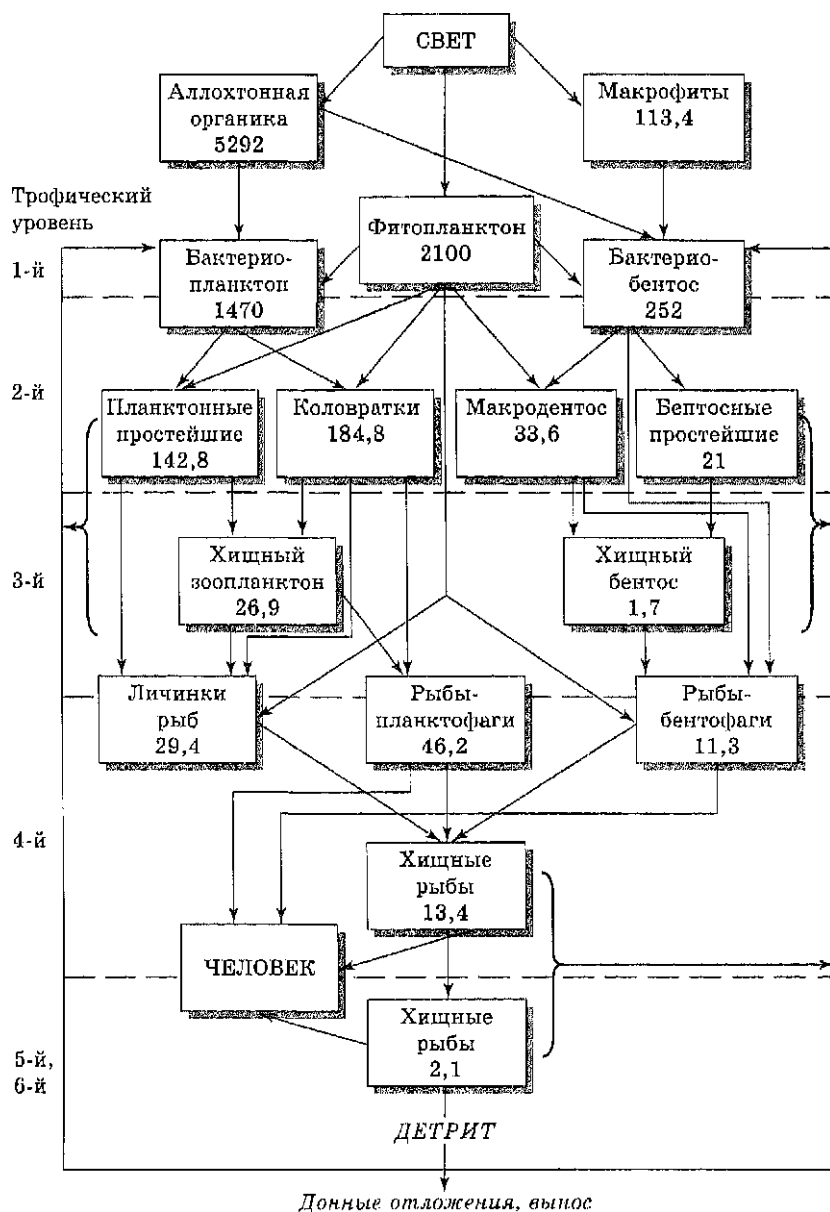
Рис. 5.9. Схема потоков энергии в трофической сети биоценоза (по Н. В. Бутурину, А. Г. Поддубному): цифры — годовичная продукция популяций, кДж/м 2
