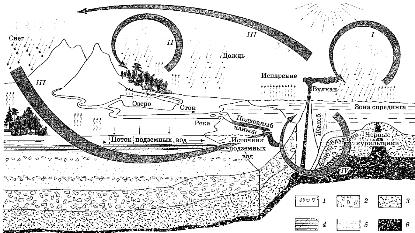
Рис. 7.19. Схема круговорота воды на Земле: I — над океаном; II — над сушей; III — над сушей и океаном; IV — геологический круговорот; 1 — осадочные породы; 2 — граниты, 3 — базальты; 4 — водоупор; 5 — морские осадки; 6 — мантийное вещество
