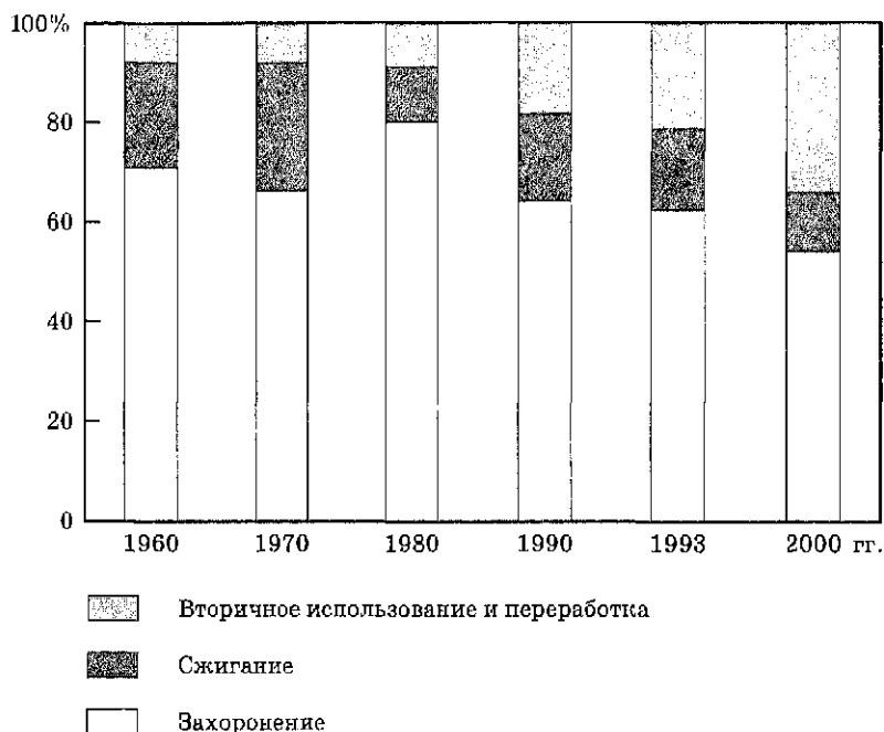
Рис. 9.13. Диаграмма изменения пропорций между методами удаления ТБО в США
