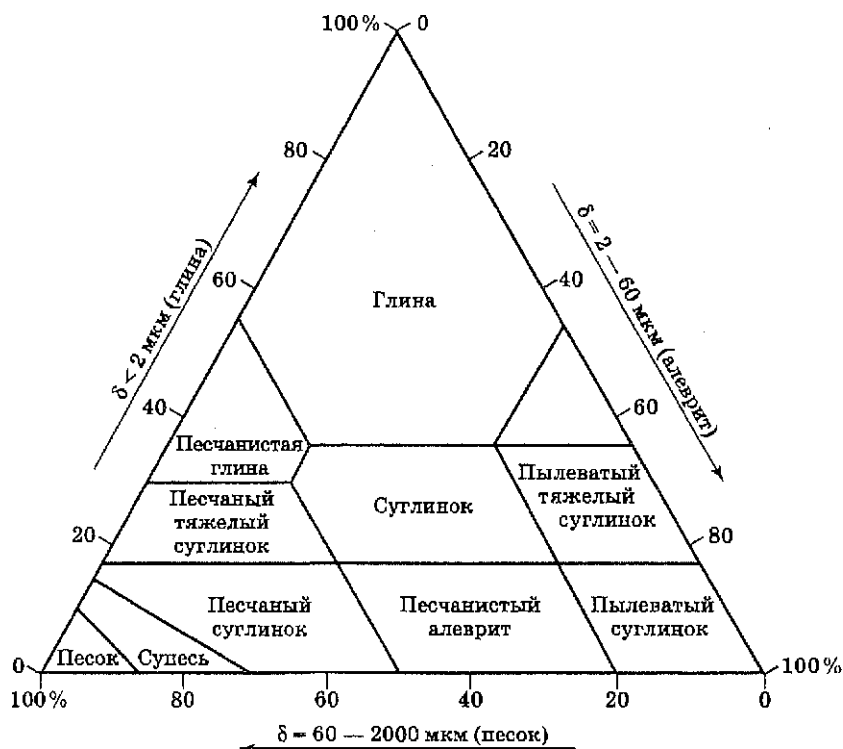
Рис. 3.9. Треугольная диаграмма классов механического состава почв: δ — размер частиц
