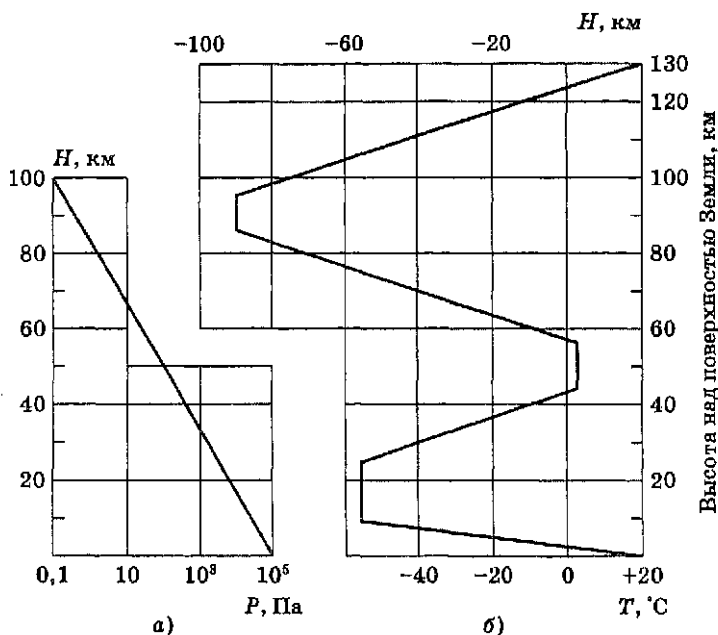
Рис. 7.5. Изменение давления (а), температуры (б) над поверхностью Земли и структура атмосферы (в)
