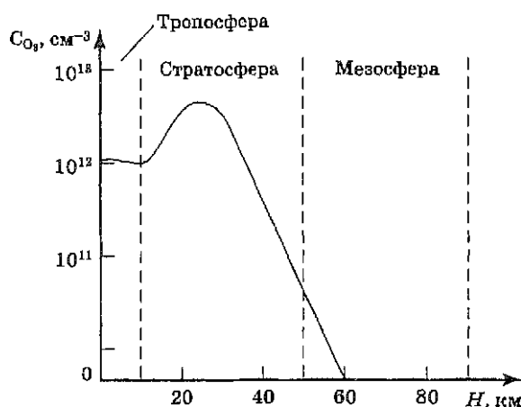
Рис. 7.7. Распределение озона в атмосфере
