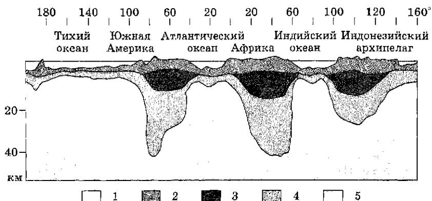
Рис. 7.3. Схема строения земной коры в экваториальном разрезе: 1 — океаническая вода; 2 — осадочные породы; 3 — граниты; 4 — базальты; 5 — мантия
