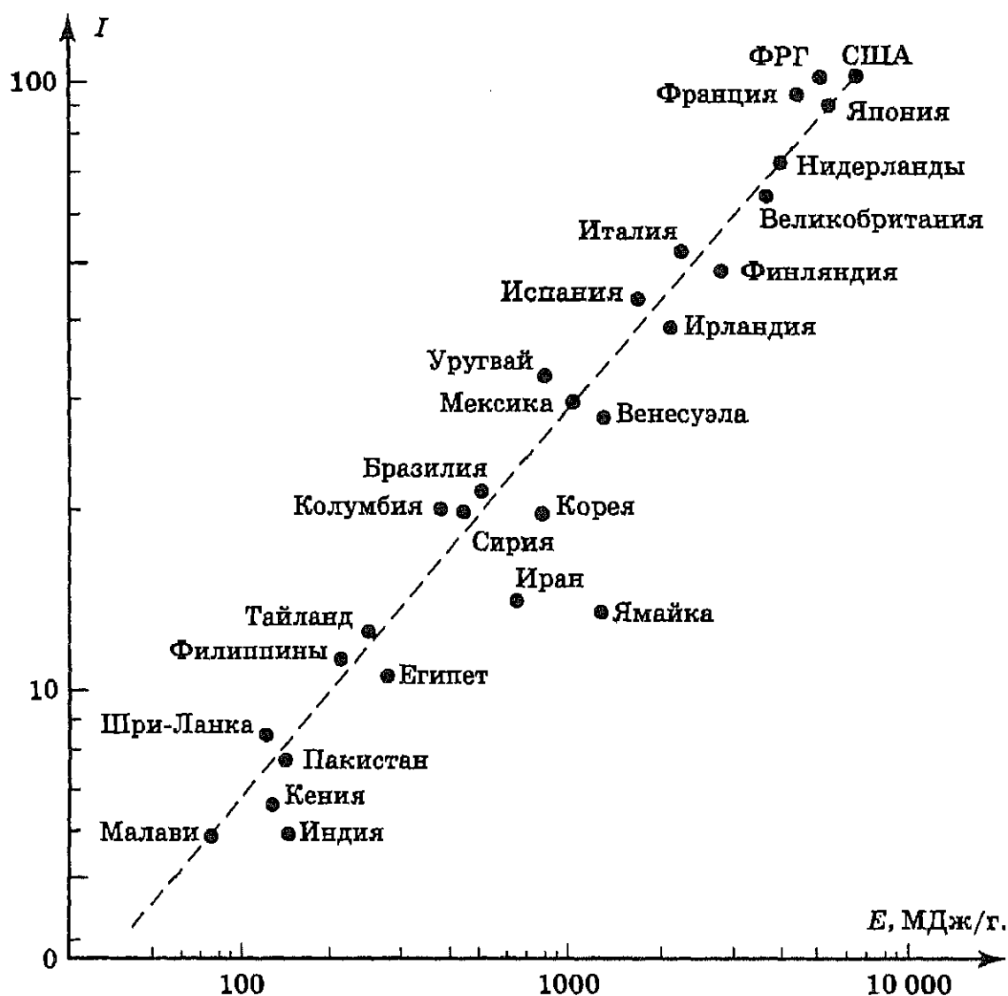
Рис. 9.16. Взаимосвязь уровня потребления энергии и уровня жизни населения в 1980 г. (по Т. А. Акимовой, В. В. Хаскину): I — индекс чистого дохода, вычисленный по действительной стоимости большого набора товаров и услуг ( I = 1 соответствует приблизительно 22,5 долл. США); E — потребление энергии на одного жителя разных стран в кг угольного эквивалента (29,3 МДж/г)
