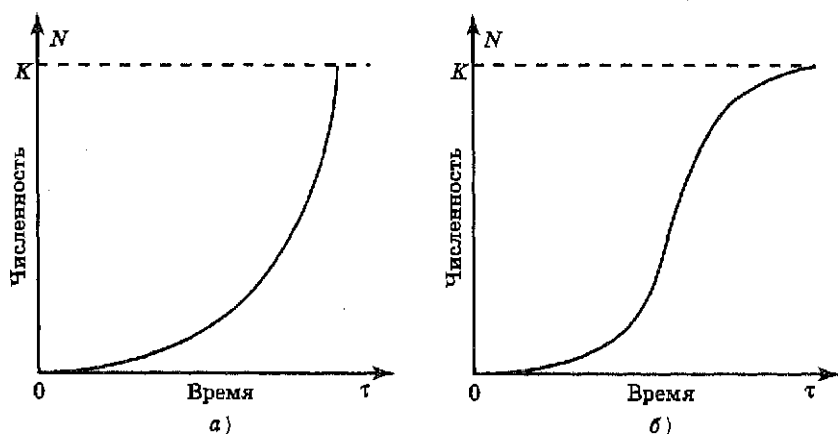
Рис. 4.5. Типы кривых роста численности популяции (модели роста популяции): а — J-образная; б — S-образная; K — поддерживающая емкость среды
