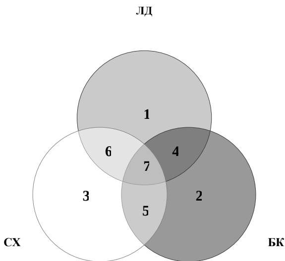
Рис. 2.2.1. Эколого-геологическая система
