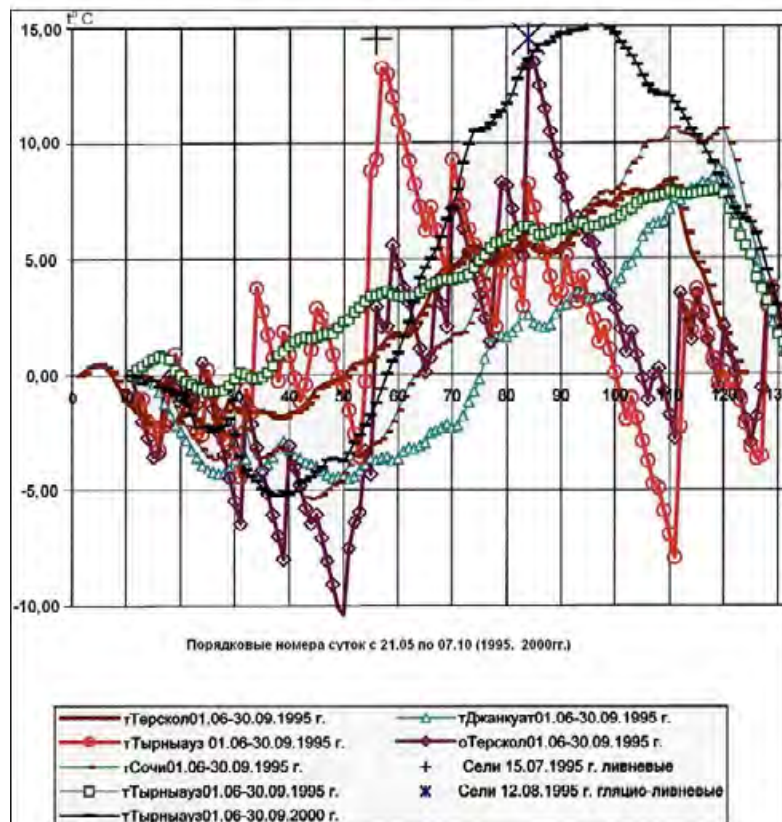
Рис. 3 - График суммы аномалий суточной температуры воздуха.
