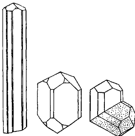
Рис. 18. Кристаллы рутила
