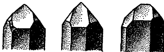
Рис. 24. В кристаллах кварца различны форма, размеры, число граней, но углы между соответствующими гранями остаются постоянными
