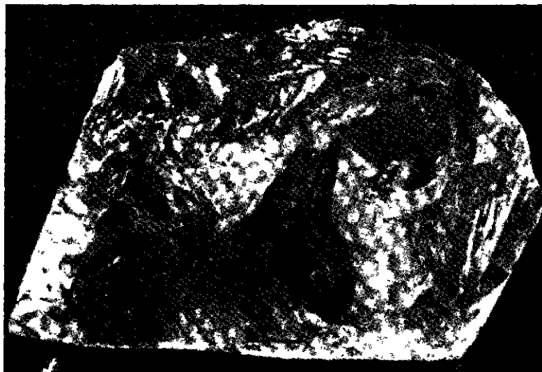
Рис. 3. Крупнейший алмаз «Куллинан» в натуральную величину
