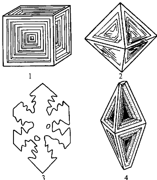
Рис. 25. Формы некоторых минералов («скелетные»), выросших при недостатке питания: 1 — галит, 2 — алмаз, 3 — кварц, 4 — сера
