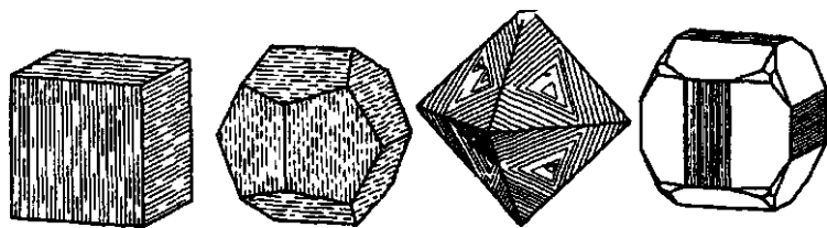
Рис 17 Кристаллы пирита
