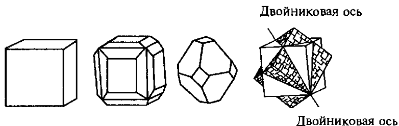
Рис. 21. Одиночные кристаллы и — справа — двойник флюорита
