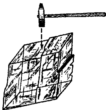
Рис. 29. Спайность кальцита, совершенная в трех направлениях
