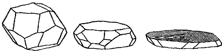
Рис 9 Кристаллы гематита
