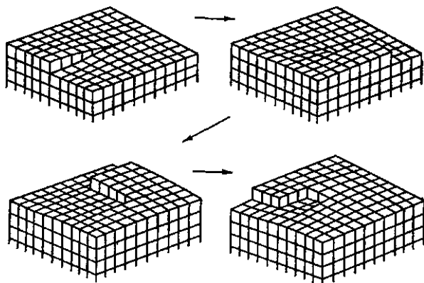
Рис. 27. Схема роста кристалла по спирали
