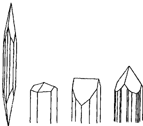
Рис. 5 Кристаллы антимонита
