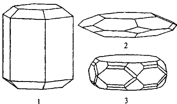
Рис. 6. Три кристалла апатита 1 — призматический, 2 и 3 — таблитчатые
