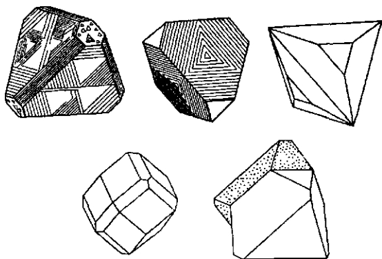
Рис. 20. Кристаллы сфалерита
