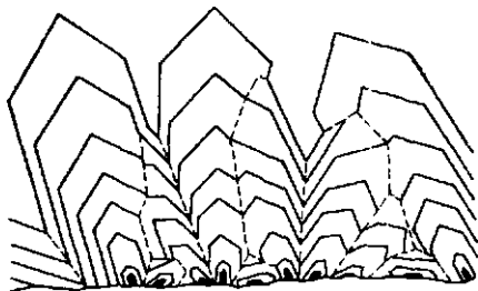
Рис. 26. «Геометрический отбор» кристаллов: получают преимущество те, которые быстрее растут, активнее «питаются»
