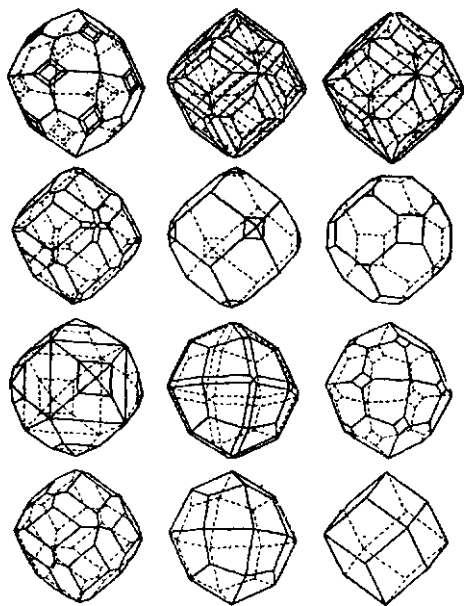
Рис. 10 Формы кристаллов граната
