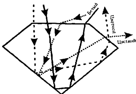
Рис 7 Путь световых лучей в бриллианте
