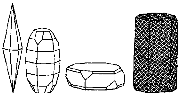
Рис 14 Кристаллы корунда
