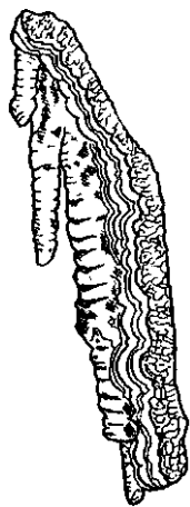
Рис. 15. Малахитовые сталактиты
