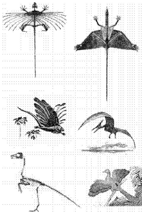
РИСУНОК 47. Завоевание воздуха рептилиями: планеры из числа триасовых низших диапсид (а-в), птерозавры (г) и предки птиц (д-е). (а) - Icarosaurus siefkei , (б) - Sharovipteryx mirabilis , (в) - Longisquama insignis , г - птеранодон, д - протоавис, е - археоптерикс.
