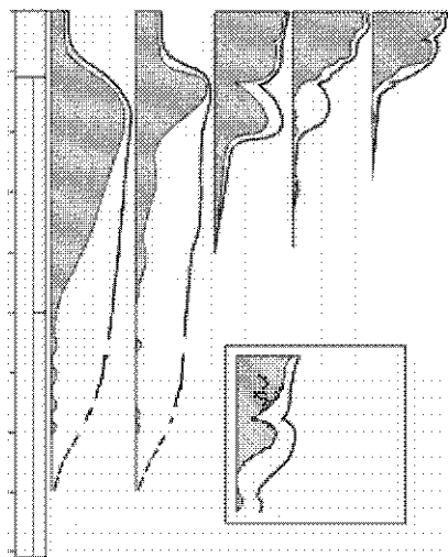
РИСУНОК 19. Изменения во времени относительного обилия основных биотических компонентов: (а) - прокариоты-строматолитообразователи, (б) - свободноживущие прокариоты, (в) - эукариотный фитопланктон, (г) - многоклеточные растения, (д) - многоклеточные животные.
