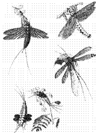
РИСУНОК 35. Растительный мир каменноугольного периода - заболоченный карбоновый лес (а) и растения, характерные для тропической Евразийской (б-г) и внетропической Ангарской (д-е) и Гондванской (ж) областей: (б) - лепидодендрон (плаунообразное), (в) - каламит (хвощеобразное), (г) - древовидный папоротник Eospermatopsis , (д) - лоблодия и томиодендрон (плаунообразные), (е) - кордаиты (хвойные), (ж) - глоссоптерис (гинкговое).
