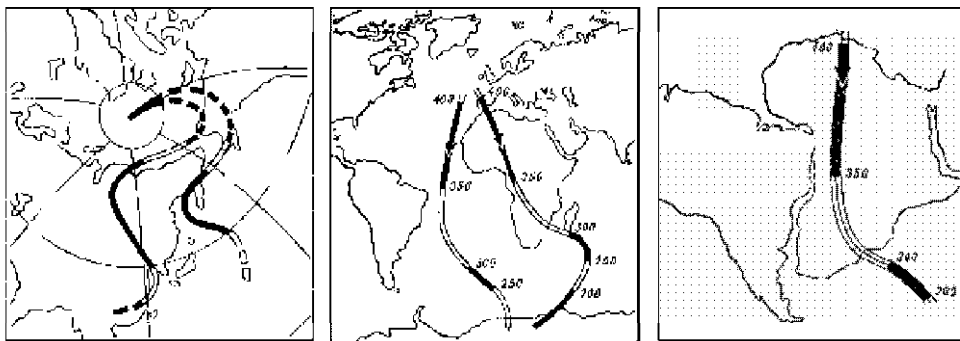
РИСУНОК 7. Траектории движения полюса относительно континентов при их современном расположении: (а) - Северного относительно Европы и Северной Америки, (б) - Южного относительно Африки и Южной Америки. (в) - те же траектории, но при совмещении приатлантических частей
