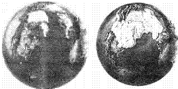
РИСУНОК 58. Оледенение Северного полушария в наши дни (а) и в последнюю ледниковую эпоху (б).
