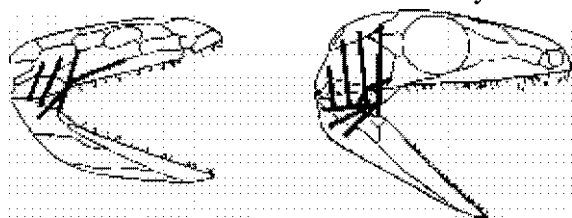
РИСУНОК 37. Расположение жевательной мускулатуры лабиринтодонта Ichthyostega (а) и примитивной капторинорморфной рептилии Paleothyris (б).
