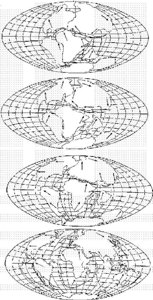
РИСУНОК 9. (а) - аномалии величины напряженности магнитного поля в районе Срединно-Атлантического хребта; (б) - карта значений карта возраста дна Северной Атлантики.
