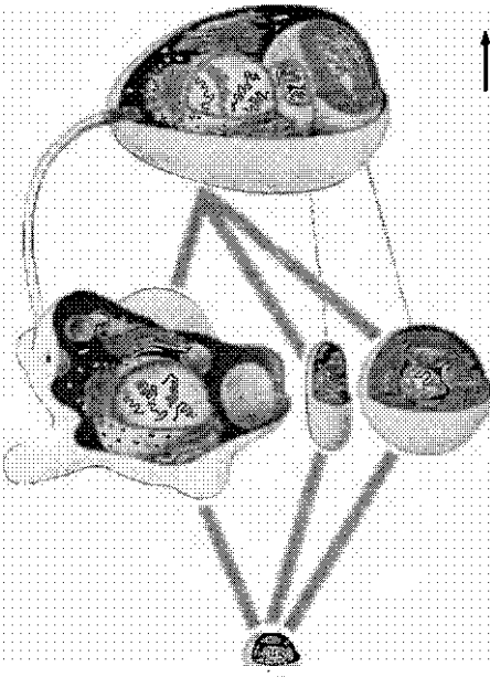
РИСУНОК 18. Схематическое изображение симбиогенеза.
