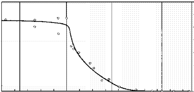
РИСУНОК 51. Эволюция насекомых в мезозое: процент вымерших семейств от общего числа семейств насекомых в поздне-мезозойских и кайнозойских фаунах.
