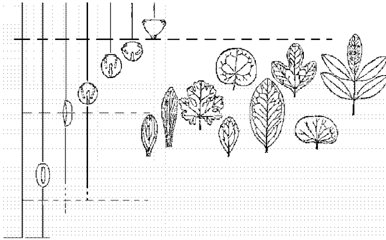
РИСУНОК 50. Распределение в меловых отложениях основных типов пыльцы и листьев покрытосеменных.
