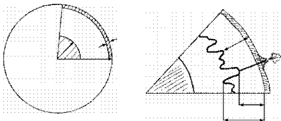
РИСУНОК 4. Структура недр планеты (со схематическим вулканом)
