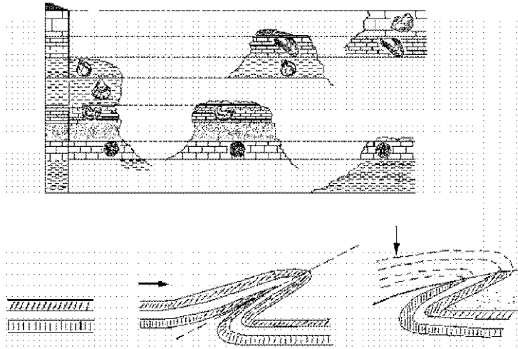
РИСУНОК 1. а - составление сводной стратиграфической шкалы на 5 разрезах; б - образование запрокинутого залегания (линия, складка и эрозия "нормальной" половинки).
