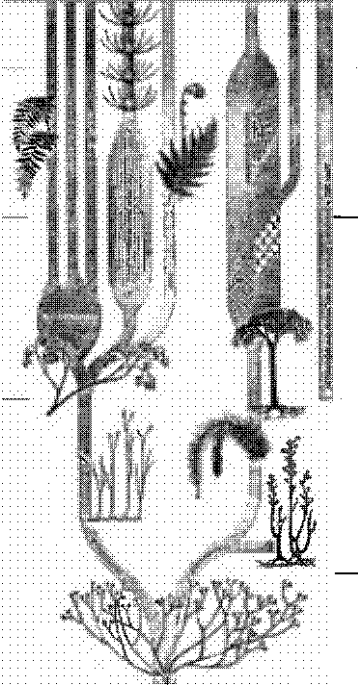
РИСУНОК 30. Родословное дерево первых наземных растений.
