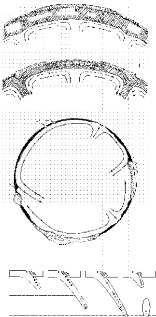
РИСУНОК 8. (а) - раздвижение литосферных плит с "впаянными" в них континентами в результате конвективных токов в мантии, выходящих на поверхность в рифтовой зоне срединно-океанического хребта. (б) - Пододвигание литосферной плиты под континент с возникновением вулканизма и глубоководных землетрясений.
