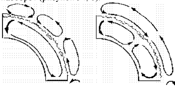
РИСУНОК 34. Циркуляция в атмосфере и гидросфере: схема термической и галинной циркуляции в океанах: (а) - криоэра, (б) - термоэра.
