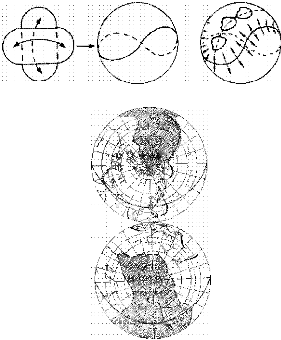
РИСУНОК 12. (а) - теннисный мяч, состоящий из двух лоскутов; (б) - схема поверхности планеты, имеющей две конвективные ячейки: "шов" - линия подъема мантийного вещества (срединно-океанические хребты), материки выстраиваются вдоль линии опускания мантийного вещества (оси каждого из лоскутов); (в) - поверхность современной Земли (заштрихован американо-антарктический "лоскут").
