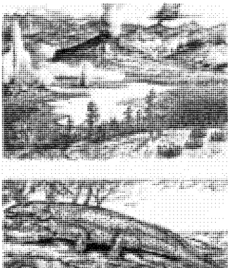
РИСУНОК 29. (а) - Реконструкция ландшафта Райни (девон Шотландии) с зарослями псилофитов; (б) - древнейшее наземное позвоночное - ихтиостега (девон Гренландии).
