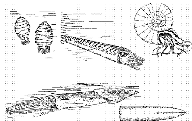
РИСУНОК 27. Палеозойские и мезозойские головоногие: (а) - исходная жизненная форма головоногих (архаичная наутилоидея Mandaloceras ); (б) - прямое головоногое (наутилоидея Michelinoceras ); (в) - свернутое головоногое (аммонит); (г) - внутреннераковинное головоногое (белемнит и его раковинвина - "чертов палец").
