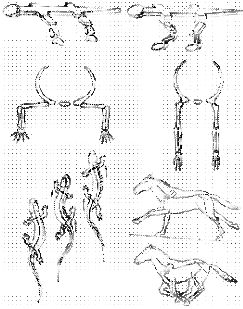
РИСУНОК 43. а - Положение конечностей в латеральном и парасагитальном положении; б - "рептильный" и "маммальный" шаг.
