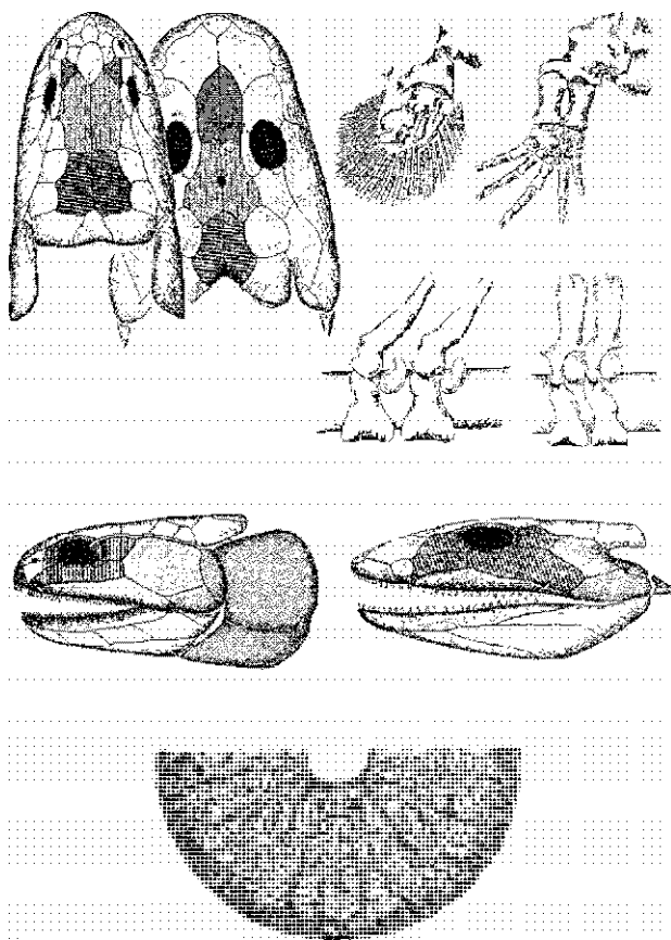
РИСУНОК 31. Преемственность анатомических структур (череп, конечности и позвонки) кистеперых рыб и амфибий: идентичные кости черепа имеют одинаковую заливку; идентичные кости обозначены одинаковыми буквами; отдельно - поперечный шлиф половинки зуба лабиринтодонта.
