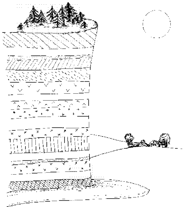
РИСУНОК 3. Соответствие стратиграфических и временных подразделений.
