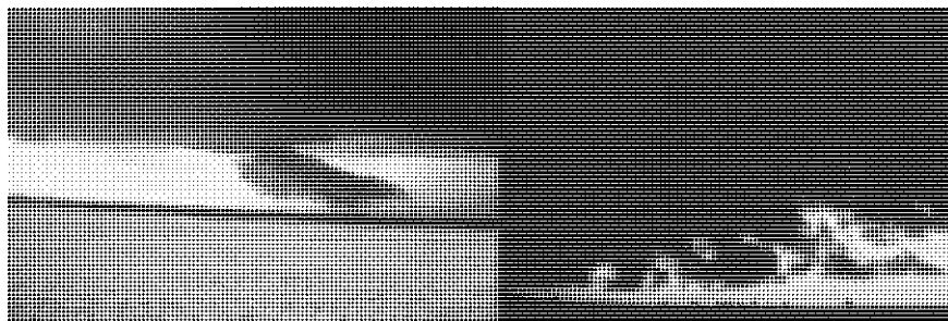
Рис. 12. Разорванные облака у основания тучи
