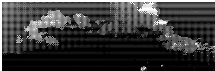
Рис. 9. Множество облаков всех ярусов
