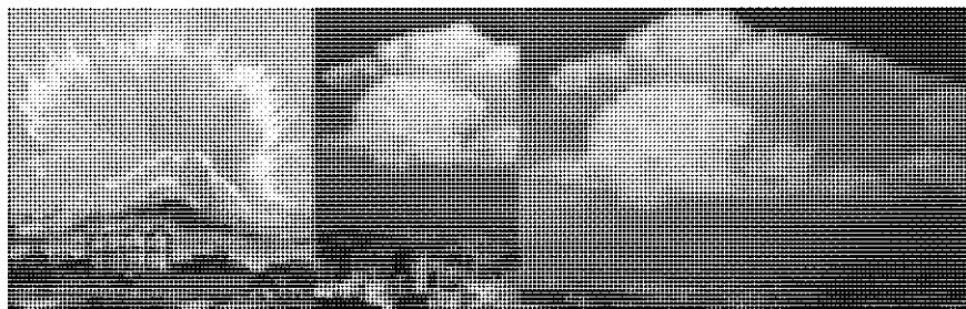
Рис. 10. Так выглядят грозовые облака
