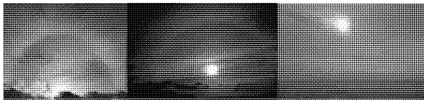
Рис. 5. Перисто-слоистые облака, сначала образующие вокруг солнца и луны большие круги (два левых рисунка), а затем — по мере уплотнения — закрывающие небо словно масляной бумагой (правый рисунок).
