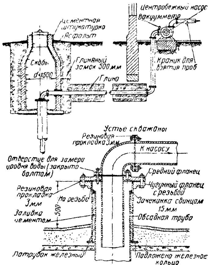
Рис. 17. Шахтнад скважиной и устье при центробежном насосе, расположенном в насосной станции
