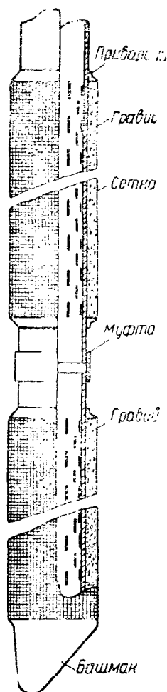
Рис. 28. Гравийный фильтр Спренера
