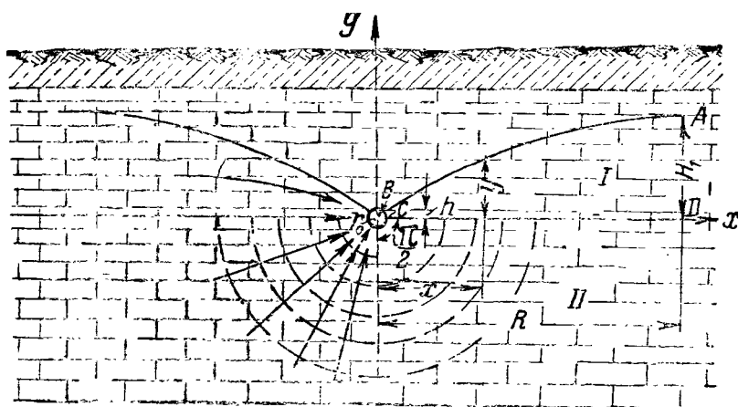
Рис. 80. Схема притока воды к дренажу в трещиноватых породах при глубоком залегании водоупора
