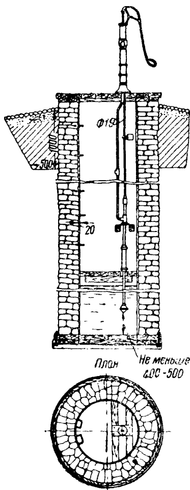
Рис. 54. Каменный колодец
