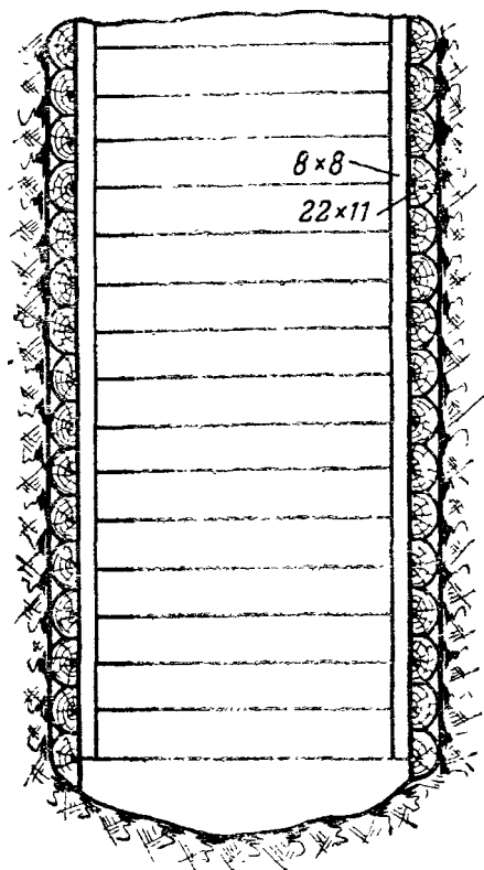
Рис. 45. Проходка шахты „сходом“
