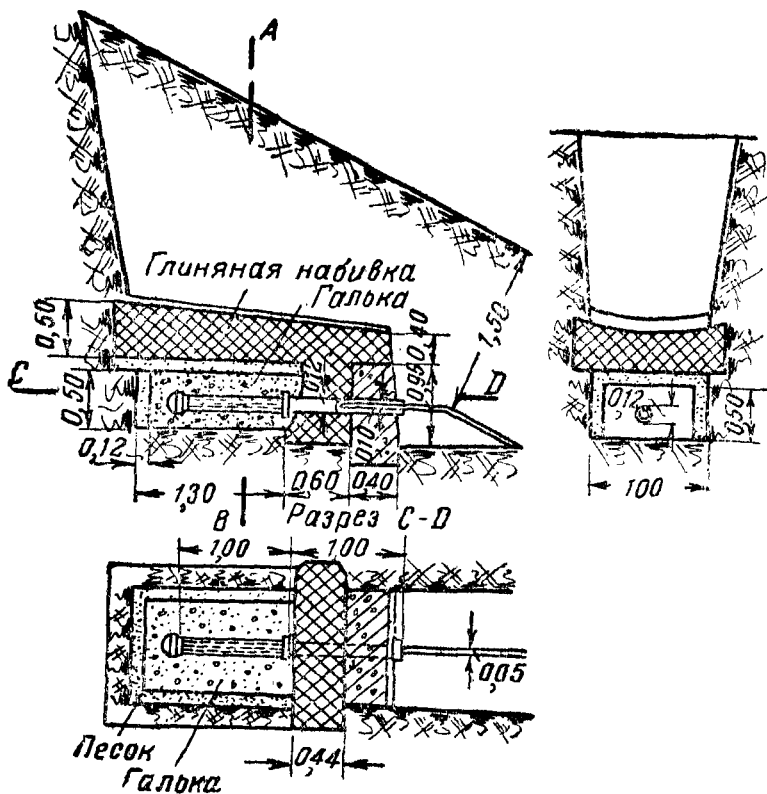
Рис. 91. Простейший тип каптажа нисходящего источника, приуроченного к песчаным породам
