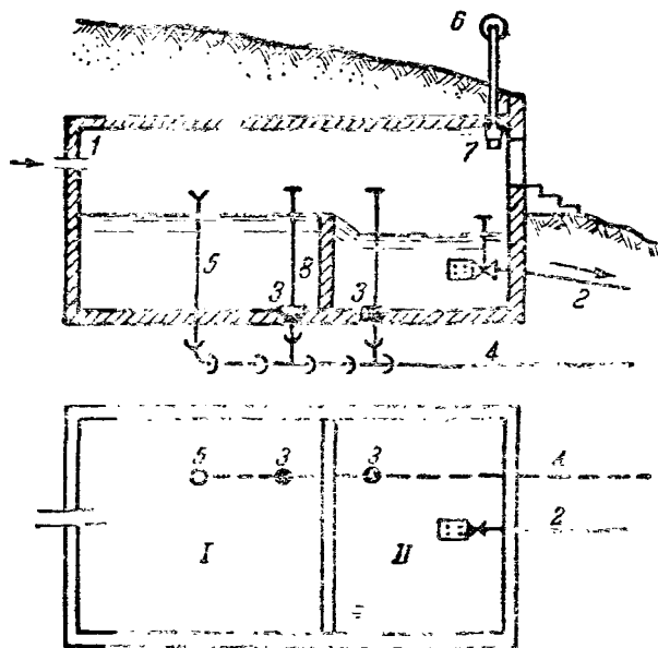
Рис. 76. Водосборный резервуар:
