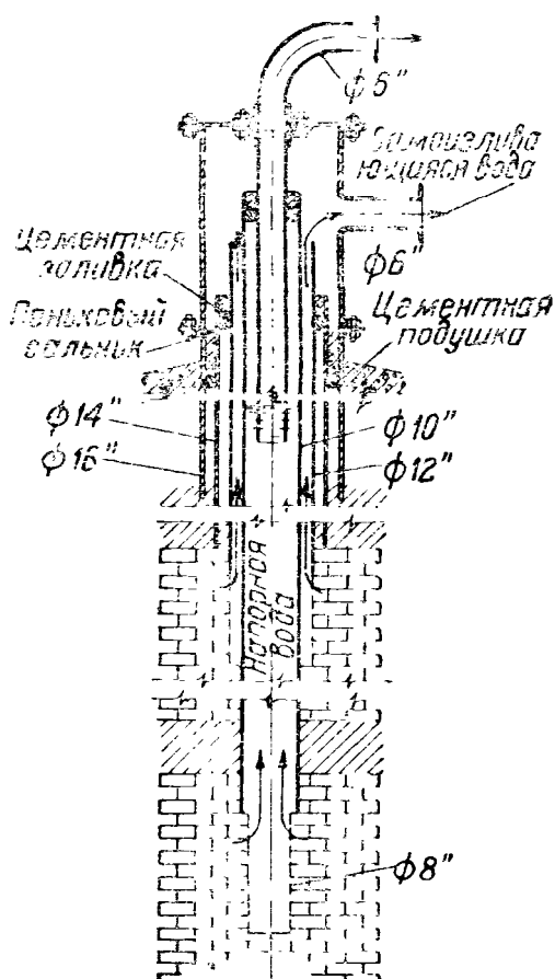
Рис. 21. Схема оборудования оголовка скважины для раздельной эксплуатации двух фонтанирующих водоносных горизонтов
