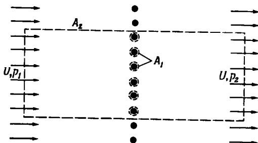
Р и с. 5.15.1. Использование теоремы о количестве движения для определения силы, действующей на решетку твердых тел.
