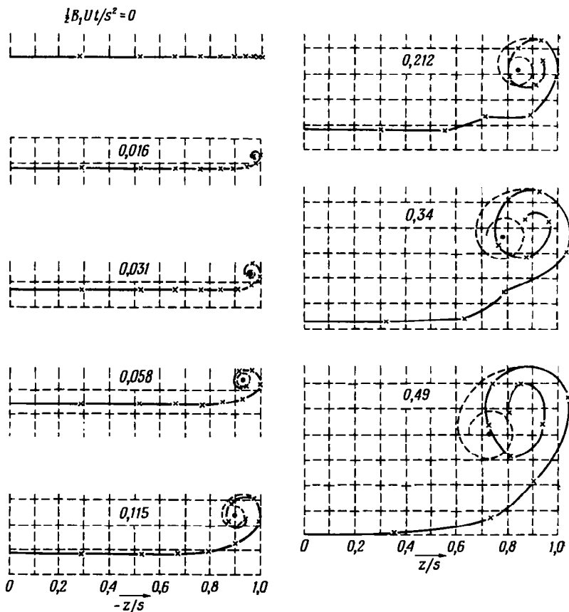
Рис. 7.8.5. Расчетные положения группы из десяти одинаковых точечных вихрей, расположенных при t = 0 вдоль прямой линии таким образом, чтобы приблизительно представить половину вихревой пелены эллиптически нагруженного крыла (см. (7.8.12)). Штриховые линии получены аналитическим путем для течения вблизи края вихревой пелены (помеченного точкой), где численное интегрирование становится невозможным (Вестуотер (1936)).
