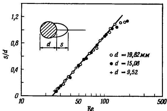
Р и с. 4.12.9. Наблюдаемые размеры области замкнутых линий тока за сферой (Танеда (19566)).
