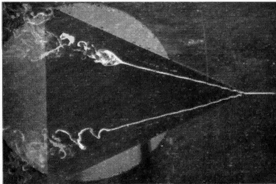
Фото 7.5.7. «Взрыв» вихрей в воде. Две полосы краски располагаются вдоль осей интенсивных вихрей, сходящихся с боков треугольного крыла (Ламбурн и Брайер (1962)).
