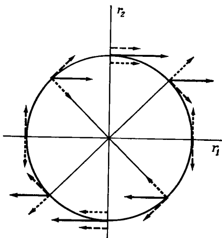
Р и с. 2.3.1. Простое движение сдвига вблизи точки, разложенное на чисто деформационное движение и вращение. Главные оси деформационного движения наклонены под углами 45^\circ к осям r_1 и r_2 . Результирующее движение обозначено сплошными стрелками, деформационное — пунктирными стрелками, а вращение — штриховыми.
