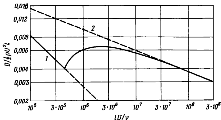
Р и с. 5.8.2. Полная сила трения D на единицу ширины гладкой плоской пластины длины l в потоке со скоростью U . Кривая линия перехода имеет форму, типичную для экспериментальных наблюдений, но ее положение на графике зависит от условий опыта. 1 — полностью ламинарный пограничный слой; 2 — полностью турбулентный пограничный слой.
