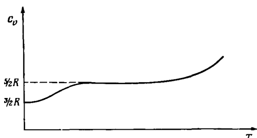
Р и с. 1.7.1. Зависимость удельной теплоемкости газа от температуры для многоатомной молекулы.
