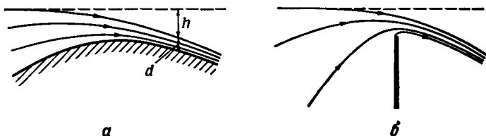
Р и с. 6.3.3. Установившееся течение над гребнем плотины. а — плотина с закругленным широким гребнем; б — плотина с острым гребнем.
