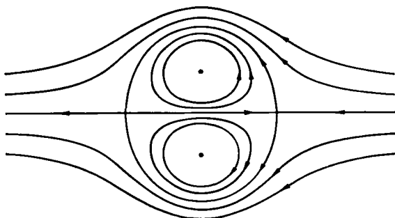
Р и с. 7.3.3. Линии тока установившегося течения относительно пары точечных вихрей с интенсивностями \kappa_1 = \kappa и \kappa_2 = -\kappa .
