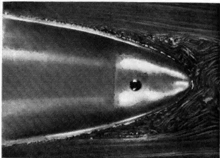
Фото 5.10.1. Отрыв установившегося пограничного слоя на кормовой части поверхности тела вращения в потоке воды. Число Рейнольдса (по длине тела) равно 1,3 \cdot 10^6 . Поверхность воды, являющаяся плоскостью симметрии тела, была сделана видимой с помощью алюминиевого порошка (Клаттер, Смит и Брэзнер (1959)).
