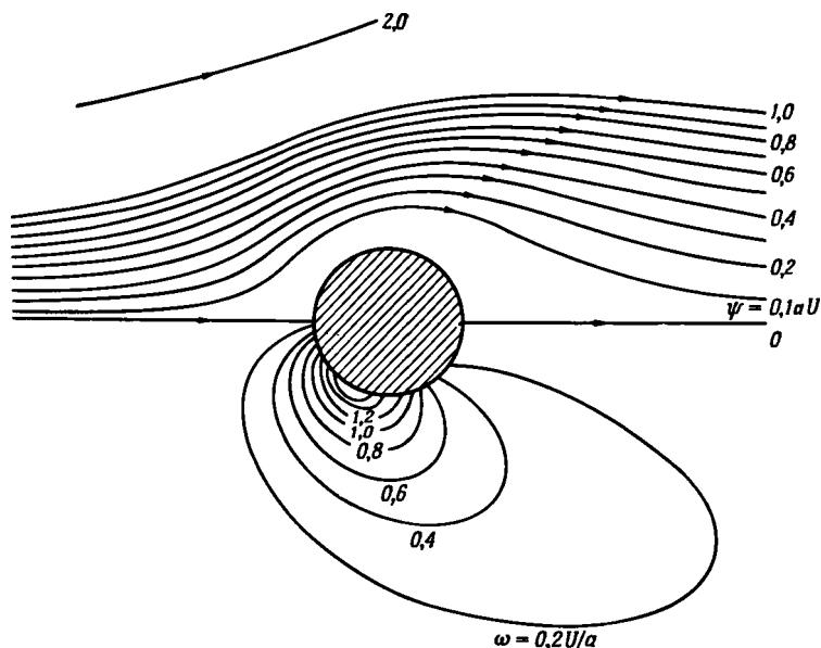
Р и с. 4.12.2. Линии тока (вверху) и линии постоянной завихренности (внизу) для обтекания кругового цилиндра при числе Рейнольдса Re = 4 (расчет Келлера и Таками (1966)).
