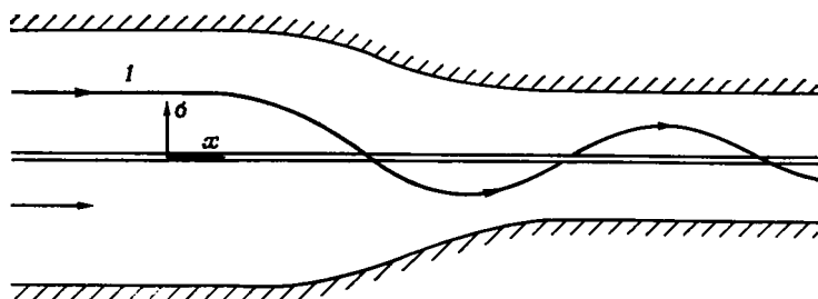
Р и с. 7.5.4. Превращение прямолинейной вихревой линии в спиральную при прохождении сужения трубы. 1 — вихревая нить.
