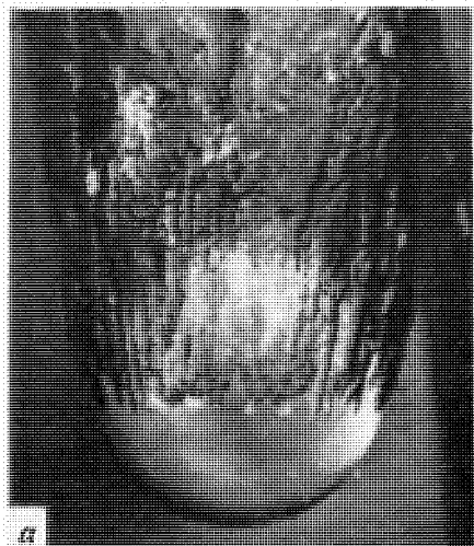
Фото 6.12.7. Фотографии сферы диаметром 22 см, входящей в воду со скоростью 64 см/сек; а — гладкая поверхность; б — в передней части сферы имеется небольшой участок песочной шероховатости, которая предположительно турбулизирует пограничный слой на сфере (фотографии ВМС США). Сравните с аналогичным эффектом в потоке без каверны, фото 5.11.7.
