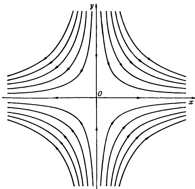
Р и с. 2.7.2. Линии тока двумерного безвихревого соленоидального течения вблизи критической точки, \psi = kxy .
