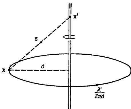
Р и с. 2.6.1. Соленоидальное распределение скоростей течения, создаваемого прямолинейной вихревой нитью интенсивности \kappa .
