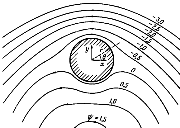
Рис. 7.4.1. Схема линий тока в двумерном течении, обусловленном неподвижным круговым цилиндром, помещенным во вращающуюся жидкость; \omega_0 a/U = 1/2 , \kappa/aU = 0 .
