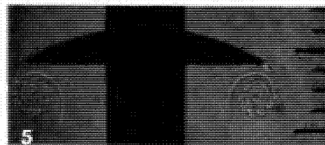
Фото 5.10.5. Серия теневых фотографий, сделанных через интервалы времени около 1,1 \cdot 10^{-3} сек (между последними двумя снимками интервал времени удвоен), показывающая положение пара, сходящего с поверхности осесимметричного тела с точкой излома; тело из состояния покоя приведено в движение в воздухе с постоянной скоростью 731 см/сек. На правой стороне каждого снимка указана неподвижная шкала с делениями через 0,63 см (Пирс (1961)).
