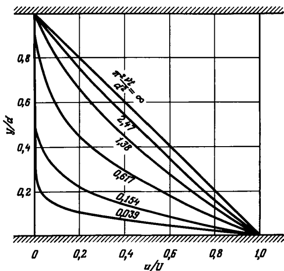
Р и с. 4.3.2. Развитие из состояния покоя установившегося течения между параллельными пластинами при их относительном движении.
