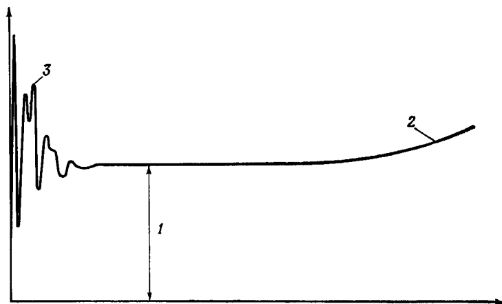
Р и с. 1.2.1. Влияние величины объема на плотность, измеряемую прибором в этом объеме. По оси абсцисс: объем жидкости, к которому относится измерение; по оси ординат: измеряемая плотность.
