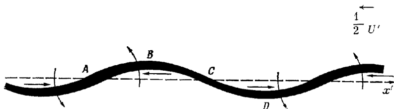
Рис. 7.1.3. Рост синусоидального возмущения в первоначально однородной вихревой пелене, имеющей положительную завихренность в направлении по нормали к плоскости чертежа. Локальная плотность напряженности пелены соответствует на рисунке толщине пелены. Стрелки показывают направление самоиндуцированного движения завихренности в пелене и объясняют (а) накопление завихренности в точках, подобных точке А, а также (б) возникновение вращения жидкости вокруг этих точек. Оба указанных эффекта приводят к экспоненциальному росту возмущения.
