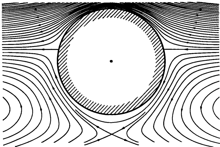
Р и с. 7.4.2. Линии тока двумерного течения, обусловленного неподвижным круговым цилиндром, помещенным в простое двумерное течение сдвига; \omega_0 a/U = 1 , \kappa/aU = 0 (Тзян (1943)).
