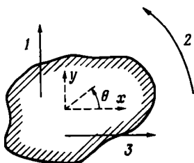
Р и с. 6.4.1. Схема к расчету силы, действующей на тело в установившемся поступательном движении при двумерном поле скоростей.
