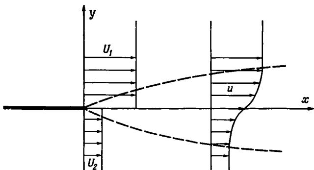
Р и с. 5.12.1. Установившийся переходный слой между двумя параллельными потоками, приведенными в соприкосновение при x = 0 .
