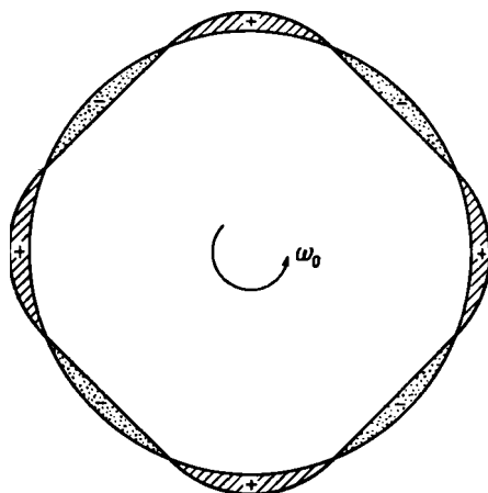
Рис. 7.3.2. Несимметричная составляющая распределения завихренности в случае, когда на круговое ядро постоянной завихренности \omega_0 наложено возмущение ( s = 4 ).
