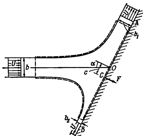
Р и с. 6.3.4. Струя жидкости, ударяющаяся о наклонную плоскую стенку (двумерный случай).
