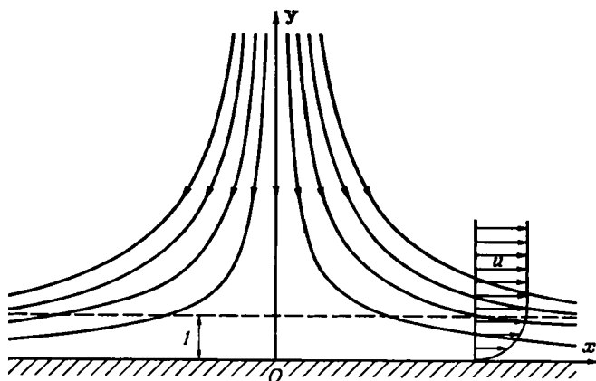
Р и с. 5.5.1. Установившееся двумерное течение в окрестности критической точки на твердой границе.
