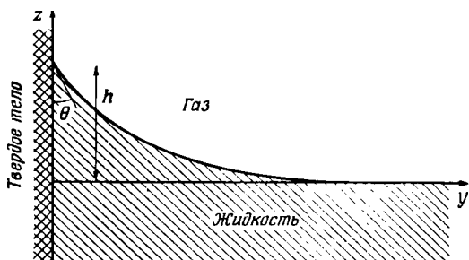
Р и с. 1.9.2. Свободная поверхность жидкости на границе с вертикальной плоской стенкой.
