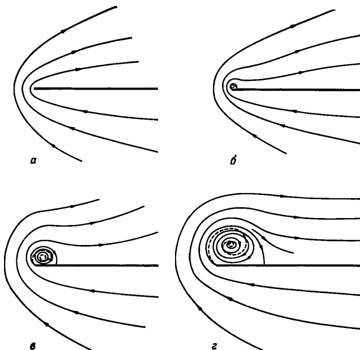
Р и с. 6.7.3. Схема линий тока при обтекании острой кромки пластины на различных стадиях после начала движения; а — полностью безвихревое течение, определяемое комплексным потенциалом w(z) = Az^{1/2} ; б, в, г — то же безвихревое течение, измененное наличием в нем спиральной вихревой пелены (штриховая линия), которая содержит завихренность, сходящую с пограничных слоев на обеих поверхностях пластины (преобладает отрицательная завихренность с нижней поверхности пластины).
