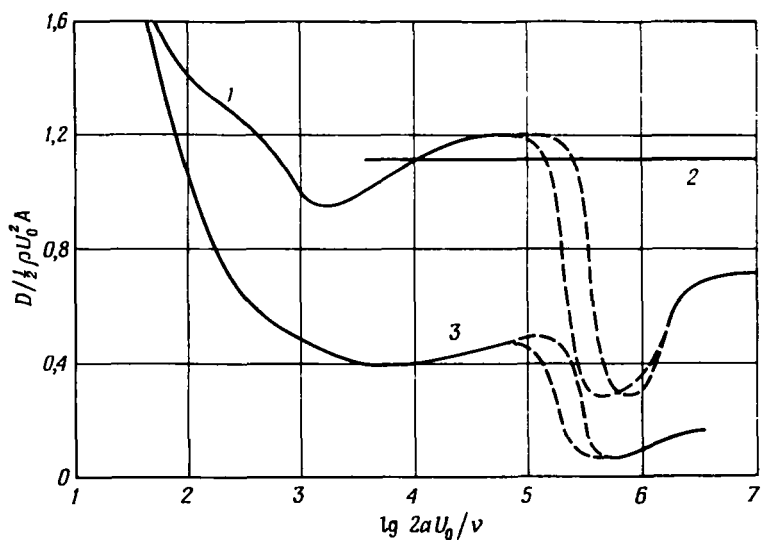
Р и с. 5.11.6. Измеренное сопротивление кругового цилиндра на единицу длины ( A = 2a ), сферы ( A = \pi a^2 ) и кругового диска, нормального к потоку ( A = \pi a^2 ); все тела имеют одинаковый радиус a . Штриховыми линиями показаны результаты, полученные в различных аэродинамических трубах.
