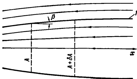
Р и с. 6.9.1. Осесимметричное безвихревое обтекание тонкого тела, представляемое распределением источников на его оси. 1 — поверхность тела.
