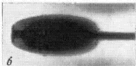
Фото 6.12.5. Стационарные каверны при K = 0,19 на круговом диске, расположенном нормально к потоку воды; а — давление в каверне поддерживается путем непрерывного подвода воздуха в каверну; б и в — каверны без подвода воздуха. Снимок б получен с выдержкой 2 сек, а снимок в — с выдержкой 10–6 сек. Асимметрия кормовой части каверны объясняется влиянием плавучести (фотографии ВМС США).
