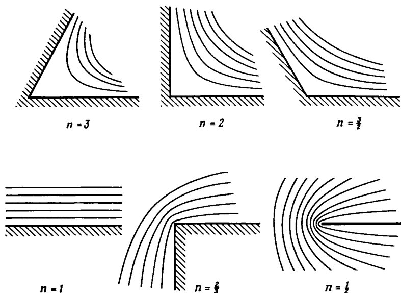
Р и с. 6.5.1. Безвихревое течение в области между двумя прямолинейными твердыми границами, пересекающимися под углом \pi/n .
