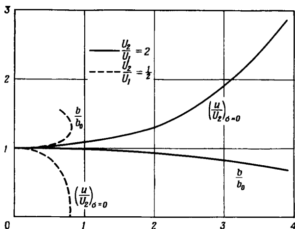
Рис. 7.5.5. Свойства вихрей при увеличении или уменьшении осевой скорости. По оси абсцисс отложены значения величины ka .
