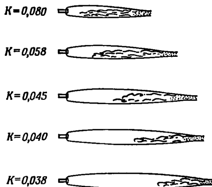
Р и с. 6.13.5. Стационарные каверны, присоединенные к круглому диску при положительных числах кавитации (Рейхардт (1946)).
