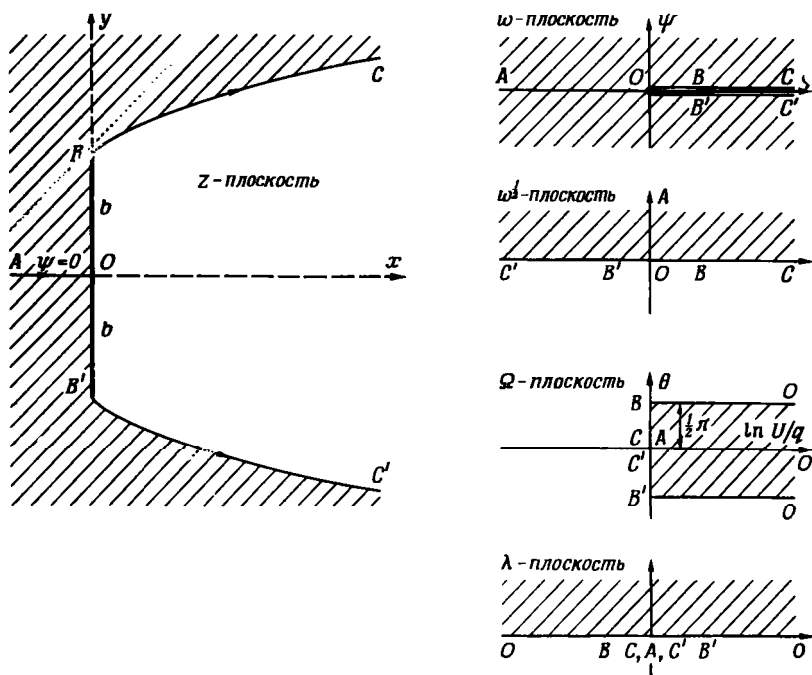
Р и с. 6.13.2. Конформные преобразования, используемые для определения обтекания плоской пластины с наветренной под давлением окружающей среды.
