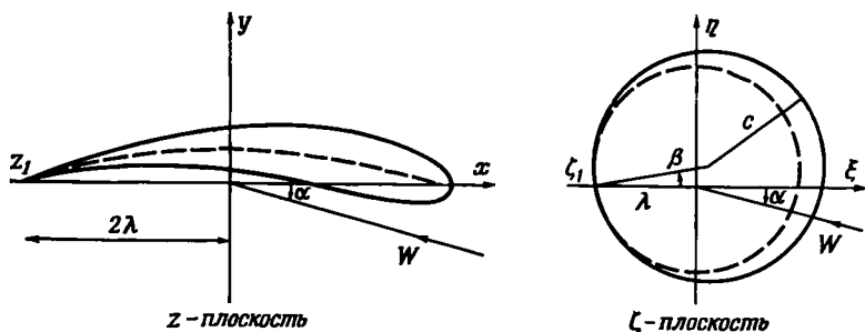
Р и с. 6.7.9. Преобразования круга в дугу окружности (штриховая линия) и в изогнутый профиль Жуковского (сплошная линия).
