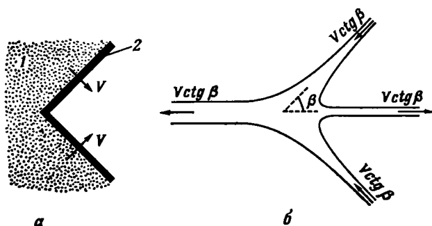
Рис. 6.3.5. Конический кумулятивный заряд. Справа скорости изображены в осях, движущихся вместе с вершиной конуса. 1 — взрывчатое вещество; 2 — полый металлический конус.
