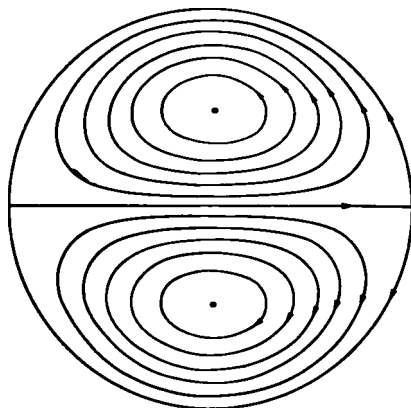
Р и с. 7.3.4. Линии тока в области r \leq a для установившегося течения, обусловленного завихренностью, пропорциональной J_1 (kr) \sin \theta ( r \leq a , ka = 3,83 ), и однородным потоком с подходящей скоростью на бесконечности.
