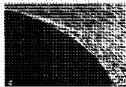
Фото 5.9.3. Последовательные стадии нарастания пограничного слоя на кормовой части плохообтекаемого тела, которое начало двигаться из состояния покоя. Наблюдатель неподвижен относительно тела; движение жидкости происходит слева направо (Прандтль и Титъенс (1935)).
