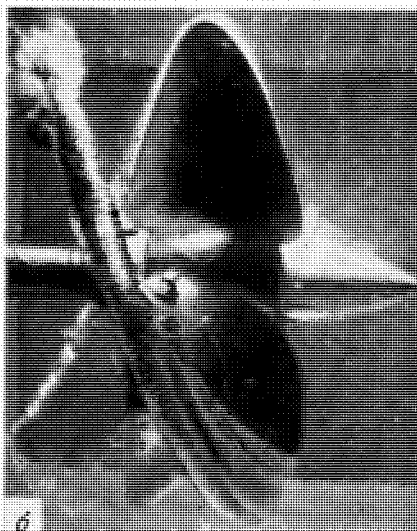
Фото 6.12.2. Кавитация, создаваемая винтом, который вращается в потоке воды (справа налево). а — каверна возникает внутри концевых вихря от каждой из трех лопастей; б — при более высоких скоростях вращения и потока на стороне разрежения каждой лопасти также наблюдается каверна, объем которой достаточно велик, чтобы влиять на распределение давления по лопасти.
