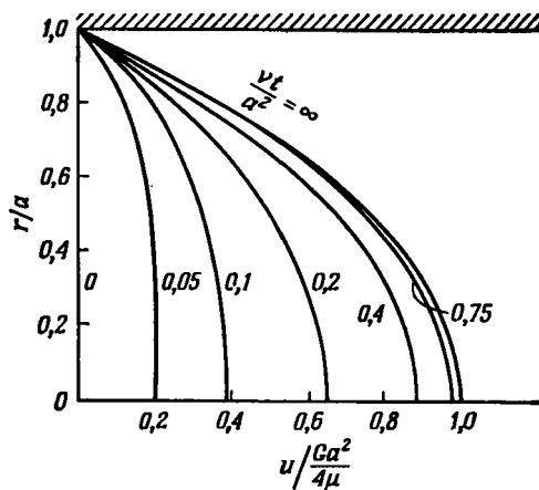
Р и с. 4.3.3. Течение в начальном участке круглой трубы. Профили скорости в различные моменты времени (Шиманский (1932)).
