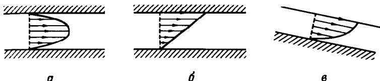
Р и с. 4.2.1. Установившееся двумерное течение: а — под действием градиента давления между двумя неподвижными твердыми плоскостями; б — вызванное относительным движением двух твердых плоскостей; в — в слое на наклонной плоскости, вызванное действием силы тяжести.
