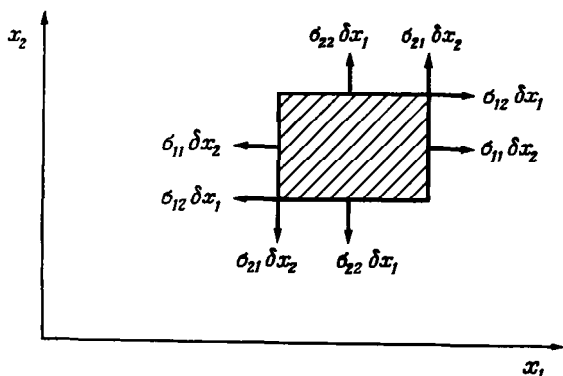
Р и с. 1.3.2. Поверхностные силы, действующие на прямоугольный элемент жидкости единичной толщины.
