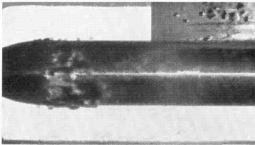
Фото 6.12.1. Образование каверн при обтекании (слева направо) осесимметричного тонкого тела в гидродинамической трубе при K = 0,26 (Кнап (1952)).
