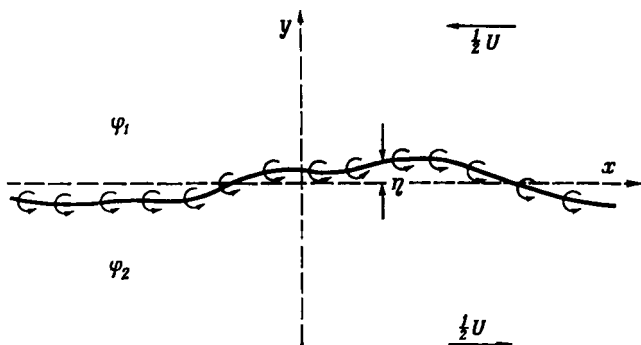
Р и с. 7.1.2. Схема возникновения неустойчивости плоской вихревой пелены по отношению к малому возмущению.
