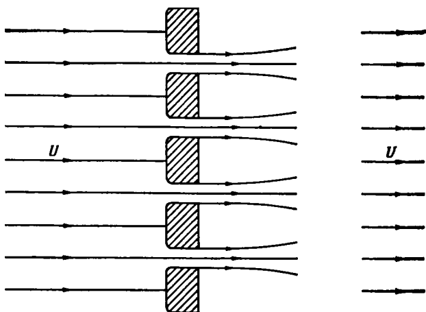
Рис. 5.15.3. Расчет сопротивления перфорированной пластины в однородном потоке.
