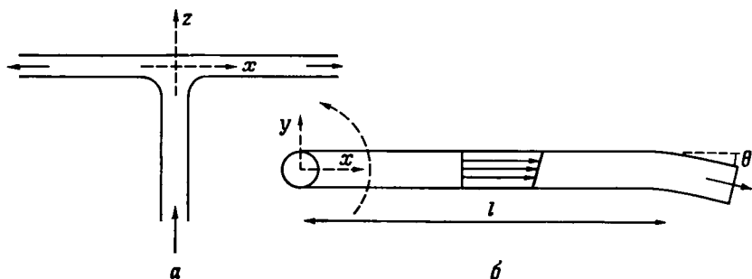
Рис. 6.3.6. Течение в колене трубы, вращающейся относительно оси z .
