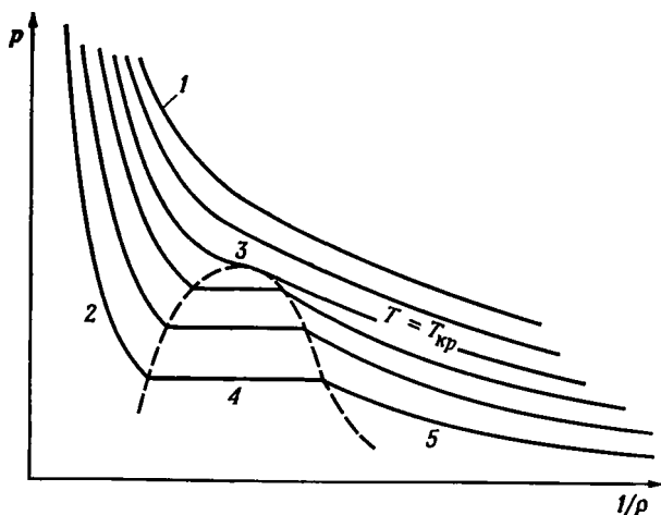
Р и с. 1.8.1. Изотермы типичных паро-жидкостных систем.
