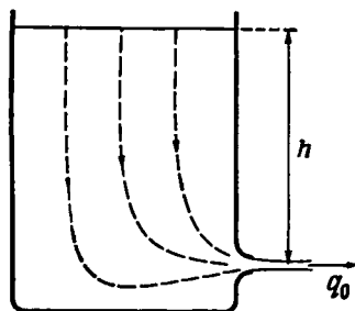
Р и с. 6.3.1. Истечение из отверстия в открытом сосуде.
