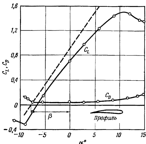
Р и с. 6.7.10. Измеренные величины подъемной силы и силы сопротивления изогнутого профиля Жуковского в зависимости от угла атаки (по Бетцу (1915)); штриховая линия соответствует теоретическому значению коэффициента подъемной силы.
