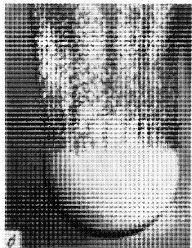
Фото 6.12.7. Фотографии сферы диаметром 22 см, входящей в воду со скоростью 64 см/сек; а — гладкая поверхность; б — в передней части сферы имеется небольшой участок песочной шероховатости, которая предположительно турбулизирует пограничный слой на сфере (фотографии ВМС США). Сравните с аналогичным эффектом в потоке без каверны, фото 5.11.7.
