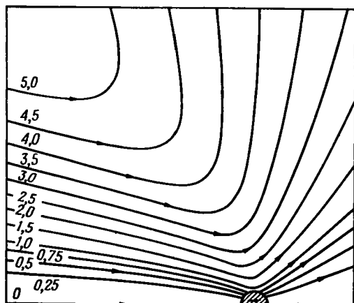
Рис. 4.10.1. Линии тока в осевой плоскости для внешней части течения, вызванного движущейся сферой, согласно уравнениям Озеена. Функция тока \psi равна произведению некоторой постоянной, умноженной на число, указанное на линиях тока.
