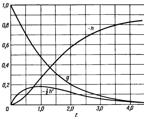
Р и с. 5.5.3. Безразмерные функции, определяющие компоненты скорости течения, вызванного вращающимся диском.
