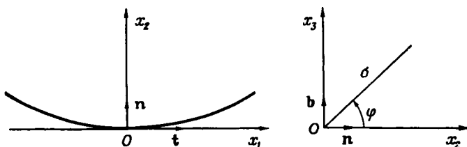
Р и с. 7.1.1. Схематическое определение индуцированной скорости вблизи вихревой нити.
