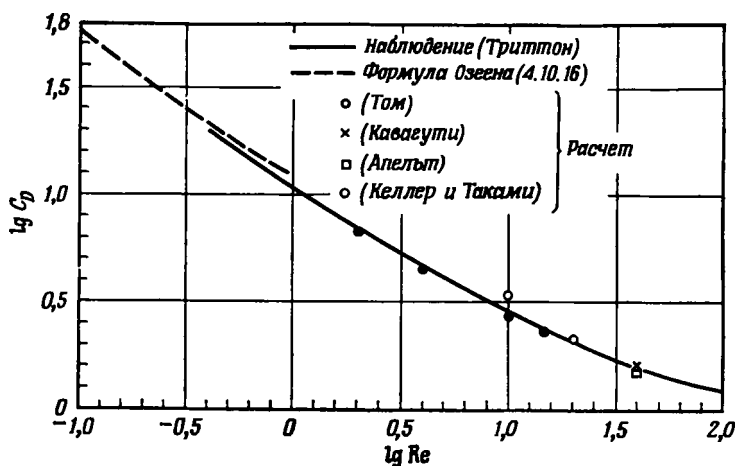
Р и с. 4.12.7. Коэффициент сопротивления цилиндра радиуса a ; C_D = D/1/2 \rho U^2 a , Re = 2aU/\nu .
