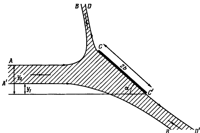
Р и с. 6.13.3. Общая картина струи, ударяющей о наклонную пластину с каверной под давлением окружающей среды.
