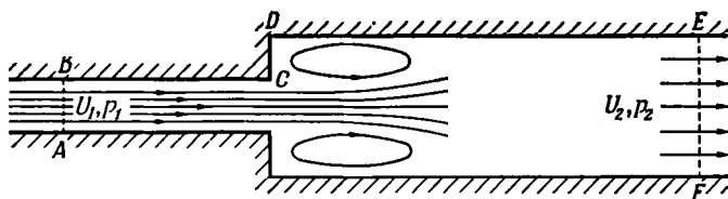
Рис. 5.15.2. Однородный поток в трубе при внезапном увеличении ее поперечного сечения.
