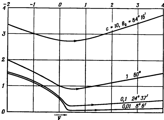
Рис. 4.6.2. Линии тока \psi/v = rf(\theta) = 1 для c = 0,01, 0,1 и 1,0 и \psi/v = rf(\theta) = 1/2 для c = 10 (величины \psi/v и r измерены в соответствующих единицах; ось абсцисс совпадает с осью симметрии).
