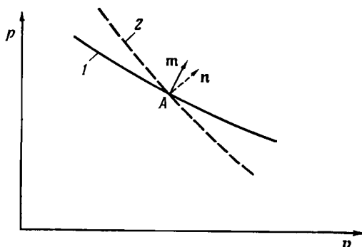
Рис. 1.5.1. Диаграмма равновесных состояний жидкости. 1 — изотермическое изменение; 2 — адиабатическое изменение.
