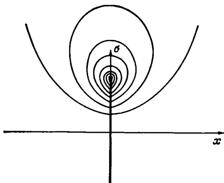
Рис. 6.8.2. Линии тока в осевой плоскости (приращения функции тока \psi одинаковы) в случае безвихревого течения, вызванного круговым диском, движущимся по нормали к своей плоскости.
