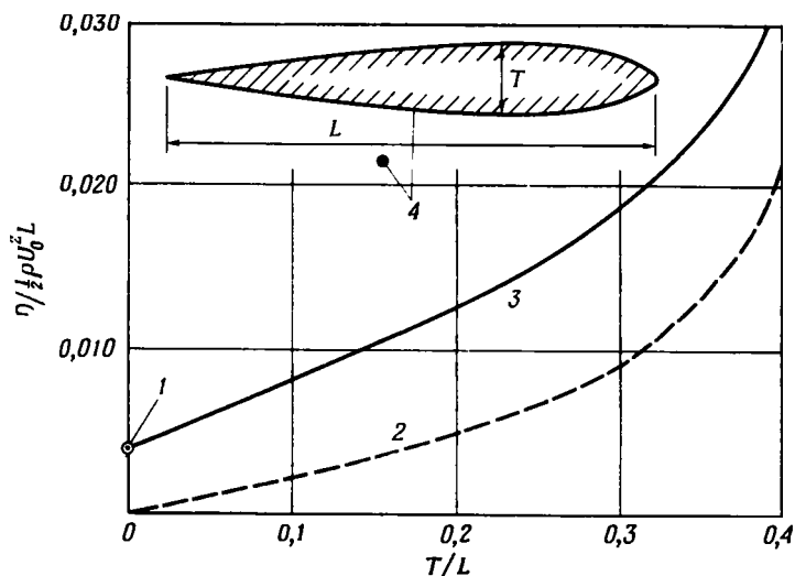
Р и с. 5.11.2. Наблюдаемые экспериментально значения полного сопротивления и сопротивления формы для семейства симметричных профилей, подобных показанному на рисунке и расположенных в потоке под нулевым углом атаки; U_0 L/\nu = 4 \cdot 10^5 (Фейдж, Фокнер и Уолкер (1929)).
