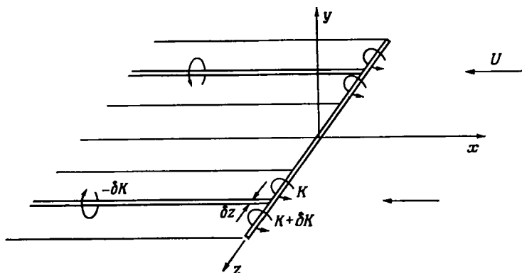
Р и с. 7.8.4. Вихревая система несущей линии. Дугообразные стрелки указывают фактическое направление циркуляции в случае, когда подъемная сила действует в положительном направлении оси y ( \delta K < 0 ).
