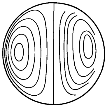
Р и с. 4.9.3. Сравнение теоретических (слева) и наблюдаемых (справа) картин линий тока в сферической капле глицерина, падающей в касторовом масле (Спеллс (1952)).
