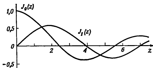
Р и с. 7.5.3. Функции Бесселя первого рода.
