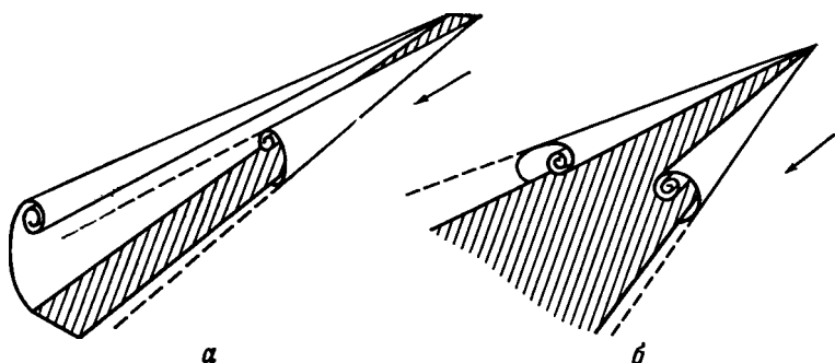
Р и с. 7.8.7. Схемы свертывания вихревой пелены, сходящей с боковых сторон удлиненных плоских несущих поверхностей.
