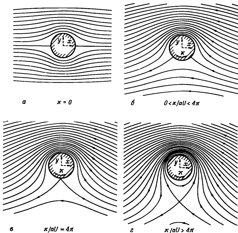
Р и с. 6.6.1. Линии тока безвихревого обтекания кругового цилиндра потоком с постоянной скоростью (-U, 0) на бесконечности и с циркуляцией скорости \kappa (в направлении против часовой стрелки).
