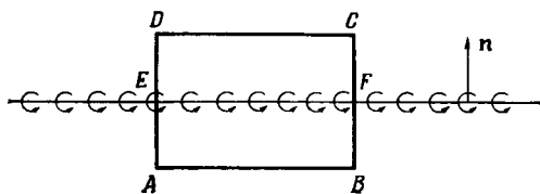
Рис. 2.6.4. Малый элемент неоднородной вихревой пелены.
