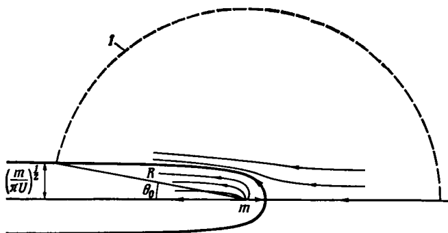
Р и с. 6.8.4. Обтекание полубесконечного тела, полученного путем наложения течения от точечного источника и однородного потока. I — контрольная поверхность.
