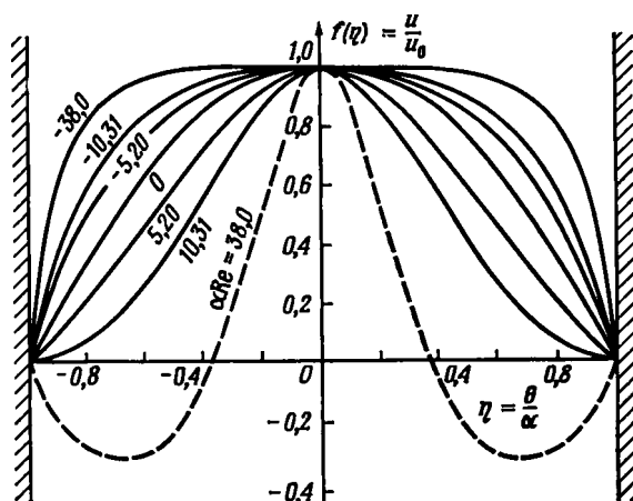
Рис. 5.6.4. Симметричные профили радиальной скорости в расширяющемся канале для различных значений \alpha Re = \alpha^2 r u_0 / \nu . Положительные значения \alpha Re соответствуют расходящемуся течению вблизи оси канала.
