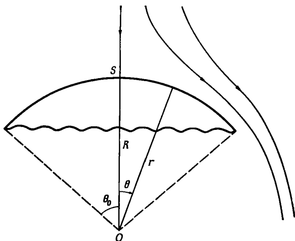
Р и с. 6.11.3. Схема течения при подъеме в жидкости пузыря в виде сферического сегмента.
