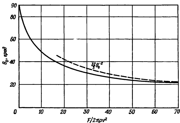
Р и с. 4.6.3. Соотношение между силой, приложенной в начале координат, и полууглом возникающей струи.
