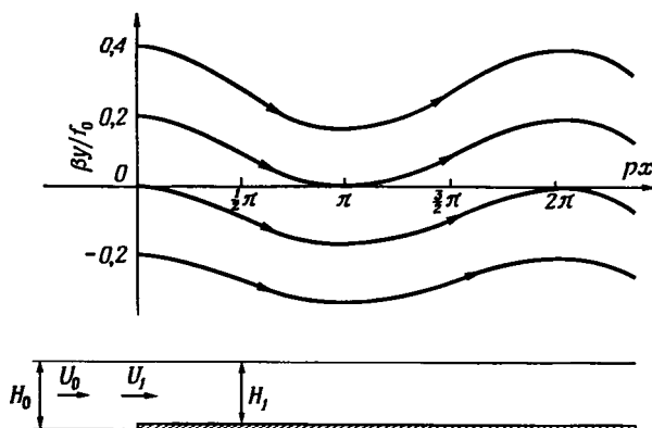
Р и с. 7.7.3. Линии тока при обтекании ступеньки, направленной с севера на юг, однородным западным ветром ( H_1 = 0,91 H_0 ).
