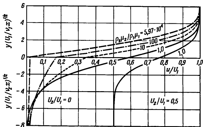
Р и с. 5.12.2. Профили скорости в установившемся переходном слое между двумя параллельными потоками жидкостей с различными плотностями и вязкостями (Лок (1951)).
