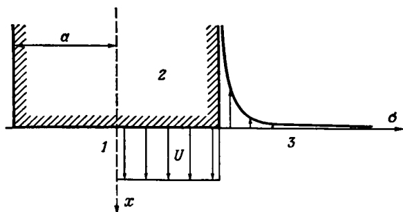
Рис. 6.10.1. Вертикальная скорость на поверхности жидкости сразу после прямого удара осесимметричного тела с плоской носовой частью. 1—ось симметрии; 2—тело; 3—свободная поверхность.
