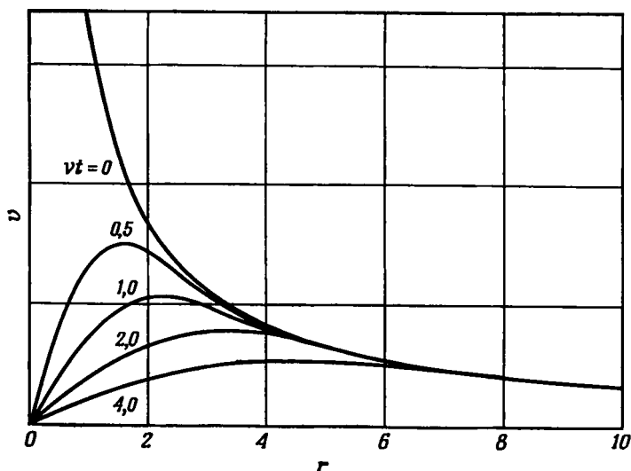
Р и с. 4.5.1. Распределение скорости, связанное с влиянием вихревой нити (радиус r и произведение vt измерены в соответствующих единицах).
