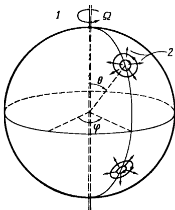
Р и с. 7.7.1. Геострофические системы циклонов в северном и южном полушариях. Завихренность относительно земной поверхности имеет тот же знак, что и f = 2\Omega \cos \theta , а давление в центре каждой системы низкое. 1 — северный полюс; 2 — силы Кориолиса, действующие в направлении от центра области.
