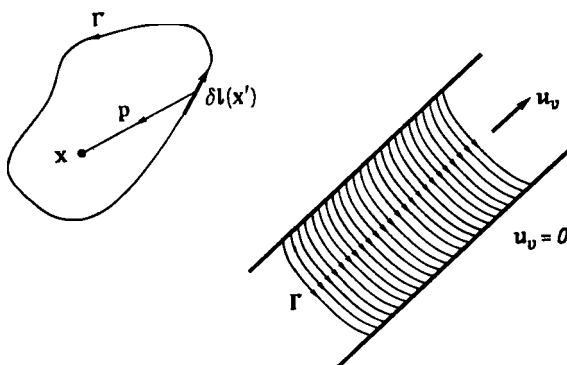
Р и с. 2.6.3. К расчету соленоидального распределения скорости в течении, создаваемом цилиндрической вихревой пеленой.
