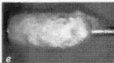
Фото 6.12.5. Стационарные каверны при K = 0,19 на круговом диске, расположенном нормально к потоку воды; а — давление в каверне поддерживается путем непрерывного подвода воздуха в каверну; б и в — каверны без подвода воздуха. Снимок б получен с выдержкой 2 сек, а снимок в — с выдержкой 10–6 сек. Асимметрия кормовой части каверны объясняется влиянием плавучести (фотографии ВМС США).
