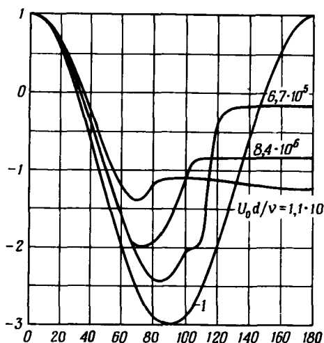
Р и с. 5.11.5. Измеренное распределение давления на поверхности кругового цилиндра, помещенного в поток со скоростью U_0 , при различных числах Рейнольдса; p_0 — давление на бесконечности.
