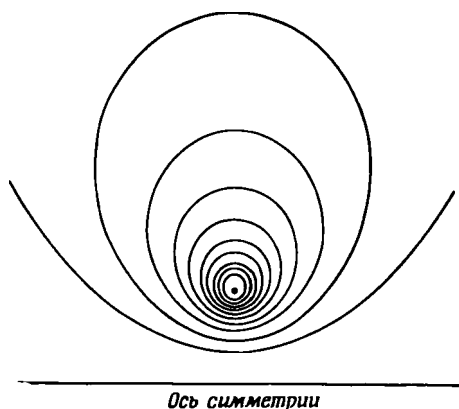
Р и с. 7.2.1. Линии тока в осевой плоскости, проведенные через равные интервалы изменения функции тока \Phi , для течения, индуцированного в покоящейся на бесконечности жидкости одиночной круговой вихревой нитью.
