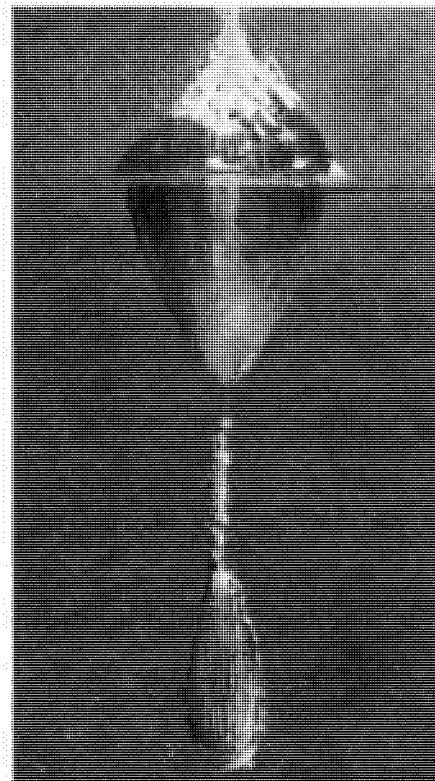
Фото 8.12.6. Каверна, образующаяся во время входа в воду сферы диаметром 9,9 см при скорости 880 см/сек (фотографии ВМС США).
