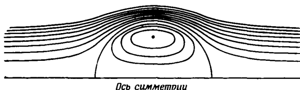
Р и с. 7.2.5. Линии тока установившегося течения относительно сферического вихря Хилла, проведенные через равные интервалы изменения функции тока \psi .
