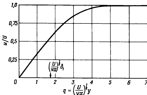
Рис. 5.8.1. Распределение скорости в пограничном слое на плоской пластине.
