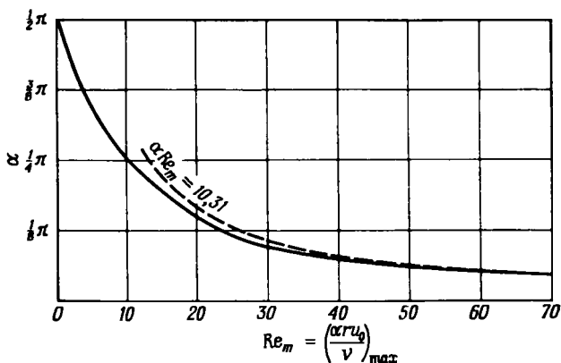
Рис. 5.6.3. Зависимость между \alpha и максимальным значением числа Рейнольдса Re_m = (\alpha u_0/\nu)_{\max} , для которого возможно чисто расходящееся течение. В области выше кривой чисто расходящийся поток невозможен; в области ниже кривой возможен.
