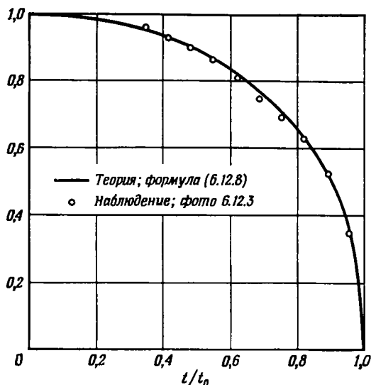
Р и с. 6.12.4. Схлопывание сферической каверны из состояния поноя под действием постоянного перепада давлений.
