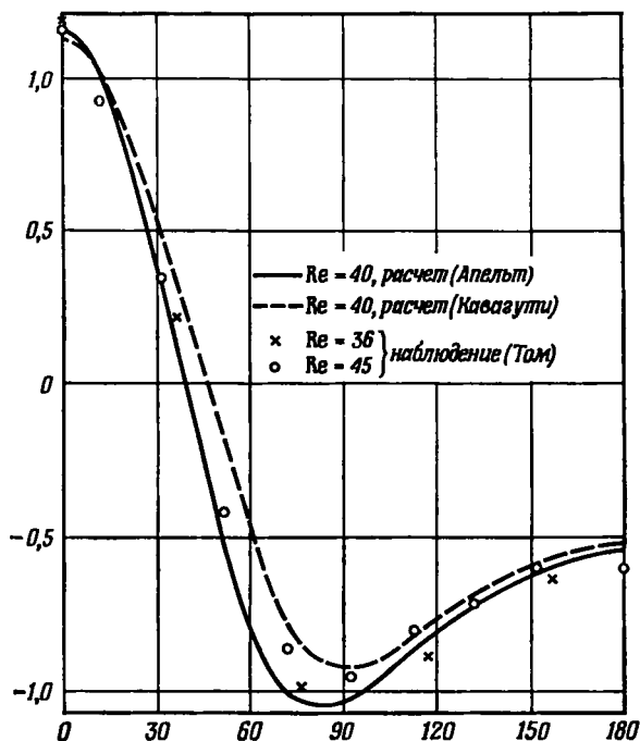
Р и с. 4.12.4. Распределение давления на поверхности кругового цилиндра (по оси абсцисс — угол в градусах, отсчитываемый от передней критической точки; по оси ординат — (p - p_0) / (\frac{1}{2} \rho U^2) ; p_0 — давление в бесконечности).
