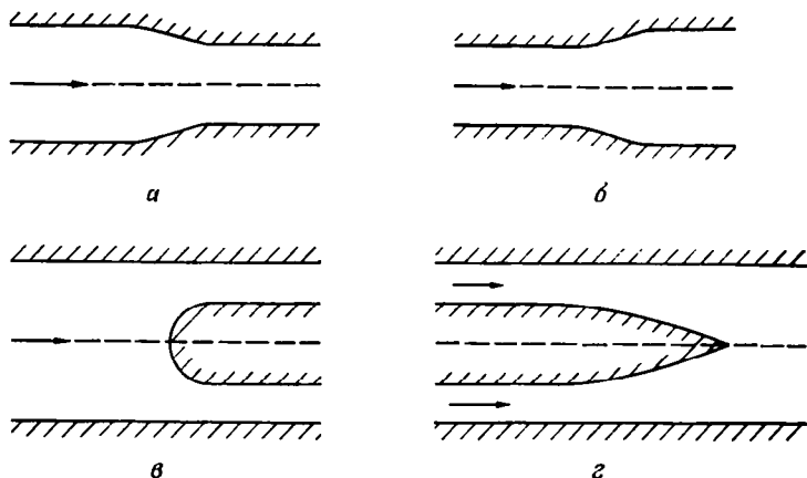
Р и с. 7.5.1. Различные варианты переходов от одного цилиндрического течения к другому.
