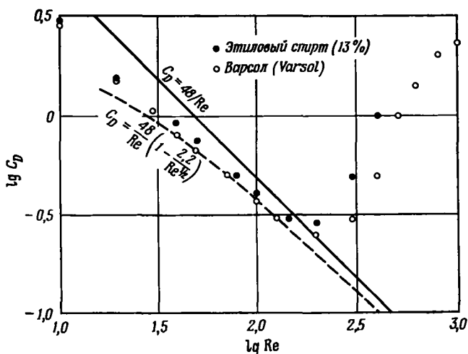
Рис. 5.14.1. Коэффициент сопротивления газовых пузырьков, поднимающихся в различных жидкостях. Экспериментальные данные для двух жидкостей взяты по экспериментальным кривым Хабермана и Мортон (1953).
