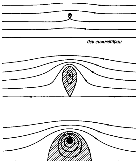
Р и с. 7.2.4. Схема линий тока установившегося течения относительно вихревого кольца при различных (малых) значениях отношения \epsilon/a . Внутренняя зачерненная область соответствует ядру вихря, а штриховной показана жидкость, переносимая вместе с кольцом.
