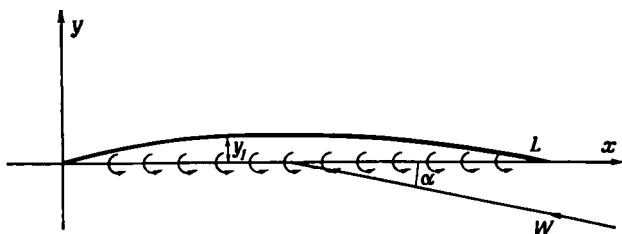
Р и с. 6.9.2. Представление бесконечно тонкого профиля (дужки) плоской вихревой пленкой.
