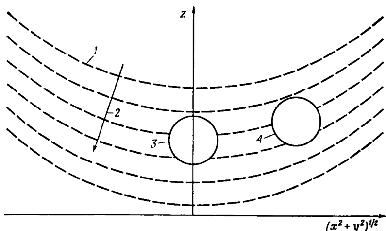
Р и с. 1.4.1. Неоднородная жидкость в состоянии покоя под действием силы тяжести и центробежной силы.
