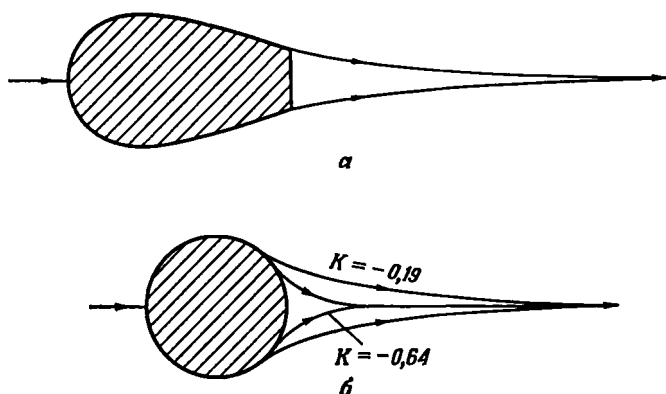
Р и с. 6.13.4. Каверны в установившемся двумерном безвихревом течении около тел с каверной под давлением, большим, чем давление окружающей среды; а — наверна за срезанным профилем при K = -0,111 , U_c/U = 0,943 , конформное преобразование (Лайтхилл (1949)); б — каверна за круговым цилиндром при K = -0,19 , U_c/U = 0,9 и K = -0,64 , U_c/U = 0,6 , численный анализ (Саусвелл и Вайси (1946)).
