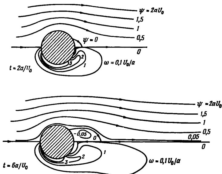
Р и с. 5.9.2. Линии тока относительно цилиндра и распределение завихренности \omega при внезапном приведении его в движение с постоянной скоростью U_0 ( 2aU_0/\nu = 100 ) в моменты времени 2a/U_0 и 6a/U_0 (Пейн (1958)).
