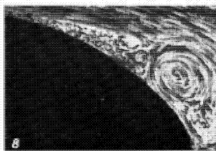
Фото 5.9.3. Последовательные стадии нарастания пограничного слоя на кормовой части плоскообтекаемого тела, которое начало двигаться из состояния покоя. Наблюдатель неподвижен относительно тела; движение жидкости происходит слева направо (Прандтль и Титъенс (1935)).
