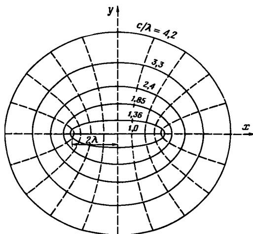
Р и с. 6.6.3. Семейство софокусных эллипсов в плоскости z , соответствующих окружностям |\zeta| = c в плоскости \zeta при преобразовании z = \zeta + \lambda^2/\zeta с различными величинами c . Штриховыми линиями показано ортогональное семейство софокусных гипербол, которые соответствуют радиальным прямым в плоскости \zeta .
