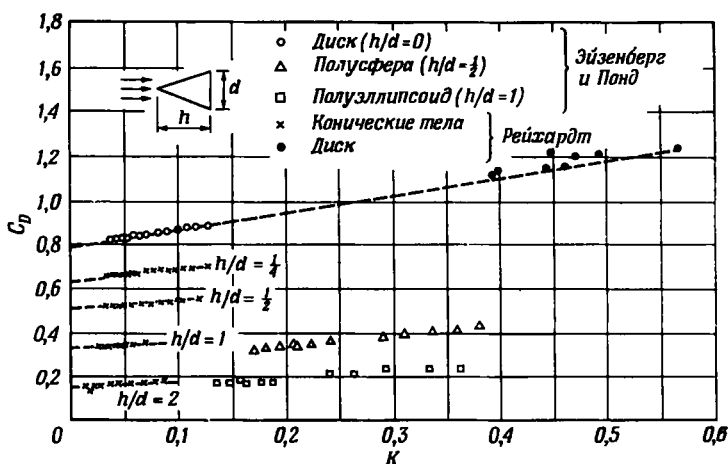
Р и с. 6.13.6. Измерения силы сопротивления различных осесимметричных тел с кавернами при положительных значениях числа кавитации (Рейхардт (1946), Эйзенберг и Понд ; (1948)). Каждая штриховая линия соответствует формуле C_D = C_{D0} (1 + K) .
