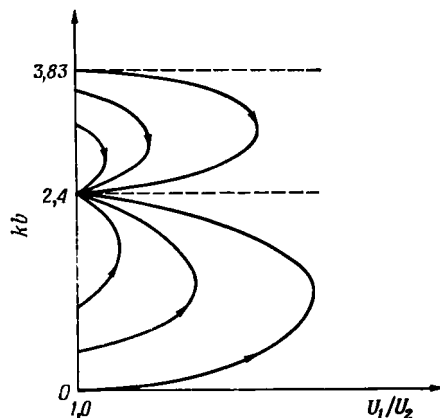
Р и с. 7.5.6. Схематическая зависимость радиуса вихря b от осевой скорости U_2 ( \leq U_1 ). Различные кривые относятся к различным значениям величины ka ; стрелки указывают направление изменения параметров от течения, соответствующего цилиндрическому вихрю радиуса a с вращением жидкости как твердого тела.
