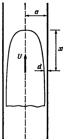
Р и с. 6.11.4. Большой пузырь, поднимающийся в вертикальной круглой трубе, наполненной водой.
