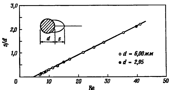
Р и с. 4.12.5. Наблюдаемые размеры области замкнутых линий тока за круговым цилиндром (Танеда (1956а)).
