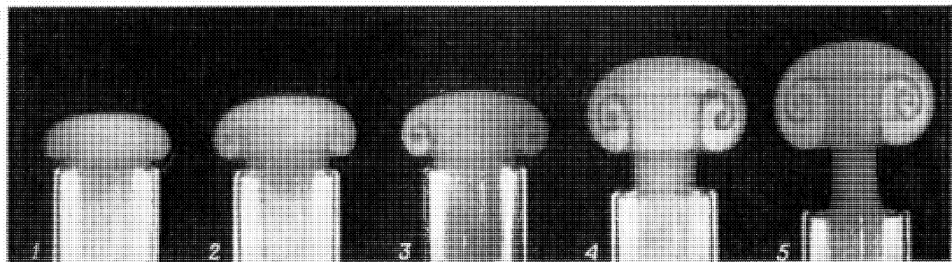
Фото 7.2.2. Различные стадии развития вихревых колец, образованных в воде при эжектировании малых количеств подкрашенной жидкости (по плотности близкой к воде) из стеклянной трубки кругового сечения с внутренним диаметром 1,5 см. На последнем снимке в центре вихревого кольца находится чистая вода, хотя это и незаметно при наблюдениях сбоку (Окаба и Иноуэ (1960)).
