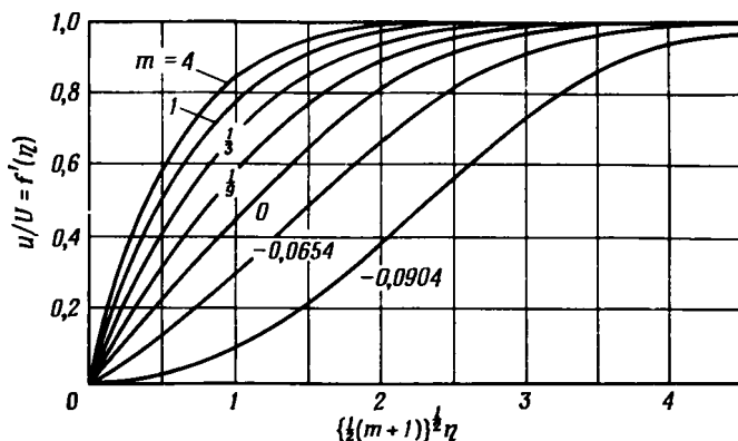
Р и с. 5.9.1. Автомоделные распределения скорости в пограничном слое при скорости внешнего потока U = cx^m .
