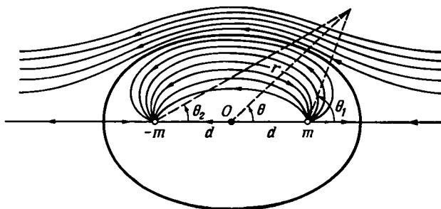
Р и с. 6.8.3. Линии тока течения в осевой плоскости, возникающего в результате наложения течений от точечного источника, от точечного стока равной интенсивности и однородного потока.
