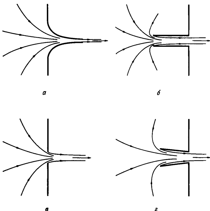
Р и с. 6.3.2. Истечение из круглого отверстия: а — плавно сужающийся насадок, \alpha = 1 ; б — насадок Борда, \alpha = 1/2 ; в — отверстие в плоской стенке, \alpha \approx 0,6 (эксперимент); г — насадок, для которого \alpha < 1/2 .
