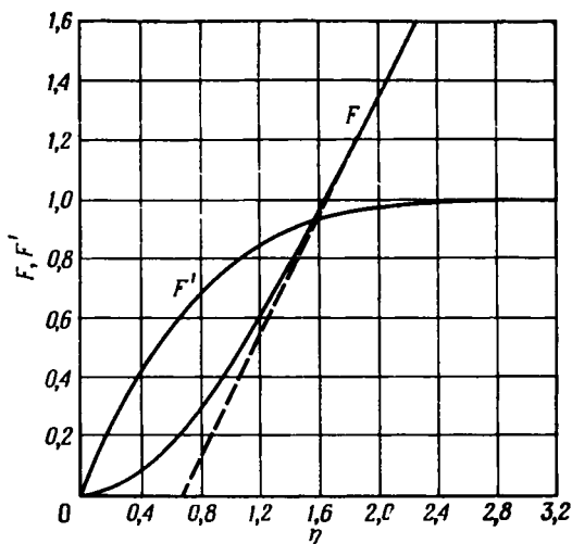
Р и с. 5.5.2. Функция F(\eta) , определяющая течение в вихревом слое.
