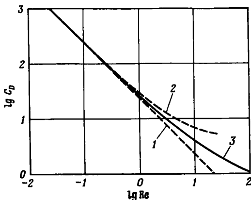
Рис. 4.9.2. Сравнение наблюдаемых значений коэффициента сопротивления сферы (из работы Кастильмана (1925)) с двумя теоретическими (по закону Стокса C_D = 24/Re и по второму приближению C_D = (24/Re)(1 + 3/16 Re) , где Re = 2a\rho U/\mu ). 1 — закон Стокса; 2 — второе приближение; 3 — наблюдение.
