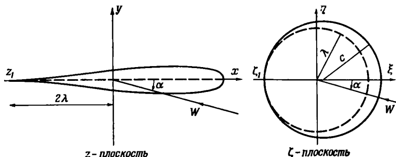
Р и с. 6.7.8. Преобразования круга в пластину (штриховая линия) и в симметричный профиль Жуковского (сплошная линия).
