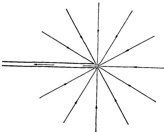
Рис. 2.5.1. Течение, возникающее при отсосе среды через открытый конец трубы, приблизительно такое же, как и течение, создаваемое точечным стоком.
