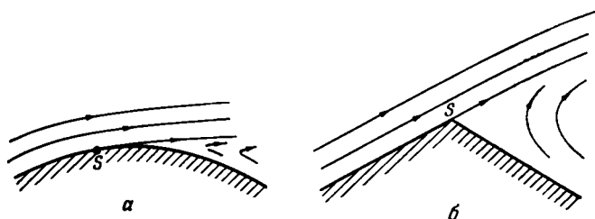
Рис. 5.10.4. Отрыв от гладкой твердой стенки (а) и от стенки с точкой излома (б).
