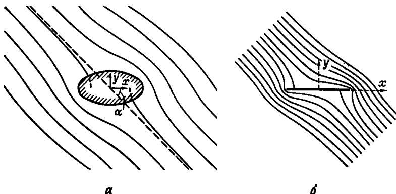
Р и с. 6.6.4. Линии тока при обтекании эллиптического цилиндра потоком с постоянной скоростью на бесконечности при \alpha = 45^\circ и с нулевой циркуляцией вокруг цилиндра; (а) b/a = 0,53 , c/\lambda = 1,80 ; (б) b/a = 0 , c/\lambda = 1 .
