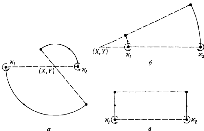
Р и с. 7.3.1. Движение двух точечных вихрей в неограниченной жидкости; a — величины \kappa_1 и \kappa_2 одного знака; b — противоположных знаков; c — случай \kappa_1 + \kappa_2 = 0 .
