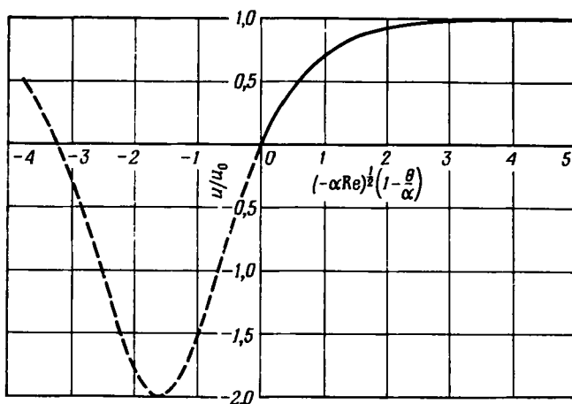
Рис. 5.6.2. Течение в сужающемся канале при больших числах Рейнольдса.
