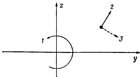
Р и с. 7.6.1. К вопросу о направлении силы Кориолиса, действующей во вращающейся системе отсчета. Плоскость (y, z) нормальна к оси вращения. 1 — направление вращения системы координат; 2 — компонента скорости u в плоскости (y, z) ; 3 — сила Кориолиса.
