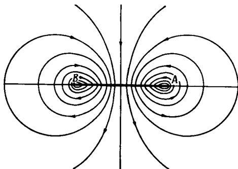
Р и с. 7.8.2. Линии тока двумерного движения непосредственно после приложения распределенного вдоль отрезка AB импульса силы, направленного вниз.
