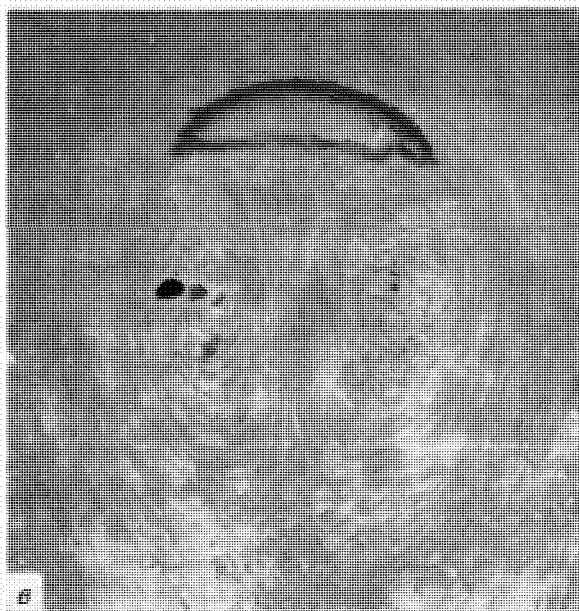
Фото 6.11.2. Фотографии больших пузырей газа, показывающие структуру следа за ними; а — искровые фотографии пузыря воздуха в нитробензоле, радиус R \approx 3 см, скорость U \approx 37 см/сек (Дэвис и Тейлор (1950)); б — пузырь воздуха в воде, радиус R \approx 5 см, скорость U \approx 45 см/сек (неопубликованная фотография Р. Коллинза); в — «двумерный» пузырь воздуха в воде между параллельными пластинами, расположенными на расстоянии 6 мм, радиус R \approx 7 см, скорость U \approx 40 см/сек (Коллинз (1965)). Фотографии б и в были сделаны камерой, неподвижной относительно пузыря, и с использованием твердых частиц для визуализации потока. На фотографиях а и б пузырь и жидкость, движущаяся вместе с ним, приблизительно ограничены сферой, а на фотографии в — окружностью.
