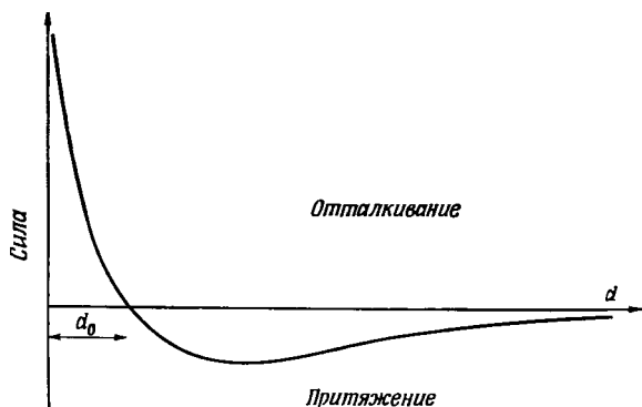
Р и с. 1.1.1. Зависимость силы взаимодействия простых (неионизированных) молекул от расстояния d между их центрами.
