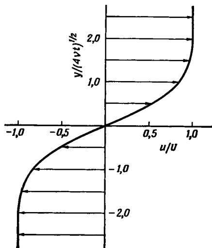
Р и с. 4.3.1. Переходный слой между двумя параллельными потоками.
