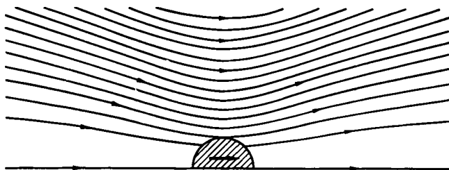
Р и с. 4.9.1. Линии тока в осевой плоскости течения, создаваемого движущейся сферой при числе Рейнольдса Re \ll 1 (без учета сил инерции).
