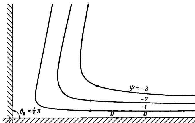
Р и с. 4.8.2. Двумерное течение в угловой области, возникающее при скольжении одной твердой плоскости по другой ( \psi в произвольных единицах).
