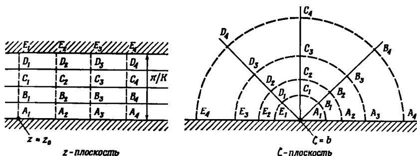
Р и с. 6.5.2. Конформное отображение бесконечной полосы в плоскости z на верхнюю полуплоскость \zeta с помощью функции \zeta = b + e^{K(z-z_0)} , где K — действительная положительная постоянная.
