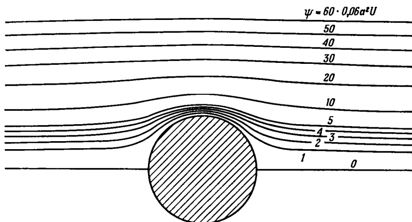
Р и с. 6.8.1. Линии тока в осевой плоскости безвихревого обтекания неподвижной сферы в потоке с постоянной скоростью на бесконечности.
