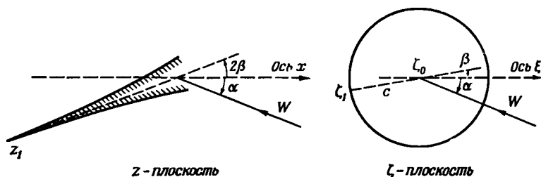
Р и с. 6.7.7. Схема к получению профиля из окружности с помощью конформного отображения.
