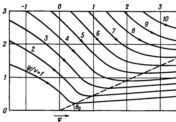
Рис. 4.6.1. Линии тока течения для c = 0,1 , \theta_0 = 24^\circ 37' (величины \psi/v и r измерены в соответствующих единицах; ось абсцисс совпадает с осью симметрии).
