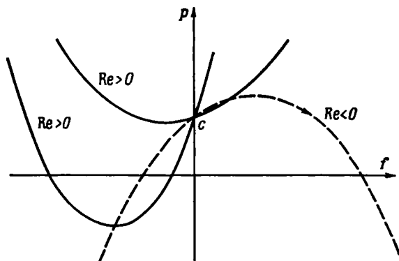
Р и с. 5.6.1. Схематическое представление функции P(f) = \frac{2}{3}\alpha \operatorname{Re} (f^3 + f) + 4\alpha^2 f + c для различных значений \operatorname{Re} .
