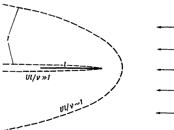
Р и с. 5.4.1. Диффузия и конвекция завихренности и теплоты от пластины, помещенной в однородный поток. 1 — граница области завихренности и повышения температуры; стрелки справа — скорость однородного потока.
