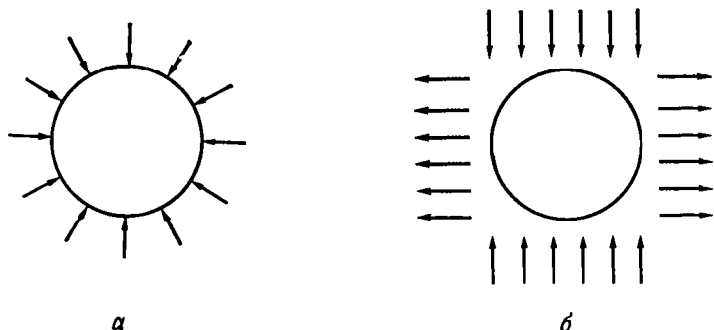
Р и с. 1.3.3. Два вида напряжений на поверхности сферического элемента жидкости: а) однородное всестороннее сжатие и б) однородное растяжение в направлении одной главной оси тензора напряжений наряду с однородным сжатием в направлении другой главной оси.
