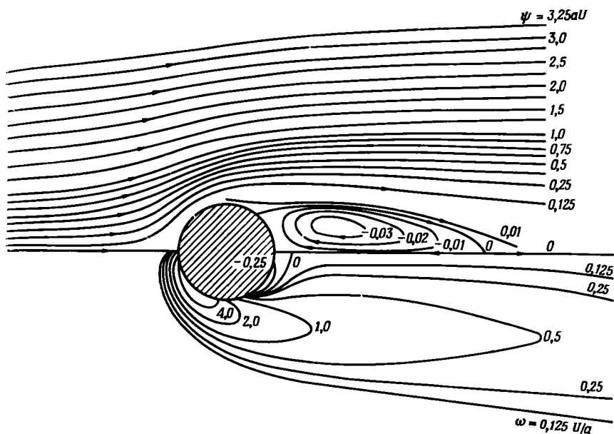
Р и с. 4.12.3. Линии тока (вверху) и линии постоянной завихренности (внизу) для обтекания кругового цилиндра при Re = 40 (расчет Апелята (1961)).
