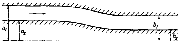
Р и с. 7.5.1. Различные варианты переходов от одного цилиндрического течения к другому.
