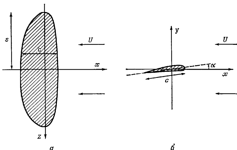
Р и с. 7.8.3. Система координат для крыла конечного размаха; ось y направлена вертикально.
