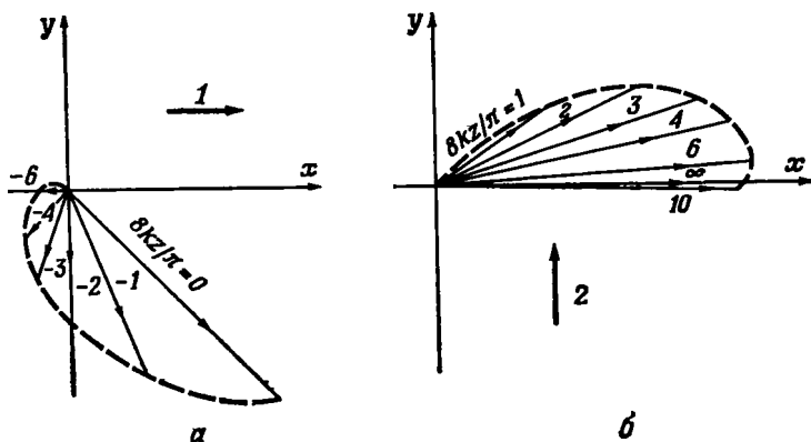
Р и с. 4.4.1. Вектор скорости во вращающейся жидкости: а — на различных расстояниях под свободной поверхностью, на которой приложено касательное напряжение, и б — на различных расстояниях над твердой плоскостью, когда имеется градиент давления. 1 — направление напряжения на свободной поверхности; 2 — направление градиента давления.
