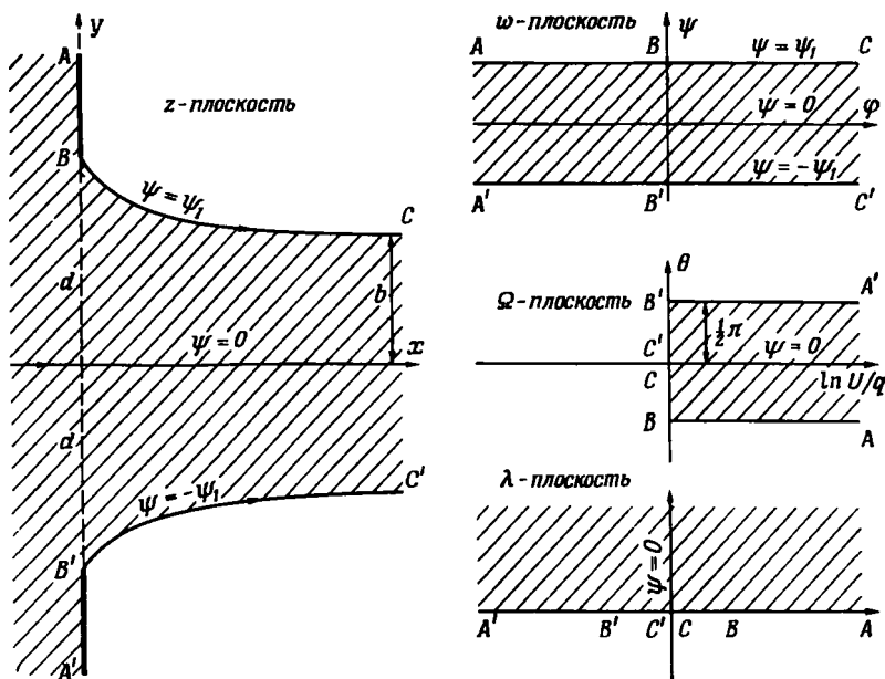
Рис. 6.13.1. Конформные преобразования, используемые для определения двумерной струи, вытекающей из отверстия в плоской стенке.
