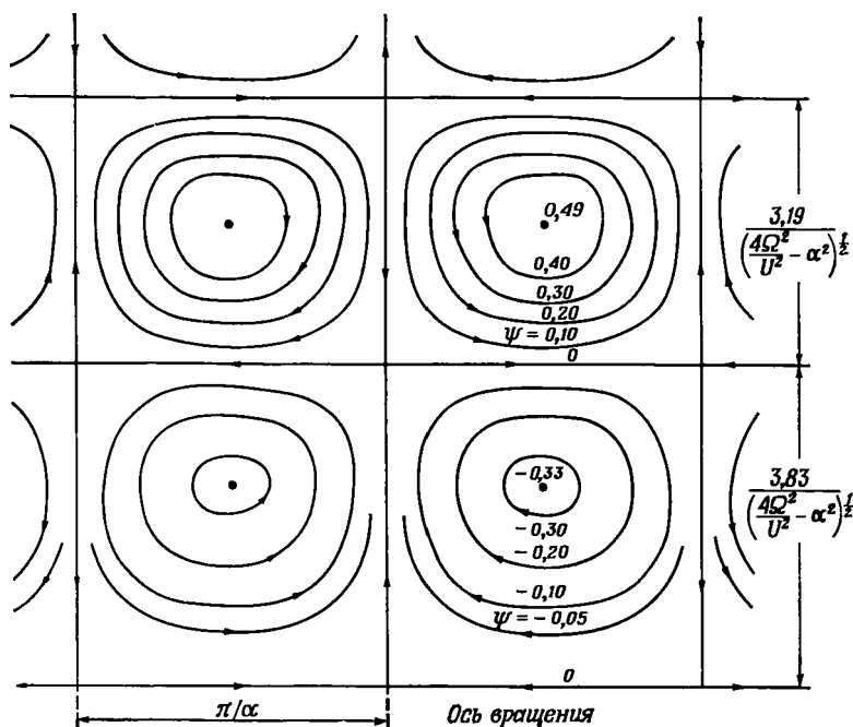
Р и с. 7.6.4. Мгновенная картина линий тока движения в проходящей через ось вращения плоскости, представляющая собой простую гармоническую волну, распространяющуюся в осевом направлении с фазовой скоростью U . Значения функции тока соответствуют соотношению (7.6.7) при A = (k^2 - \alpha^2)^{1/2}/3,83 . (Линии тока для стоячей волны, образующейся при наложении двух таких прогрессивных волн малой амплитуды, имеют такую же форму, см. (7.6.10).)
