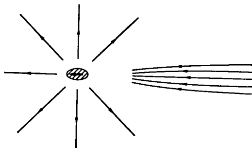
Р и с. 5.12.4. Течение на большом расстоянии от тела, которое движется справа налево в жидкости, покоящейся на бесконечности; оно состоит из течения в следе и компенсирующего его течения от источника.
