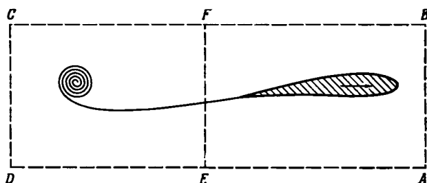
Р и с. 6.7.4. Схема, показывающая, что циркуляция скорости вокруг профиля при установившемся движении равна по величине и противоположна по знаку потоку завихренности, сходящей с профиля.
