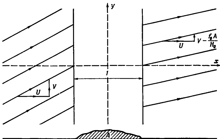
Рис. 7.7.2. Отклоняющее действие горного хребта на однородный поток с компонентами скорости U и V относительно вращающейся системы координат. I — горный хребет; поперечное сечение хребта заштриховано.
