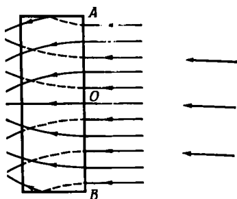
Р и с. 7.8.1. Возникновение завихренности вниз по потоку от крыла вследствие подсаживания жидкости на концах крыла с нижней стороны повышенного давления на верхнюю. Завихренность в спутном потоке имеет циркуляцию на участке OA против часовой стрелки относительно направления течения, а на участке OB — по часовой стрелке.
