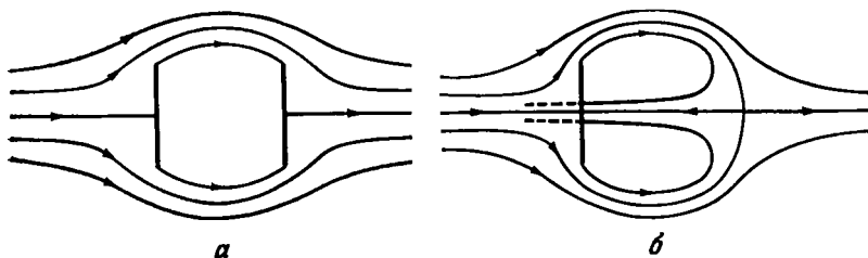
Рис. 6.13.7. Две схемы течения около плоской пластины с каверной под давлением меньшим, чем давление окружающей среды ( K > 0 ); а — схема с отраженной пластиной; б — схема с возвратной струей.
