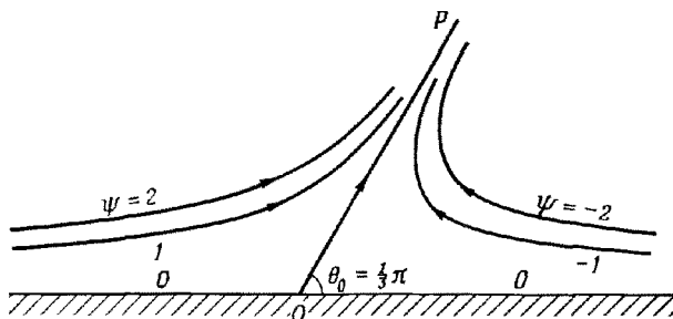
Р и с. 4.8.3. Двумерное течение вблизи точки с нулевым трением на плоской твердой границе (построено в соответствии с выражением (4.8.28) при \theta_0 = \pi/3 и A < 0 ; \psi в произвольных единицах).
