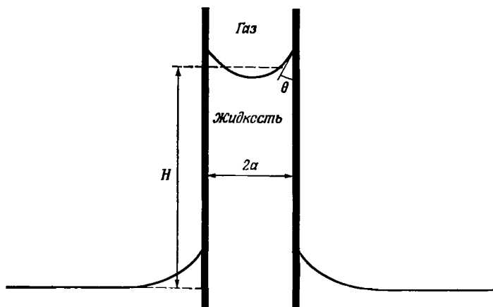
Р и с. 1.9.3. Капиллярный подъем жидкости в тонкой трубке.
