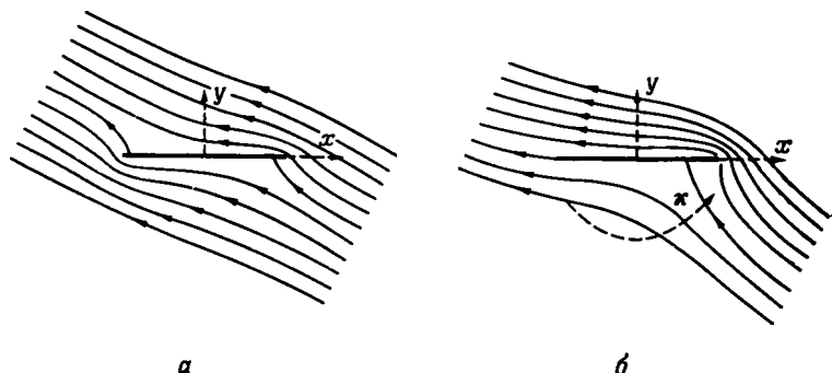
Р и с. 6.7.1. Линии тока при обтекании пластины потоком с постоянной скоростью на бесконечности при \alpha = 26^\circ : а — течение с нулевой циркуляцией; б — течение, в котором циркуляция выбрана так, что происходит плавный сход потока с обеих сторон кормовой кромки пластины.
