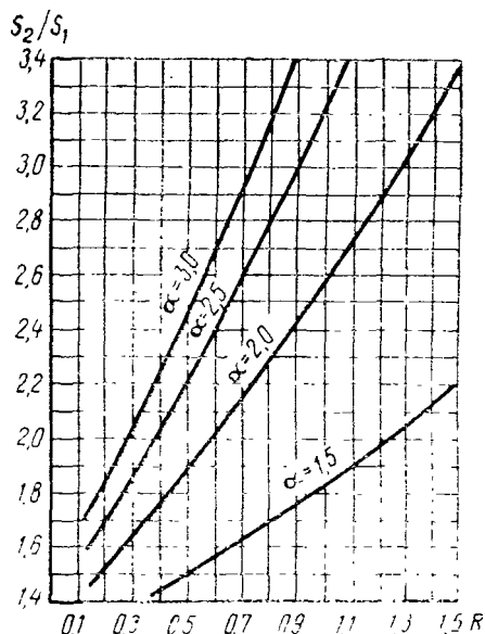
Рис. 43. График зависимости отношения понижений уровня от коэффициента пьезопроводности
