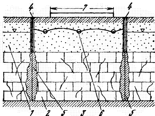
Рис. 52. Комбинированная кольцевая противофильтрационная завеса в дренаж для защиты подземных вод от инфилирующих стоков:
