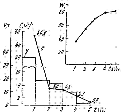
Рис. 80. Концентрации и количество хрома, извлекаемого проектируемым защитным дренажем на территории химического завода:
