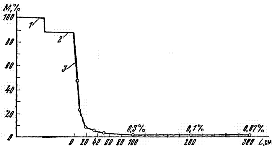
Рис. 11. Изменение содержания бактерий в воде (M) по пути фильтрации (L) из инфильтрационного бассейна:
