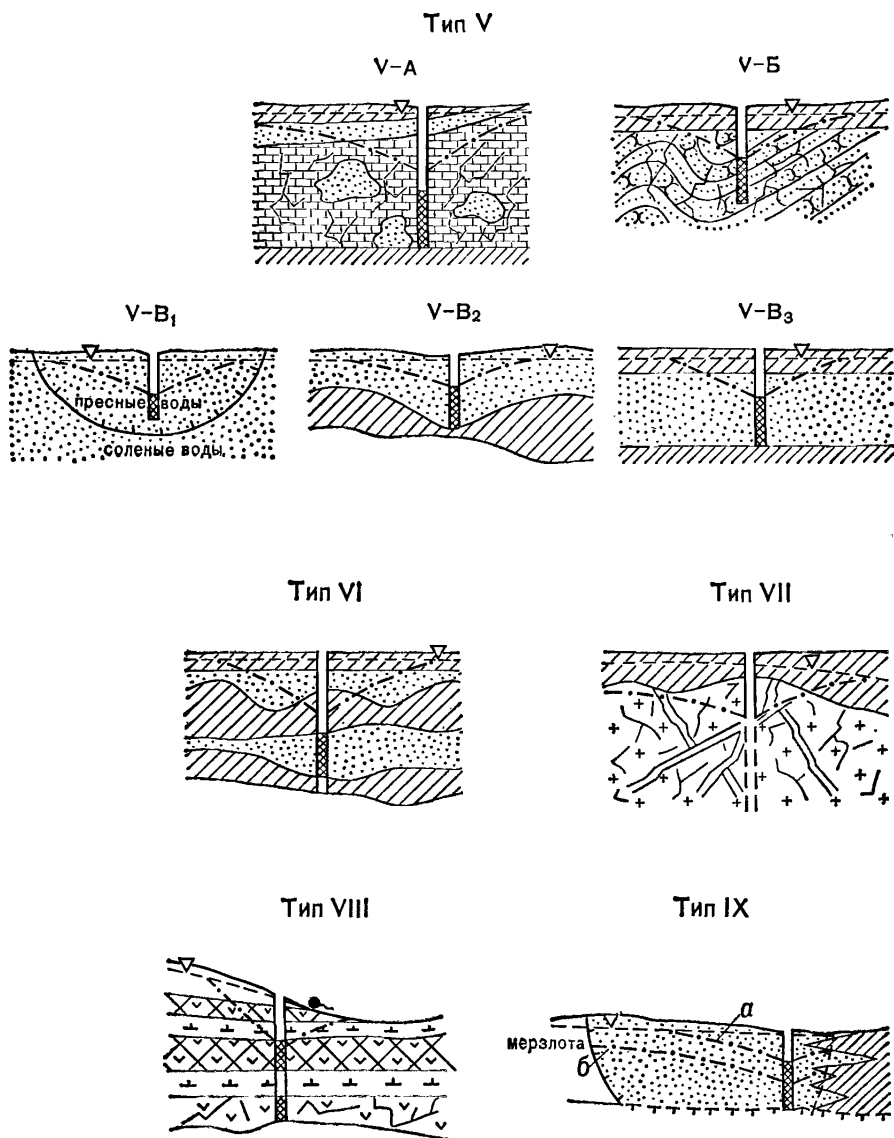
Рис. 62. Схематические разрезы основных типов месторождений подземных вод (табл. 13.1):
