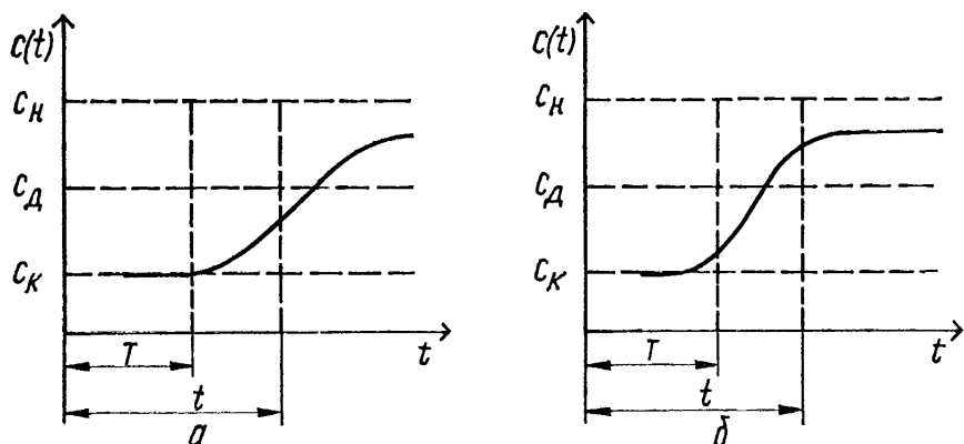
Рис. 57. Графики изменения качества воды во времени без превышения концентрации загрязняющих веществ (а) допустимой нормы и при формировании в течение расчетного периода эксплуатации некондиционных вод (б)
