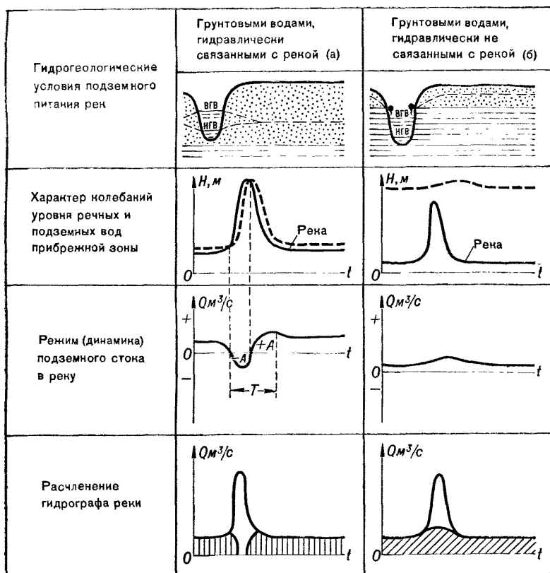
Рис. 14. Типовые схемы расчленения гидрографа реки (по Б. И. Куделину, 1960): 1 — водоносные породы; 2 — водоупорные породы; 3 — поверхностный сток; 4 — подземный сток из водоносных горизонтов, гидравлически не связанных с рекой; 5 — то же для гидравлически связанных с рекой; 6 — уровень подземных вод
