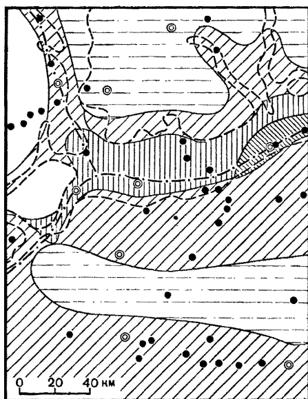
Рис. 24. Фрагмент карты вертикального коэффициента фильтрации верхнеюрских глин Средне-Клязьминского месторождения подземных вод (по Б. В. Боревскому, М. В. Кочеткову, Т. А. Плугиной, Н. Н. Шарапанову, 1981):
