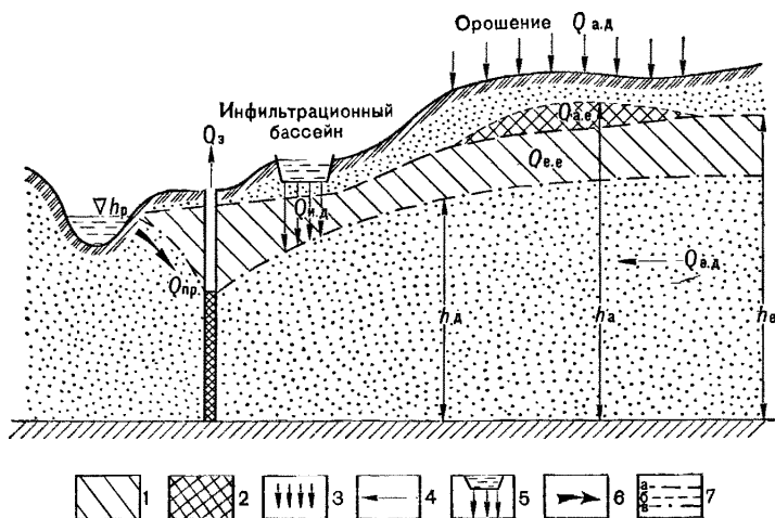
Рис. 4. Схема формирования ЭЗПВ ( Q_z ) за счет различных источников:
