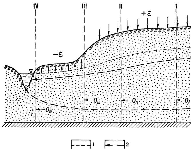
Рис. 8. Схема формирования расхода грунтового потока в различных поперечных сечениях:
