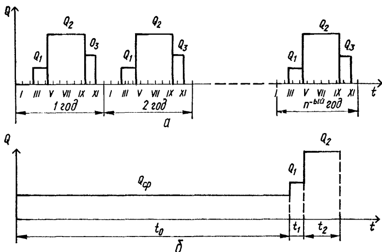
Рис. 60. График ступенчатого периодического водоотбора для орошения (а) и его расчетная схематизация (б)
