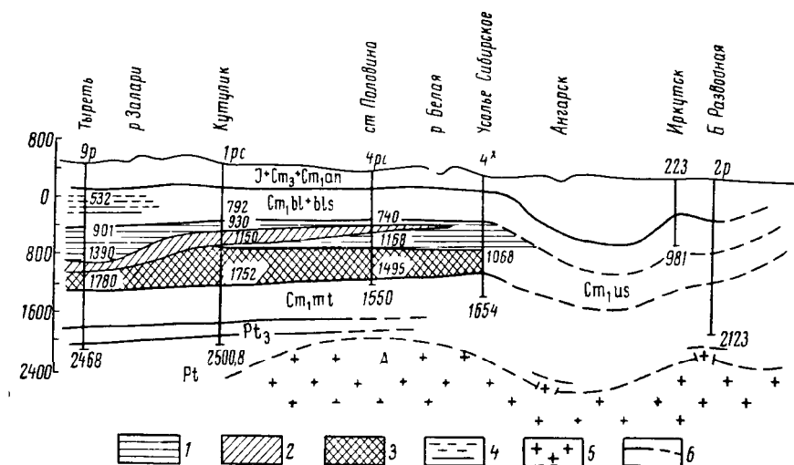
Рис. 97. Схема залегания нижнекембрийских соляных отложений на участке Тиреть — Иркутск. Составил П. И. Трофимук, 1965 г.
