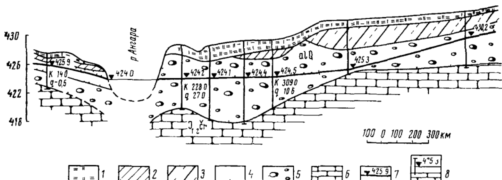
Рис. 29 Гидрогеологический разрез через долину р. Ангары у г. Иркутска Составил В. Л. Мирошниченко по материалам МОСГИДЕПА, 1965 г
