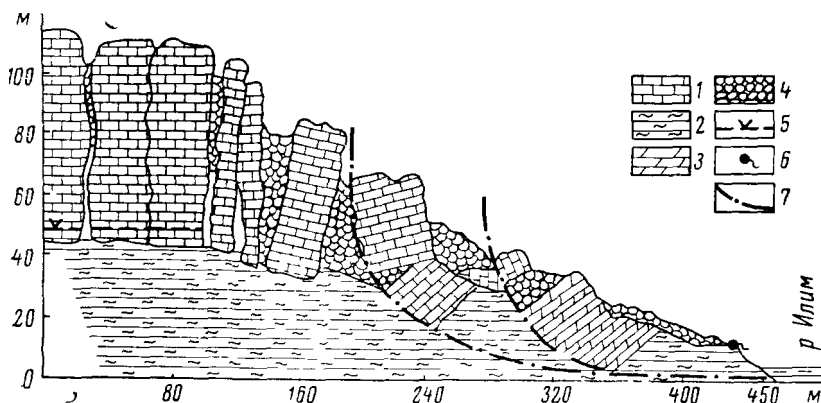
Рис. 93. Схема развития глыбовых оползней илимского типа (по С. М. Большакову, 1964)
