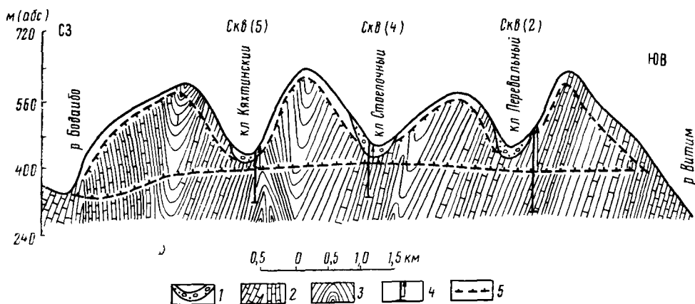
Рис. 47. Мерзлотно-гидрогеологический разрез по трассе туннеля Нижне-Бодайбинской ГЭС (по А. И. Голубкову, 1945 г.)
