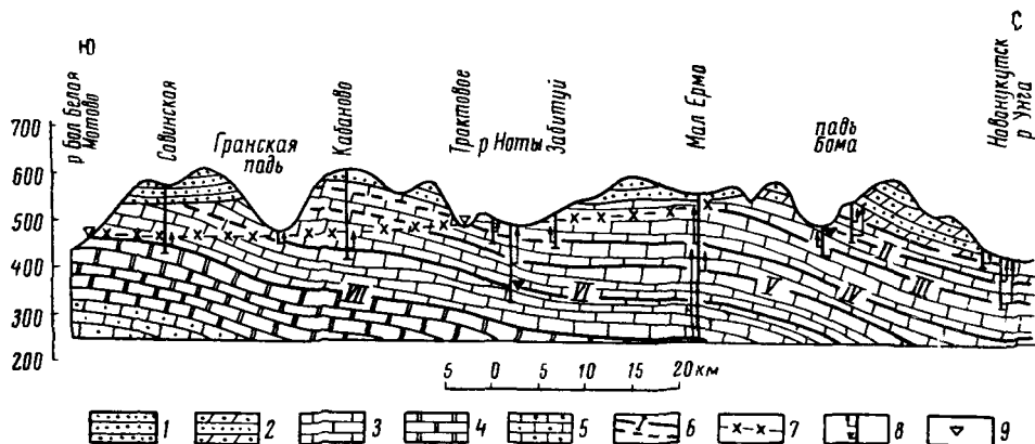
Рис. 42. Гидрогеологический разрез отложений ангарской свиты нижнего кембрия. Составил Е. В. Пиннекер, 1964 г.
