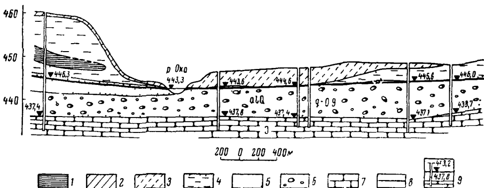
Рис. 30 Гидрогеологический разрез через долину р. Оки у г. Зимы Составил В. Л. Мирошниченко, 1965 г
