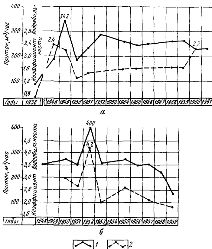
Рис 77. Графики притока воды в шахты им. Кирова (а) и № 8 (б) Черемховского каменноугольного месторождения. Составил Я. И. Зарубинский, 1963 г.
