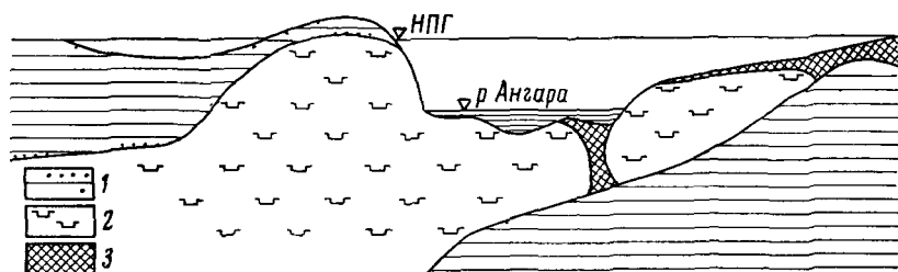
Рис. 96 Схематический геологический разрез по створу Толстый Мыс (по материалам Гидроэнергопроект)
