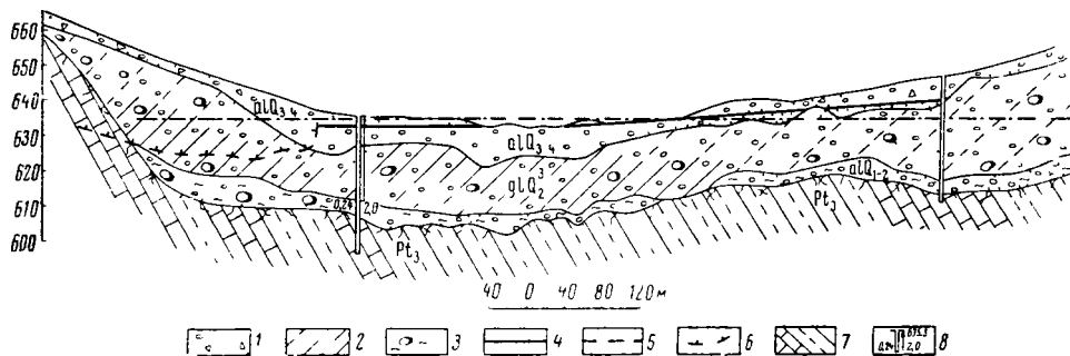
Рис. 32. Гидрогеологический разрез по долине р. Маракан у пос. Усть-Маракан (по С. А. Бойкову, О. Г. Боярскому и др., 1963 г.)
