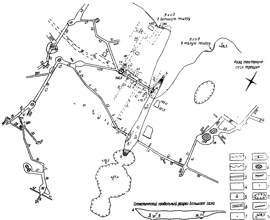
Рис 21. План Балаганской пещеры
