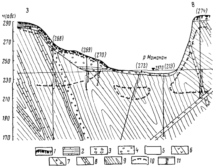
Рис 48 Мерзлотно-гидрогеологический разрез долины р. Мамакана (по Р. А. Оркину, 1958 г)
