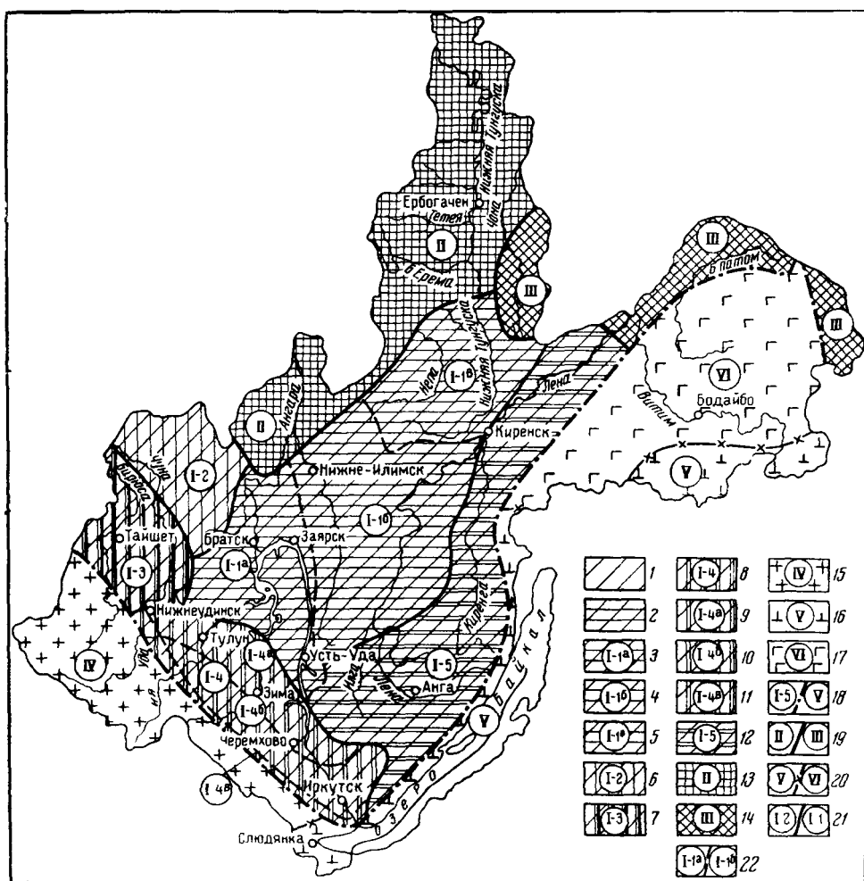
Рис 53 Гидрогеологическое районирование Иркутской области, 1965 г
