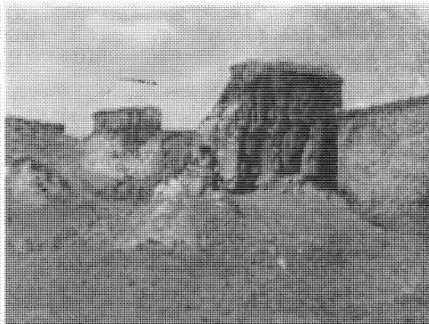
Рис. 91. Столбчатая отдельность лессовидных суглинков на правом склоне р. Ангарты в районе Лисихи (г. Иркутск). Фото Ф. Н. Лещикова, 1959 г.
