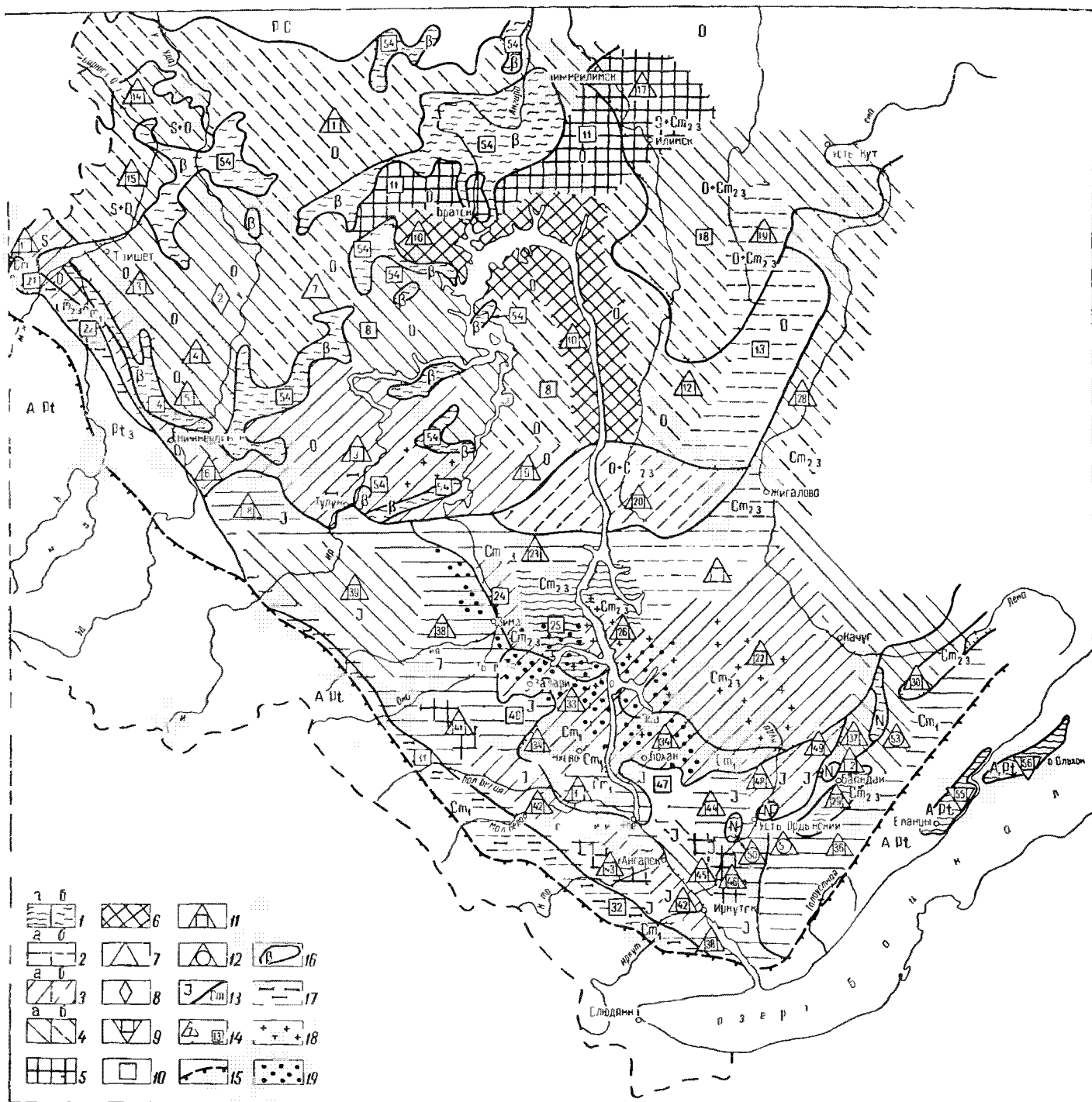
Рис 67 Карта специального гидрогеологического районирования южной части Иркутской области для прогнозной оценки запасов подземных вод Составил П И Трофимук при участии А И Анненковой, М В Нечаевой, З И Павловой, 1963 г
