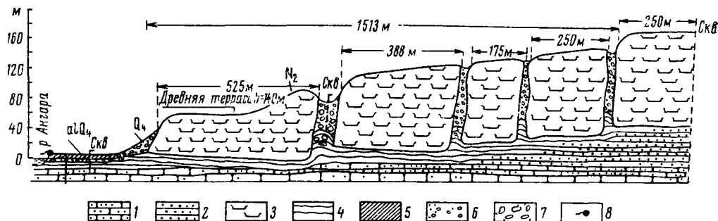
Рис. 94. Схематический разрез по оползневому склону в среднем течении Ангары в районе устья р. Илима (по Г. Б. Пальшину и Ю. Б. Тржцинскому, 1963 г.)
