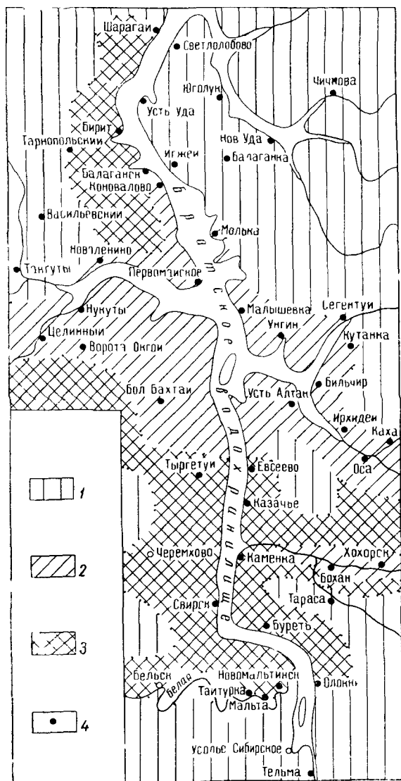
Рис 68 Схема условий водоснабжения подземными водами на верхнем участке Братского водохранилища. Составили Е. В. Пиннекер и З. А. Хлебникова, 1963 г.
