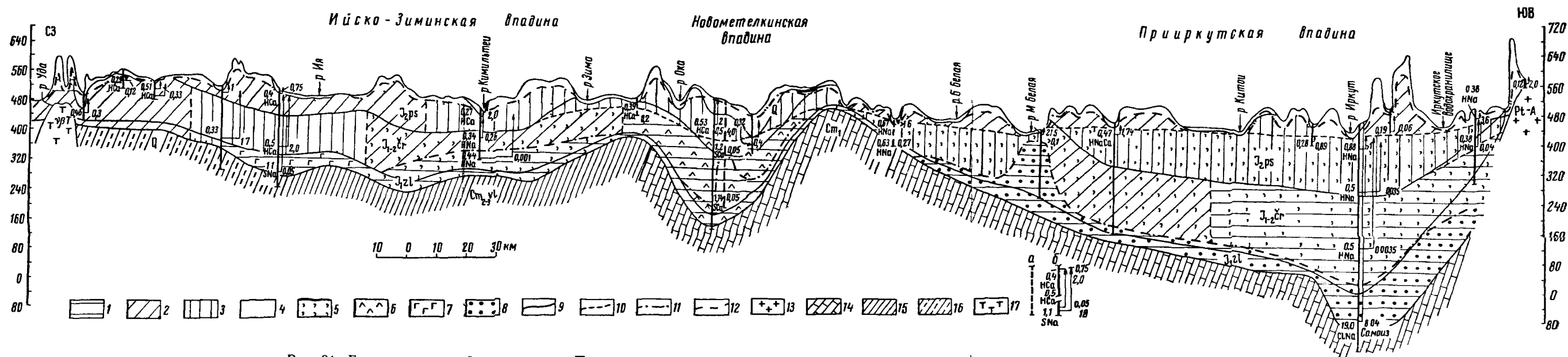
Рис 34 Гидрогеохимический разрез через Присаянские впадины Иркутского артезианского бассейна Составил Я И Зарубинский, 1965 г.
