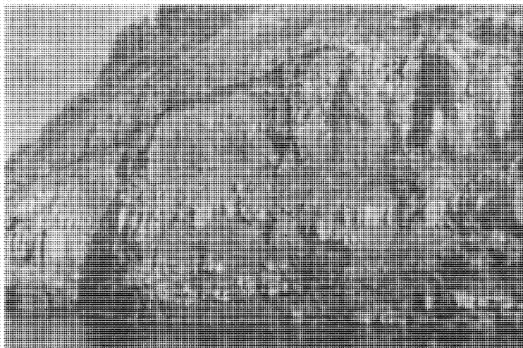
Рис 13 Обнажение юрских пород на берегу Иркутского водохранилища. Фото Е. В. Пиннекера, 1960 г.
