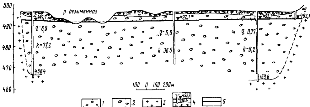
Рис 31 Гидрогеологический разрез через долину р Безымянной в нижнем течении (по И А Лившицу 1962 г)
