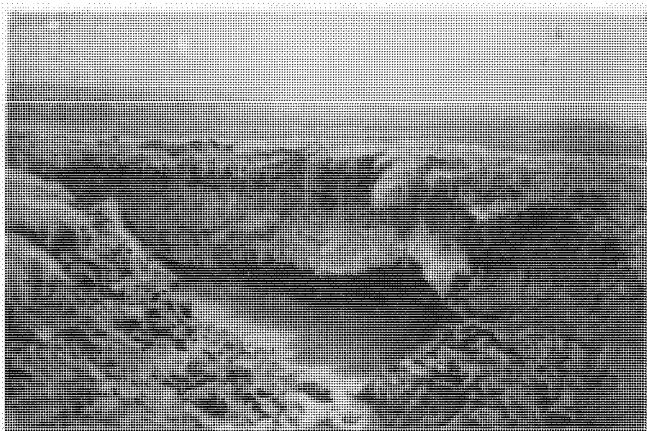
Рис 26 Ядро бугра пучения в долине р. Баяндайки. Фото Ф. Н. Лещикова
