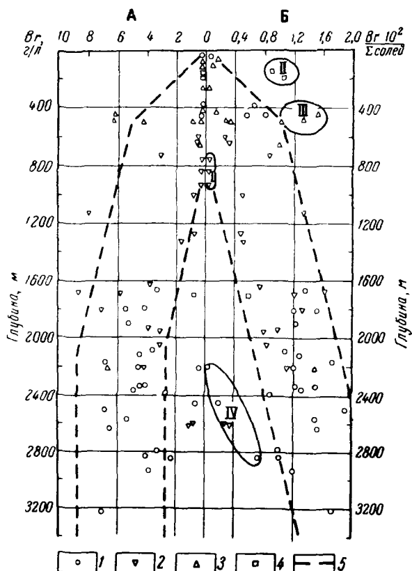
Рис 60 Графики изменения концентрации брома (А) и процентного содержания брома (Б) с ростом глубины залегания рассолов Составил Е В Пиннекер, 1964 г.
