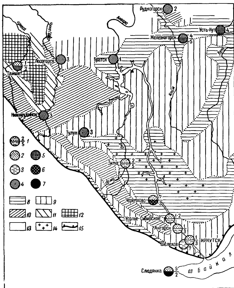
Рис. 69. Схема обеспеченности эксплуатационными запасами (по группам водоснабжения) пресных подземных вод городов южной части Иркутской области. Составил П. И. Трофимук, 1965 г.
