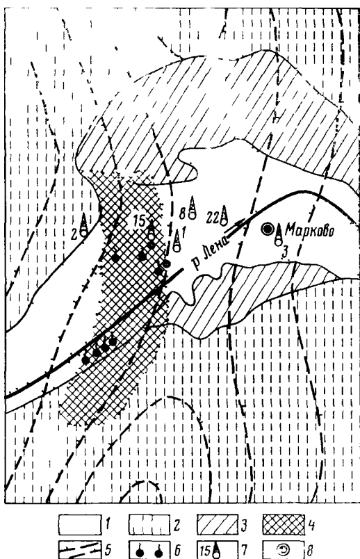
Рис. 46 Карта разгрузки рассолов на Марковской антиклинальной структуре Соста вил Е. В. Пиннекер, 1963 г.
