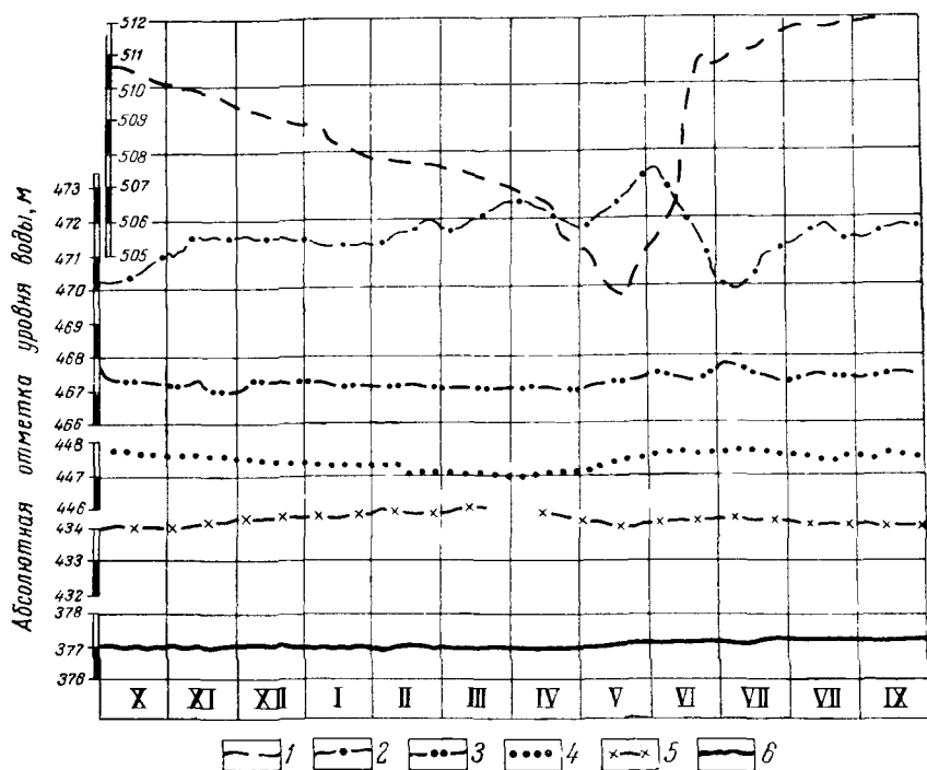
Рис. 65 Типичные графики уровня подземных вод провинции сезонного питания Составил В А Малий, 1964 г
