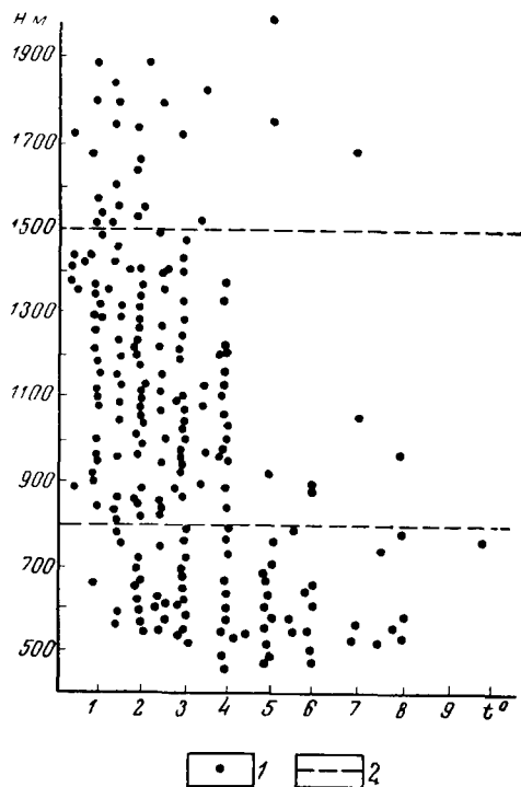
Рис. 56. График зависимости температуры воды от абсолютной высоты родника для юго-западного побережья оз. Байкал. Составил Б. И. Писарский, 1964 г.
