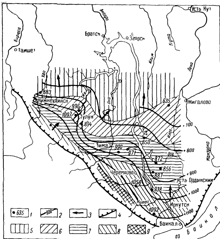
Рис 45 Схема приведенных гидростатических уровней парфеновского рассолоносного горизонта Составил Е В Пиннекер, 1964 г Условные обозначения те же что и на рис 44
