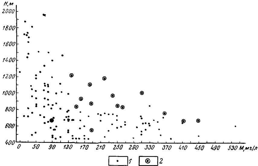
Рис. 55. График зависимости минерализации воды от абсолютной высоты родника для горноскладчатого обрамления Иркутской области Составил Б. И. Писарский, 1964 г. 1 — родник из изверженных и метаморфических (некарбонатных) пород; 2 — родник из карбонатных пород
