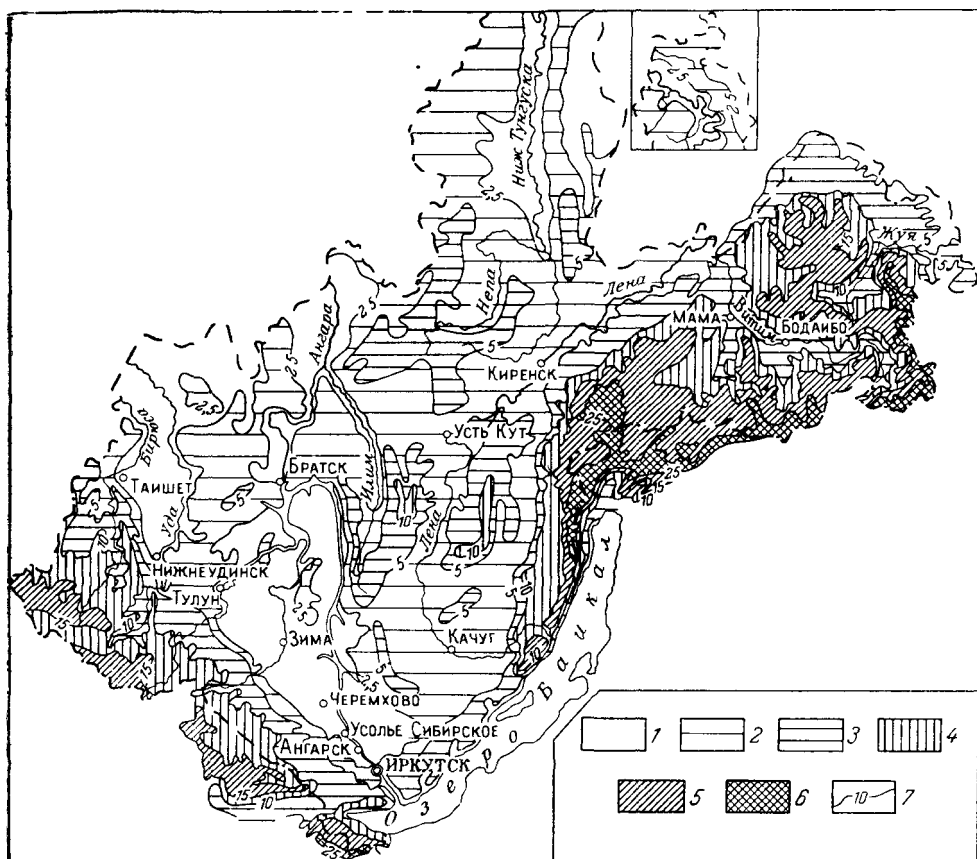
Рис 7 Карта среднегодового стока рек Иркутской области (по А. Н. Афанасьеву, 1962 г.)
