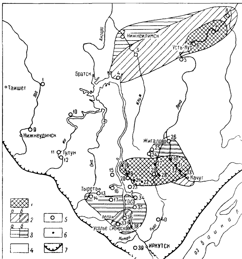
Рис. 98. Схема глубин залегания кровли первого от поверхности слоя каменной соли нижнекембрийских отложений мощностью от 20 м и более. Составил П. И. Трофимук, 1965 г.
