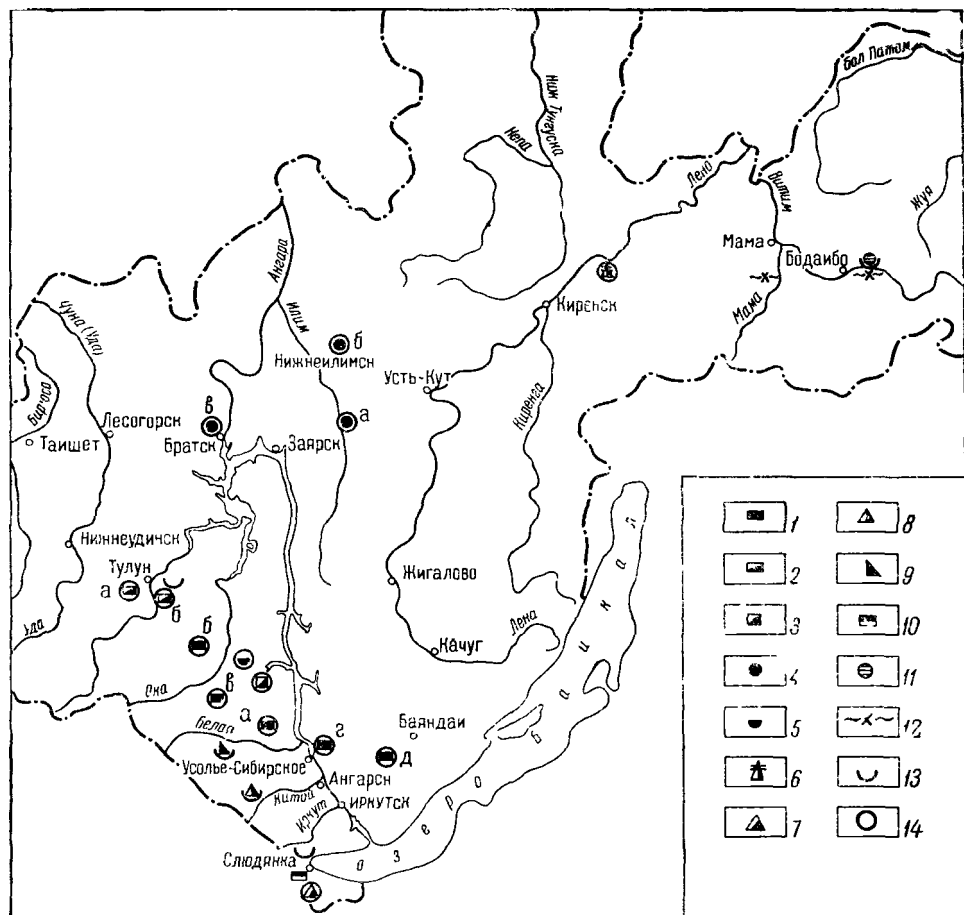
Рис. 74 Схематическая карта расположения месторождений полезных ископаемых Иркутской области Составили Я. И. Зарубинский и И. А. Лившиц, 1965 г
