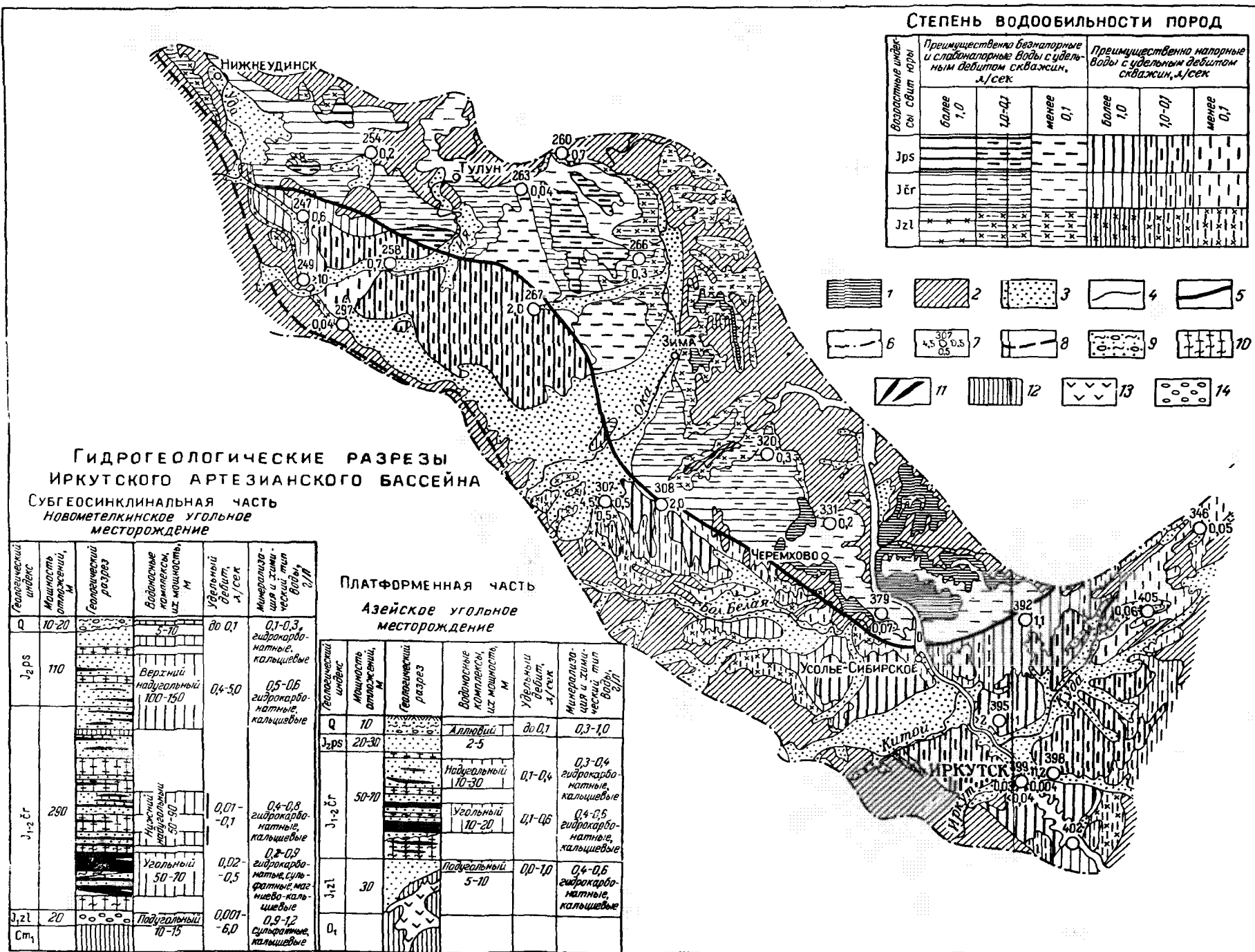
Рис. 33. Карта водообильности юрских отложений Иркутского артезианского бассейна. Составил Я. И. Зарубинский, 1965 г.
