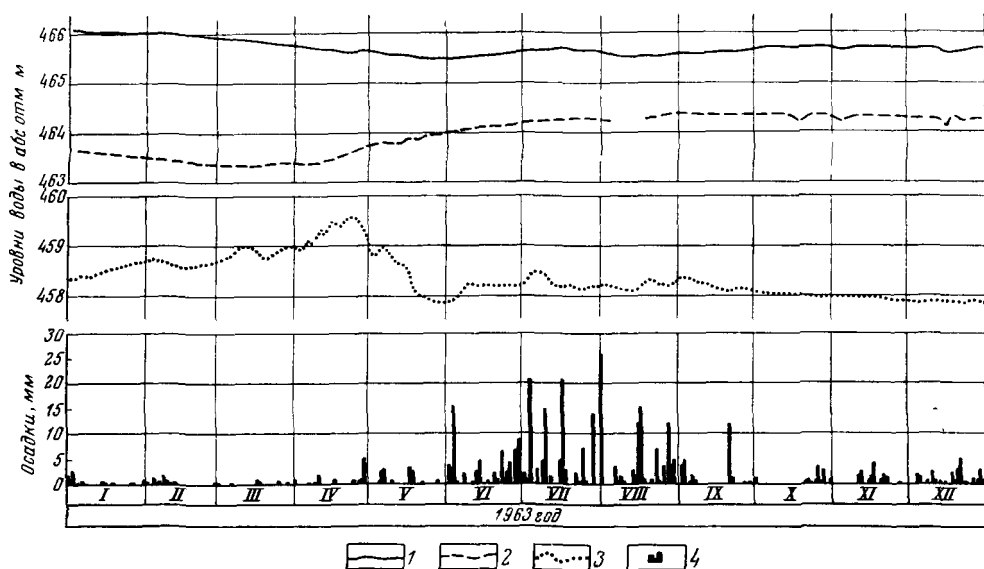
Рис. 66 Колебания уровня подземных вод на Азейском месторождении угля в 1963 г. Составил В. А. Малий, 1963 г.
