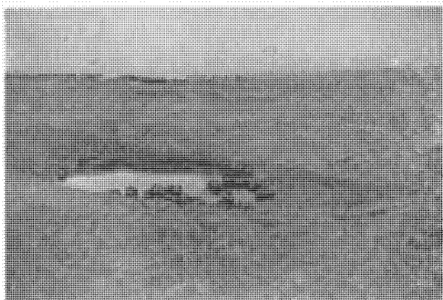
Рис. 25 Термокарстовая воронка у дер. Горхон Баяндаевского района Фото Ф. Н. Лешикова
