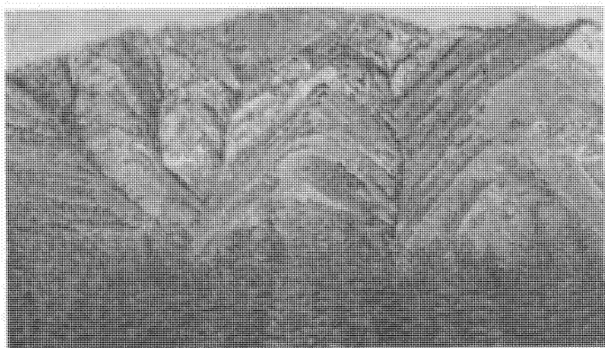
Рис 11 Выход мраморов дербинской свиты протерозоя в Восточном Саяне. Дендритообразные эрозионные формы Фото В. М. Колосницына, 1963 г.
