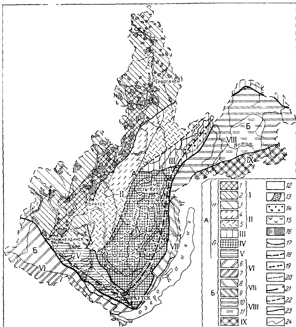
Рис 16 Схема геоморфологического районирования Иркутской области Составил А. Г. Золотарев, 1963 г
