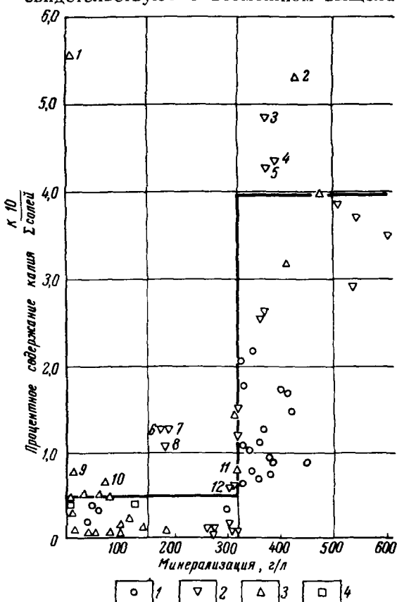
Рис. 82 Зависимость процентного содержания калия от минерализации подземных вод Составил Е. В. Пиннекер, 1965 г.
