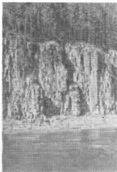
Рис 14 Столбчатые отдельности в траппах на правом берегу р Бирюсы Фото Н. Н. Шурановой, 1963 г.
