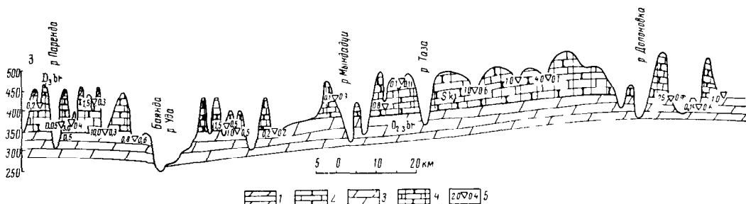
Рис 36 Схематический гидрогеологический разрез отложений нижнего силура (по В. П. Качура, 1965 г)
