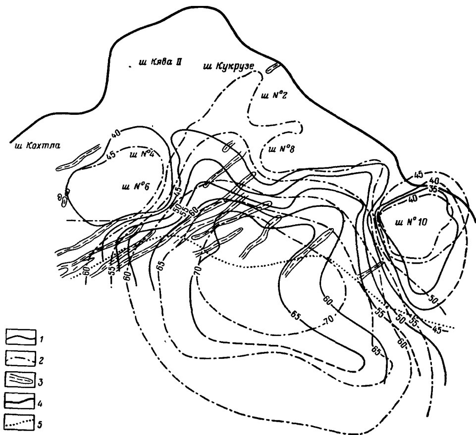
Рис 60 Схема гидроизогипс ордовикского водоносного комплекса. Центральная часть эстонского месторождения горючих сланцев
