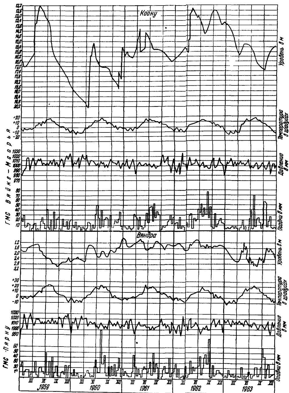
Рис. 31. График режимных наблюдений по ордовикскому водоносному комплексу
