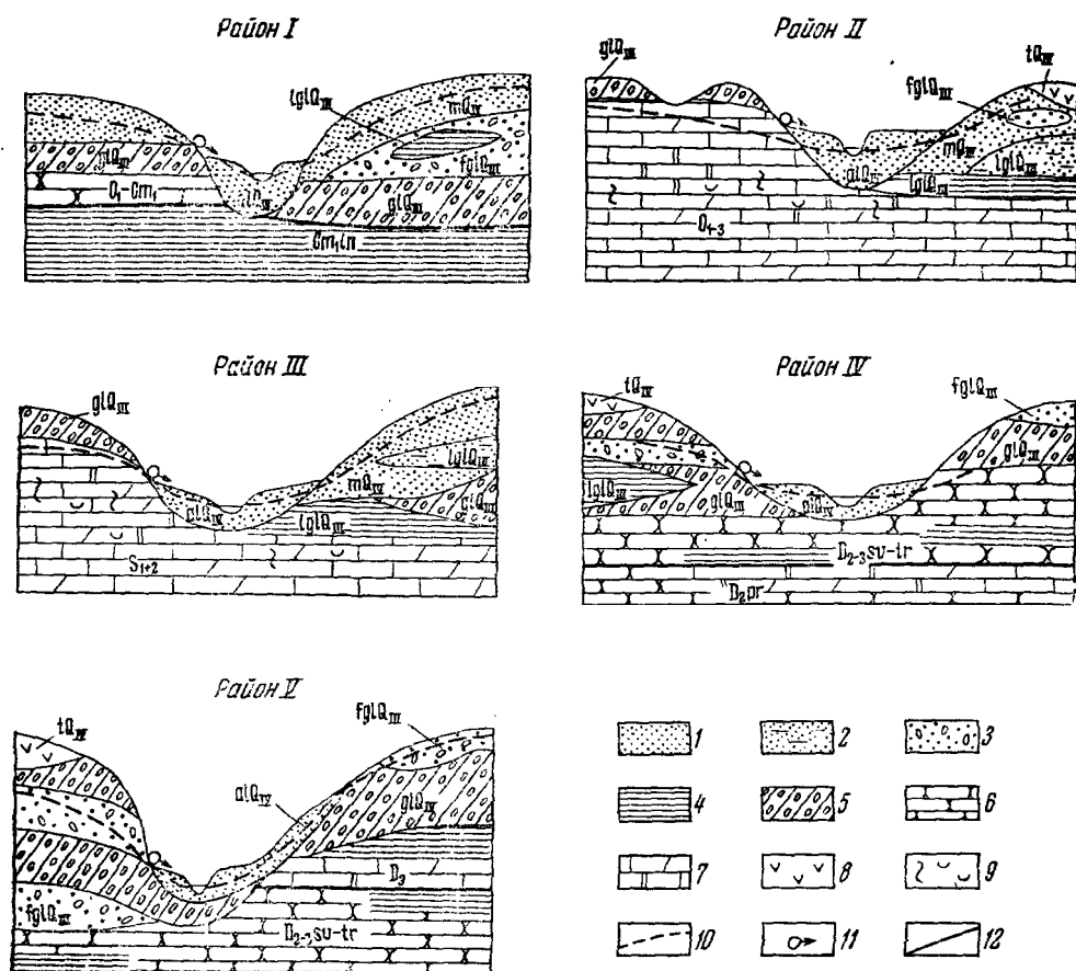
Рис. 51. Схемы дренирования водоносных комплексов и горизонтов
