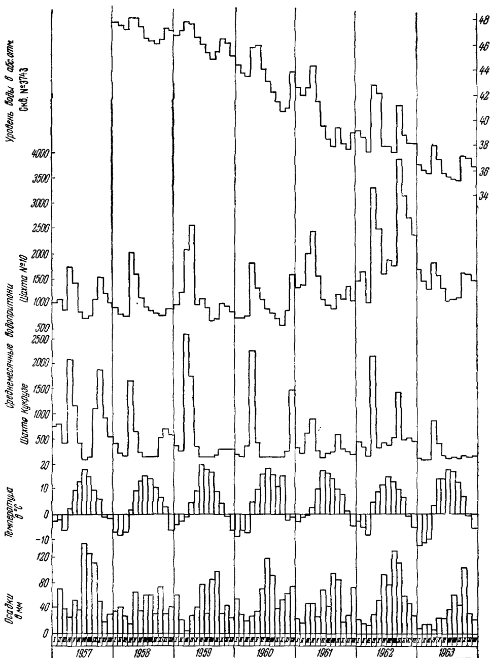
Рис. 59. Динамика водопритоков в зависимости от уровня подземных вод и климатических факторов
