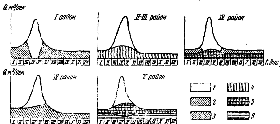
Рис. 52. Схемы генетического расчленения гидрографа стока
