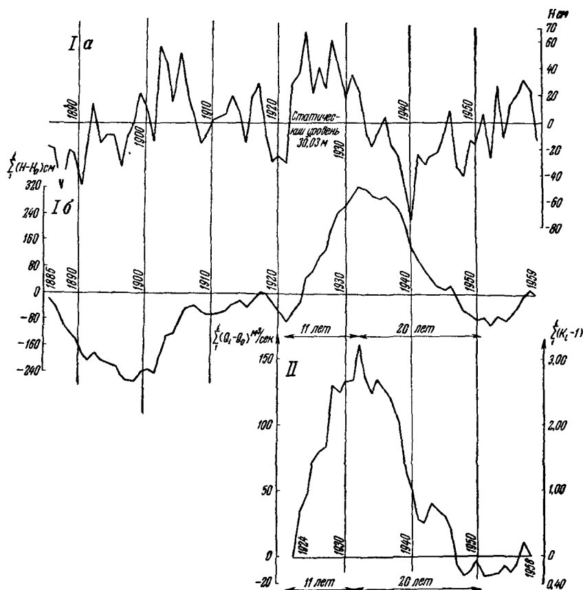
Рис. 48. Кривые цикличности поверхностного стока (по Т.Ф. Эйпре) Озеро Чудское, пост Муствез (период 1885—1959 гг.): Ia — отклонение средних годовых уровней от среднего многолетнего уровня (см); Ib — интегральная кривая отклонений средних годовых уровней от среднего многолетнего уровня Река Пярну, пост Орекюла (период 1922—1958 гг.): II — интегральная кривая отклонений расходов — среднегодовых от среднемноголетних ( Q_0=49,9 \text{ м}^3/\text{сек} ), или разностная интегральная кривая модульных коэффициентов
