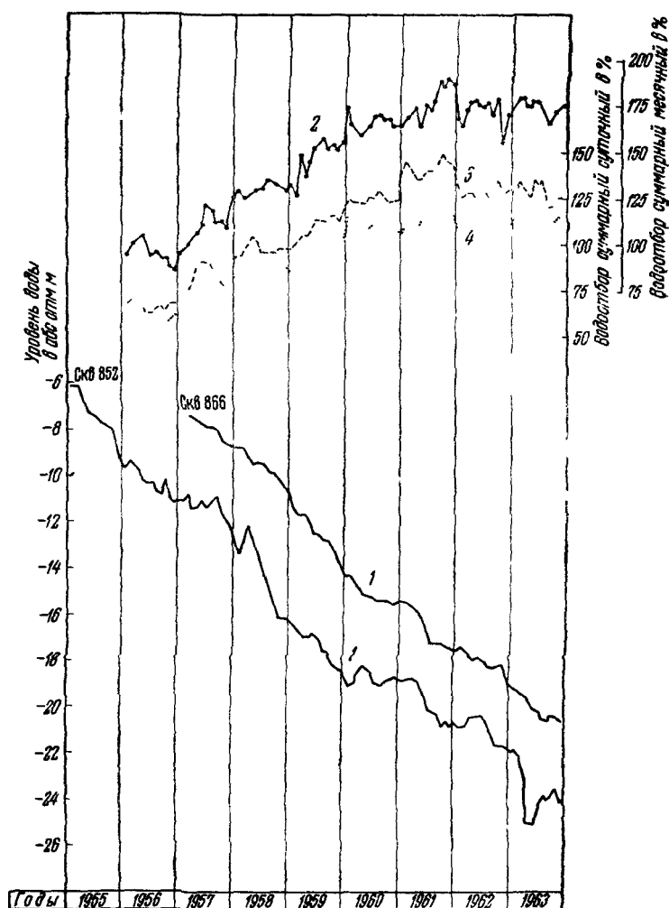
Рис 57 График зависимости изменения уровня воды по скважинам от суммарного водоотбора в зоне г. Кохтла-Ярве в период с 1956 по 1963 г.
