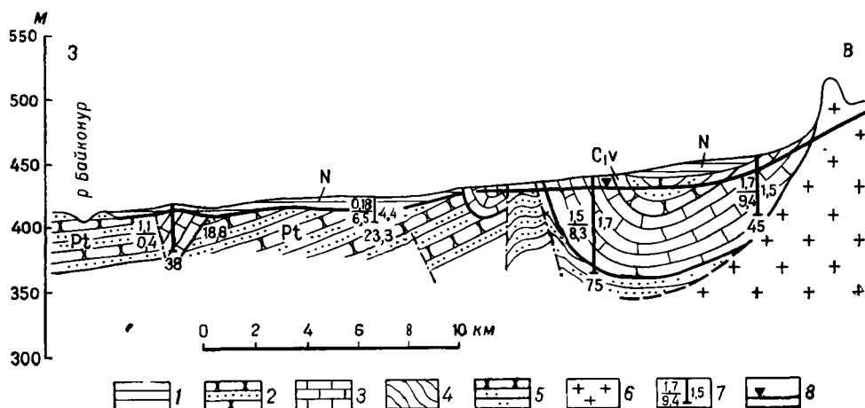
Рис. 20. Гидрогеологический разрез по приразломной Сарысайской мульде (составил М. А. Хордикийнен по материалам В. Н. Островского)
