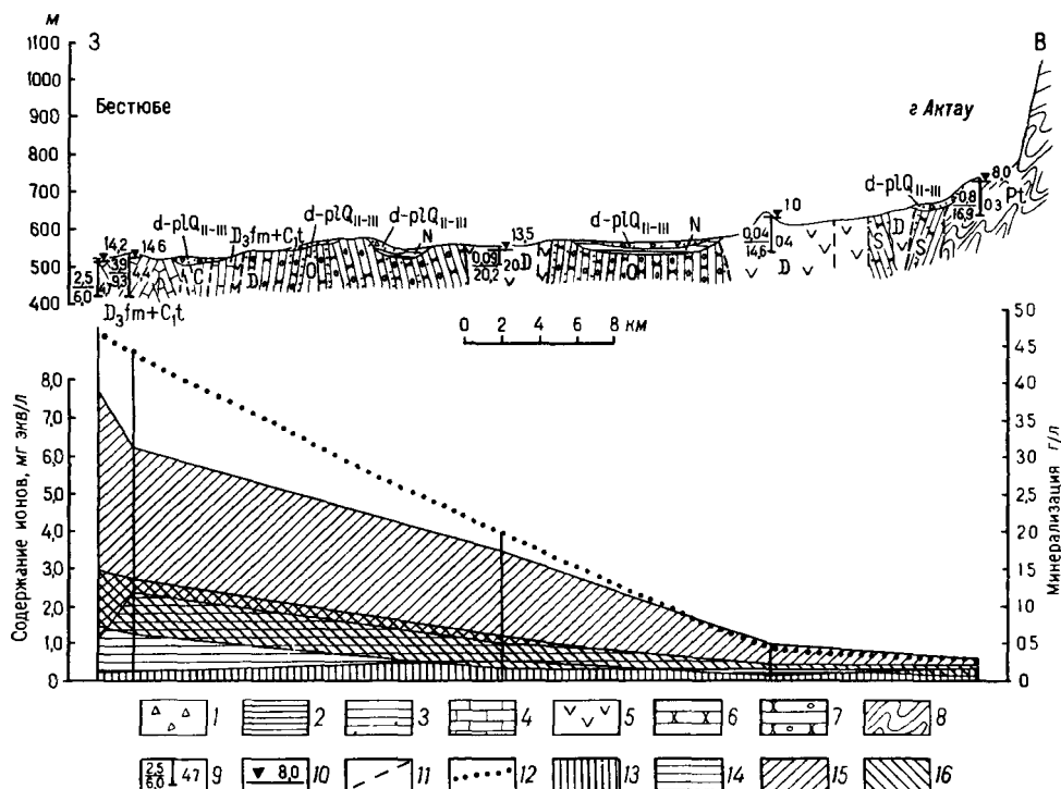
Рис 43 Гидрогеологический разрез и гидрохимический профиль восточного крыла Джаильминской синклинали по линии Бестюбе-Актау (составил Л. Я. Тененбаум) 1 — воды спорадического распространения делювиально-пролювиальных средне-верхнечетвертичных отложений ( dplQ_{II-III} ). Супеси и суглинки с линзами песков; 2 — водоупорные пестроцветные неогеновые глины ( N ); 3 — водоносный комплекс осадочных каменноугольных отложений ( C ) Аргиллиты, пересланяющиеся с алевролитами и песчанками; 4 — водоносный комплекс карбонатных фаменских и турнейских отложений ( D_3fm-C_{1t} ) Известняки; 5 — подземные воды зоны открытой трещиноватости эффузивных девонских пород ( D ) Порфириды, альбитофиры, туфы; 6 — водоносный комплекс осадочных силурийских отложений ( S ) Песчанники и алевролиты; 7 — водоносный комплекс осадочных ордовикских отложений ( O ) Песчанники с прослоями конгломератов и алевролитов; 8 — подземные воды зоны открытой трещиноватости метаморфических протерозойских пород ( Pt ) Кварциты и метаморфические сланцы; 9 — скважины слева в числителе — дебит (л/сек), в знаменателе — понижение (м), справа — минерализация воды (г/л); 10 — уровень подземных вод; 11 — тектонические нарушения, на гидрохимическом профиле; 12 — линия общей минерализации воды (г/л); содержание ионов (мг.экв/л) 13 — HCO_3^- , 14 — SO_4^{2-} , 15 — Cl^- , 16 — Mg^{2+} Содержание Ca^{2+} откладывается от нуля графика
