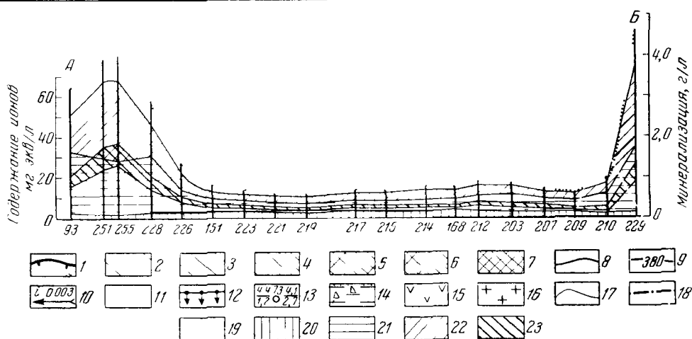
Рис 49 Гидрогеологическая карта низовья долины р Токрау (составил В. И Андру севич по материалам К И Сычева и К И Ишмакова)
