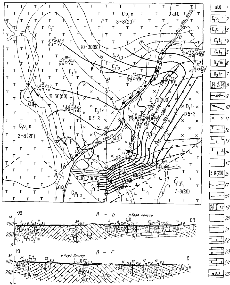
Рис 23 Гидрогеологическая карта Айдооской антиклинали (составили М. А. Хор дикий и А. А. Емельянов)
