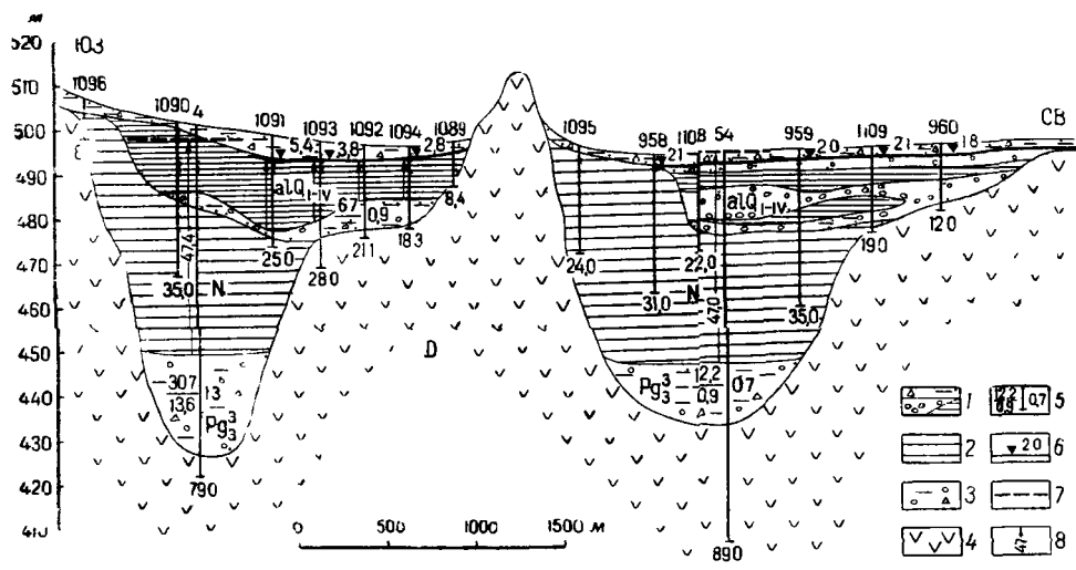
Рис 28 Гидрогеологический разрез Жаргас-Котурского участка долины р. Джон по линии В—Г (составила Э. Д. Кузьмина по материалам В. А. Курдюкова)
