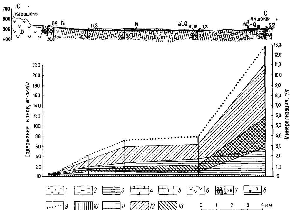
Рис. 42 Гидрогеологический разрез и гидрохимический профиль центральной части Джанильминской синклинали по линии Карашоки-Акшоки (составил Л. Я. Тененбаум) 1 — водоносный горизонт аллювиальных среднечетвертичных — современных отложений (alQ II-IV ) Пески с гравием, супеси; 2 — воды спорадического распространения делювиально-пролювиальных верхнеплиоценовых — верхнечетвертичных отложений (N 2 2 —Q III ). Супеси и суглинки с линзами песков; 3 — водоупорные пестроцветные неогеновые глины (N); 4 — водоносный комплекс осадочных каменноугольных отложений (C). Аргиллиты, алевролиты, песчаники; 5 — водоносный комплекс карбонатных фаменских и турнейских отложений (D 3fm —C it ) Известняки, 6 — подземные воды зоны открытой трещиноватости эффузивных девонских пород (D) Порфириты, альбитофиры, туфы; 7 — скважины: слева в числителе — дебит (л/сек), в знаменателе — понижение (м), справа — минерализация воды (г/л); 8 — уровень подземных вод; на гидрохимическом профиле: 9 — линия общей минерализации воды (г/л); содержание ионов (мг·экв/л), 10 — HCO 3 - ; 11 — SO 4 2- ; 12 — Cl - ; 13 — Mg 2+ . Содержание Ca 2+ откладывается от нуля графика
