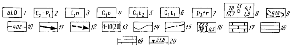
Рис 22 Гидрогеологическая карта Жанайской антиклинали (составил М. А. Хорди-кайнен по материалам С. К. Калугинна)
