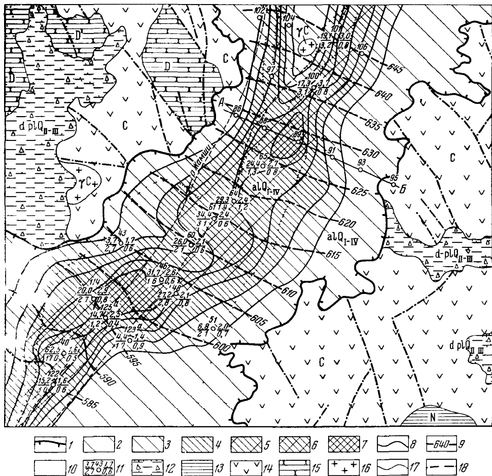
Рис 45 Гидрогеологическая карта Акжальского участка долины р Жамши (составила Л. А. Денисова по материалам Е. А. Кожевниковой и В. Г. Логинова)
