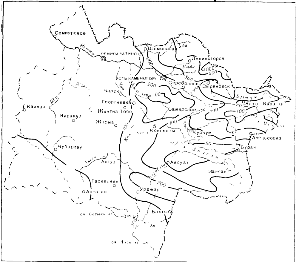
Рис. 11 Карта распределения твердых осадков в изотоничном слое воды в мм (по Р. И. Гальперину)
