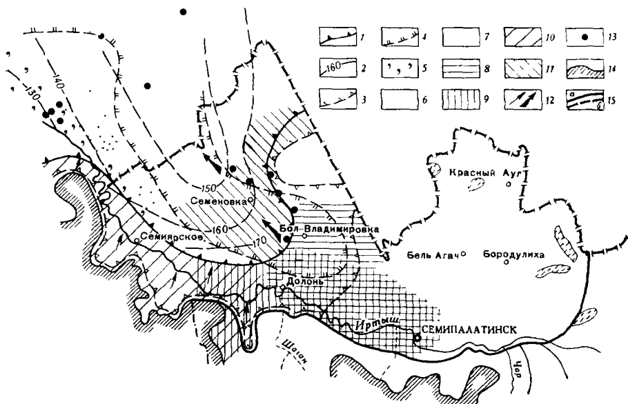
Рис 31. Схематическая гидрогеологическая карта водоносного комплекса нерасчлененных меловых отложений Иртышского артезианского бассейна (составила Б. Е. Антипо)
