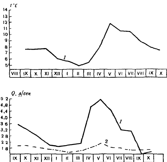
Рис. 34 График колебаний температуры и расходов грунтовых трещинных вод по родникам из осадочных пород палеозоя в центральной части Калбинского хребта (составила Г. Х. Казовская) 1 — родник № 5, 2 — родник № 15
