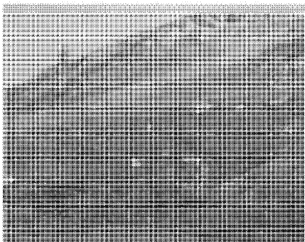
Рис 23. Южный Алтай. На переднем плане карстовая воронка в известняках
