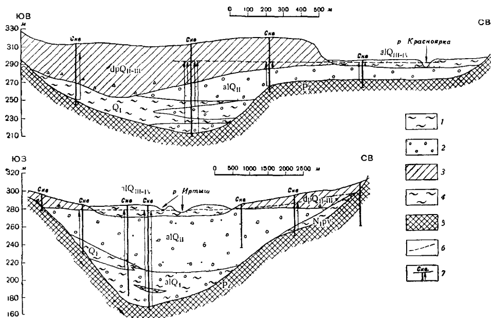
Рис. 21 Гидрогеологические разрезы долины р. Красноярки выше ст. Предгорное и долины р. Иртыша у г. Усть-Каменогорска (составил В. И. Белянин) — песок глинистый, 2 — гравийно-галечные отложения (участками заглинизированные) 3 — супесь с обломками коренных пород 4 — глина, 5 — палеозойские породы, 6 — уровень подземных вод, 7 — пьезометрические уровни по скважинам
