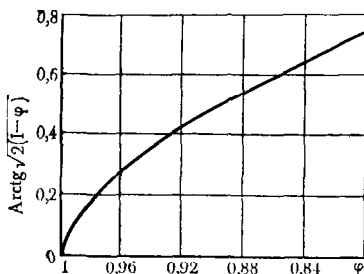
Рис. IV.10. Зависимость \operatorname{Arctg} \sqrt{2(1-\varphi)} от \varphi
