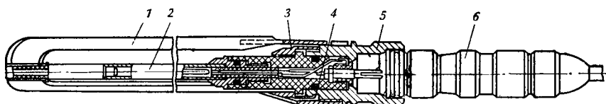
Рис. II.18. Термокондуктивный расходомер СТД:
