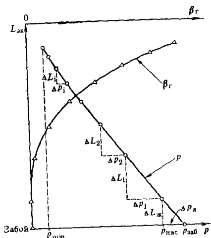
Рис. VI.6. Изменение давления и объемной расходной доли свободного газа \beta_g в потоке вдоль ствола скважины при постоянном дебите жидкости
