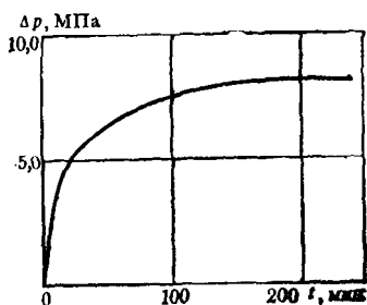
Рис. 1.11. Кривая восстановления давления
