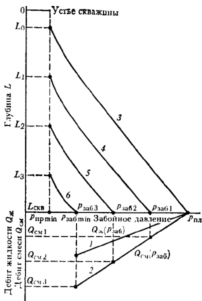
Рис. IV.7. Определение максимального отбора жидкости из скважины: 1 — граница добычных возможностей установки; 2 — зависимость производительности системы (по газожидкостной смеси) от глубины спуска насоса
