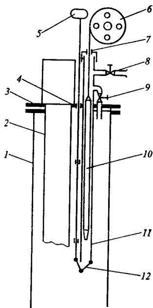
Рис. II.4. Схема оборудования устья насосной скважины для спуска приборов в межтрубное пространство:
