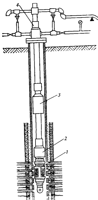
Рис. VIII.22. Схема оборудования скважины при виброобработке забоя:
