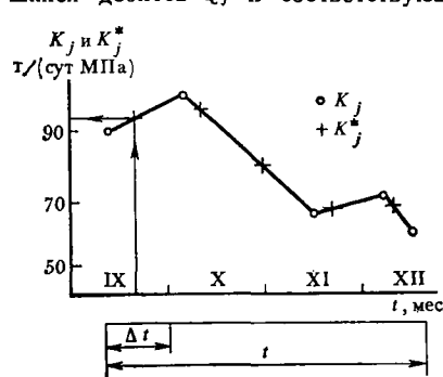
Рис. VIII.5. Изменение коэффициента продуктивности скважины во времени
