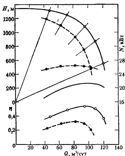
Рис. VI.9. Водяная характеристика погружного центробежного электронасоса при работе на воде и на водонефтяной эмульсии
