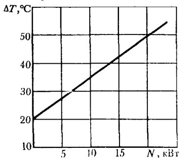
Рис. VII.5. Зависимость перепада температуры между скважинной жидкостью и начальной пластовой от мощности электронагревателя
