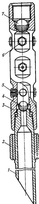
Рис. VIII.9. Перфоратор ПЗК:
