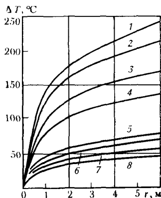
Рис. VII.12. Изменение избыточной скважинной температуры от радиуса зоны воздействия в нефтенасыщенном песчанике:
