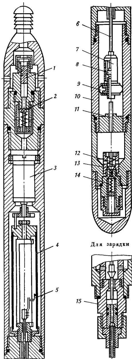
Рис. II.10. Схема дифманометра ДГМ-4М:
