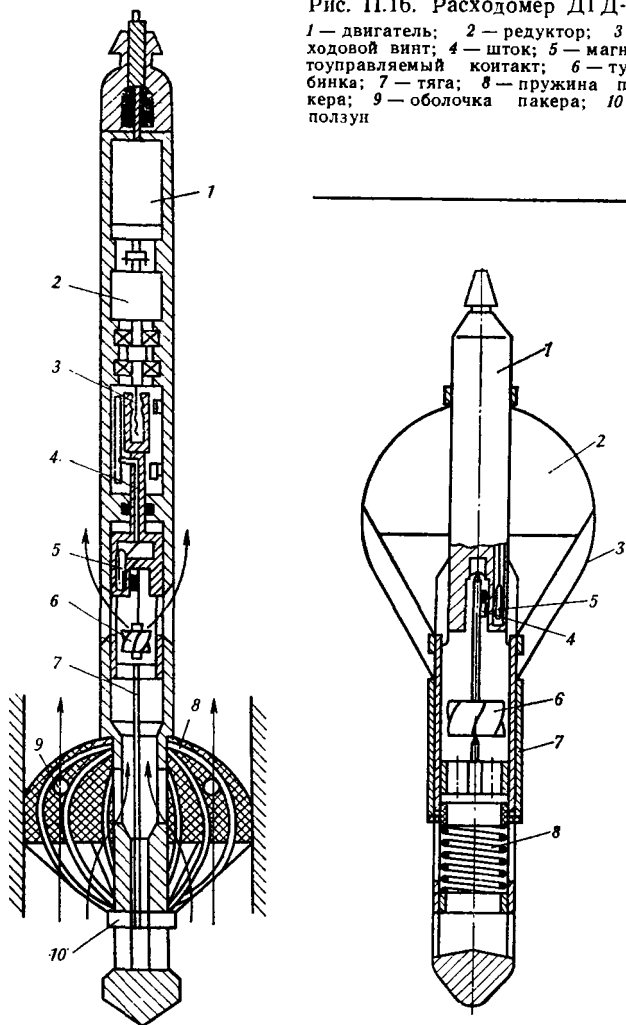
Рис. II.17. Расходомер «Терек-3» с бесприводным пакером:
