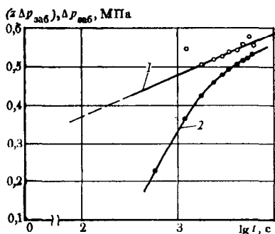
Рис. 1.8. К примеру обработки кривой восстановления давления с учетом дополнительного притока дифференциальным методом:
