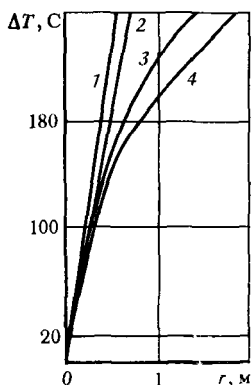
Рис. VII.14. Изменение избыточной скважинной температуры от радиуса зоны воздействия в заглинзировавшем пласте (обозначения см. на рис. VII.12)
