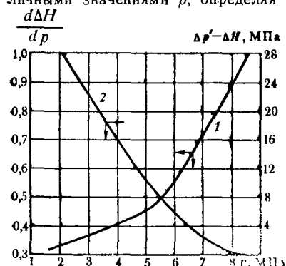
Рис. 1.3. Зависимость подынтегральной функции d\Delta H/dr и поправки (\Delta p' - \Delta H) от давления
