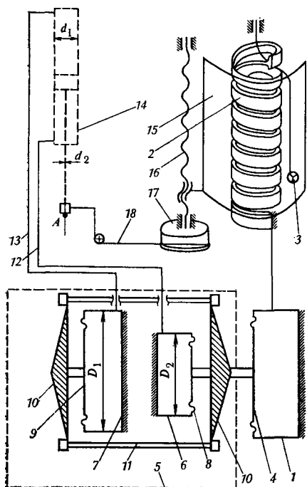
Рис. V.9. Схема гидравлического динамографа:
