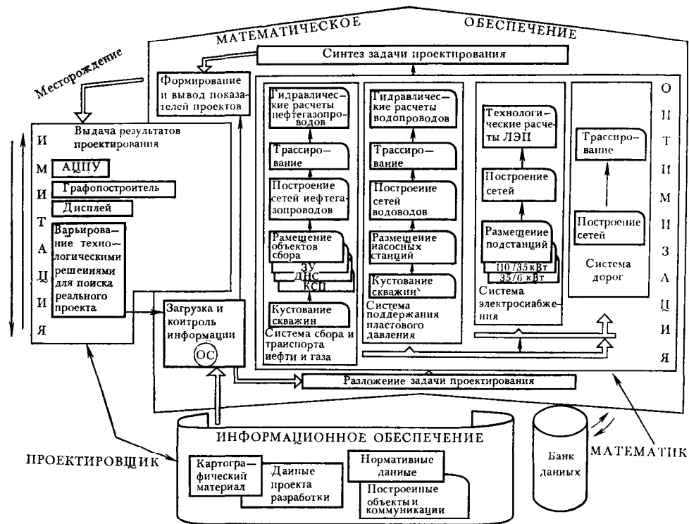
Рис. II.1. Схема функционирования Системы проектирования генеральных схем обустройства нефтяных месторождений на ЭВМ
