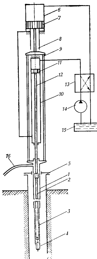
Рис. V.1. Принципиальная схема штанговой гидроприводной глубиннонасосной установки типа АГН:
