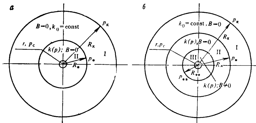
Рис. 1.5. Характерные зоны фильтрации вокруг скважин
