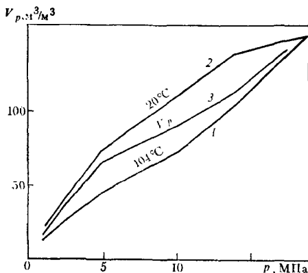
Рис. III.1. Схематическая зависимость между количеством растворенного газа и давлением:
