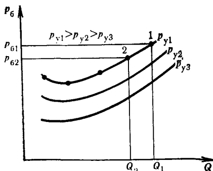
Рис. III.13. Характеристические кривые
