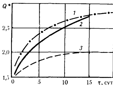
Рис. VII.8. Изменение относительного дебита Q^* (отношение текущего дебита при прогреве к дебиту непрогретой скважины) при граничном условии 1-го рода: 1, 2 — Z=80 ; 3 — Z=20 . Удельный дебит в момент пуска q_0=0,005 м 3 /м·ч. Соотношение проницаемостей k/k_a=6 ; 1 — прогрев начал через три месяца после начала эксплуатации; 2 и 3 — прогрев начинается одновременно с началом эксплуатации
