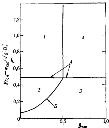
Рис. VI.1. Карта структурных форм водонефтяного и водонефтегазового потоков в колонне подъемных труб и в стволе скважины. 1 — w_{cm} \geq 0,487 \sqrt{g d_r} , \beta_{vж} \leq 0,5 ; эмульсионная структура водонефтяного потока типа В/Н; эмульсионно-пузырьковая структура водонефтегазового потока типа (B+\Gamma)/H , если \varphi_r \leq 0,65 или p \geq 7 МПа; эмульсионно-снарядная структура водонефтегазового потока типа (B+\Gamma)/H , если \varphi_r \leq 0,65 при p \leq 7 МПа;
