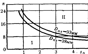
Рис. IV.3. Области применимости формул для определения максимальной и минимальной нагрузок
