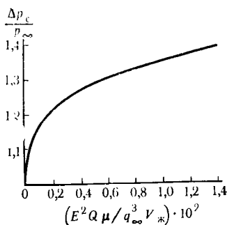
Рис. VIII.16. График зависимости \Delta p_c/p_{\infty} от E^2 Q \mu / q_{\infty}^3 V_{ж}
