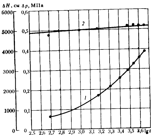
Рис. 1.9. Обработка результатов прослеживания уровня в нагасной скважине
