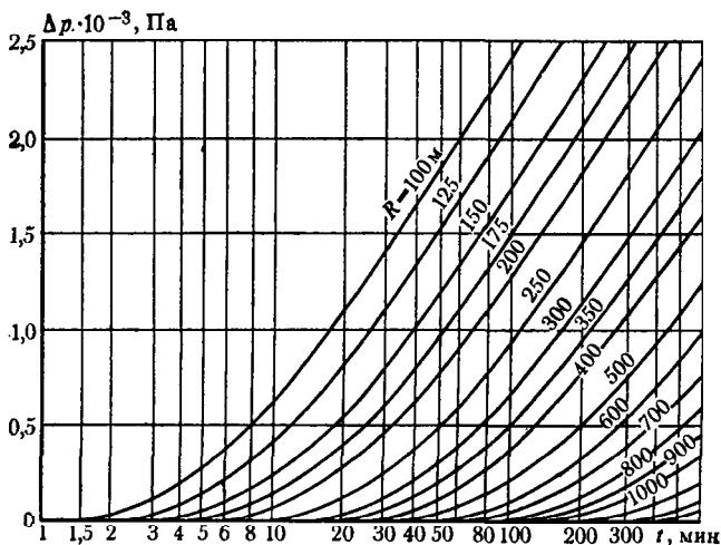
Рис. 1.18. Эталонные кривые \Delta p(t) - t для различных расстояний R между возмущающей и реагирующей скважинами
