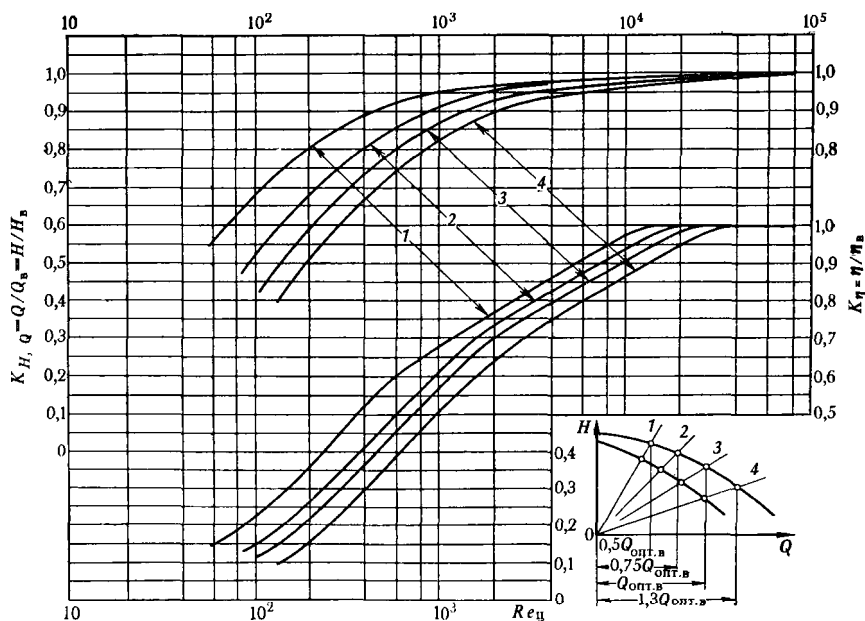
Рис. VI.8. Зависимость относительных подачи и напора K_Q и относительного к. п. д. K_\eta погружного центробежного насоса от модифицированного числа Re_\psi потока в его меллопаточных каналах для различных соответственных режимов Q_v/Q_{опт.в} :
