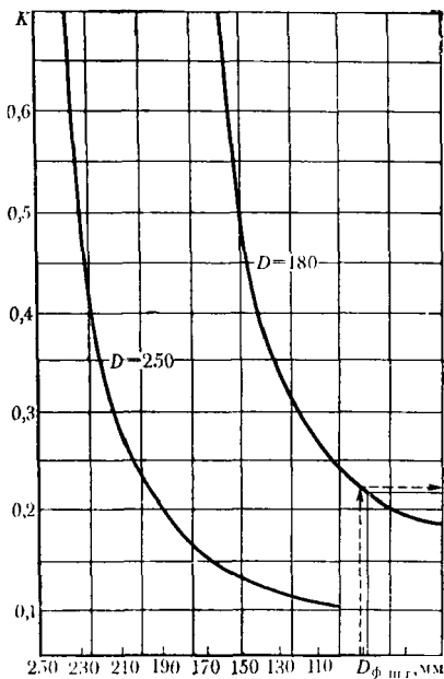
Рис. V.5. Номограмма для определения диаметра фальшштока
