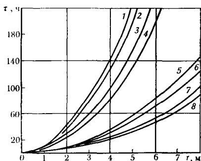
Рис. VII.9. Продолжительность обработки нефтенасыщенного песчаника в зависимости от радиуса зоны воздействия:
