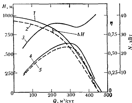
Рис. VI.7. Характеристика насоса 13ЦН6-250-800 при работе на воде по паспортной характеристике.
