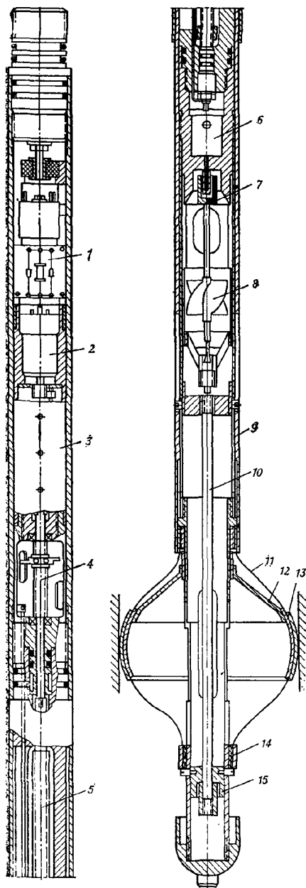
Рис. II.14. Скважинный расходомер РГД-2М:
