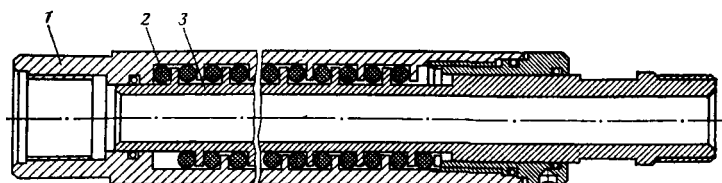
Рис. VIII.23. Амортизатор:
