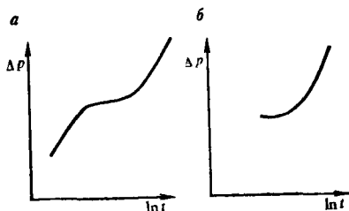
Рис. I.10. Формы кривых восстановления давления для трещиноватых коллекторов
