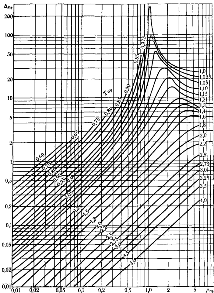
Рис. VI.3. Изотермическая поправка на давление к изобарной теплоемкости \Delta c_p для газов и паров
