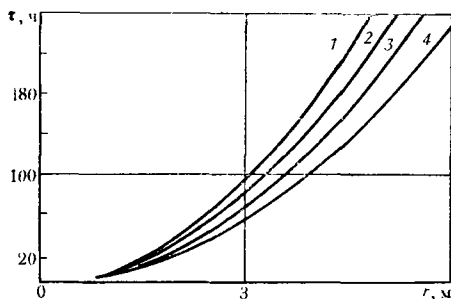
Рис. VII.10. Продолжительность обработки водонасыщенного песчаника в зависимости от радиуса зоны воздействия (обозначения см. на рис. VII.9)
