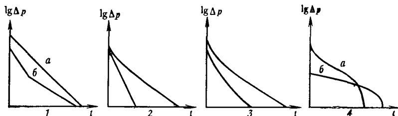
Рис. VIII.2. Типовые конфигурации графиков восстановления давления в зависимости от типа дренируемого коллектора:
