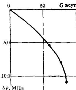
Рис. 1.12. Индикаторная линия
