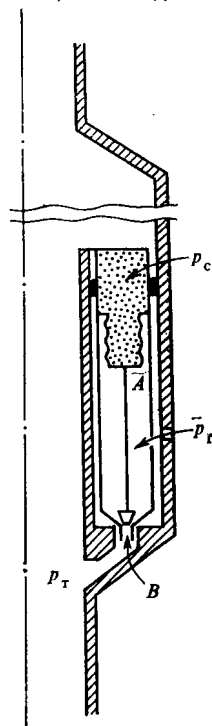
Рис. III.23. Схема сильфонного газлифтного клапана
