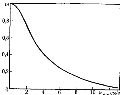
Рис. III.11. График для определения поправочного коэффициента m в зависимости от приведенной скорости нефти или воды
