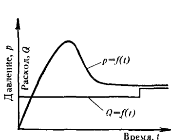
Рис. VIII.12. Изменение расхода и давления при гидравлическом разрыве пласта с образованием новых трещин
