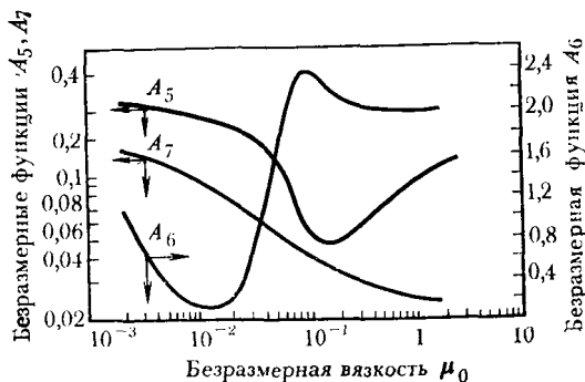
Рис. III.8. Зависимость безразмерных функций A_5 — A_7 от безразмерной вязкости \mu_0 .
