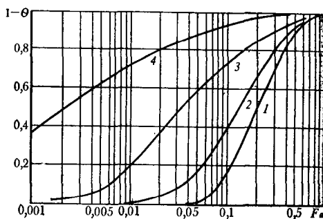
Рис. VII.6. Снижение безразмерной температуры от F_0 для различных точек пласта после обработки:
