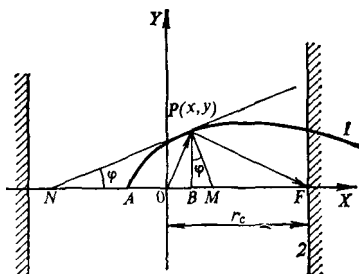
Рис. VIII.28. Схема строения отражателя, фокусирующего импульсы давления на стенке скважины в одну линию по окружности:
