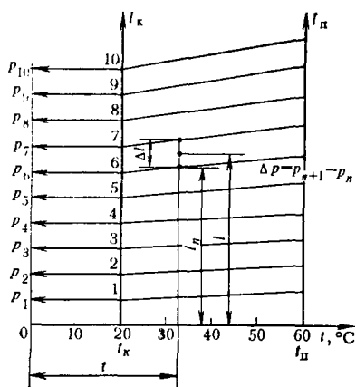
Рис. II.8. Градуировочный график манометра:
