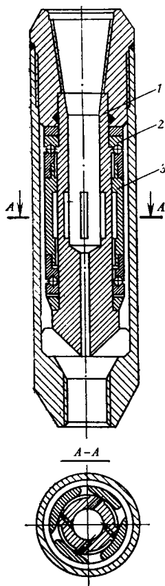
Рис. VIII.19. Гидравлический вибратор золотникового типа ГВЗ:
