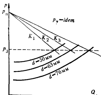
Рис. III.14. Определение диаметра колонны НКТ для фонтанной скважины
