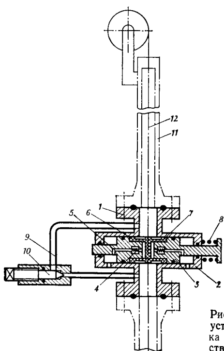
Рис. II.3. Устройство для предотвращения и ликвидации аварий
