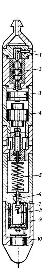
Рис. II.6. Автономный манометр МГН-1 с вращающимся поршнем:
