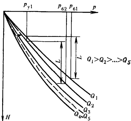
Рис. III.12. Схематическое распределение давления по длине колонны НКТ при различных дебитах скважины Q_1=1,2,3,4,5
