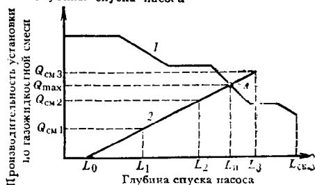
Рис. IV.7. Определение максимального отбора жидкости из скважины: 1 — граница добычных возможностей установки; 2 — зависимость производительности системы (по газожидкостной смеси) от глубины спуска насоса
