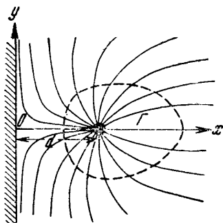
Рис. 8. Схема линий тока в полуограниченном пласте с непроницаемым контуром z — область квазирадialного течения
