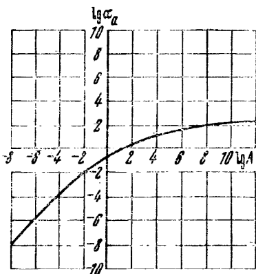
Рис. 15. График зависимости A = f(\alpha_a) (по Ф. М. Бочеверу и В. М. Шестакову)
