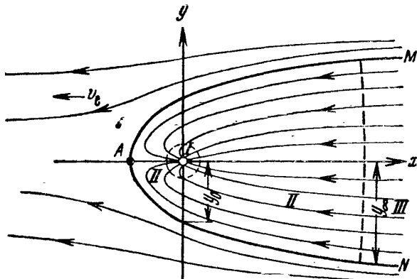
Рис. 4. Структура фильтрационного течения к водозабору в неограниченном пласте в условиях потока I — область плоско-радиального течения; II — область плоско-криволинейного течения; III — область плоско-параллельного течения
