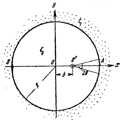
Рис. 23. Схема круговой линзы пресных вод
