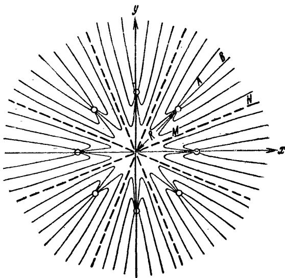
Рис. 16. Схема линий тока к кольцевой батарее скважин в неограниченном пласте
