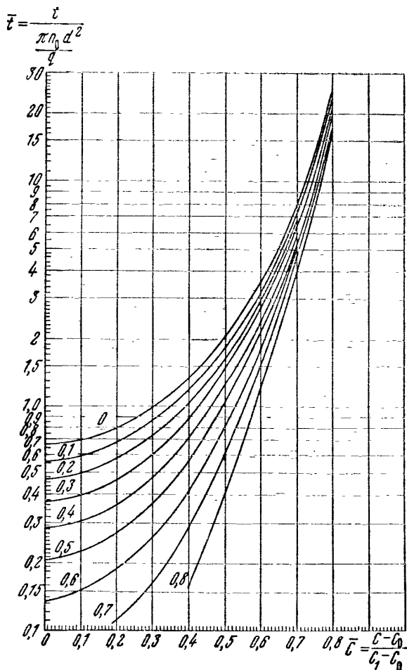
Рис. 26. График зависимости \bar{t} = f(\bar{C}, \bar{x}_1) для одиночного водозабора в полуограниченном пласте с контуром постоянного напора в условиях бассейна при подтягивании соленых вод со стороны контура
