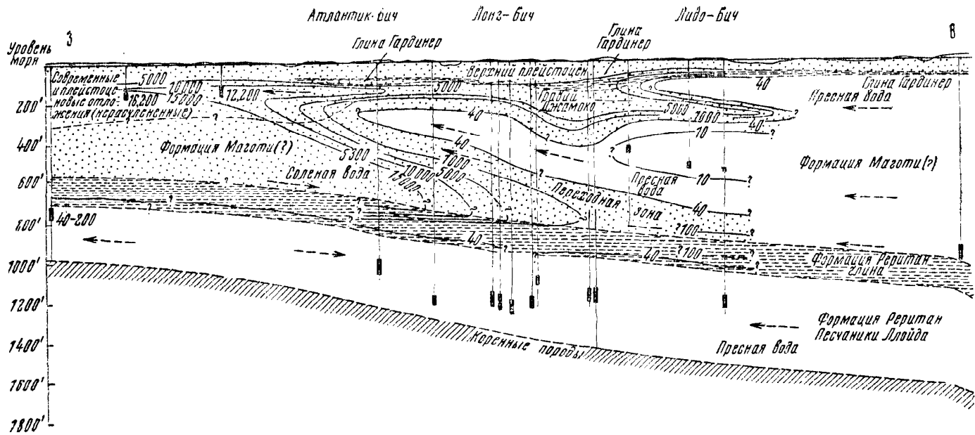
Рис. 1. Вторжение морских вод в пресные подземные воды четвертично-мелового комплекса на побережье Атлантического океана в штате Нью-Джерси, США (по И. Апсону).
