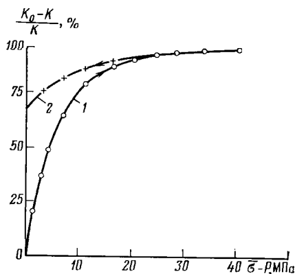
Рис. 4.18. График зависимости относительного изменения проницаемости (K_0 - K)/K от эффективного давления (\sigma - P) для трещиноватого известняка Кортней (Парижский бассейн) [5]. Кривые: 1 — сжатия; 2 — снятия нагрузки
