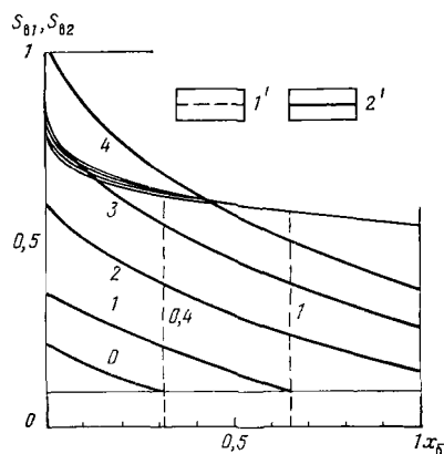
Рис. 9.65. Распределение водонасыщенности \rightarrow S_{в1} (1') и S_{в2} (2') в трещиновато-пористой среде для \mu_6=1,25 [19]. Шифр кривых — t_6
