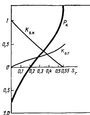
Рис. 11.19. Псевдофункции капиллярного давления и относительных проницаемостей при давлении 38,23 МПа [7]
