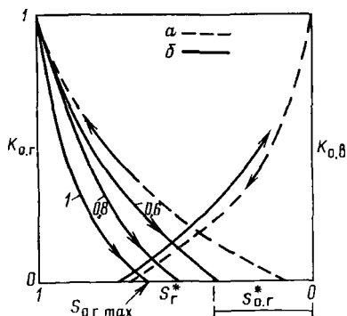
Рис. 4.42. Влияние начальной газонасыщенности S_{г.нач}^* на кривые относительной проницаемости при дренаже и при пропитке
