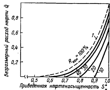
Рис. 10.16. Зависимость безразмерного расхода нефти Q от средней нефтенасыщенности S_n^* при различных величинах нефтеотдачи R_{\text{кон}} (1 — кривая относительной проницаемости для нефти) [2]
