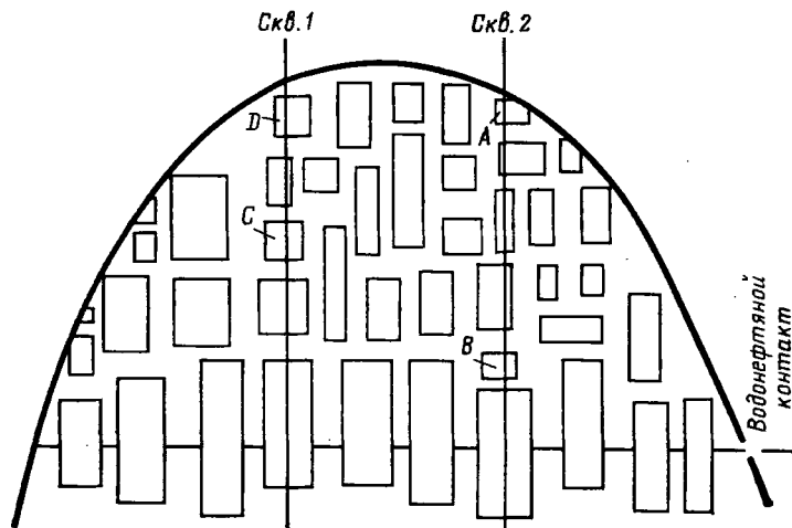
Рис. 4.19. Трещиноватый пласт-коллектор, образованный блоками матрицы различного размера. А, В, С, D — блоки матрицы
