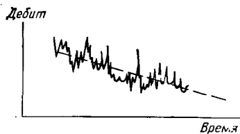
Рис. 10.30. Изменение дебита во времени по промысловым данным
