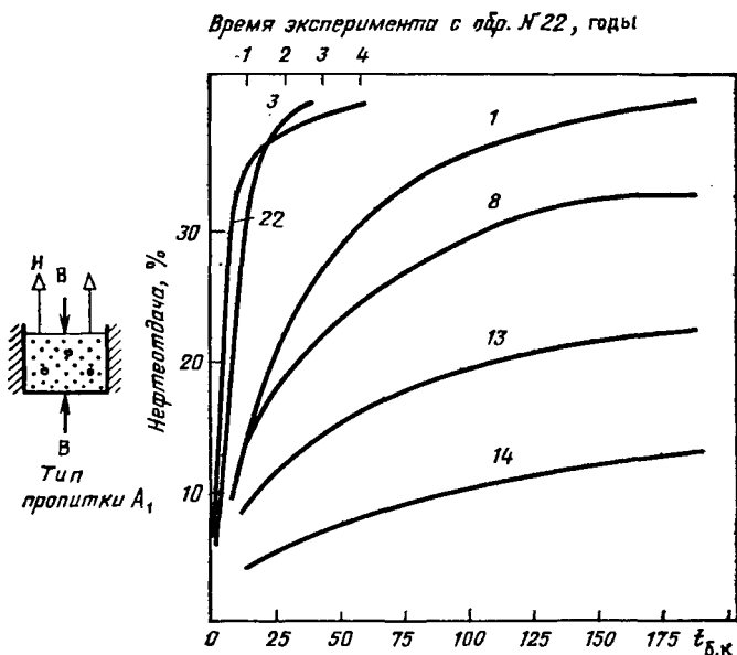
Рис. 9.53. Зависимость нефтеотдачи от t_{d,k} для различных значений капиллярно-гравитационного отношения CGR [11].
