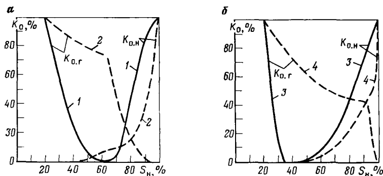
Рис. 4.44. Кривые зависимости относительной проницаемости K_o от нефтенасыщенности S_n по данным табл. 4.18 [31]
