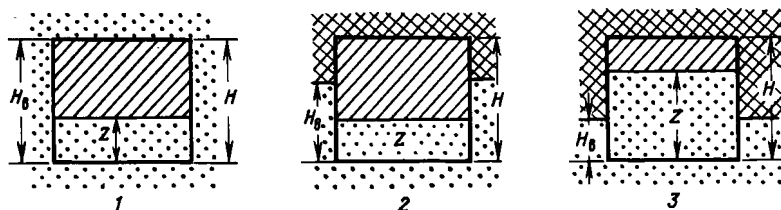
Рис. 9.31. Относительные перемещения ВНК в трещинах и блоках матрицы. Положение ВНК в трещине равно глубине погружения блока в воду. Погружение блока: 1 — полное, H_{\text{в}} = H при Z = 0 ; 2 — частичное, Z < H_{\text{в}} < H ; 3 — частичное, H_{\text{в}} < Z < H ( H_{\text{в}} — положение ВНК в трещине; Z — положение ВНК в матрице)
