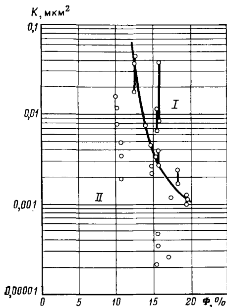
Рис. 4.24. График зависимости K — \Phi для трещиноватых образцов керна.
