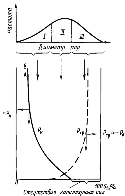
Рис. 4.63. Характер изменения капиллярных P_K и гравитационных P_{Gr} сил в зависимости от насыщенности S_B пласта-коллектора и распределения пор по размерам.
