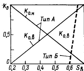
Рис. 4.46. Кривые зависимости относительной проницаемости K_o от водонасыщенности S_w [22]
