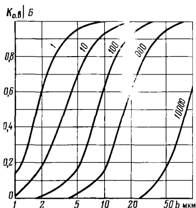
Рис. 4.53. Кривые зависимости K_{0.в}/B от ширины трещин b для различных значений aK_M в случае идеализированной модели пласта-коллектора с кубическими блоками.
