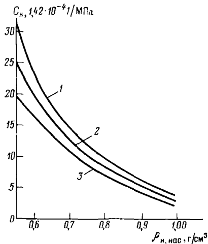
Рис. 4.32. График зависимости сжимаемости нефти ( P > P_{\text{нас}} ) от ее плотности при P_{\text{нас}} .
