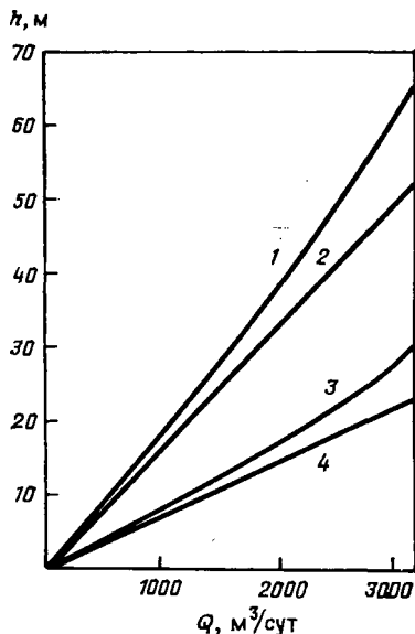
Рис. 6.23. Кривые зависимости критической и безопасной высот конусов h_v и h_r от дебита Q .
