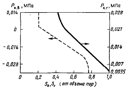
Рис. 12.4. Средние капиллярные давления для систем нефть—вода, нефть—газ месторождения Хафт-Кел [1]
