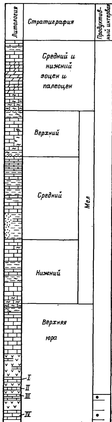
Рис. 3.7. Типичный разрез отложений на месторождении Духан (Даниэль, 1954).
