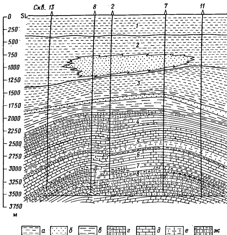
Рис. 3.12. Геологические разрезы месторождения Джела [9].
