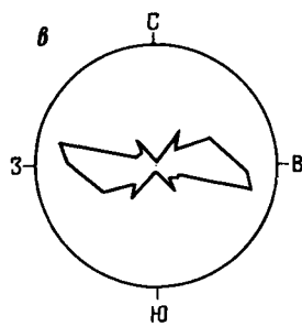
Рис. 2.40. Распределение напряжений сжатия (а) при наличии горизонтальных левосторонних (б) и правосторонних (в) зеркал скольжения
