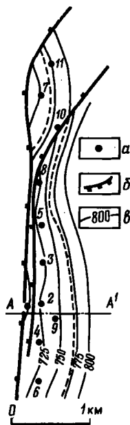
Рис. 2.43. Структурная карта месторождения Айшау [8]. а — скважины разного назначения; б — нормальный сброс; в — изогипсы, м
