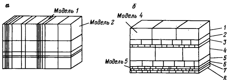
Рис. 2.21. Идеализированные породы:
