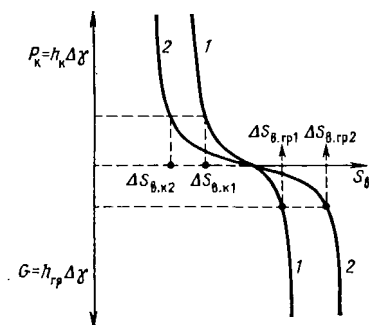
Рис. 9.24. Капиллярные кривые, соответствующие двум типам (1 и 2) пород с различными размерами пор
