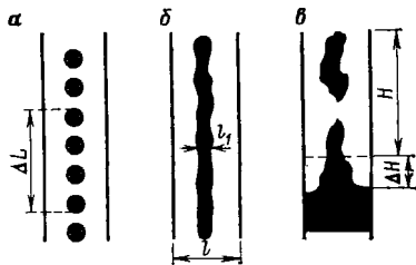
Рис. 4.55. Измерения насыщенности в трещине в процессе сегрегации.
