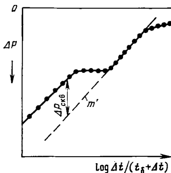
Рис. 7.17. Кривая восстановления давления \Delta P - \log \Delta t / (t_b + \Delta t) в скважине в трещиноватом пласте для случая ограниченного (конечного) пласта
