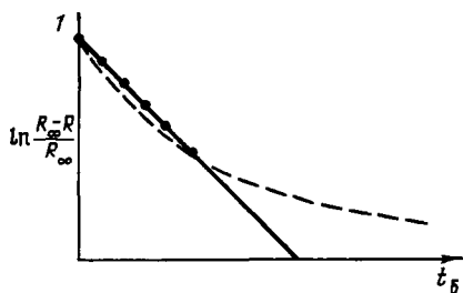
Рис. 9.34. Зависимость относительной нефтеотдачи от безразмерного времени
