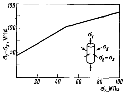
Рис. 1.22. Прочностные характеристики известняка при долговременнои нагружении
