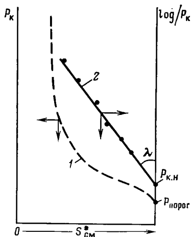
Рис. 4.38. Кривые зависимости P_K - S_{см}^* в обычных (1) и полулогарифмических (2) координатах ( S_{см}^* = (S_{в.о} - S_{в.о}) / (1 - S_{в.о}) )
