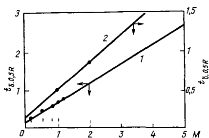
Рис. А.4. Зависимость времени t_{6,0,5R} от M при преобладании гравитационных (1) и капиллярных (2) сил
