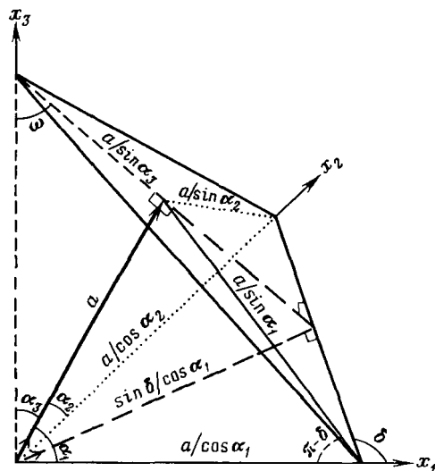
Рис. 2.5. Ориентация трещин в декартовой системе координат. \delta — азимут; \omega — угол падения
