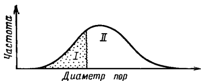
Рис. 4.35. Кривая распределения пор по размерам и флюидонасыщенность. Фазы: I — смачивающая; II — несмачивающая
