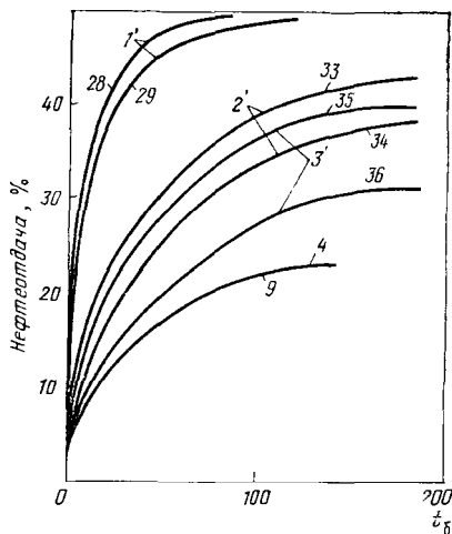
Рис. 9.48. Зависимость нефтеотдачи от безразмерного времени t_6 для различных типов жидкостей и разных физических характеристик образцов [11] при капиллярной пропитке по типу A_2 (см. рис. 9.47):
