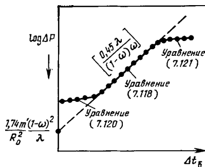
Рис. 7.18. Кривая восстановления давления \log \Delta P - \Delta t_b в скважине в трещиноватом пласте для случая ограниченного (конечного) пласта
