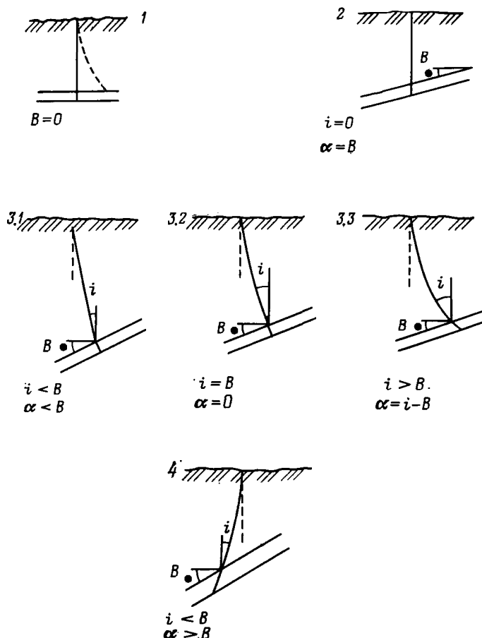
Рис. 2.18. Определение ориентации трещин в зависимости от направления (отклонения) ствола скважины (материалы Висёра).
