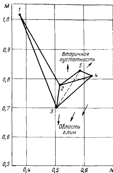
Рис. 5.23. График для выделения вторичной пустотности в породах с различным минералогическим составом (диаграмма литотипов).
