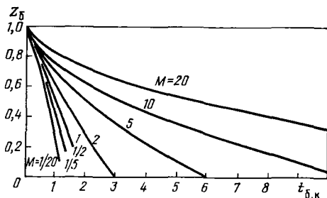
Рис. 9.6. Зависимость коэффициента вытеснения Z_\delta от времени t_{\delta,\kappa} при различных отношениях подвижностей M [1]
