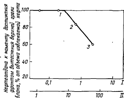
Рис. 9.38. Сопоставление положения ↑ ВНК в трещинах и фронта вытеснения в блоках матрицы при различных скоростях перемещения ВНК.
