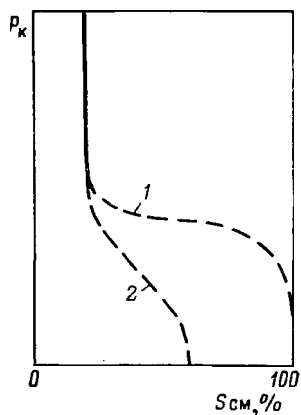
Рис. 4.57. Кривые капиллярного давления P_K при дренировании (1) и пропитке (2)
