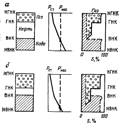
Рис. 10.10. Зональность залежей на поздних стадиях истощения до (а) и после (б) взаимопроникновения зоны вторгшегося газа и заводненной зоны.
