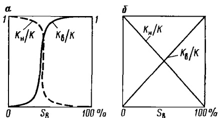
Рис. 4.34. Аномальные кривые зависимости относительной ( K_h/K и K_v/K ) проницаемости от водонасыщенности S_w .
