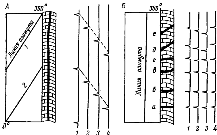
Рис. 5.10. Диаграмма наклонотрии в идеальном случае.
