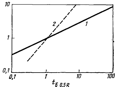
Рис. 9.55. Связь безразмерного времени \rightarrow t_{б.0.5R} и капиллярно-гравитационного отношения CGR для случаев капиллярной пропитки (1) и гравитационного вытеснения (2) [9]
