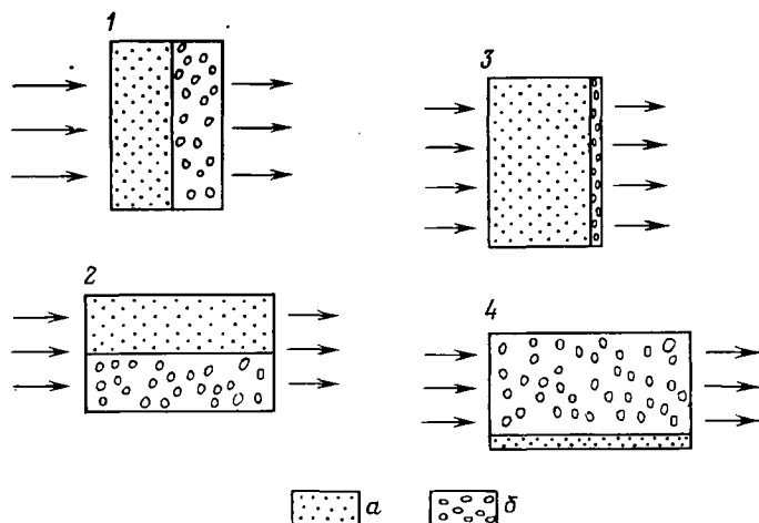
Рис. 4.43. Перпендикулярное и параллельное сочленение слоев. Слон с проницаемостью, мкм 2 : а — 0,1, б — 0,01. Случаи 1—4 см. в табл. 4.18.
