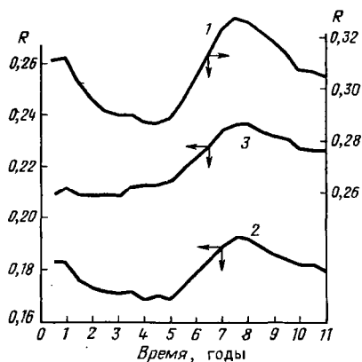
Рис. Е.5. Сопоставление кривых нефтеотдачи и чистой продукции во времени: 1 — R_g ; 2 — R_b ; 3 — P'/(V_{г,3} + V_{г,3})
