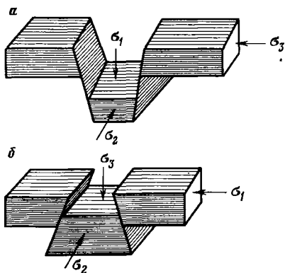
Рис. 1.12. Пример сбросообразования.
