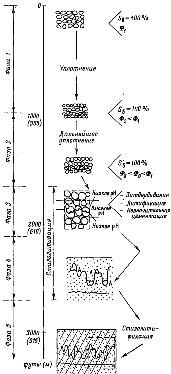
Рис. 1.30. Схема процесса стиололитизации и стиололитификации. S_g — водонасыщенность осадков; \Phi — пористость
