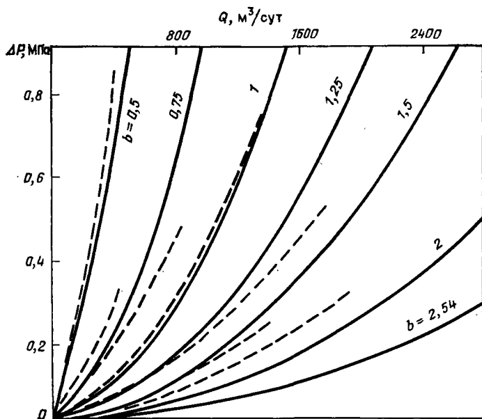
Рис. 6.15. Зависимость Q-\Delta P для различных значений раскрытости трещин, полученная в результате эксперимента на модели Бейкера. b — раскрытость трещины, мм
