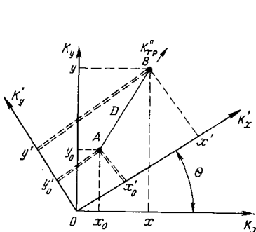
Рис. 8.12. Оценка угла \theta по наблюдениям и расчетным данным о падении давления. K''_{\text{тр}} — проницаемость трещины по главной оси
