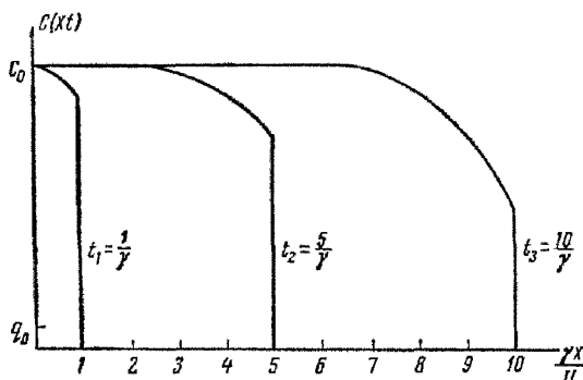
Рис. 29. Кривые распределения вещества в подвижной фазе при фильтрации в слабо сорбирующей среде
