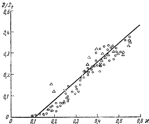
Рис. 7. Зависимость \frac{D}{D_0} от свободной пористости x для газов по данным Ван Бавела ( \Delta ), Лемана ( \Delta ) и Тейлора ( \bullet )
