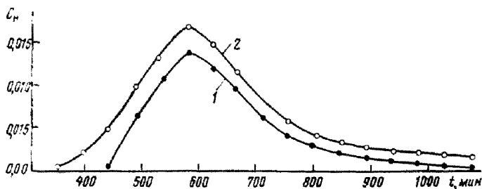
Рис. 35. Выходные кривые ионов меди (1) и хлора (2) при промывании раствором \text{CuCl}_2 через колонку
