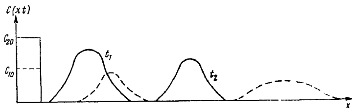
Рис. 31. Размывание полосы из двух сорбирующих веществ при фильтрации
