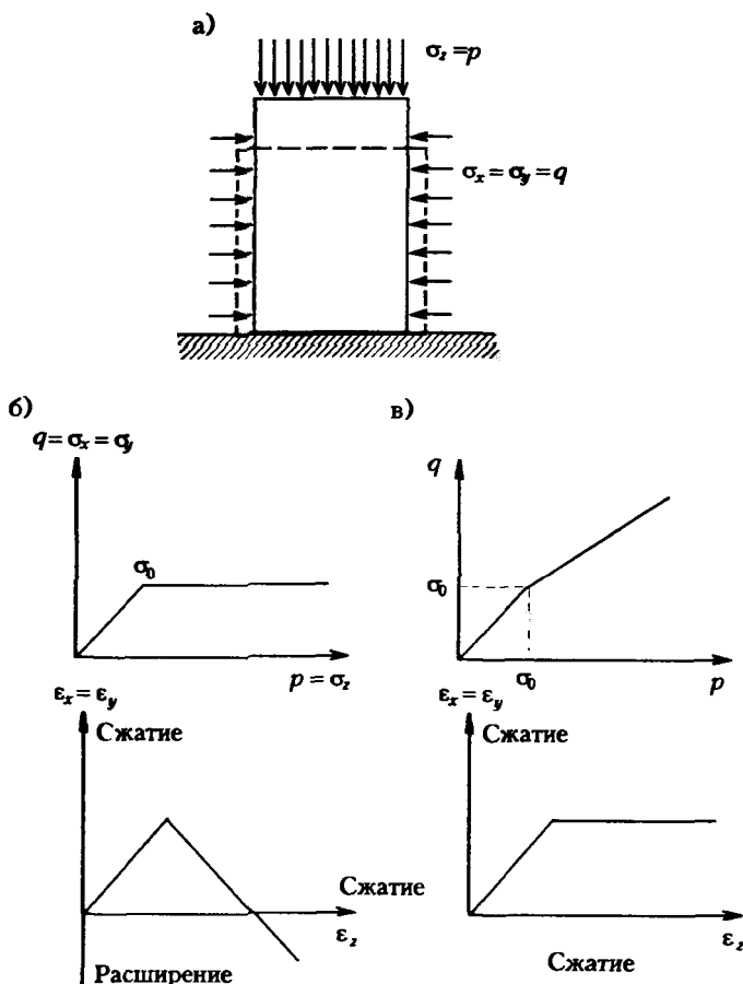
Рис.М.4.9. Стабилометр:
