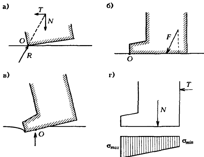
Рис.М.12.18. Схема для расчета устойчивости на опрокидывание:
