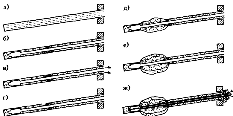
Рис.Ф.13.9.Б. Технология устройства анкера с инъекционной трубой
