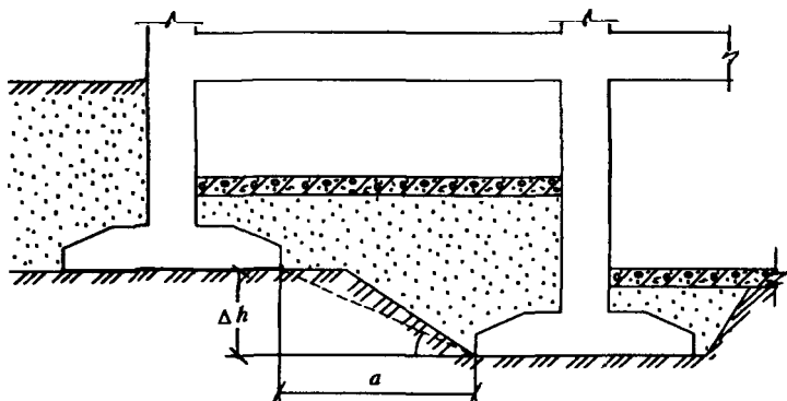
Рис.Ф.9.4. Заложение соседних фундаментов на разной глубине
