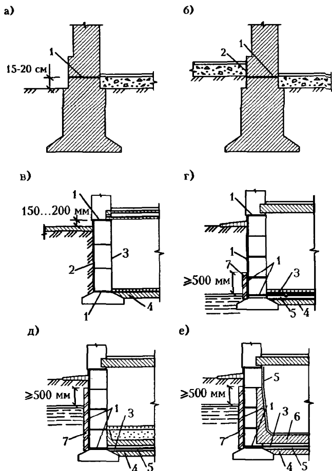
Рис.Ф.17.16. Гидроизоляция:
