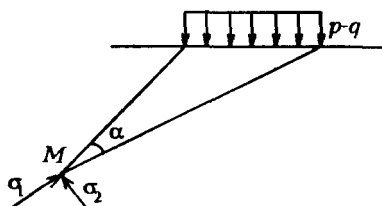
Рис.М.12.5. Определение критической нагрузки на грунт в условиях плоской деформации при \sigma_1 > \sigma_2 :
