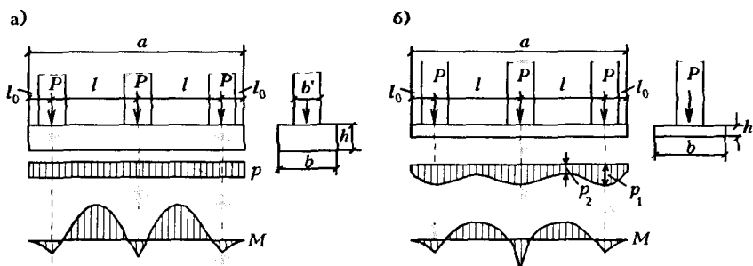
Рис.Ф.12.3. Распределение реактивных давлений по подошве фундаментов:
