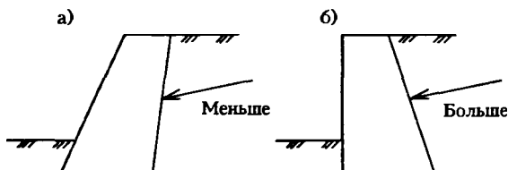
Рис.М.14.10. Влияние наклона задней грани стены на величину активного давления грунта на нее
