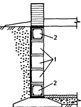
Рис.Ф.9.16. Устройство железобетонного пояса:
