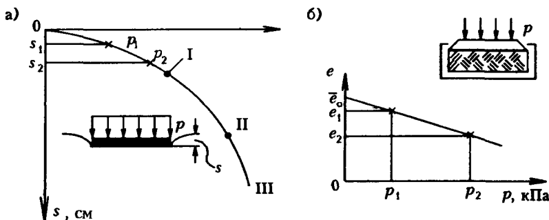
Рис.М.9.13. Определение величины модуля деформации грунта E_0 :
