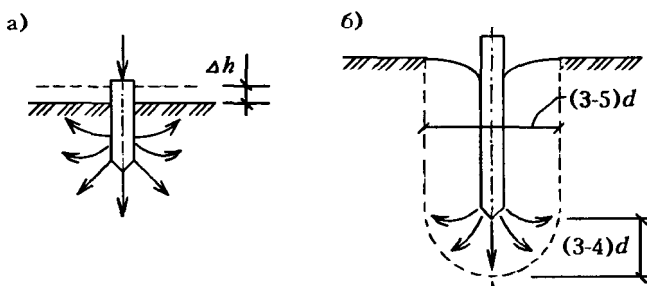
Рис.Ф.14.37. Деформация грунта вокруг свай
