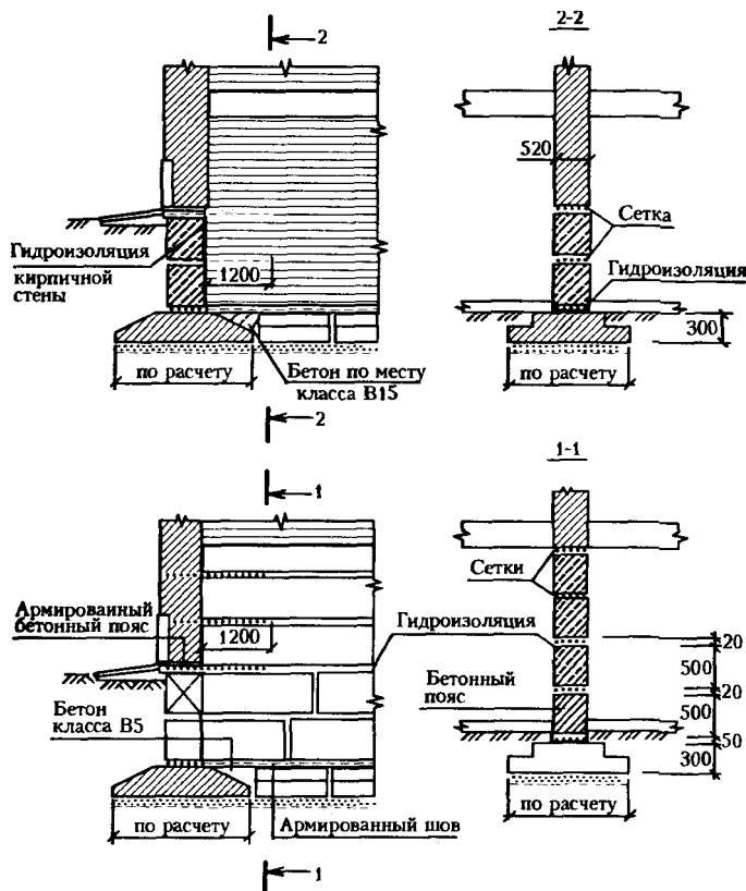
Рис.Ф.9.28 (окончание). План ленточных фундаментов и разрезы
