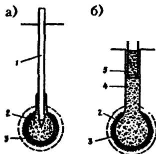
Рис.Ф.14.25. Сваи с камуфлетным уширением: а - со сборным стволом; б - с набивным стволом; 1 - забивная свая; 2 - уширенная камуфлетная пятя; 3 - уплотненная взрывом грунтовая оболочка; 4 - бе- тонный ствол; 5 - арматурный каркас
