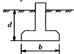
Рис.М.12.2. Фундамент мелкого заложения
