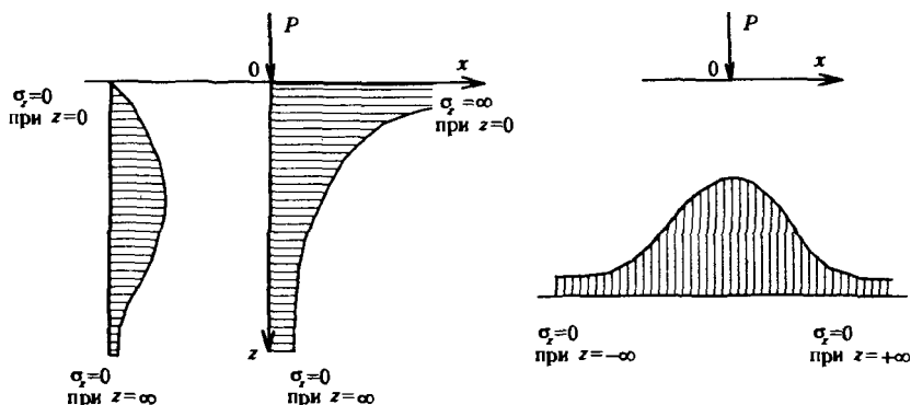
Рис.М.7.8. Эпюры напряжений \sigma_z в полупространстве по вертикальным и горизонтальным сечениям
