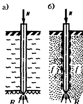
Рис.Ф.14.8. Схемы передачи нагрузки на основание
