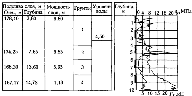
Рис.Ф.2.13. Примерный график статического зондирования:
