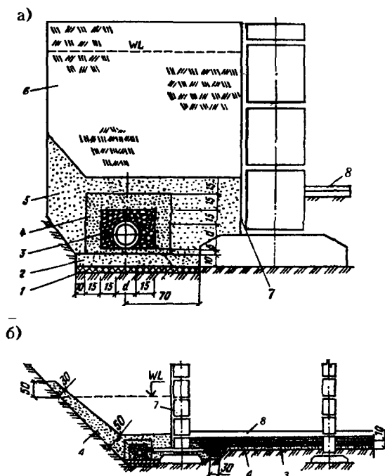
Рис.Ф.17.15. Дренаж:
