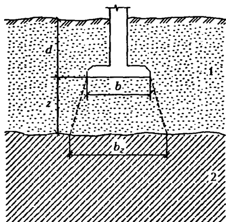
Рис.Ф.10.24. Проверка прочности слабого слоя грунта
