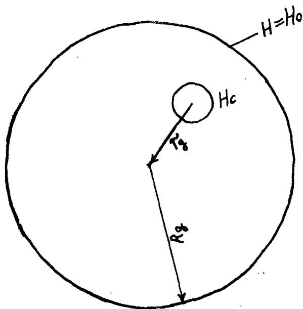
Рис. 3.11. Схема скважины, расположенной эксцентрично в круговом пласте
