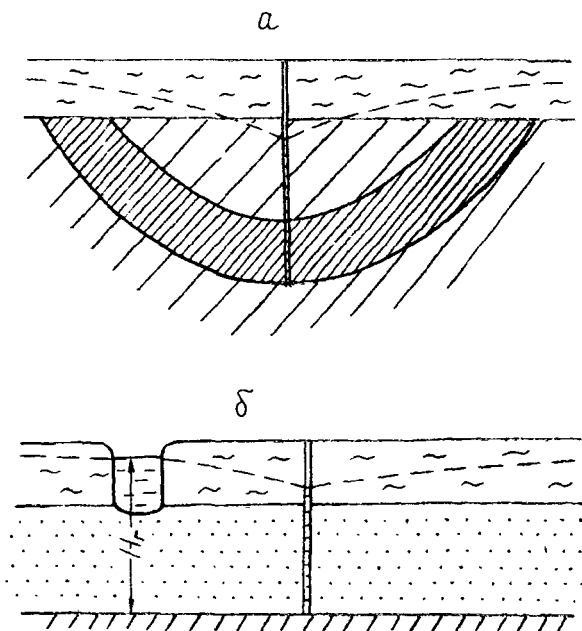
Рис. 2.9. Схемы закрытого водоносного пласта (а) и безнапорного пласта с границей обеспеченного питания (б)
