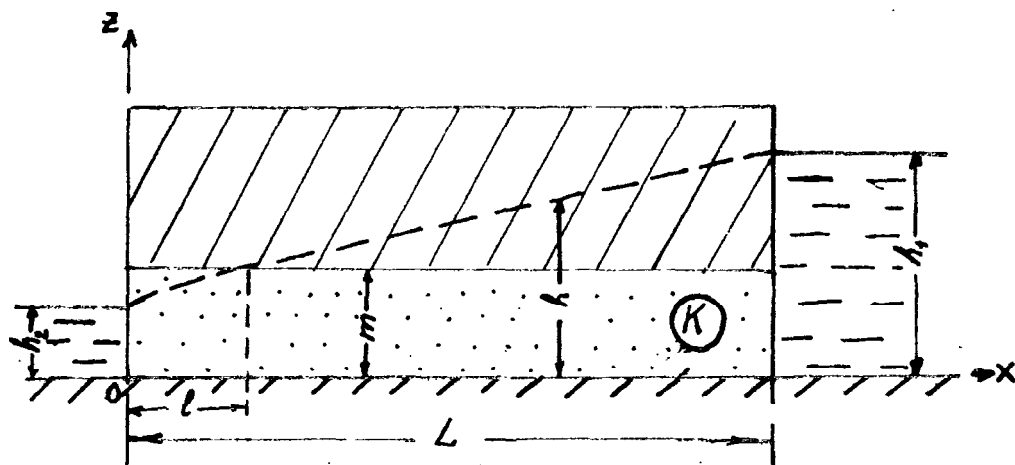
Рис. 3.4. Схема напорно-безнапорной фильтрации между двумя бассейнами
