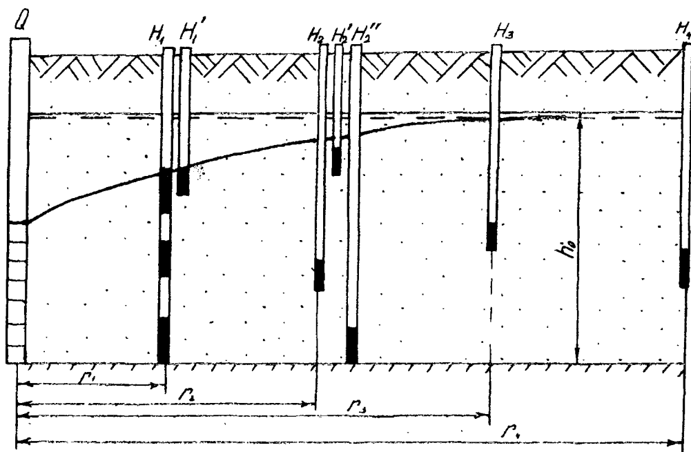
Рис. 7.3. Схема опытного куста при откачке в однородном безнапорном пласте:
