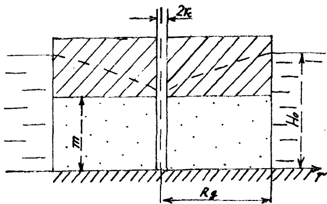
Рис. 3.8. Схема напорной фильтрации к скважине в круговом пласте
