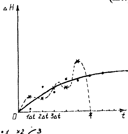
Рис. 4.9. Схематизированное представление результатов расчета фундаментальной фильтрационной задачи: 1 - данные расчета по неявной схеме; 2 - то же, по явной схеме; 3 - точное аналитическое решение
