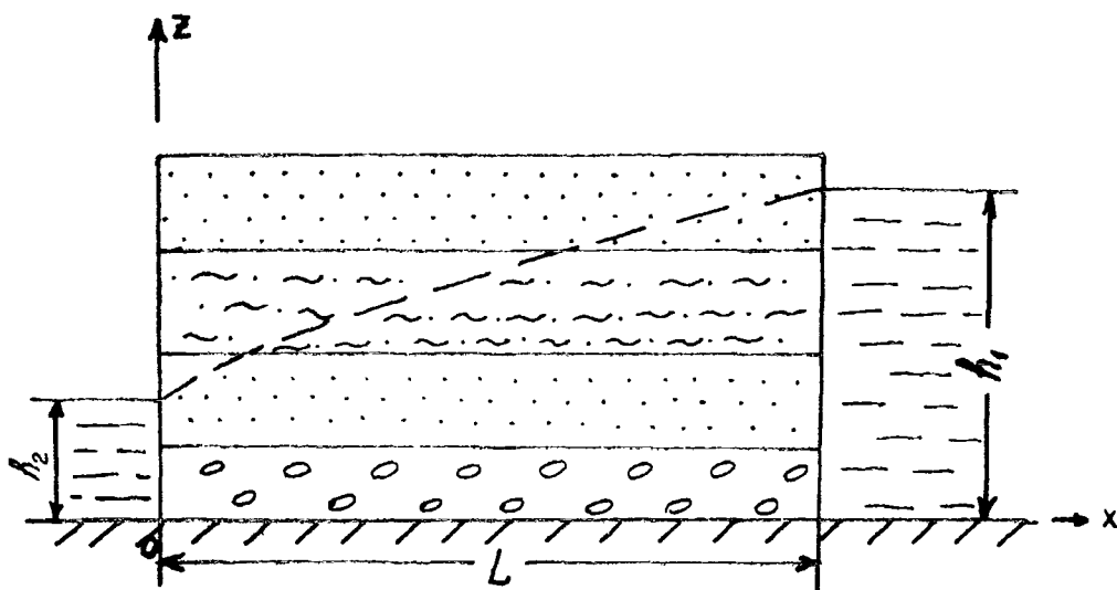
Рис. 3.3. Схема фильтрации в безнапорном слоистом пласте
