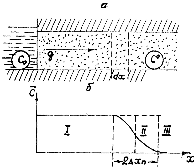
Рис. 6.10. Схема миграции в водоносном пласте (а) и характерный график пространственного изменения концентрации (б)
