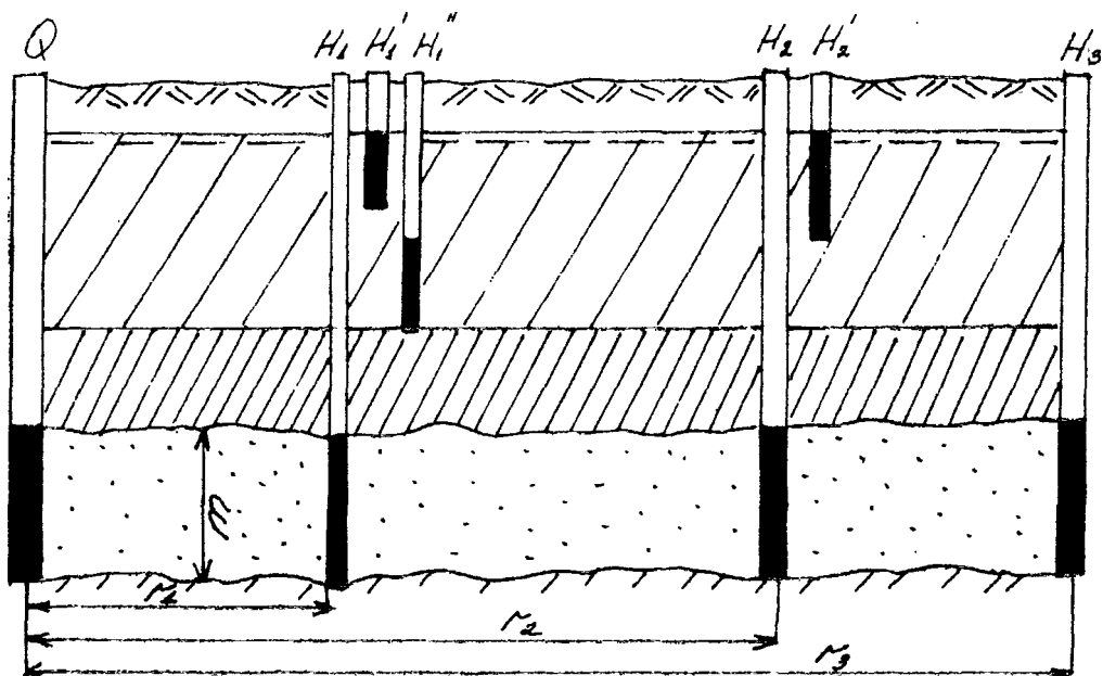
Рис. 7.2. Схема опытного куста при откачке в двухслойном пласте; Q - центральная скважина; H_1 - H_3 - пьезометры на основной слой; H_1' , H_2' , H_1'' - пьезометры-«дублиры» на слабопроницаемый слой
