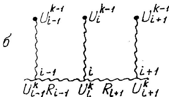
Рис. 4.7. Моделирование нестационарной фильтрации: а - исходная схема напорного пласта; б - схема резисторной сетки
