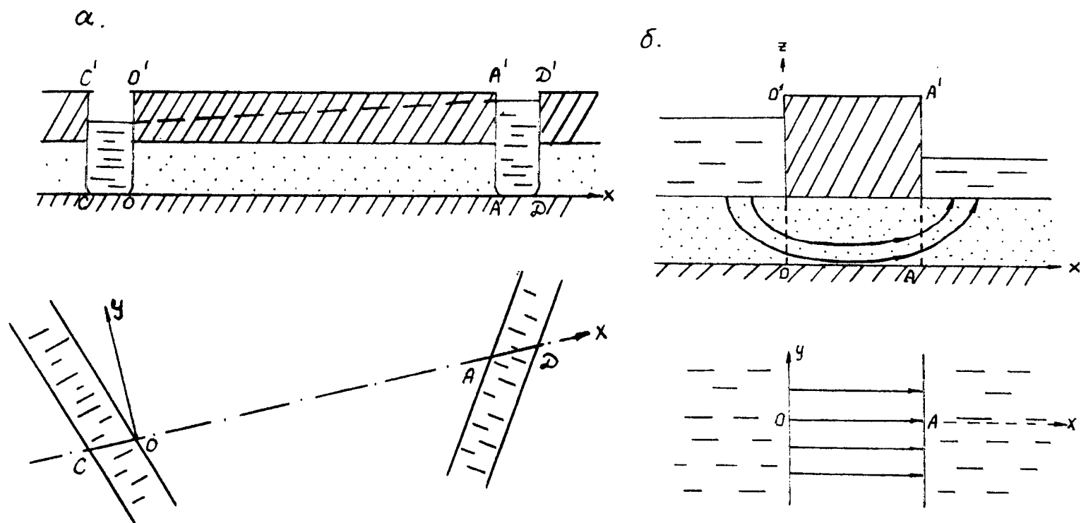
Рис. 2.4. Схемы двухмерной фильтрации: а - плановой; б - профильной
