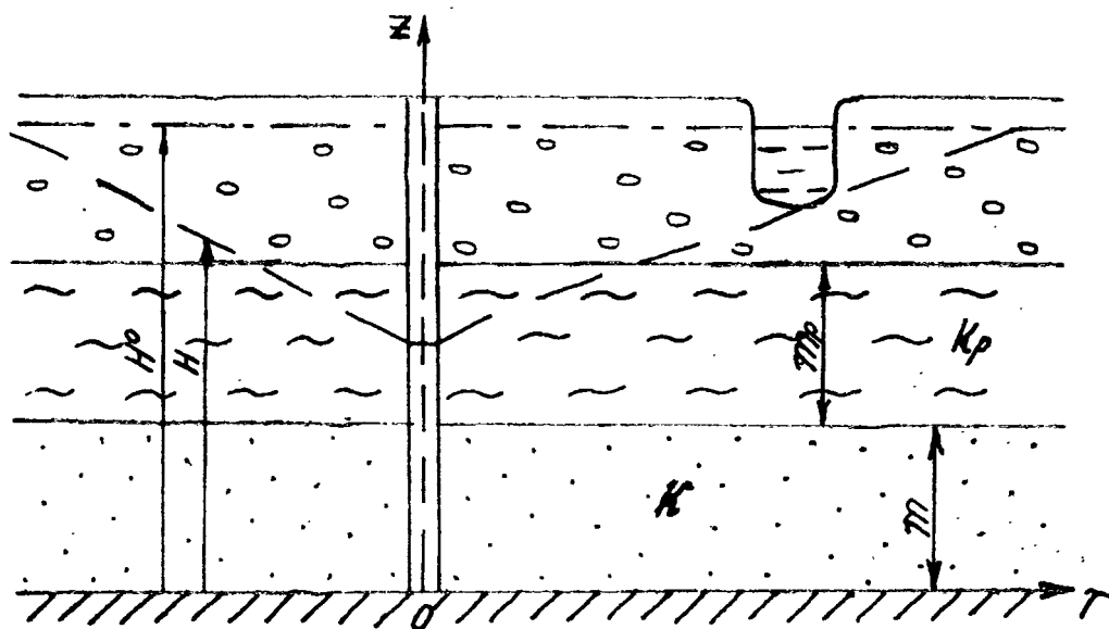
Рис. 3.9. Схема напорной фильтрации к скважине в условиях перетекания
