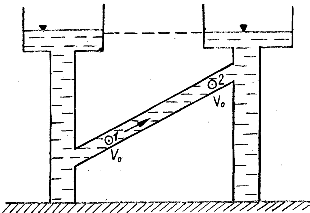
Рис. 1.5. Схема к оценке изменения энергии фиксированного объема в движущейся жидкости
