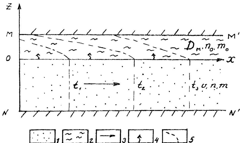
Рис. 6.12. Схема миграции подземных вод в двухслойном пласте: 1 - хорошопроницаемый слой; 2 - слабопроницаемый слой; направления потоков: 3 - конвективного; 4 - диффузионного; MM' и NN' - границы расчетного элемента, непроницаемые для воды и вещества; 5 - положение концентрационного фронта на различные моменты времени t
