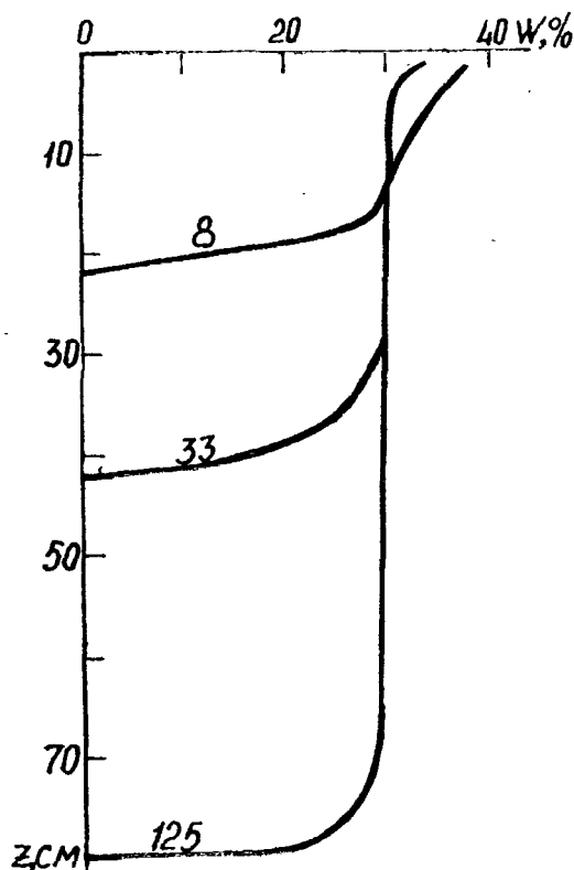
Рис. 6.25. Характерные опытные графики зависимости влажности от глубины просачивания (цифры на кривых - время от начала опыта, мин.)
