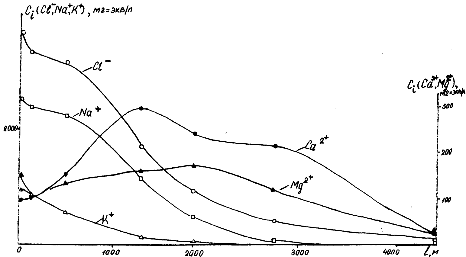
Рис. 6.4. Закономерности изменения содержания ионов при миграции хлоридно-натриевых рассолов в комплексе карбонатно-глинистых пород ( l - расстояние от рассолонакопителя)
