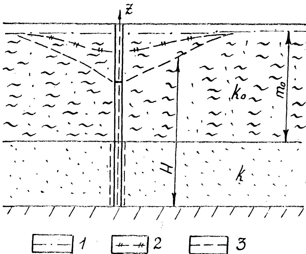
Рис. 5.5. Схема безнапорного двухслойного пласта:
