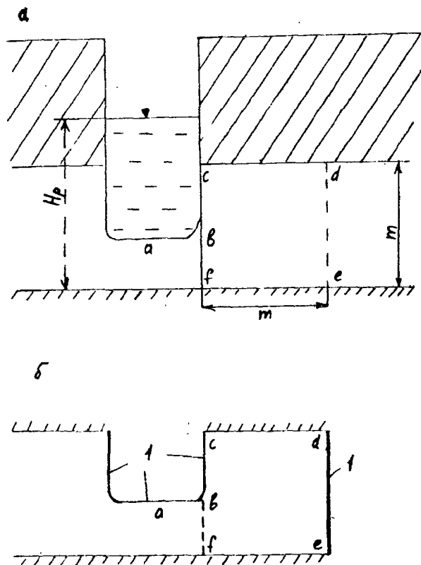
Рис. 3.18. Схемы к моделированию фильтрации (а) и элемент сетки сопротивлений (б);
