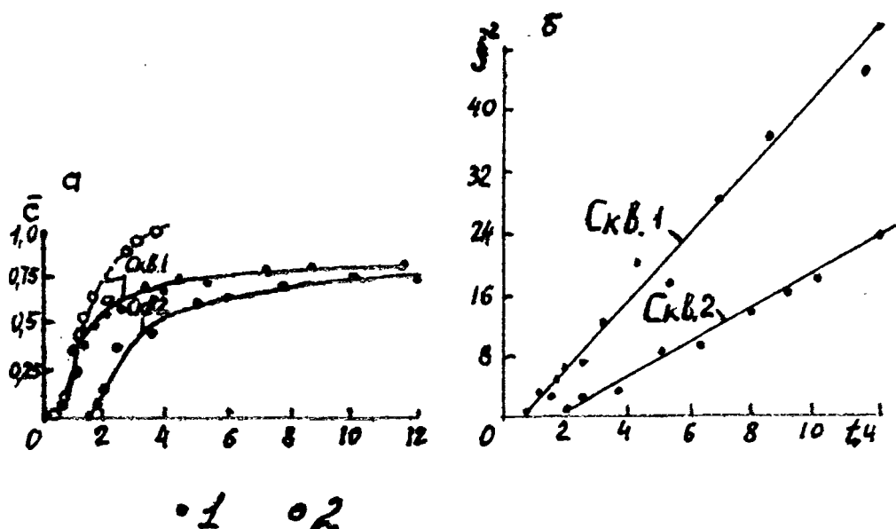
Рис. 7.4. Графики изменения относительных концентраций индикаторов в наблюдательных скважинах (а) и представление опытных данных при графоаналитическом способе их интерпретации (б):
