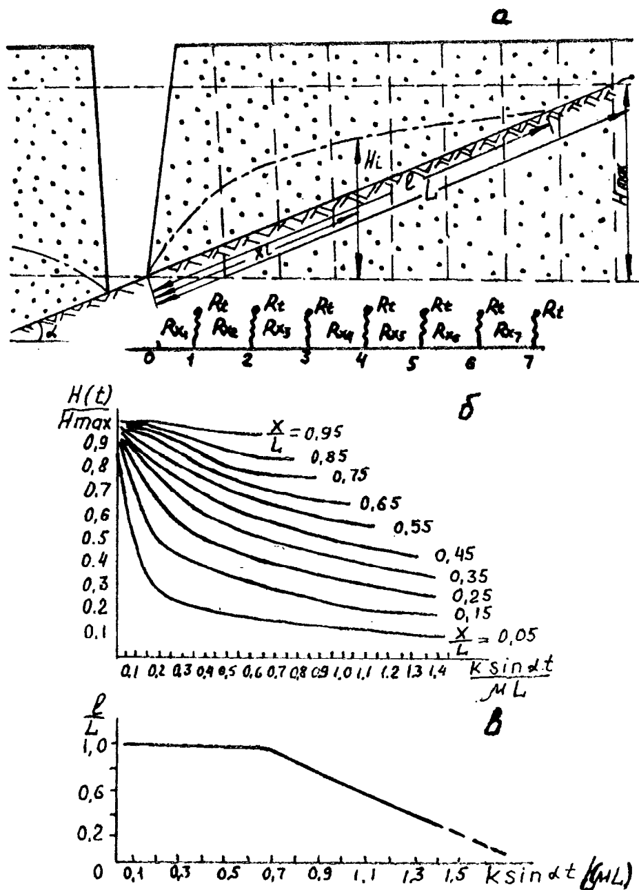
Рис. 8.10. Схема и результаты моделирования фильтрации в безнапорном пласте на наклонном водоупоре, вскрываемом горной выработкой:
