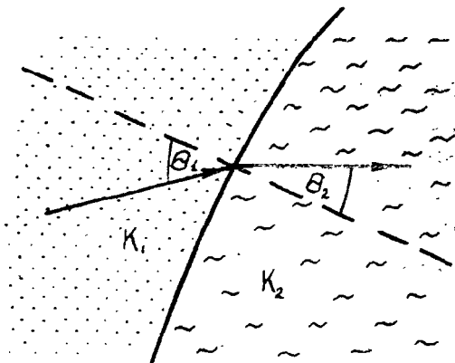
Рис. 2.11. Преломление линий тока на границе двух зон с различной проницаемостью
