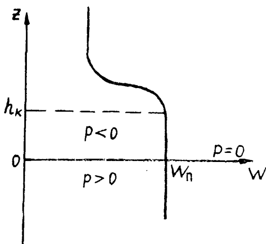
Рис. 1.10. Характерная кривая изменения влажности вблизи капиллярной каймы
