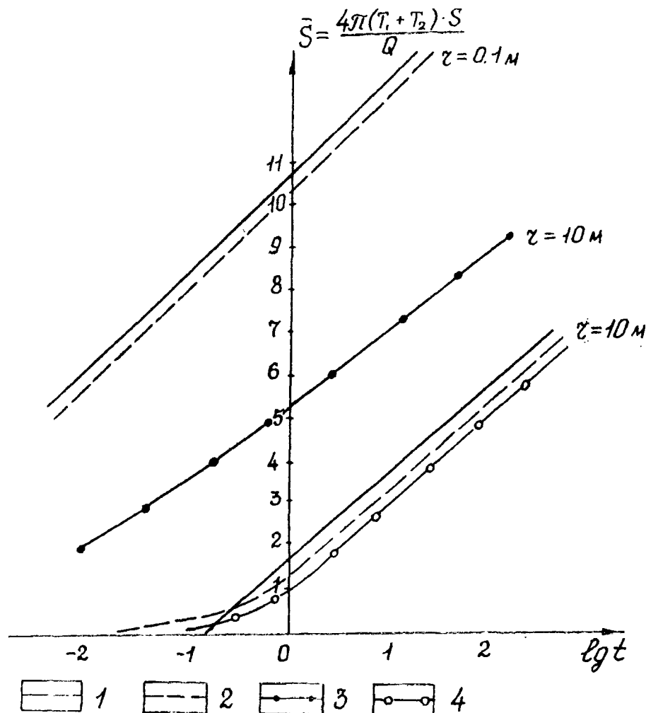
Рис. 5.8. Расчетные графики приведенных понижений для двухслойной системы:
