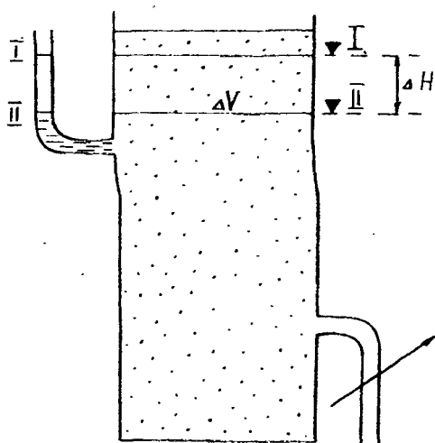
Рис. 1.17. Схема опыта по определению гравитационной водоотдачи
