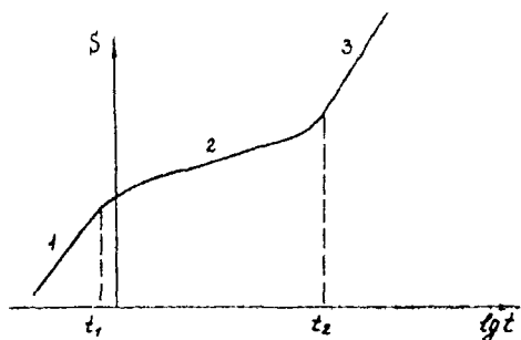
Рис. 5.9. Типовой индикаторный график откачки из пласта пород с двойной емкостью
