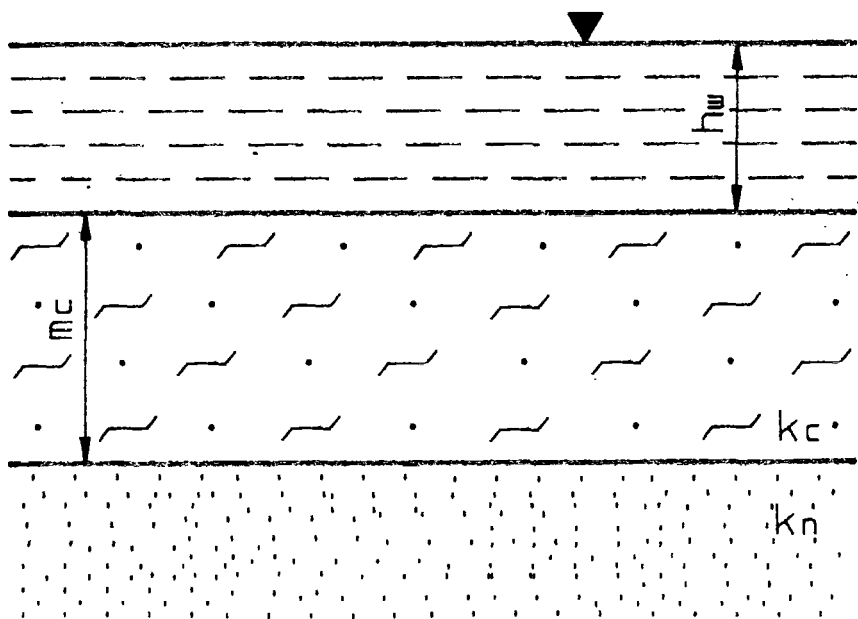
Рис. 6.27. Схема оценки условий образования насыщенного потока при наливе в двухслойную толщу
