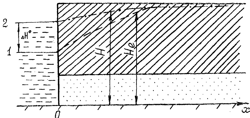
Рис. 4.2. Развитие подпора вблизи водохранилища:
