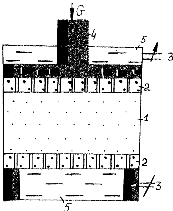
Рис. 1.24. Схема опыта с образцами песка в компрессионном приборе: 1 - образец; 2 - пористые прокладки; 3 - краны; 4 - дырчатый поршень, передающий внешнюю нагрузку на образец; 5 - камеры с водой под напором
