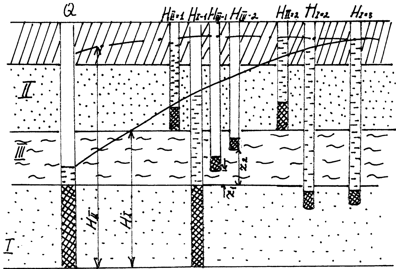
Рис. 7.1. Схема опытного куста при опробовании взаимодействующих пластов: I - основного; II - взаимодействующего; III - разделяющего; Q - центральная скважина; H_{I-1} - H_{I-3} - наблюдательные скважины на основной пласт; H_{II-1} - H_{II-2} - пьезометры на взаимодействующий пласт; H_{III-1} - H_{III-2} - пьезометры на разделяющий пласт
