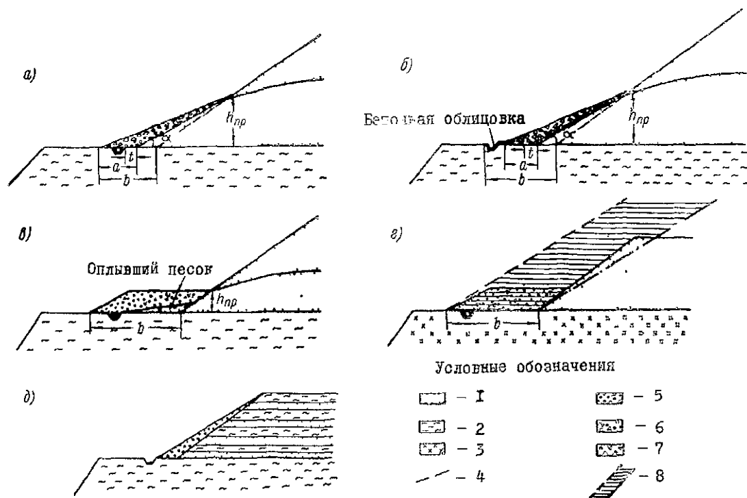
Рис.8. Схемы дренажных пригрузок
