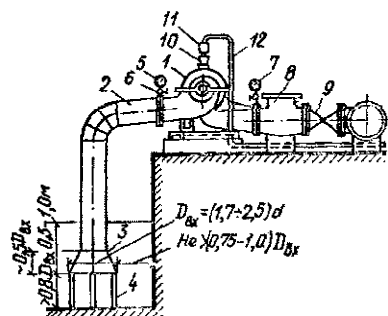
Рис. 5.4. Схема оборудования арматурой горизонтального центробежного насоса
