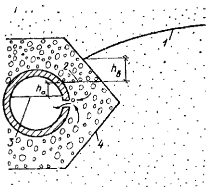
Рис. 9.9. Схема к гидравлическому расчету водоприемного отверстия трубы
