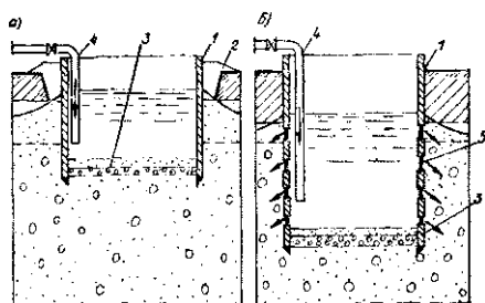
Рис. 13.7. Схемы шурфов
