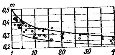
Рис. 4.5. Зависимость пористости породы от \eta
