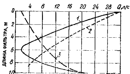
Рис. 14.9. Графики расходомертин двухколонной конструкции скважин при различном положении вала насоса
