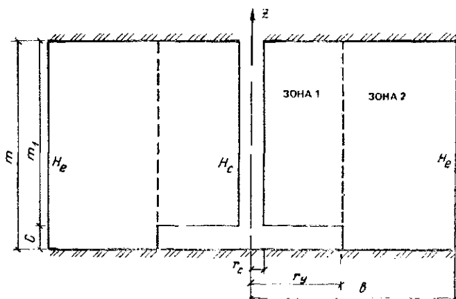
Рис. 14.5. Схема к расчету скважины с уширенным основанием
