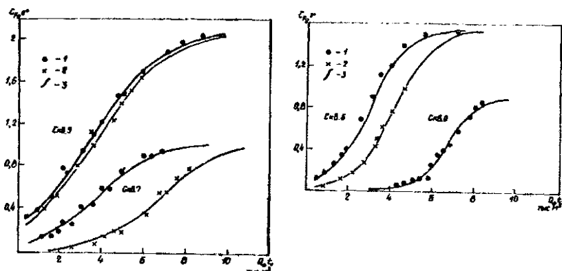
Рис. 21.9. Выходные кривые
