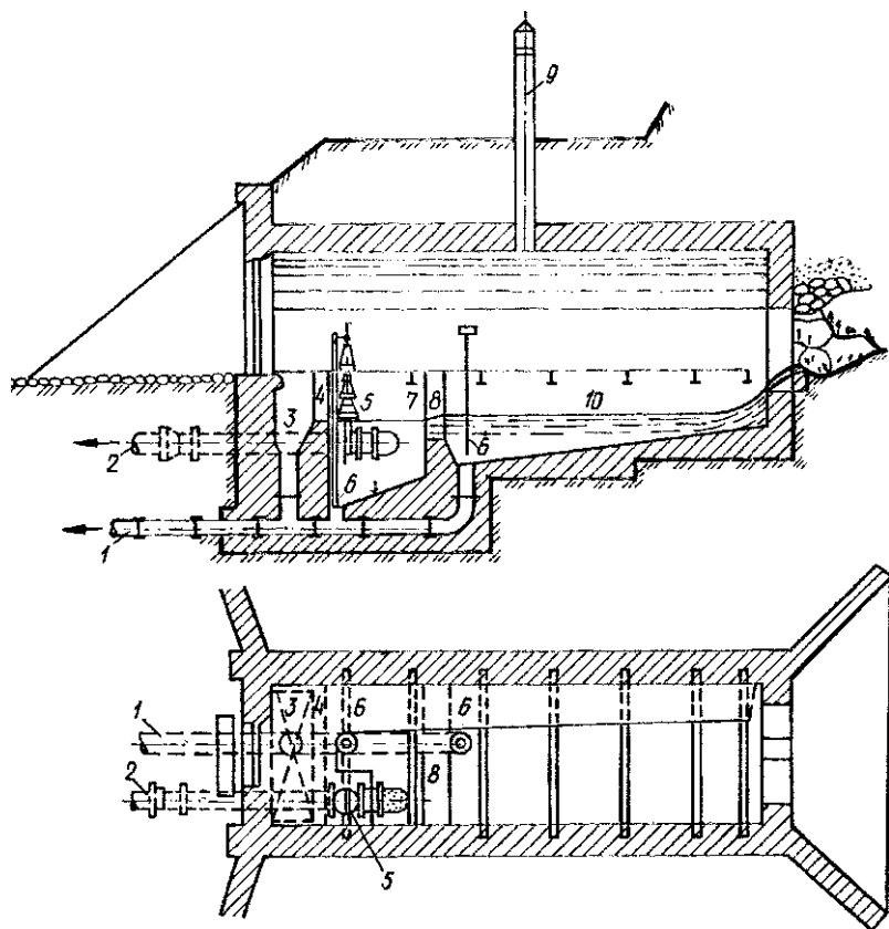
Рис. 11.8. Каптаж нисходящего сосредоточенного выхода источника в виде каптажной камеры
