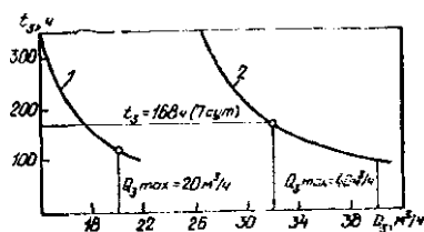
Рис. 21.24. Зависимости t_3 = f(Q_3)
