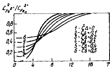
Рис. 21.16. Расчетные выходные кривые
