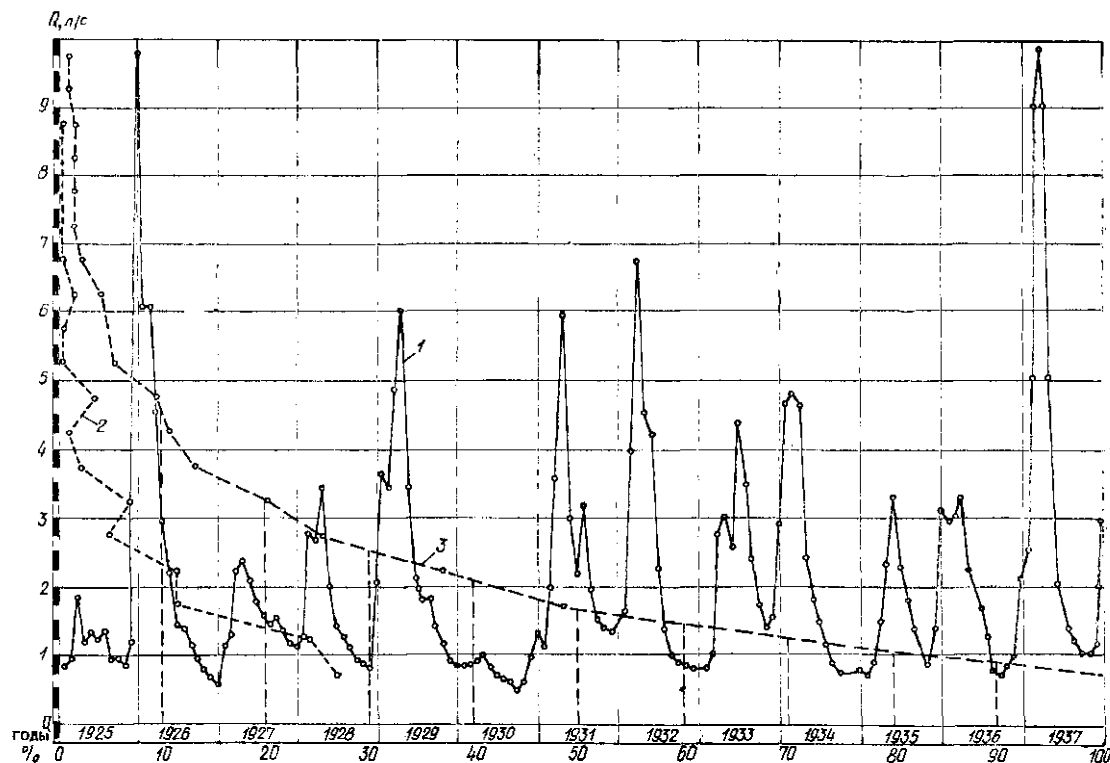
Рис. 11.4. График расхода одного из источников в Крыму (срок наблюдения — 13 лет) 1 — хронологический график расхода; 2 — кривая частоты; 3 — кривая обеспеченности
