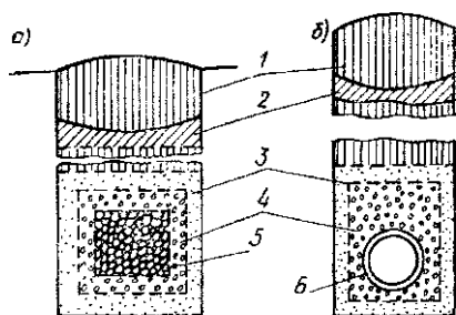
Рис. 9.1. Траншейные водозаборы а — каменно-щебенчатого типа; б — трубчатого типа: 1 — обратная засыпка траншей местным грунтом; 2 — глина; 3 — крупно-зернистые пески; 4 — гравий; 5 — рваный камень; 6 — дренажная труба
