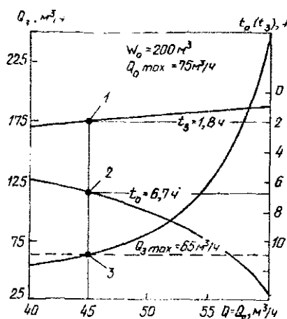
Рис. 21.21. Графоаналитический метод расчета установки на максимальную производительность
