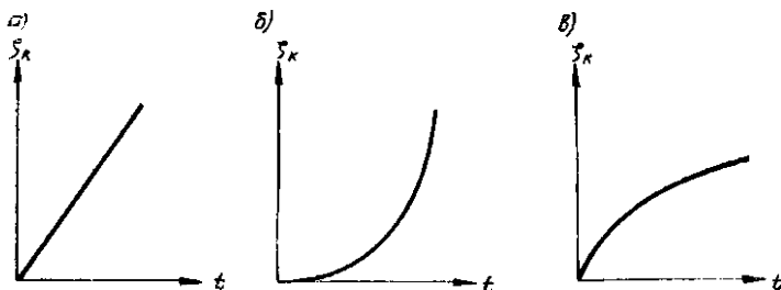
Рис. 13.15. Возрастание сопротивления \xi_k , обусловленного проявлением различного вида кольматации
