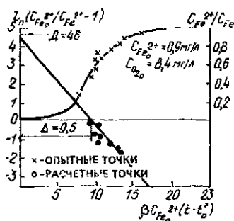
Рис. 21.12. Выходная кривая C_{Fe^{2+}}/C_{Fe^{2+}} по скважине № 3 и вспомогательный график для расчета параметров процесса
