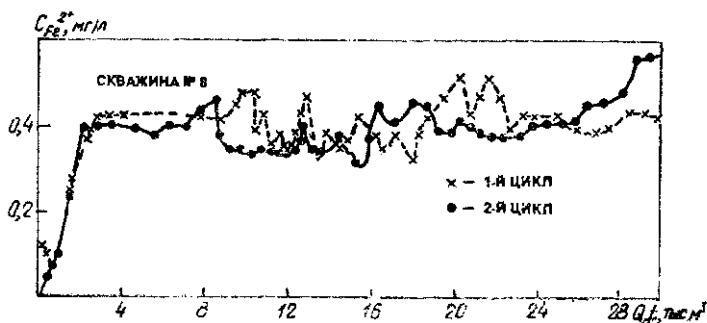
Рис. 21.15. Выходные кривые
