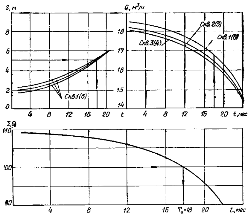
Рис. 7.9. Расчетные значения изменения S_j(t) , Q_j(t) и \Sigma Q_j(t) при насосной эксплуатации скважин
