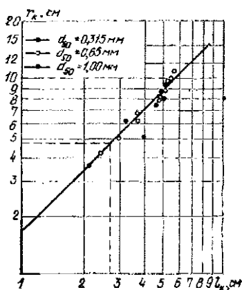
Рис. 14.3. Зависимость глубины каверны от ее радиуса
