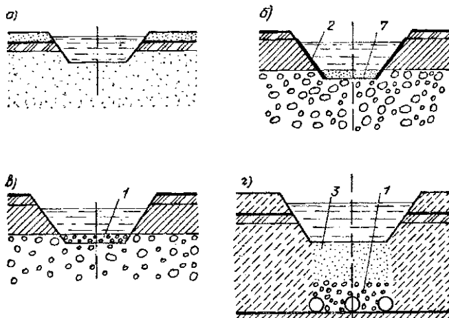
Рис. 13.5. Схемы инфильтрационных бассейнов
