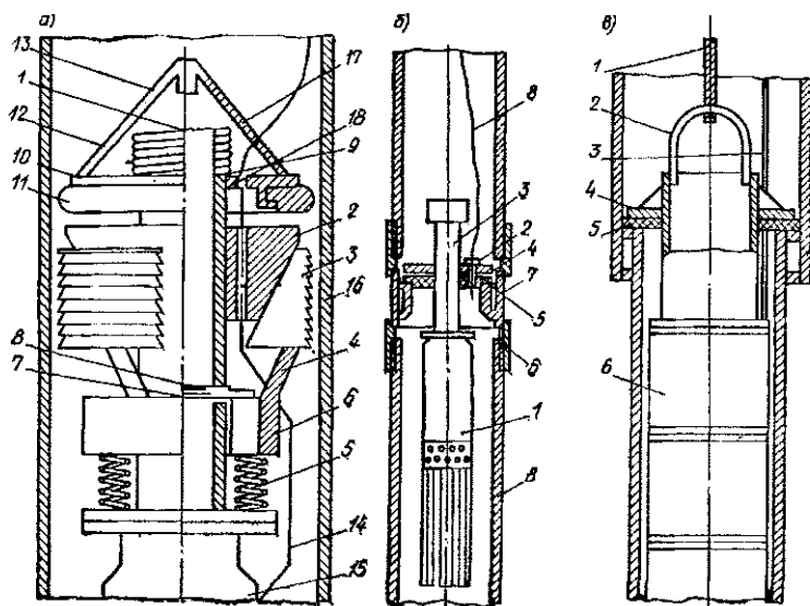
Рис. 5.7. Беструбная подвеска с герметизацией и опорой в месте их установки а — с подпружиненным кольцом; б — с посадочным гнездом треста Курсксельхозводстрой; в — с опорным фланцем ЦНИИКИВР
