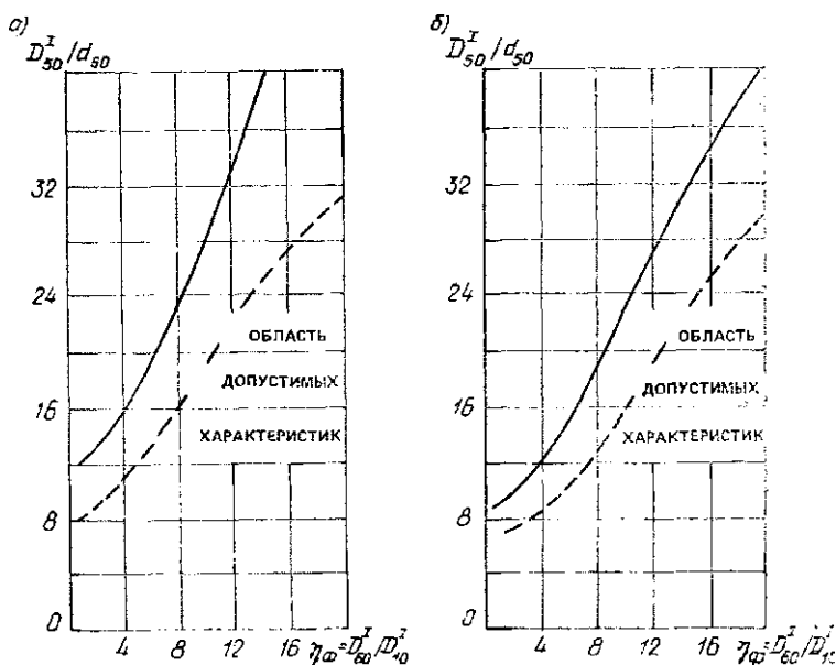
Рис. 9.6. Кривые для подбора состава первого слоя фильтра (схема движения воды сверху вниз)
