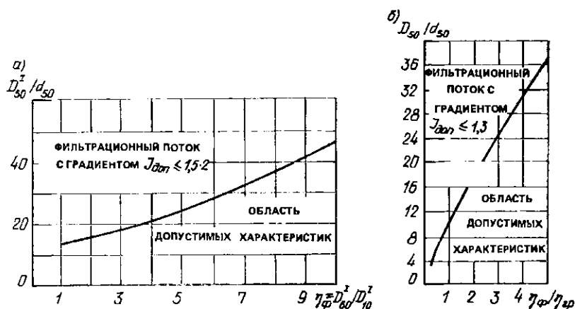
Рис. 9.7. Кривые для подбора состава первого слоя фильтра D_{60}/D'_{10} \leq 10 а — при движении воды снизу вверх на песчаном основании; б — при боковом движении воды при I \leq 1,3d_{60}/d'_{10} \leq 10
