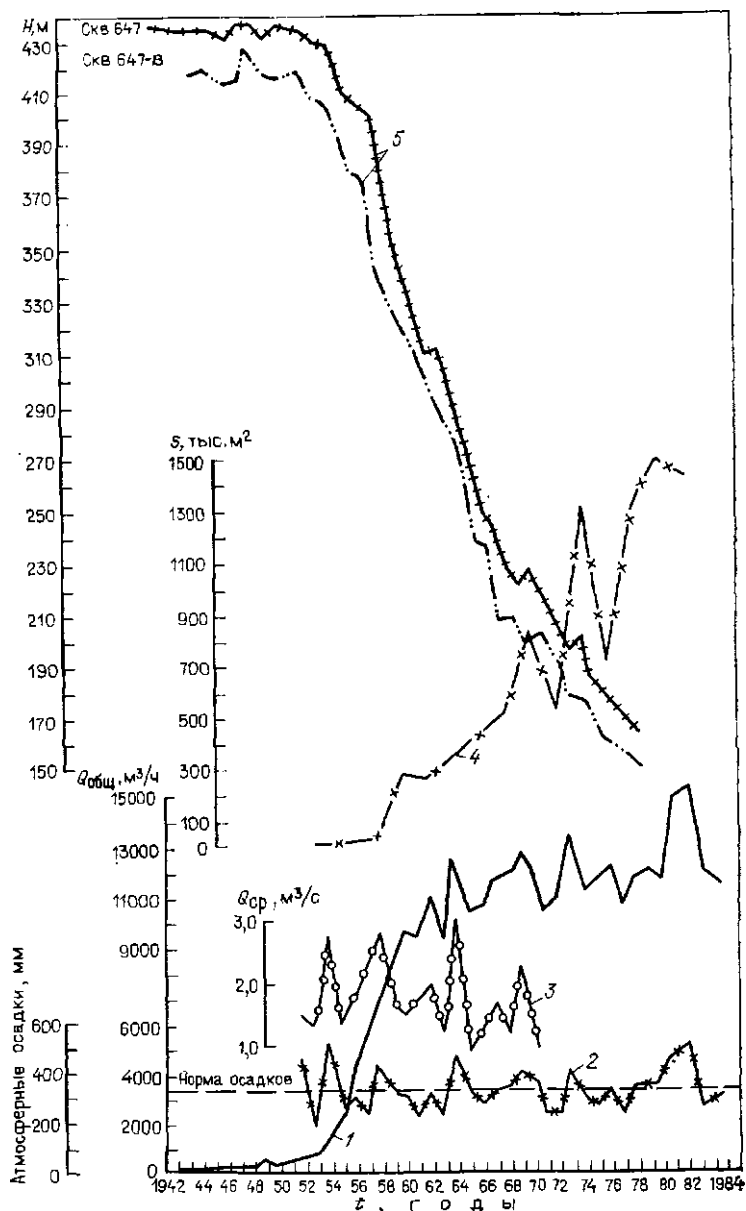
Рис. 68. Комплексный график:
