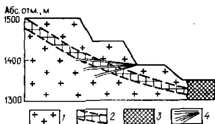
Рис. 16. Схема осушения Западного борта рудного месторождения.
