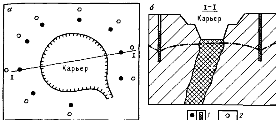
Рис. 11. Схема осушения карьера с помощью водопонижительных скважин.
