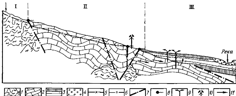
Рис. 67. Геолого-гидрогеологический профиль:
