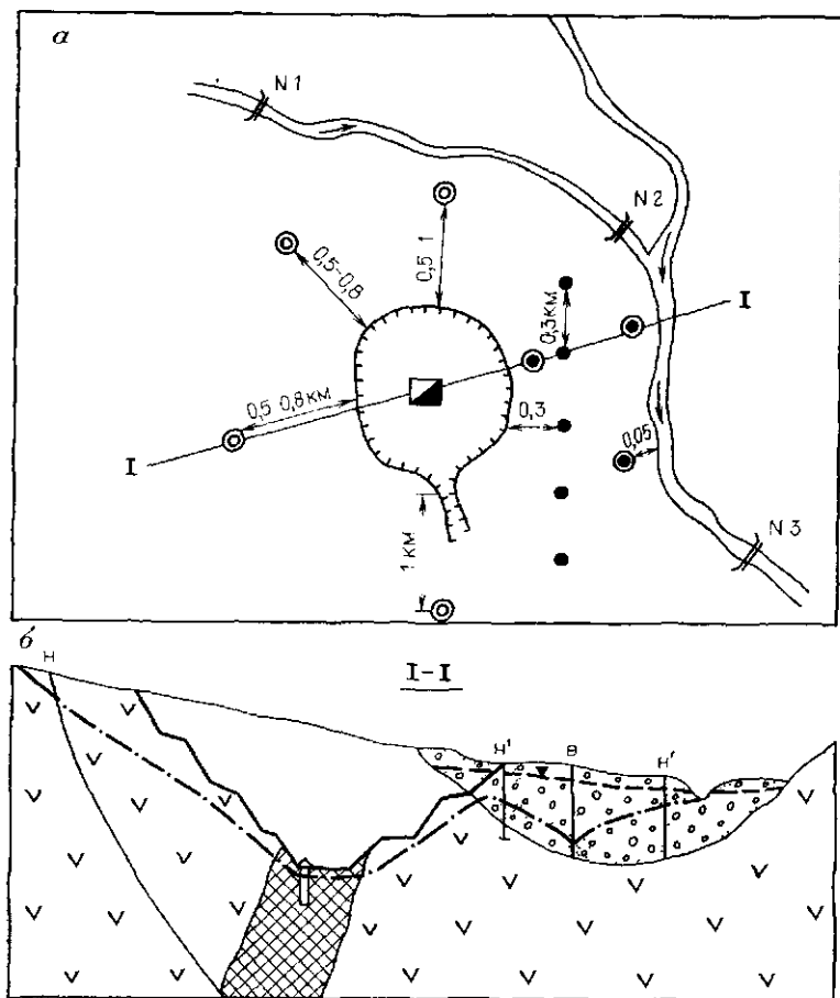
Рис. 29. Схема расположения опорных наблюдательных постов при карьерной отработке месторождения.
