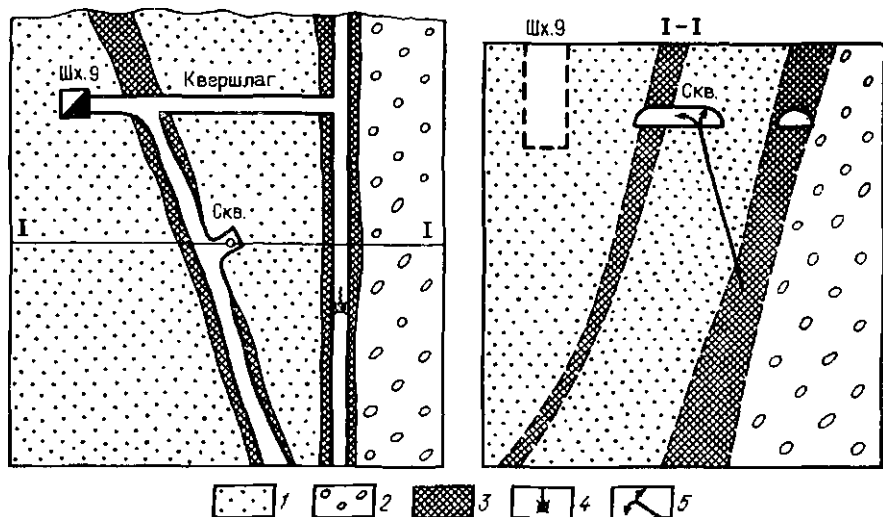
Рис. 5. Схематический план и разрез по линии I—I горизонта месторождения.
