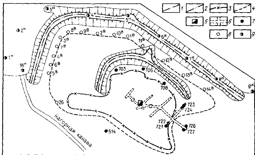
Рис. 75. Схема защиты карьеров опытно-промышленного участка (ОПУ) и опытно-промышленного производства (ОПП) от поверхностных и подземных вод:
