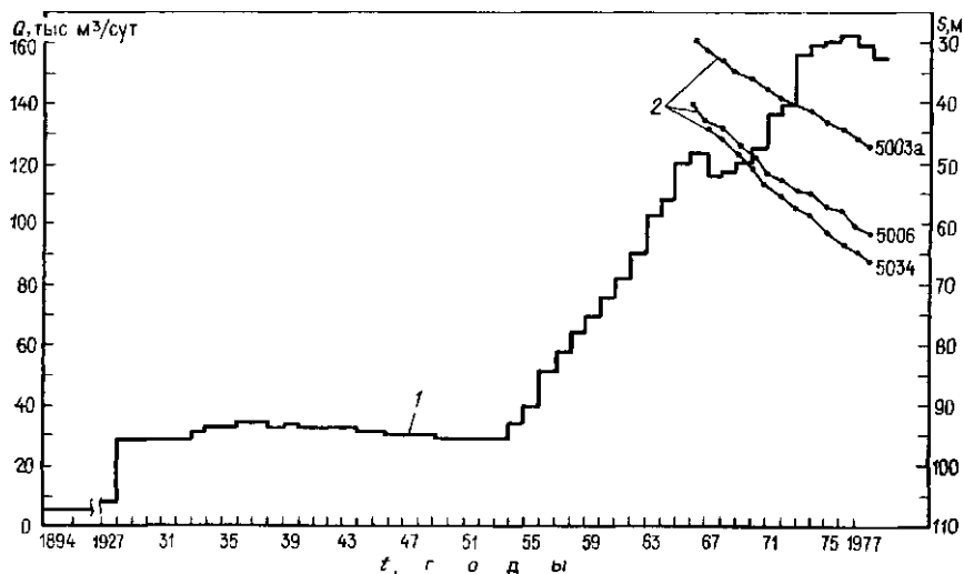
Рис. 59. Графики изменения водоотбора (1) и уровней подземных вод (2) на водозаборе.
