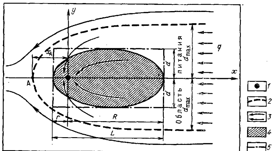
Рис. 38. Принципиальная схема движения подземных вод к водозабору при наличии естественного потока.
