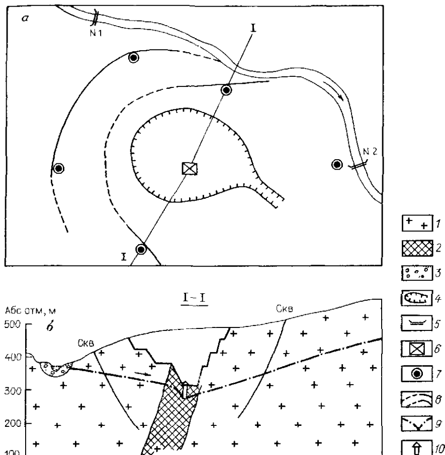
Рис. 28. Размещение опорной наблюдательной сети при карьерной отработке рудного месторождения.
