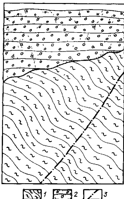
Рис 19 Литологический разрез второй модели геологической среды
