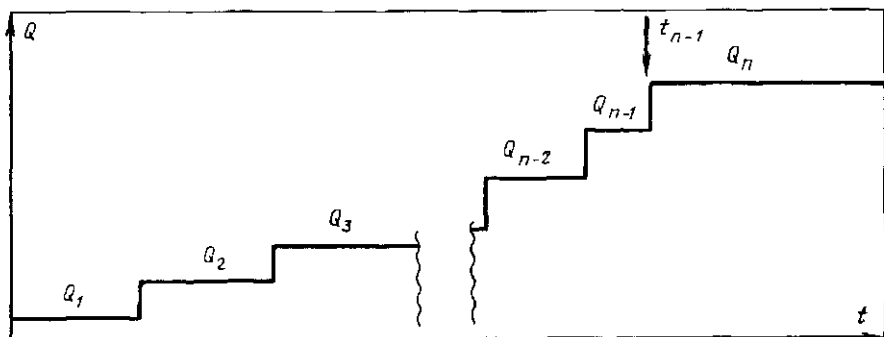
Рис 56. Ступенчатый график водоотбора
