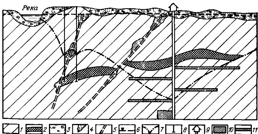
Рис 13 Схематический геологический гидрогеологический разрез рудного месторождения
