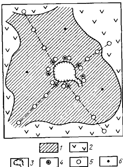
Рис. 30. Схема расположения наблюдательной сети на месторождениях третьей группы.
