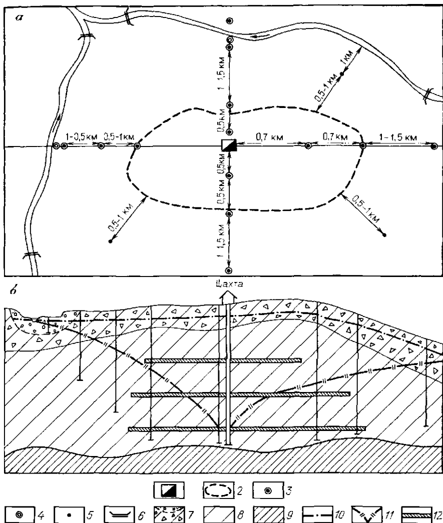
Рис. 27. Схема размещения наблюдательных постов (а) и гидрогеологический разрез (б) по линии I—I.
