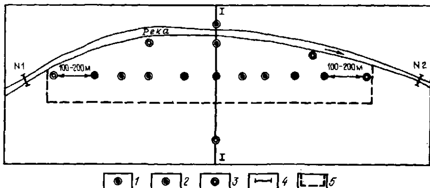
Рис. 32. Схема расположения опорной наблюдательной сети на инфильтрационном водозаборе.
