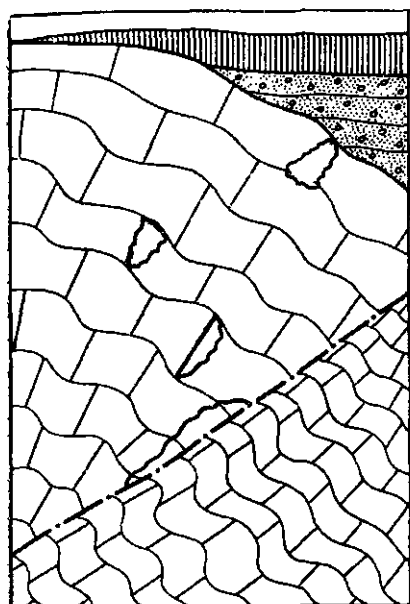
Рис. 20. Литологический разрез третьей модели геологической среды.
