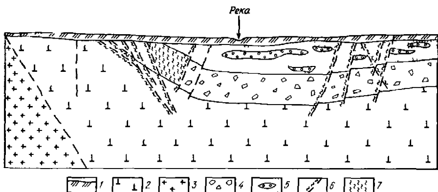
Рис. 4. Схематический геологический разрез месторождения
