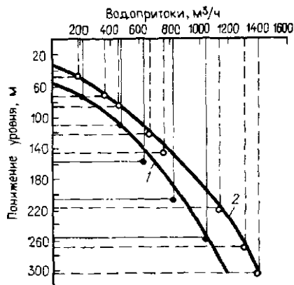
Рис. 25. Графики изменения водопритоков от понижения уровня при карьерной отработке Западного (1) и Дальнезападного (2) месторождений
