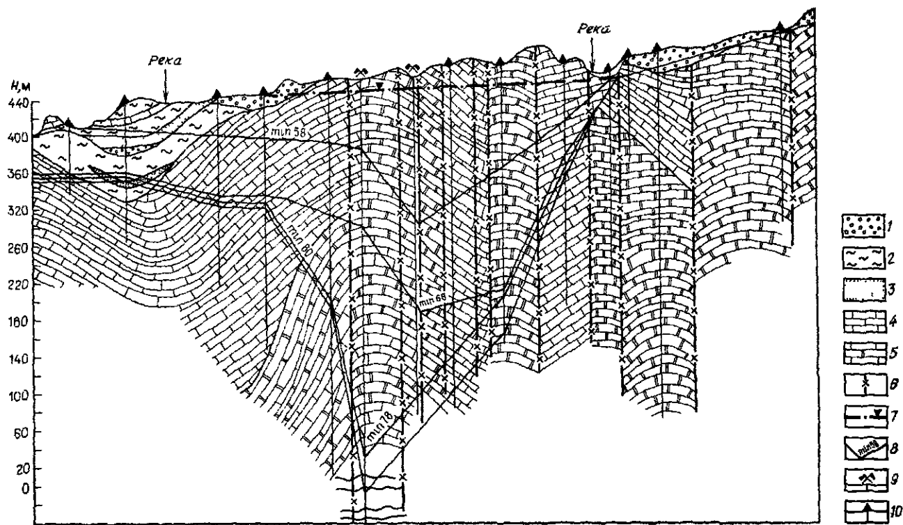
Рис 70 Геолого-гидрогеологический профиль
