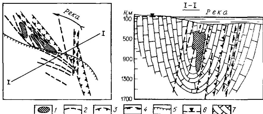
Рис. 73. Тектоническая схема (а) и схематический гидрогеологический разрез по линии I—I (б) месторождения:
