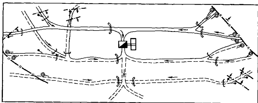
Рис. 24. Совмещенный план горных разработок и схема расположения опорной наблюдательной сети за режимом рудничных вод.
