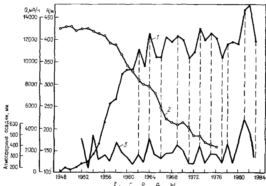
Рис. 53. Комплексный график:
