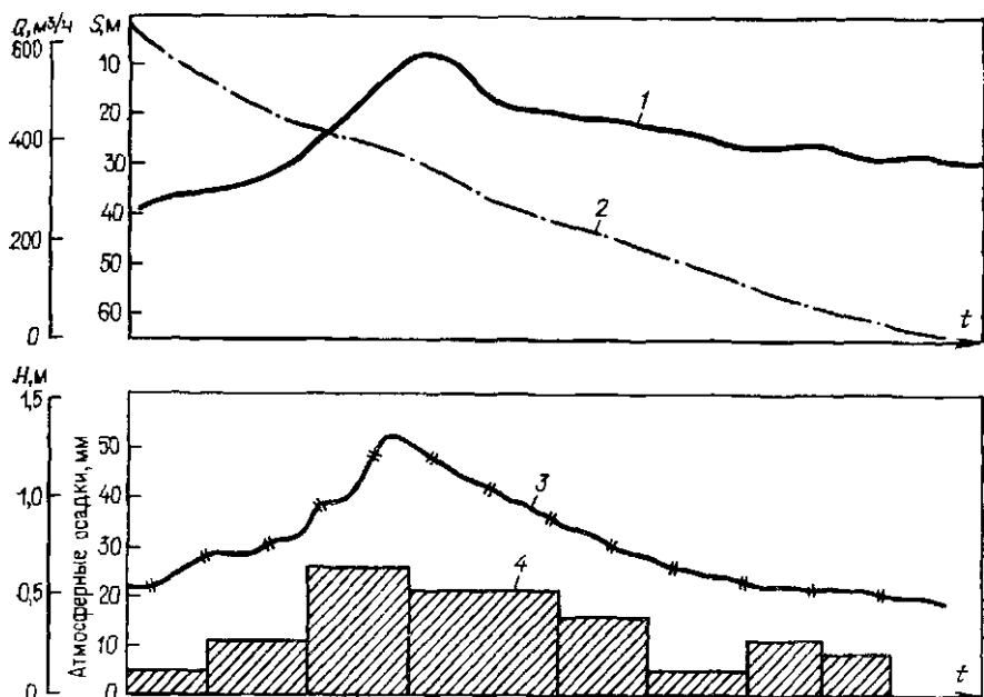
Рис. 46. Комплексные графики:
