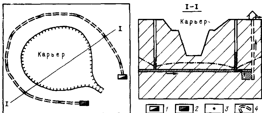
Рис. 12. Комбинированная схема осушения карьера:
