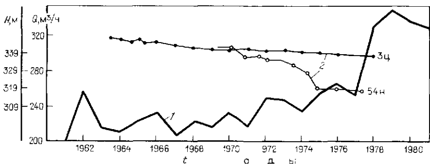
Рис. 47. Графики режима водопритоков (1) и уровней в наблюдательных скважинах (2) Сибайского карьера
