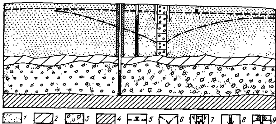
Рис 35 Схема ярусного размещения наблюдательных скважин
