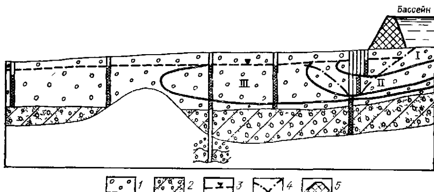
Рис 44 Геолого химический профиль по линии I—I (см рис 47)
