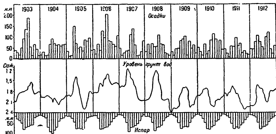
Рис. 143. График колебаний уровня грунтовых вод (средний) в связи с атмосферными осадками (вверху) и испаряемостью (внизу) для с. Василевичи за 10 лет (по Е. В. Оппокову).
