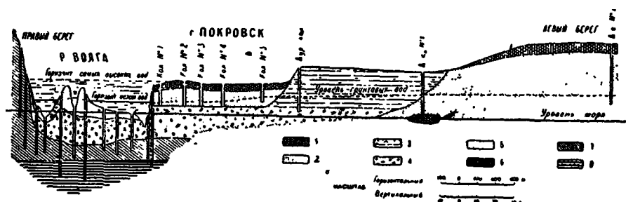
Рис. 66. Разрез левого берега Волги против Саратова, составленный по материалам Фаас и Эрасси (разрез Волги), по колодцам г. Покровска и буровым скважинам 1919 г.
