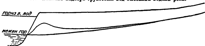
Рис. 70. Поверхность грунтовых вод при быстром спаде весенних вод.
