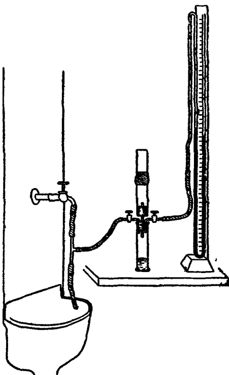
Рис. 29. Капиллярметр Энгельгардта.
