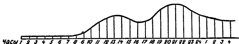
Рис. 51. Кривая концентрации раствора индикатора в наблюдательной скважине.
