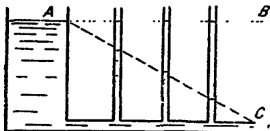
Рис. 107 Модель, показывающая положение пьезостатического уровня AB и гидродинамического AC .
