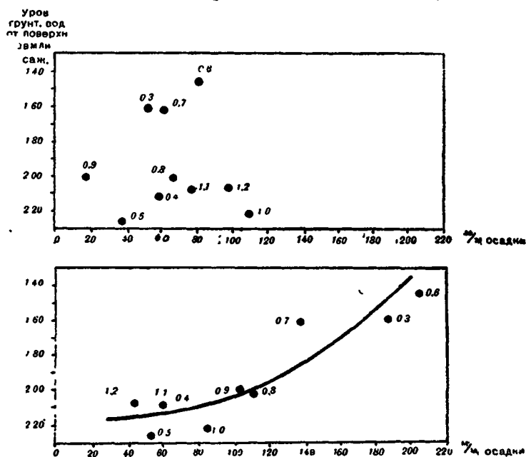
Рис. 144. Сопоставление уровня грунтовых вод за август с количеством атмосферных осадков за тот же месяц (верхний чертеж) и за предшествующий (нижний чертеж) по годам с 1903 г. по 1912 г. в с. Василевичи (составлено по данным Е. В. Оппокова).
