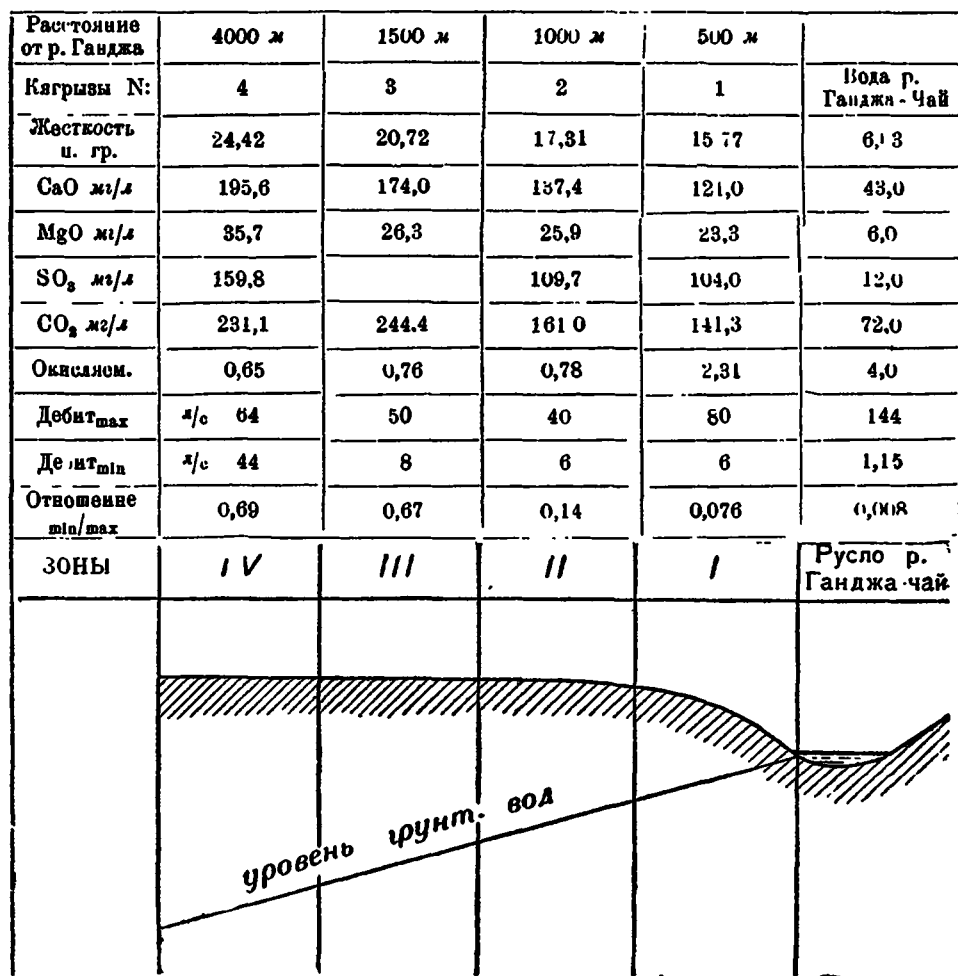
Рис. 91. Колебания дебита и химического состава грунтовых вод в зависимости от удаленности от р. Ганджа-Чай, по данным Д. В. Сухина (из книги К. Н. Паффенюльда „Озеро Гей-Гель и р. Ганджа-Чай как возможные источники водоснабжения г. Гандже“. 1933).
