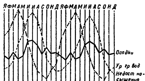
Рис. 146. Двухгодичный период колебания уровня грунтовых вод, осадков и недостатка насыщения для Берлина (из Кейльгака).
