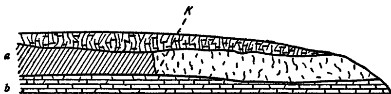
Рис. 60. Продольный разрез оврага (по А. П. Павлову).
