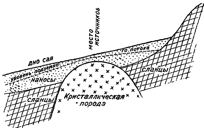
Рис. 35. Схематический чертеж Сасык-Булак-Сая, показывающий условия образования плотинных источников. (По Ф. Ф. Мужикину — Плотинные источники Сасык-Булак-Сая Зирабулакского района Бухарской республики).
