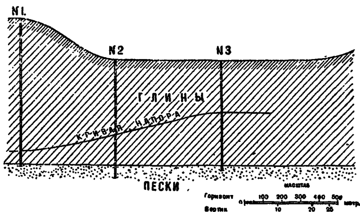
Рис. 112. Полунапорные воды в области сыртовых глин Заволжья.
