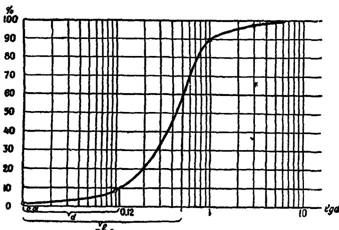
Рис. 21. Кривая механического состава песка (логарифмическая).
