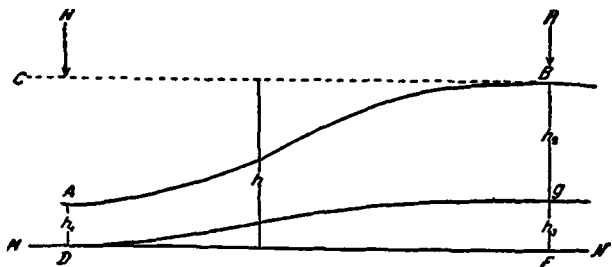
Рис. 57. Зависимость формы поверхности грунтовых вод от рельефа в связи с потерей барометрического давления.
