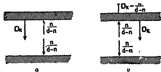
Рис. 148, а и 148, б. Влияние сжатия воздуха на просачивание воды в почву (по Энгельгарду).
