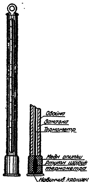
Рис. 138. Ленивый термометр.
