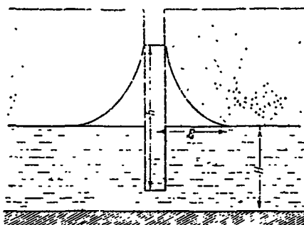
Рис. 131. Разрез поглощающего колодца.
