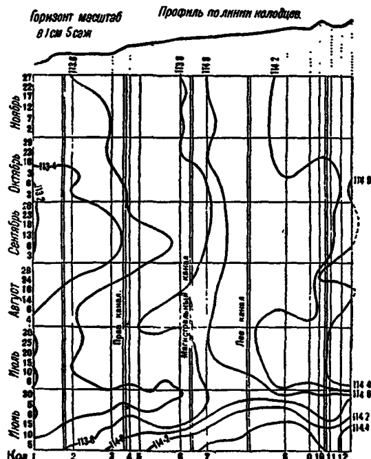
Рис. 53. Гидроизоплесты по линии колодцев № 1—12 на „Сукином бодоте“ за июнь—ноябрь (из работы А. Д. Брудастова).
