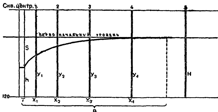
Рис. 128. Разрез депрессионной кривой при откачке.
