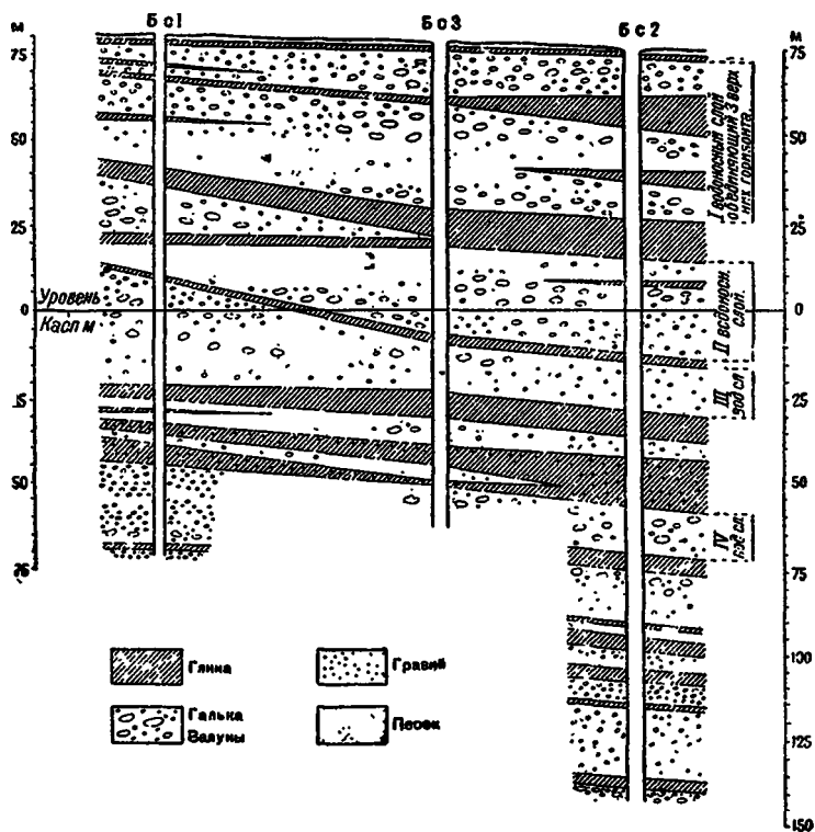
Рис. 94. Разрез по трем скважинам Шохтарского района с указанием главных водоносных горизонтов.
