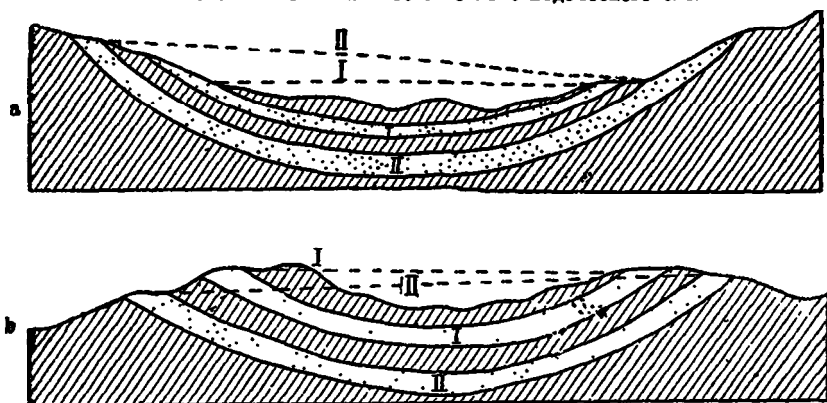
Рис. 106а и 106б. Этажное расположение артезианских водоносных горизонтов.
