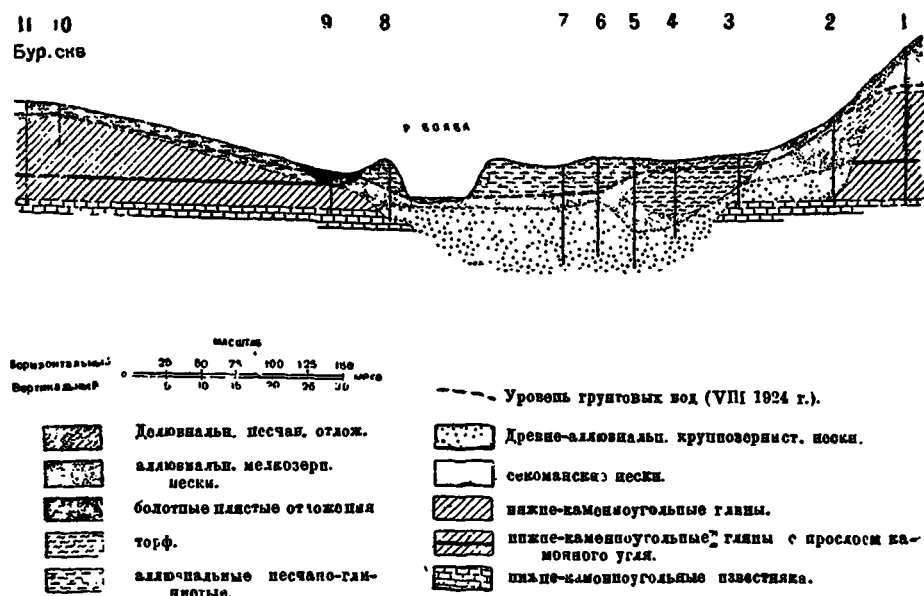
Рис. 75. Разрез через долину р. Болвы (из работ Ф. П. Саваренского).
