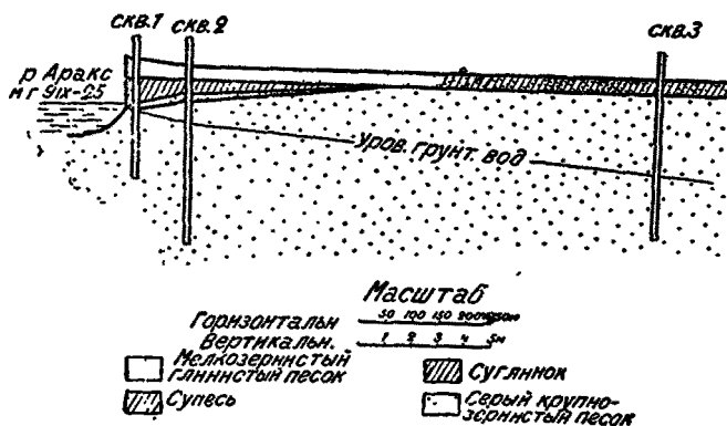
Рис. 72. Разрез по поперечнику буровых скважин к Араксу.
