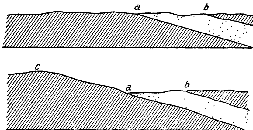
Рис. 58. Различные случаи питания водоносного слоя.
