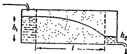
Рис. 123. Схематический разрез ящика Форхгеймера.
