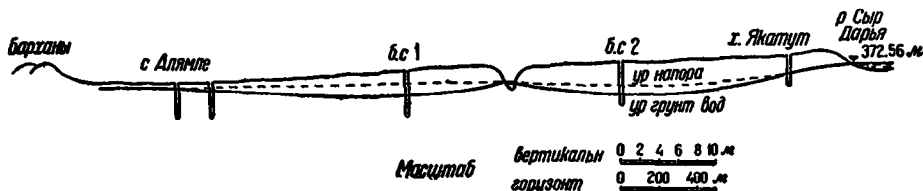
Рис. 74. Профиль через левобережье р. Сыр-Дарья в Фергане к Н от г. Коканда (по работам Ф. П. Саваренского).
