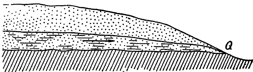
Рис. 31. Грунтовый поток.
