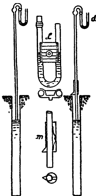
Рис. 42. Прибор Куната.
