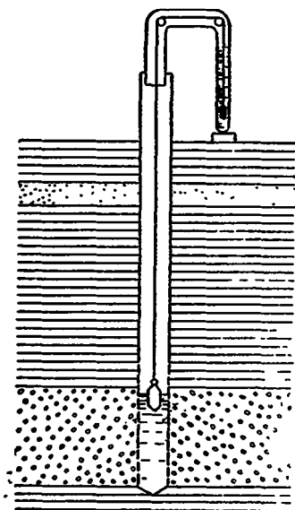
Рис. 147. Прибор С. А. Яковлевского для наблюдений над колебанием уровня грунтовых вод вне зависимости от барометрического давления воздуха.
