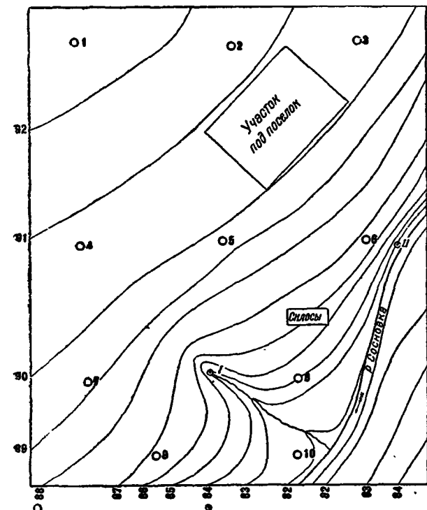
Рис. 56. Карта земель колхоза „Красная Зорька“ с указанием буровых скважин и источников. Для упрощения в построения гидроэвгипс.
