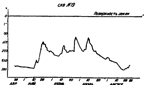
Рис. 142. Графики колебаний уровня воды в канале и в скважинах, заложенных: в дне канала (№ 15), в 18,2 м от оси канала (№ 18) и в 38,5 м от канала (№ 19).
