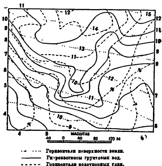
Рис. 50. Гидрогеологическая карточка территории Политехнического института в Новочеркасске (по К. И. Лисицину, схематизировано).
