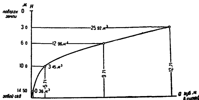
Рис. 98. Зависимость расхода воды при нагнетании в алмазную скважину № 2520 при равной высоте поглощения от забоя скважины.
