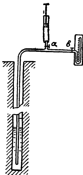
Рис. 43. Манометрический измеритель Н. К. Тихомирова.
