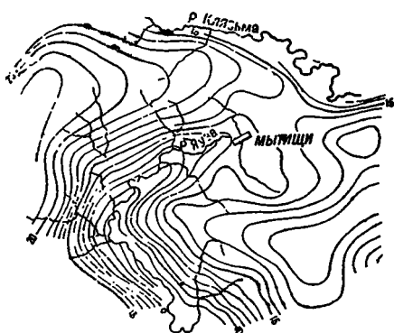
Рис. 77. Карта грунтовых вод Мытищинского района Московской в гидроэтинсах.
