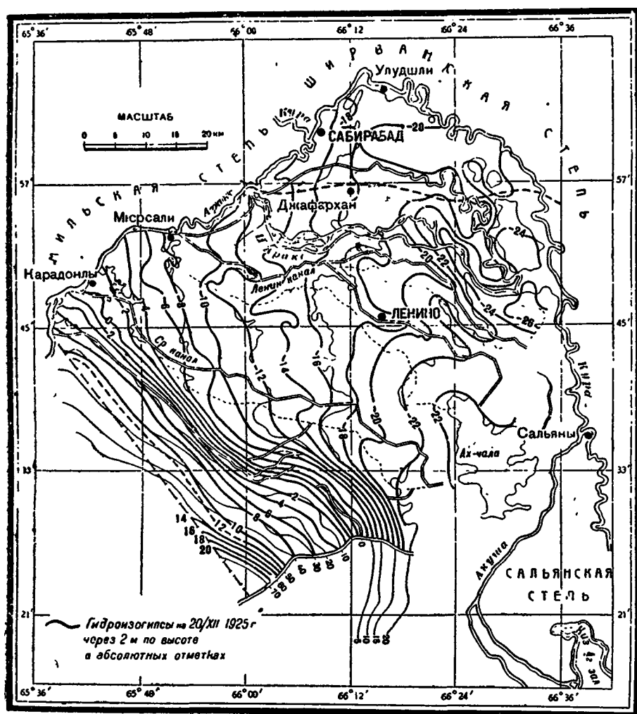
Рис. 49. Карта зеркала грунтовых вод Мунайской степи в гидроизогипсах на 20 декабря 1925 г.
