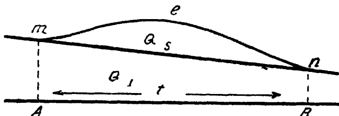
Рис. 18. Кривая расхода с волной паводка (по Труфанову).
