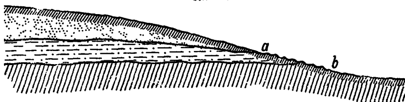
Рис. 37. Выход водоносного слоя, проявляющийся в заболачивании склона на протяжении ab .
