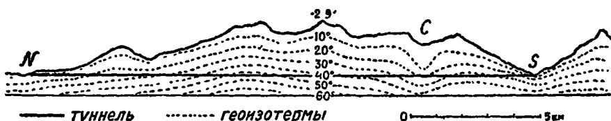
Рис. 5. Геоизотермы по профилю Симеоновского туннеля.
