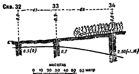
Рис. 90. Понижение уровня грунтовых вод под лесом (по П. В. Отоцкому).
