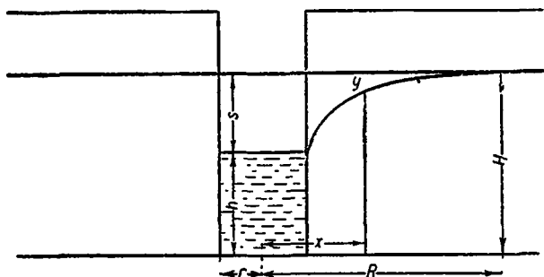
Рис. 125. Разрез колодца с воронкой депрессии.
