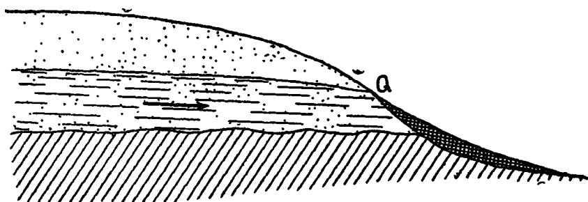
Рис. 34. Грунтовый поток, подпертый глинистым делювием.
