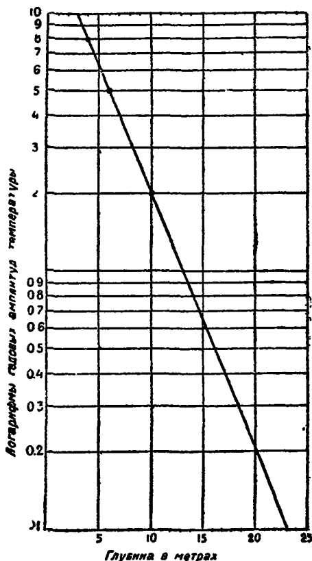
Рис. Графический способ определения глубины постоянного слоя температуры (по Огильви).
