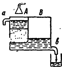
Рис. 121. Ящик Дарси для определения коэффициента фильтрации.
