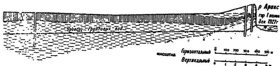
Рис. 71. Разрез левого берега р. Аракса в Араздайнской степи (Армения) по линии шурфов (из работ В. Ф. Захарова).
