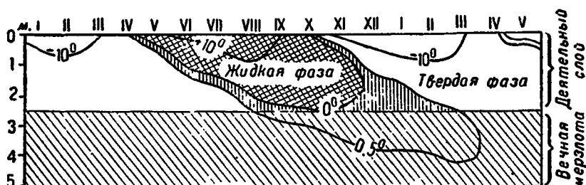
Рис. 101. График режима верховодки надмерзлотного слоя (схематизированный чертеж по И. Д. Белокрылову, заимствованный из статьи Н. И. Толстихина).
