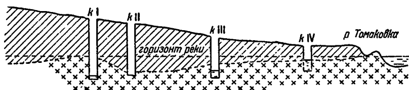
Рис. 97. Разрез левого берега р. Томаковки по колодцам с. Аяновки.
