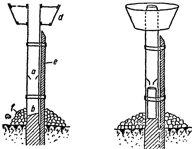
Рис. 7. Суммарные дождемеры (по В. К. Давыдову).
