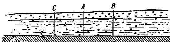
Рис. 132. Поперечный и продольный разрезы грунтового потока.
