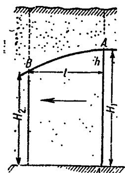
Рис. 120 Разрез участка подземного потока.
