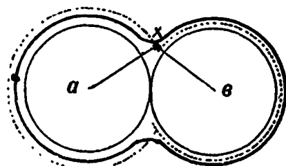
Рис. 24. Перемещение пленочной воды с одной частицы a на другую b .
