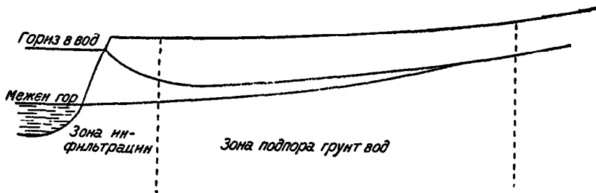
Рис. 69. Влияние подпора грунтовых вод высокими водами реки.
