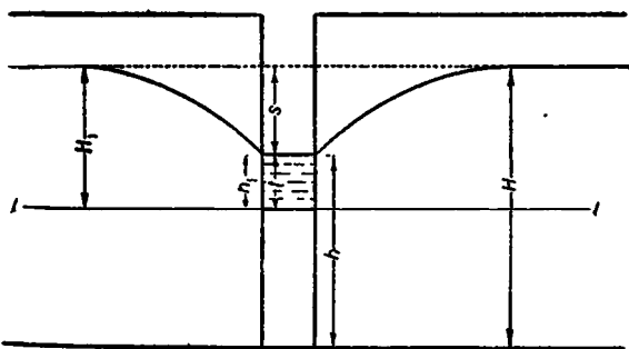
Рис. 126. Разрез несовершенного колодца.
