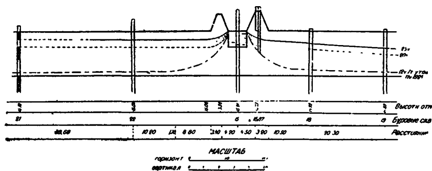
Рис. 141. Инфильтрация воды из канала в Муганской степи.
