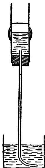
Рис. 28. Капилляр- метр.
