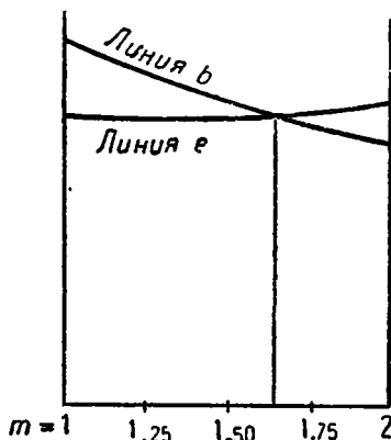
Рис. 127. Графический способ нахождения коэффициента m в формуле Сирекера.
