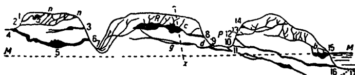
Рис. 100. Схематический профиль, объясняющий некоторые явления гидрографии карста, связанные с действием подземных карстовых каналов (по Кейльгаку).
