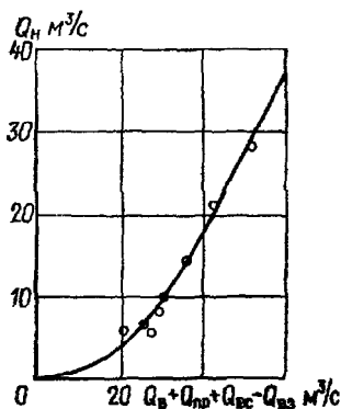
Рис. 6.8. Зависимость Q_n = f(Q_b + Q_{\text{пр}} + Q_{\text{вс}} - Q_{\text{вз}}) для участка р. Чу от Бурулдайского моста до г. Токмак.
