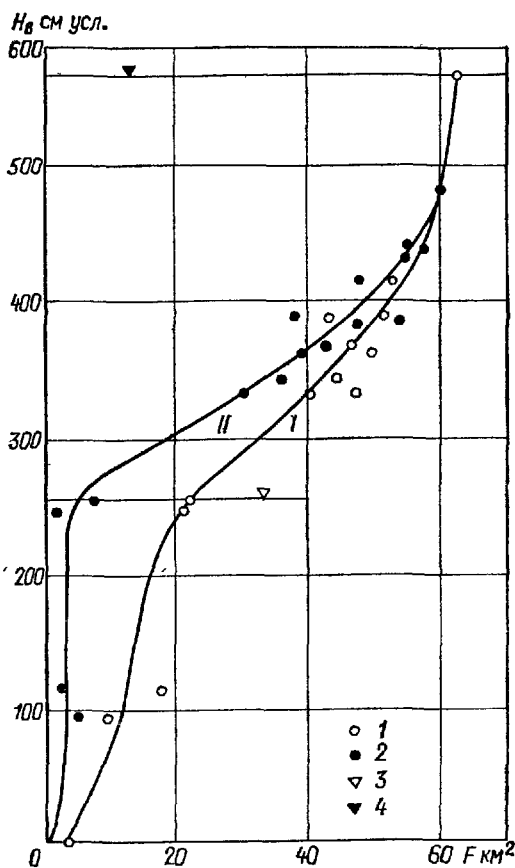
Рис. 6.3. Зависимость общей площади затопления F (I, 1) экспериментального участка р. Чу между 1-й и 3-й фермами Муюнкумского совхоза и его площади с открытой водной поверхностью F_B (II, 2) от уровня воды в верхнем створе участка H_B .
