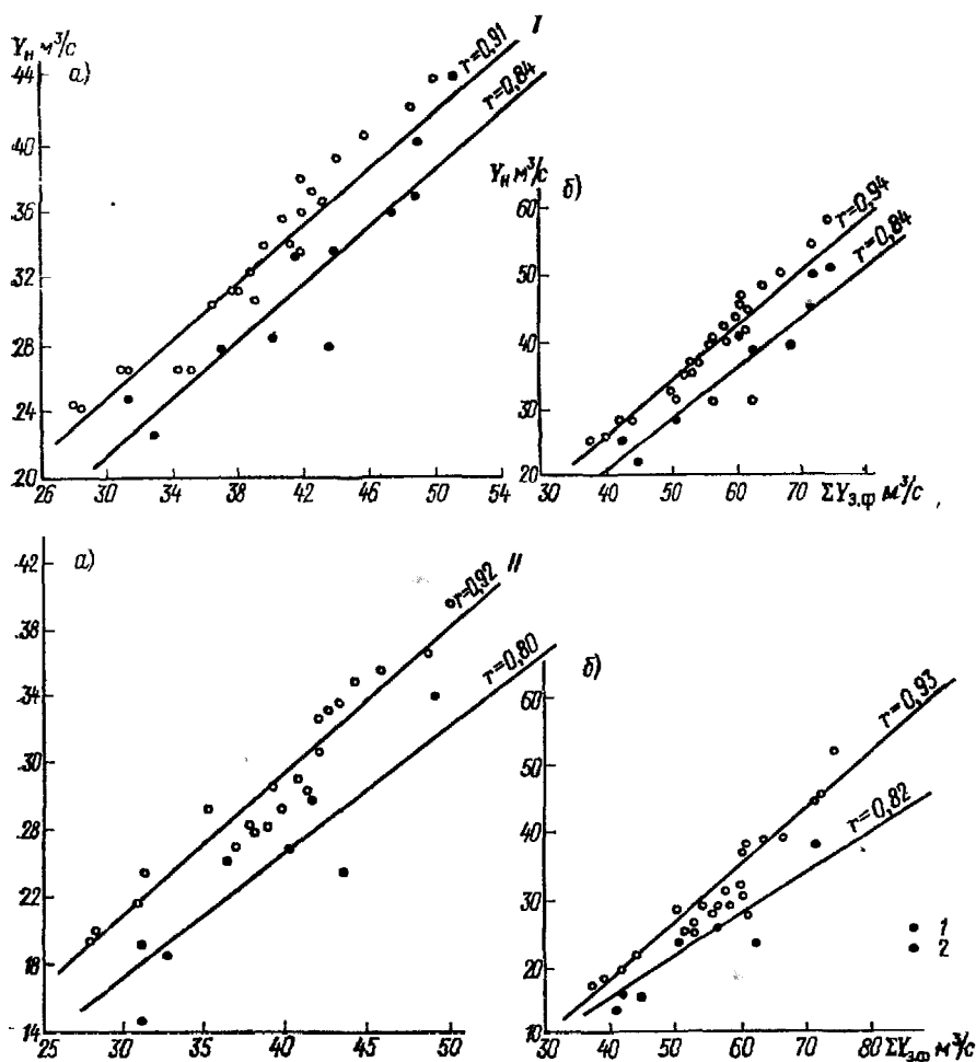
Рис. 9.4. Зависимость стока р. Талас у с. Кировское (I) и у с. Гродеково (с. Покровка) (II) ( Y_H ) от стока зоны формирования ( \Sigma Y_{з.ф.} ).
