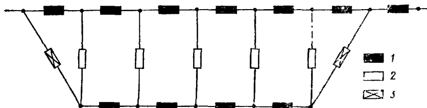
Рис. 9.8. Схематический разрез электрической модели Чуйской межгорной долины.
