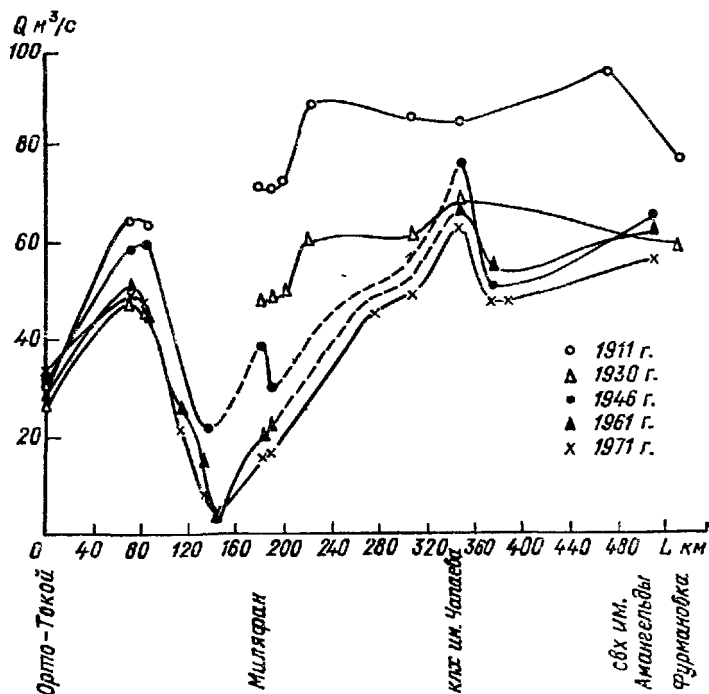
Рис. 9.1. Изменение стока р. Чу по ее долине за различные годы.
