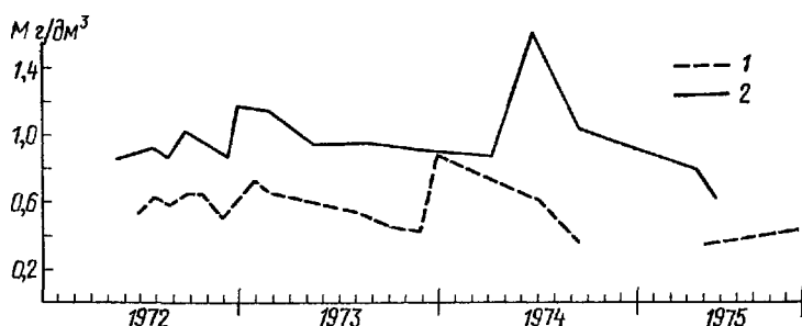
Рис 59 Изменение минерализации коллекторно-дренажных вод на Георгиевском орошаемом массиве
