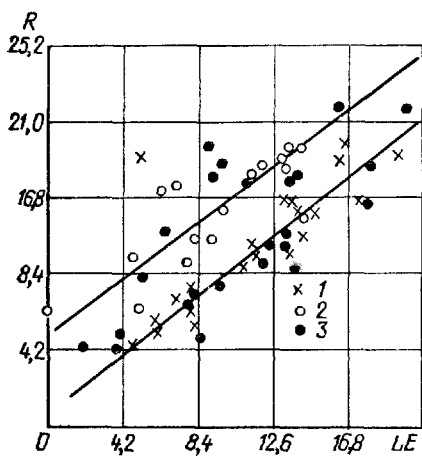
Рис 4.6 Зависимость затрат тепла на испарение LE от радиационного баланса R , люцерна, \text{МДж}/(\text{м}^2 \cdot \text{сут}) .
