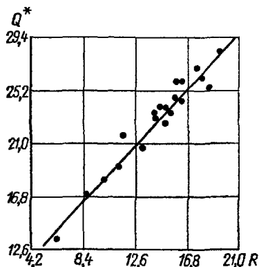
Рис. 4.3. Зависимость радиационного баланса орошаемого поля R , занятого сахарной свеклой, от суммарной радиации Q^* , МДж/(м 2 ·сут).
