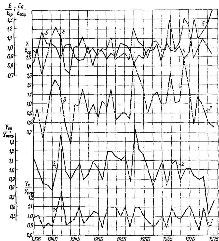
Рис. 10.1. Изменение во времени модульных коэффициентов притока Y_{пн}/Y_{пн.ср} (1) и оттока Y_{п}/Y_{п.ср} (2) поверхностных вод, осадков X/X_{ср} (3), испарения E/E_{ср} (4), испаряемости E_0/E_{0.ср} (5).
