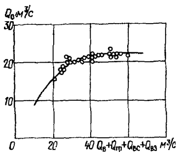
Рис. 6.9. Зависимость Q_0 = f(Q_b + Q_{\text{пр}} + Q_{\text{вс}} - Q_{\text{вз}}) для участка р. Чу от Бурулдайского моста до г. Токмак.
