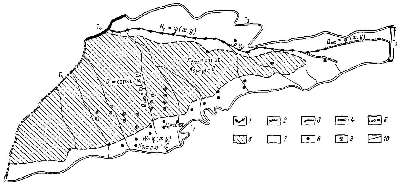
Рис. 9.7 Схема задания граничных условий при решении обратной стационарной задачи 1 — контур русла р. Чу с граничными условиями первого рода ( H_p = \varphi(x, y) ), 2 — контур русла р. Чу с граничными условиями второго рода ( Q_{p\Phi} = \varphi(x, y) ); 3 — контур модели с граничными условиями первого рода ( H\Gamma_4 = \text{const} ), 4 — внешний контур модели с граничными условиями второго рода ( Q\Gamma_4 = 0 , Q\Gamma_5 \neq 0 ), 5 — внешний контур модели по р. Кургата с граничными условиями третьего рода ( Q\Gamma_5 = (H_1 - H_{13})/\Phi ), 6 — участок, схематизированный как трехслойная система, 7 — участок, схематизированный как однослойный безнапорный водоносный горизонт, 8 — водозаборы, эксплуатирующие горизонт грунтовых вод ( Q_2 = \text{const} ), 9 — водозаборы, эксплуатирующие горизонт напорных вод; 10 — внутреннее русло реки типа «карасу», заданные граничными условиями второго рода ( Q_{кар} = \varphi(x, y) )
