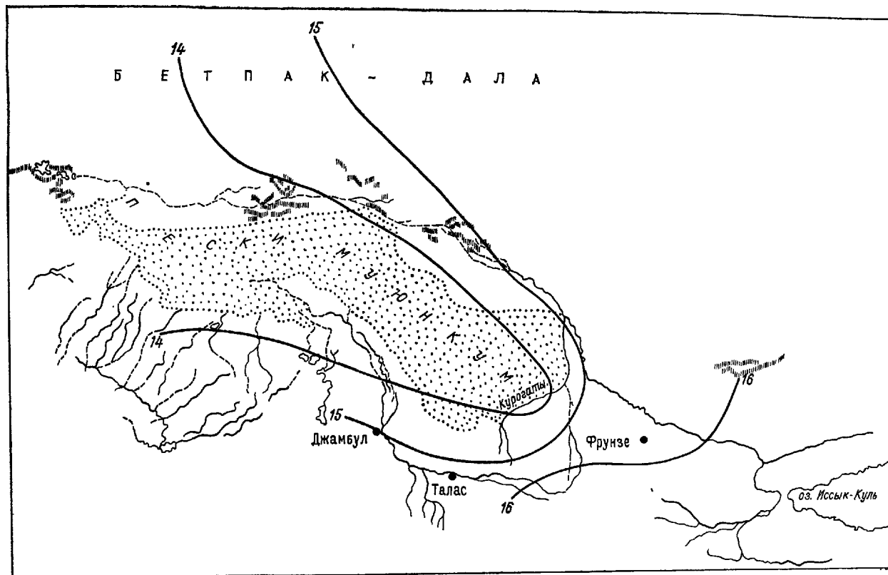
Рис. 7.2. Продолжительность периода вегетации сахарной свеклы (число декад),
