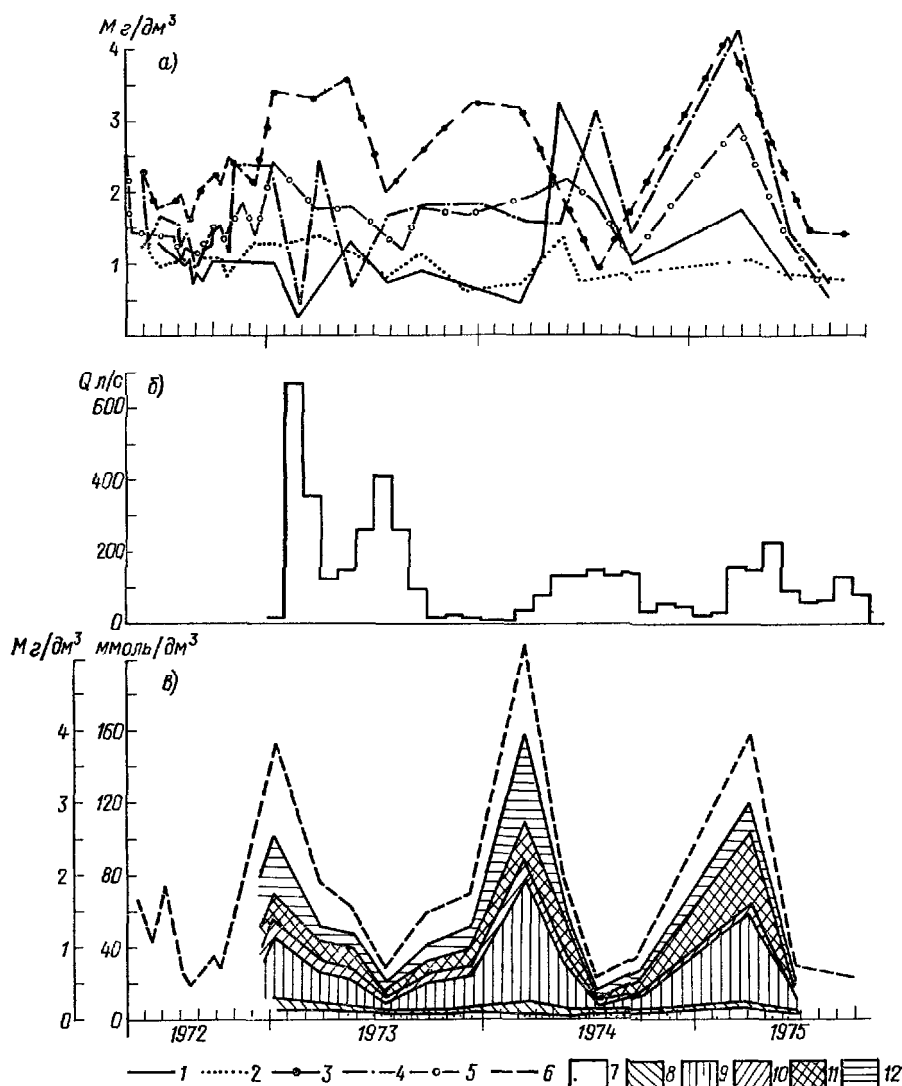
Рис. 5.7. Минерализация ( \text{г/дм}^3 ) и ионный состав ( \text{ммоль/дм}^3 ) коллекторно-дренажных вод орошаемого массива ЗБЧК.
