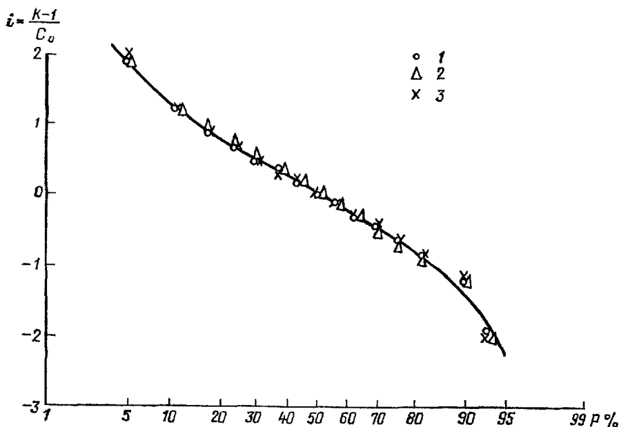
Рис. 7.5. Обобщенная кривая обеспеченности сумм недостатков водопотребления за период вегетации различных сельскохозяйственных культур.
