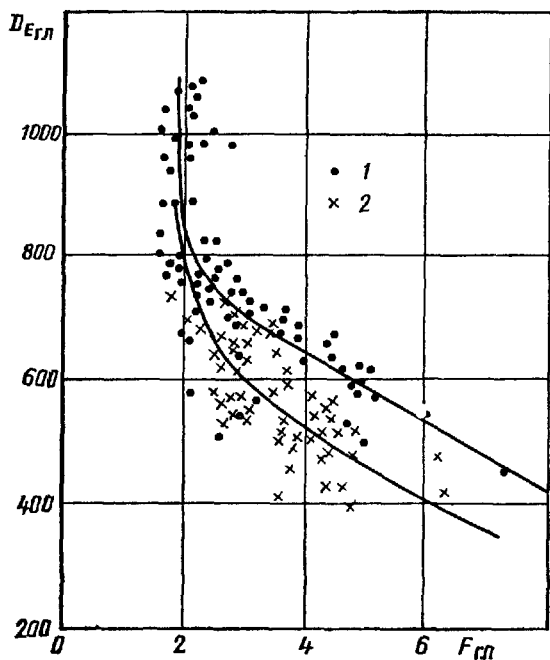
Рис. 7.9. Зависимость F_{ГЛ}=f(D_{E_{ГЛ}}) для сахарной свеклы.
