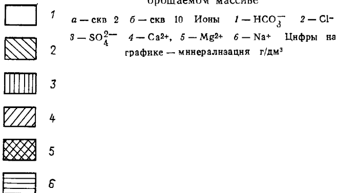
Рис 5 11. Ионный состав (ммоль/дм 3 ) и минерализация грунтовых вод на Ат-Башинском орошаемом массиве
