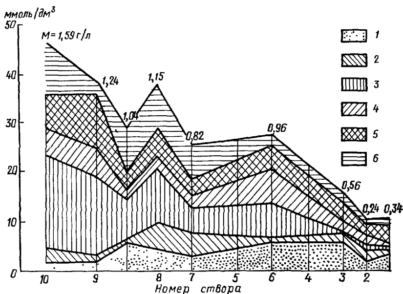
Рис. 5.12. Гидрохимический разрез правого склона долины р. Чу в осенний период.
