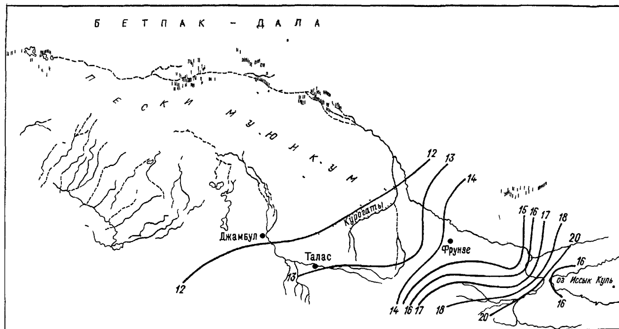
Рис 71 Продолжительность периода вегетации яровой пшеницы (число декад)
