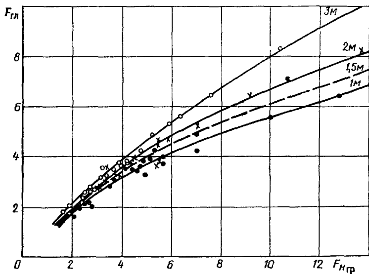
Рис. 7.10. Зависимость F_{НГР}=f(F_{ГЛ}) .
