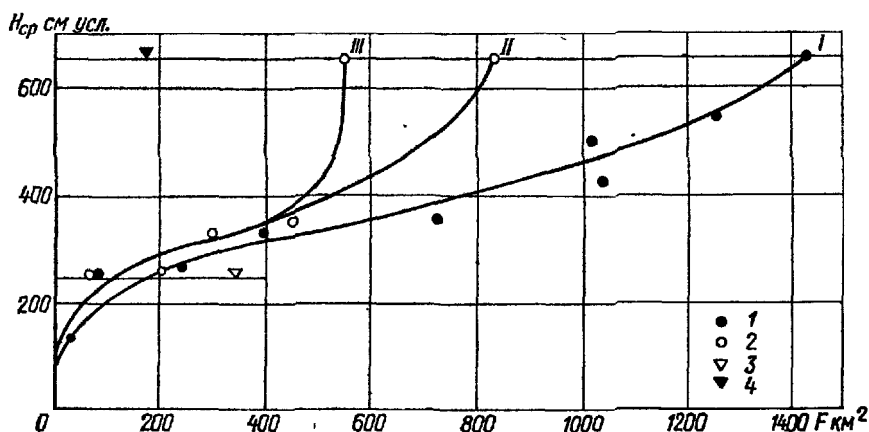
Рис. 6.1. Зависимость общей площади затопления F (I, I) участка р. Чу от свх им. Амангельды до 1-й фермы Муюнкумского совхоза, площади этого участка, занятой полупогруженными тростниковыми и тугайными зарослями F_{\text{тр}} + F_{\text{туг}} (II, 2) и площади, занятой полупогруженными тростниковыми зарослями F_{\text{тр}} (III), от среднего уровня воды на участке H_{\text{ср}} .
