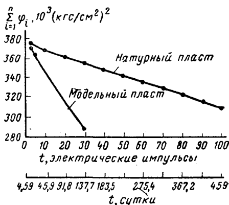
Рис. 100. Зависимости \sum_{i=1}^n \varphi_i = f(t) для скважин натурной и модельной залежей [19]
