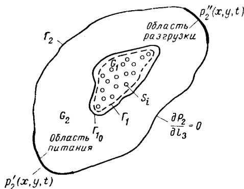
Рис. 63. Схема двумерной задачи с подвижной границей раздела газ—вода:
