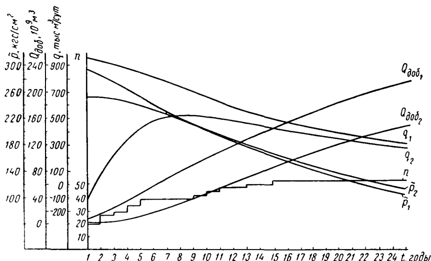
Рис. 65. Изменение во времени показателей разработки месторождения C в условиях газового режима (вариант с p_{н1} = 300 кгс/см 2 , p_{н2} = 250 кгс/см 2 )
