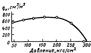
Рис. 75. Исходная для расчетов изотерма конденсации [66]
