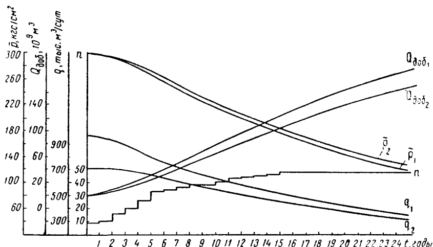
Рис. 64. Изменение во времени показателей разработки месторождения C в условиях газового режима (вариант с p_{H1} = p_{H2} = 300 \text{ кгс/см}^2 )
