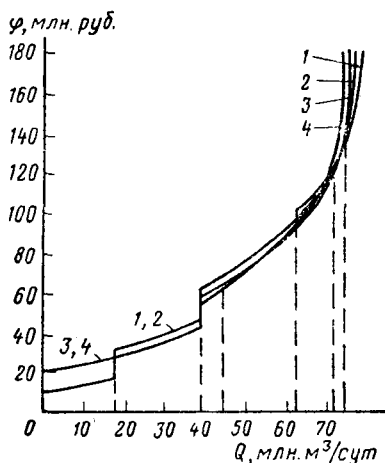
Рис. 94. Зависимость экономического показателя разработки многопластового месторождения от темпа отбора газа из него для различных вариантов разработки и обустройства:
