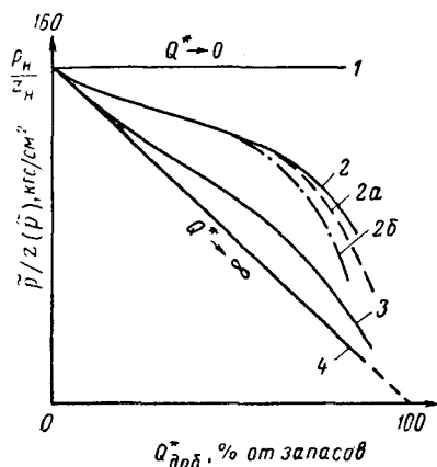
Рис. 4. Примеры зависимостей \bar{p}/z(\bar{p}) = f[Q_{\text{доб}}^*(t)] для газовой залежи
