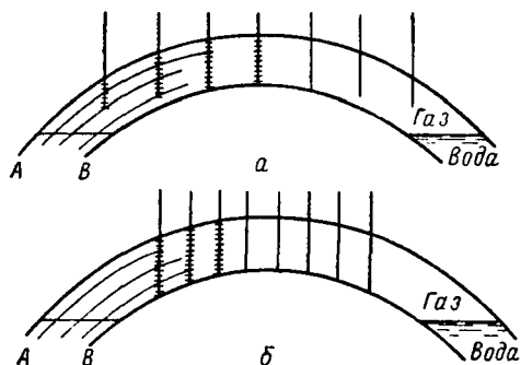
Рис. 27. Схемы равномерного размещения скважин с избирательным вскрытием и размещением скважин в центральной зоне с полным вскрытием продуктивного пласта
