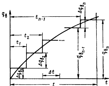
Рис. 59. Аппроксимация зависимости изменения во времени дебита поступающей в залежь воды ступенчатой зависимостью
