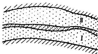
Рис. 69. Продуктивные пласты I и II, разделенные слабопроницаемой перемычкой
