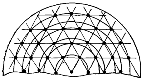
Рис. 22. К возможности сведения равномерной сетки размещения скважин к системе размещения в виде батарей
