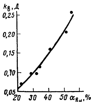
Рис. 13. Зависимость коэффициента фазовой проницаемости для воды от коэффициента начальной водонасыщенности модели
