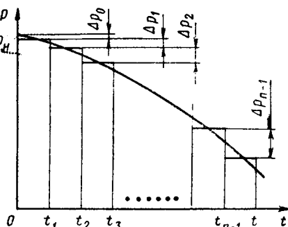
Рис. 54. Аппроксимация зависимости изменения во времени давления на стенке укрупненной скважины ступенчатой зависимостью
