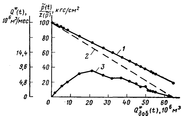
Рис. 6. Изменение отбора газа Q^* из залежи в процессе разработки (3) и зависимость \bar{p}/z(\bar{p}) = f[Q_{\text{доб}}^*(t)] для газового (2) и водонапорного (1) режимов
