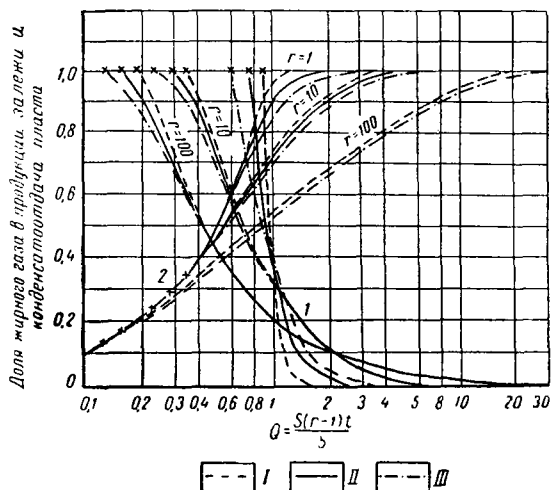
Рис. 87. Расчетные кривые изменения относительного содержания жирного газа в продукции скважин, а также конденсатоотдачи пласта в зависимости от отношения объема закачанного газа к общему газонасыщенному объему в случае сложистой модели пласта:
