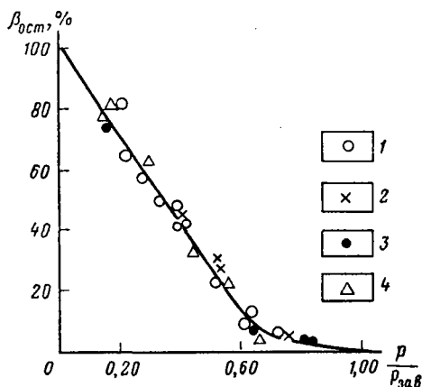
Рис. 14. Изменение коэффициента газоотдачи (по заземленному газу) обводненной модели при снижении давления в ней. Номера опытов: 1—10; 2—11; 3—12; 4—13; 5—14
