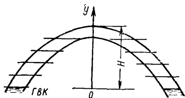
Рис. 60. Разбивка залежи на элементарные объемы: Н — этаж газонасыщенности
