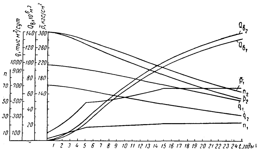
Рис. 72. Изменение во времени показателей разработки месторождения C в условиях водопарного режима и слабопроницаемой перемычки между пластами
