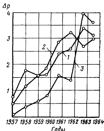
Рис. 99. Изменение во времени темпа падения пластового давления в разных частях Северо-Ставропольского месторождения. Темп падения пластового давления:
