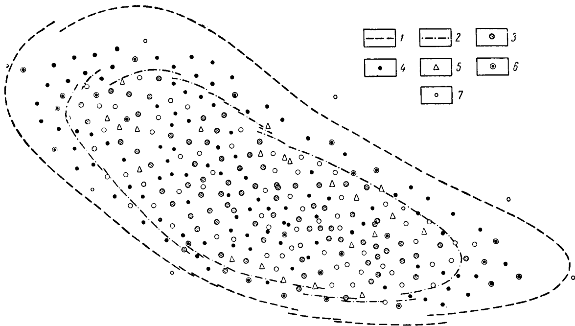
Рис. 25. Карта размещения существующих и проектных скважин на свиту медистых песчаников Шеллинского месторождения (по уточненному проекту разработки, 1964 г.):
