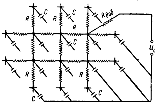
Рис. 40. Схема сетки RC
