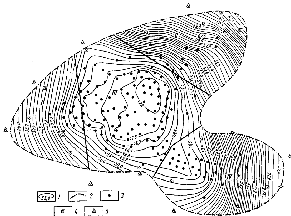
Рис. 96. Карта изобар хадумской газовой залежи на 15/VI 1964 г:
