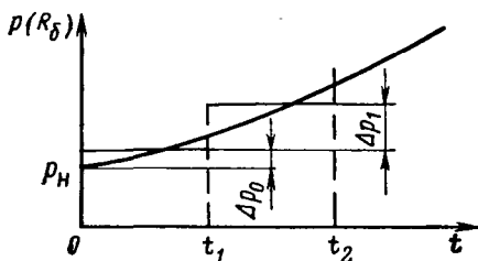
Рис. 88. Аппроксимация зависимости изменения во времени давления на линии нагнетания ступенчатой зависимостью
