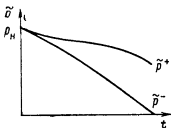
Рис. 55. Зависимости изменения во времени завышенных \tilde{p}^+ и заниженных \tilde{p}^- средних пластовых давлений в залежи
