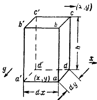
Рис. 10. Элементарный объем пласта
