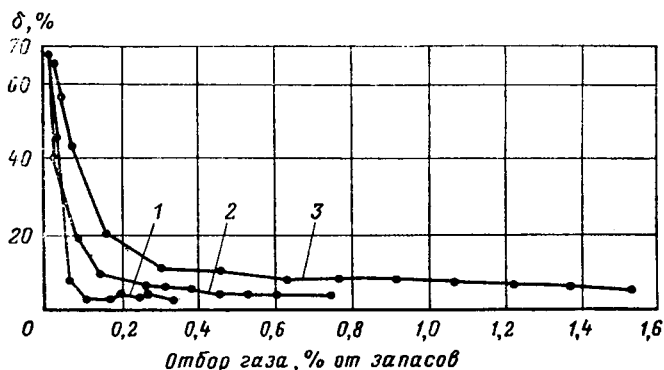
Рис. 101. Зависимость погрешности определения запасов газа от суммарного отбора из месторождения при различном числе эксплуатационных скважин [19]
