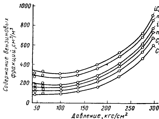
Рис. 77. Изменение выхода бензиновых фракций в процессе разработки газоконденсатного месторождения
