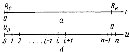
Рис. 37. К переходу от пространственной координаты r (а) к координате u = \ln r (б)
