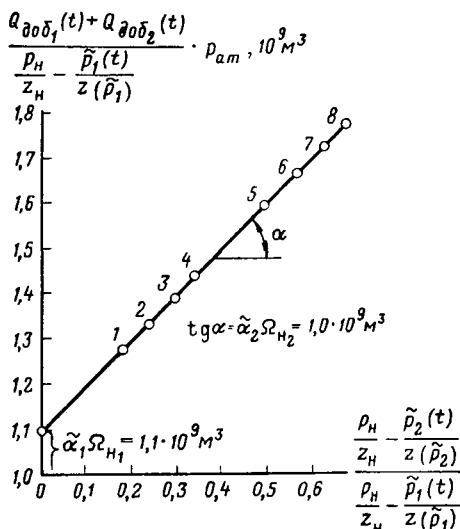
Рис. 103. К определению запасов газа отдельных пластов и интегрального фильтрационного параметра слабопроницаемой перемычки
