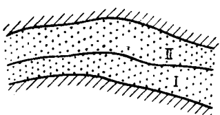
Рис. 68. Схема непосредственного контакта продуктивных пластов I и II
