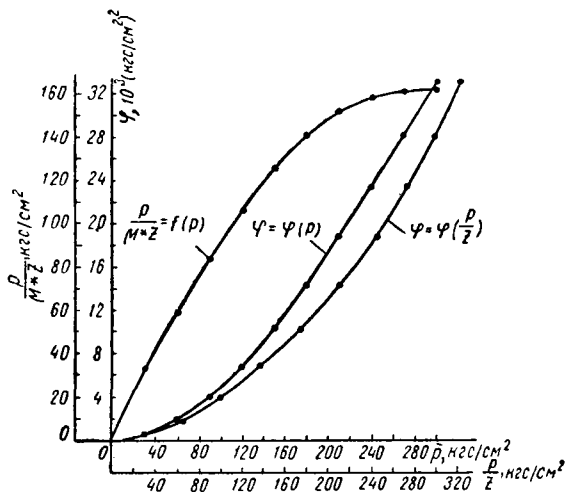
Рис. 34. Зависимости \varphi = \varphi(p) , \bar{\varphi} = \varphi(p/z) и подынтегрального выражения (3) для газа месторождения А
