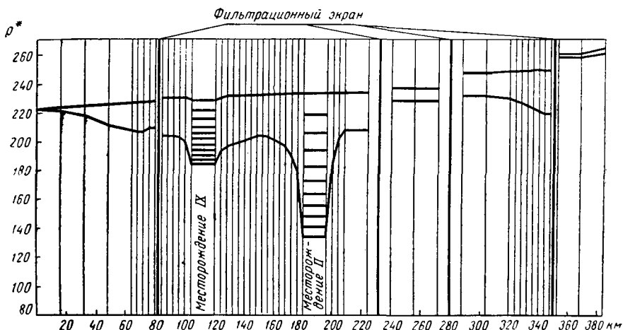
Рис. 74. Расчетные профили (по сечению I—I — см. рис. 73) приведенного пластового давления по водонапорной системе нижнемеловых отложений Западного Предкавказья на разные даты
