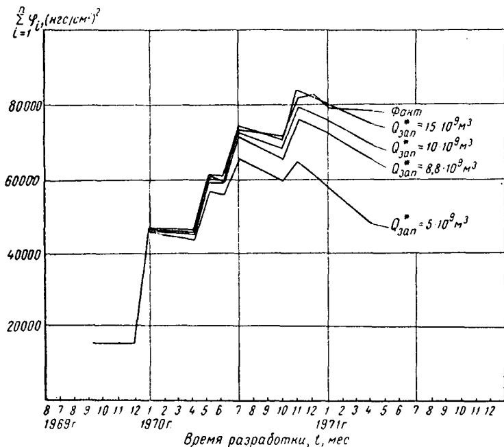
Рис. 102. Последовательные приближения при определении запасов газа Совхозного месторождения
