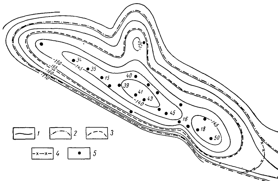
Рис. 1. Структурная карта Султангуловского месторождения:
