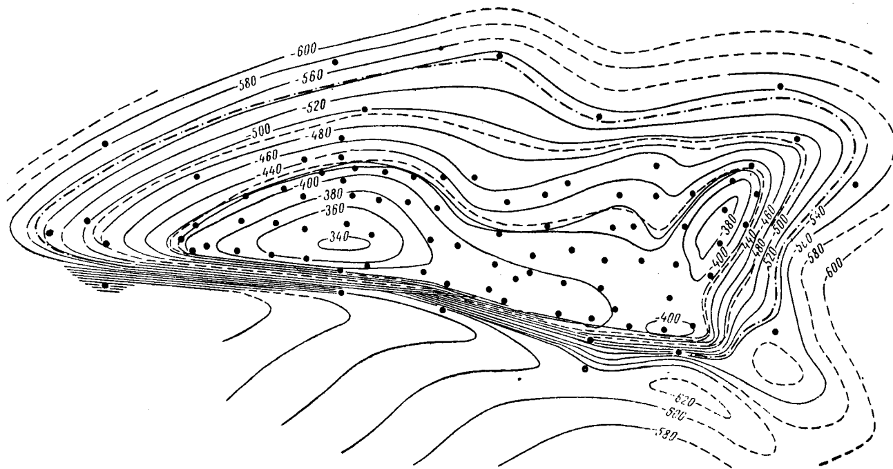
Рис. 24. Карта размещения проектных скважин на IX горизонт месторождения Газли (по проекту разработки 1960 г.)
