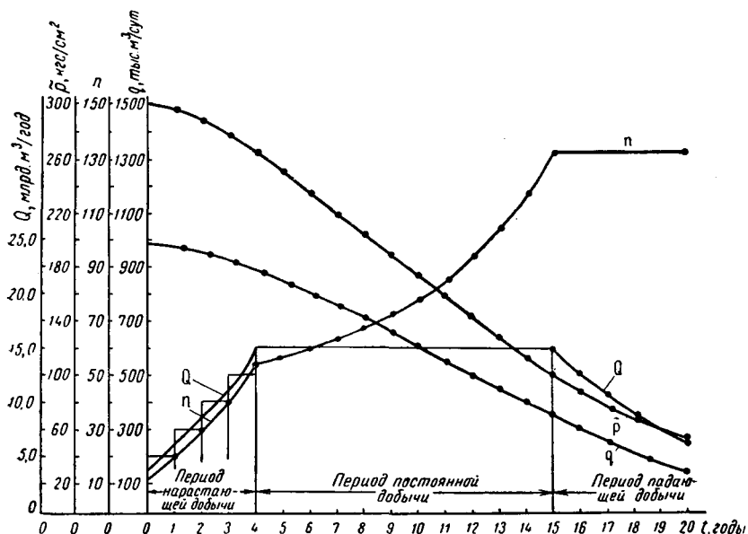
Рис. 15. Изменение во времени показателей разработки месторождения А при газовом режиме, равномерном размещении скважин по площади газоносности и пренебрежении реальными свойствами газа
