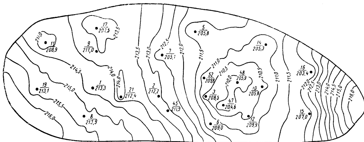
Рис. 50. Расчетная карта изобар месторождения Б после четырех лет разработки
