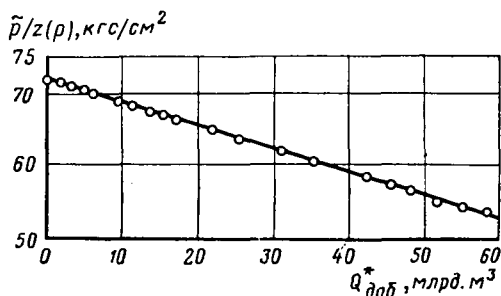
Рис. 95. Зависимость \bar{p}/z(\bar{p}) = f\{Q_{доб}^*(t)\} для Северо-Ставропольского месторождения
