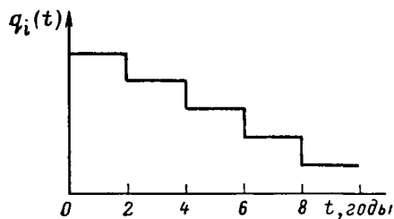
Рис. 49. Характер изменения дебитов скважин месторождения Б
