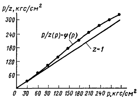
Рис. 32. Зависимость p/z(p) = \varphi(p) для газа месторождения А
