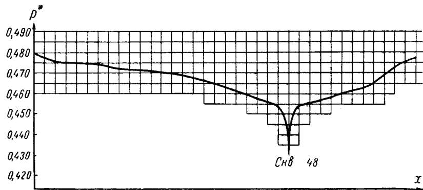
Рис. 53. Профиль безразмерного давления вдоль горизонтальной линии ( j=14 )
