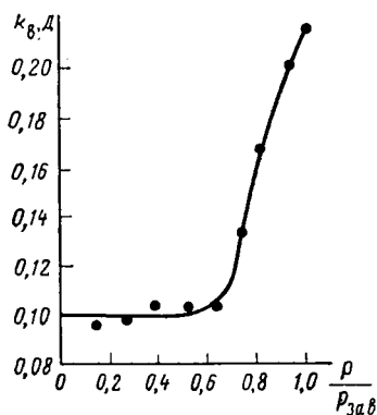
Рис. 12. Изменение коэффициента фазовой проницаемости для воды при снижении давления в обводненной модели пласта (модель № 1) [71]
