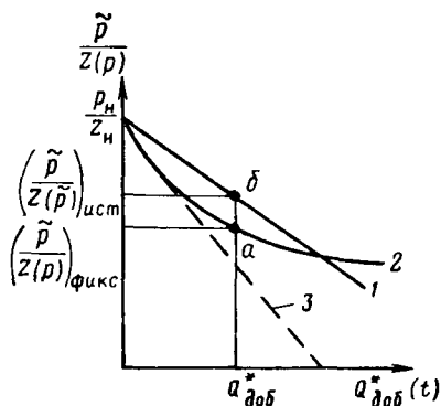
Рис. 8. Влияние неравномерности дренирования продуктивных отложений по мощности на характер зависимости \tilde{p}/z(\tilde{p}) = f[Q_{доб}^*(t)]
