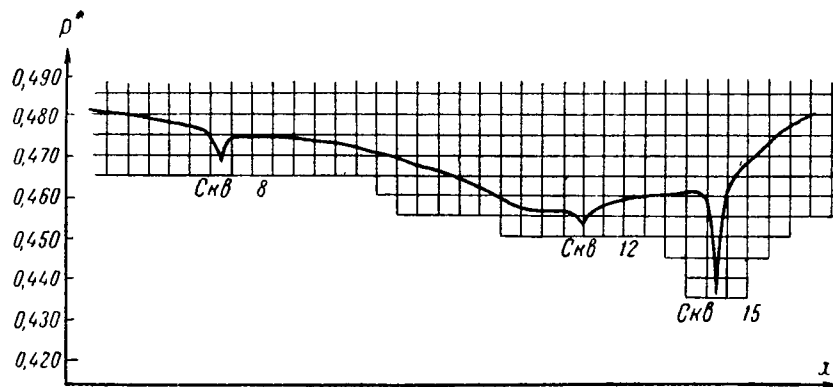
Рис. 52. Профиль безразмерного давления вдоль горизонтальной линии ( j=7 )
