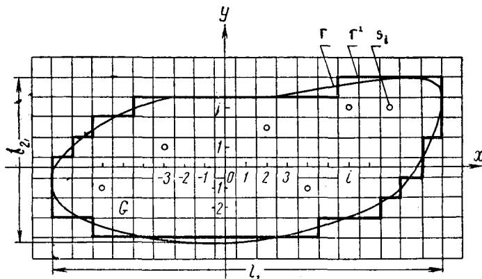
Рис. 46. Схема аппроксимации области газоносности сеточной областью
