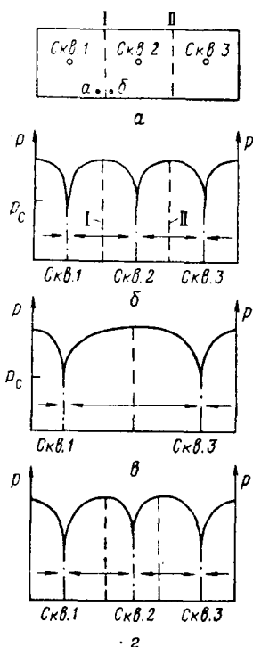
Рис. 2. Профили пластового давления по Султангуловскому месторождению на разные даты после закрытия эксплуатационных скважин (по оси абсцисс указаны номера эксплуатационных скважин)
