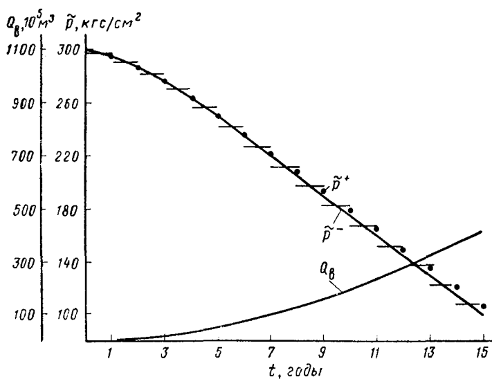
Рис. 58. Результаты расчетов по продвижению воды в месторождение А при ухудшенной проницаемости пласта в водоносной зоне
