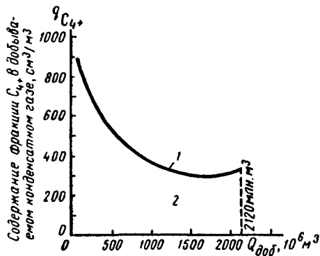
Рис. 79. 1 — изменение содержания конденсата в добываемом газе в функции суммарного количества газа; 2 — площадь, соответствующая суммарной добыче конденсата 935 тыс. м 3
