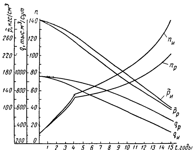
Рис. 33. Изменение во времени показателей разработки месторождения А с учетом реальных свойств газа (индексы «р») и без учета этих свойств (индексы «и»)
