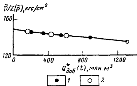
Рис. 5. Зависимость \bar{p}/z(\bar{p}) = f[Q_{\text{доб}}^*(t)] для залежей 2 и 3 в III горизонте Анастасиевско-Троицкого месторождения:
