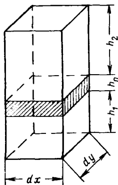
Рис. 70. Элементарный объем при наличии между пластами слабопроницаемой перемычки
