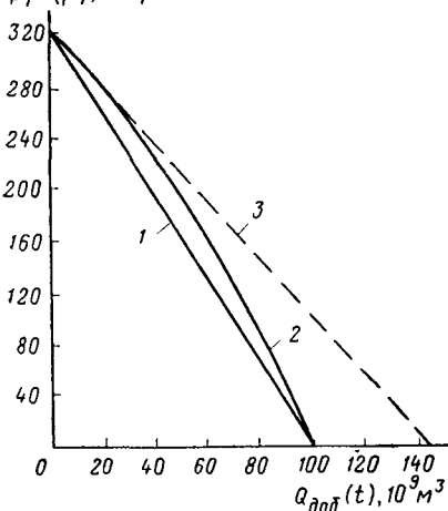
Рис. 9. Зависимости \tilde{p}/z(\tilde{p}) = f[Q_{доб}(t)] для деформируемого (2) и недеформируемого (1) коллекторов при одинаковых запасах газа в залежи
