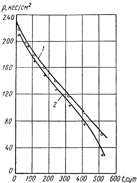
Рис. 42. Сопоставление результатов решения задачи на ЭВМ и на электроинтеграторе (см. табл. 10 и 11):
