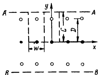
Рис. 82. Схема расположения цепочки нагнетательных и двух цепочек эксплуатационных скважин
