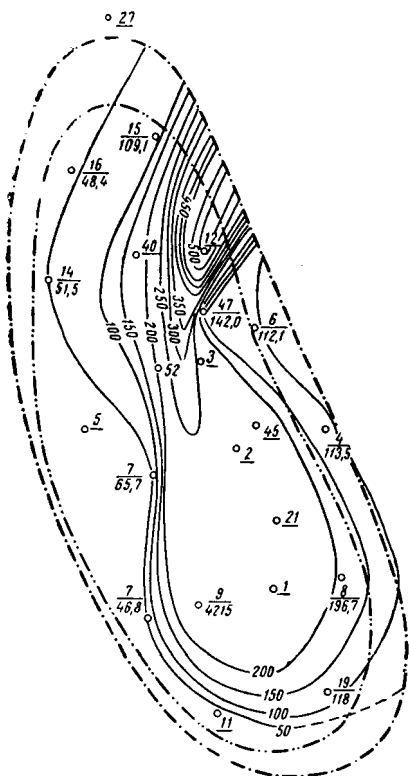
Рис. 47. Карта равных значений параметра проводимости месторождения Б
