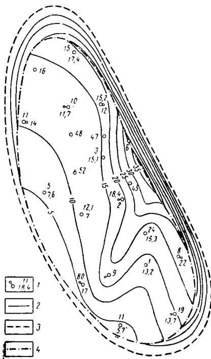
Рис. 48. Карта равных значений эффективной мощности пласта месторождения Б:
