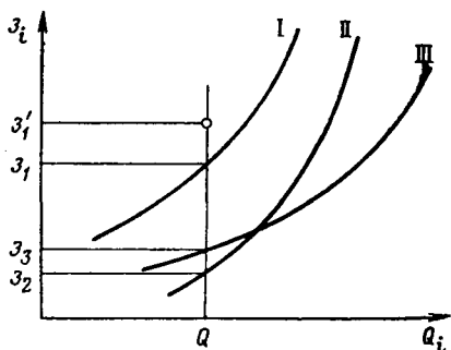
Рис. 91. Зависимости приведенных затрат от уровня добычи газа для месторождений I, II и III
