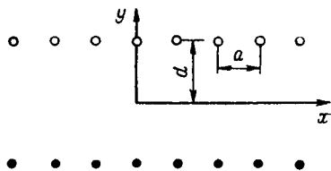
Рис. 80. Схема размещения эксплуатационных и нагнетательных скважин в виде цепочек
