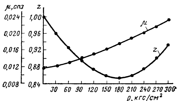
Рис. 31. Зависимости коэффициентов сверхсжимаемости газа и динамической вязкости от давления для газа месторождения А
