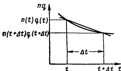
Рис. 29. К построению численной методики определения показателей разработки газовой залежи в период падающей добычи
