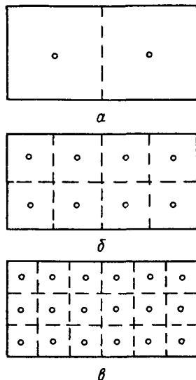
Рис. 21. Схема уплотнения сетки скважин
