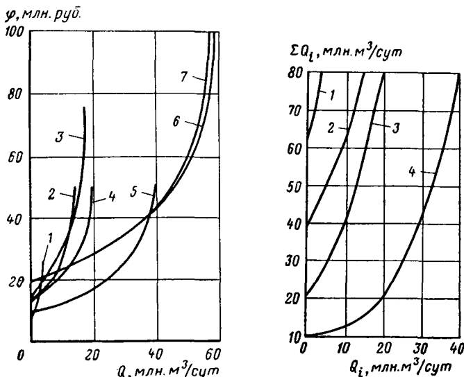
Рис. 92. Целевые функции для различных вариантов разработки многопластового месторождения (типа Газли):
