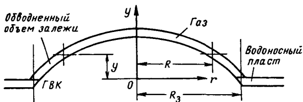
Рис. 62. Схематизация залежи и водоносного пласта при расчете продвижения в залежь контурной воды
