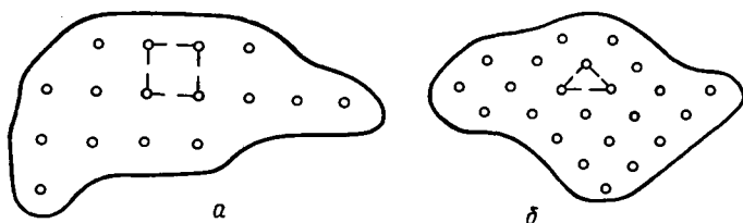
Рис. 16. Схема размещения скважин по равномерной сетке: а — квадратная сетка; б — треугольная сетка
