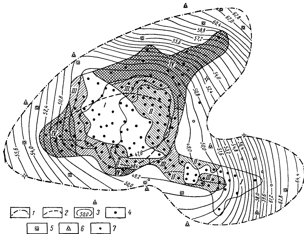
Рис. 98. Схема ввода в разработку отдельных участков хадумской залежи Северо-Ставропольского месторождения:
