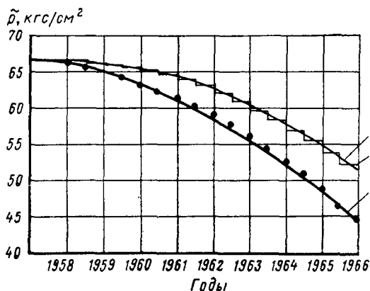
Рис. 104. К уточнению параметров водоносного пласта по данным разработки Северо-Ставропольского месторождения
