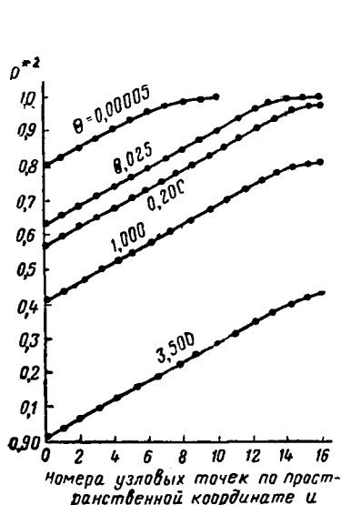
Рис. 38. Профили квадратов давления в разные моменты безразмерного времени для Q^* = 0,01 [39]
