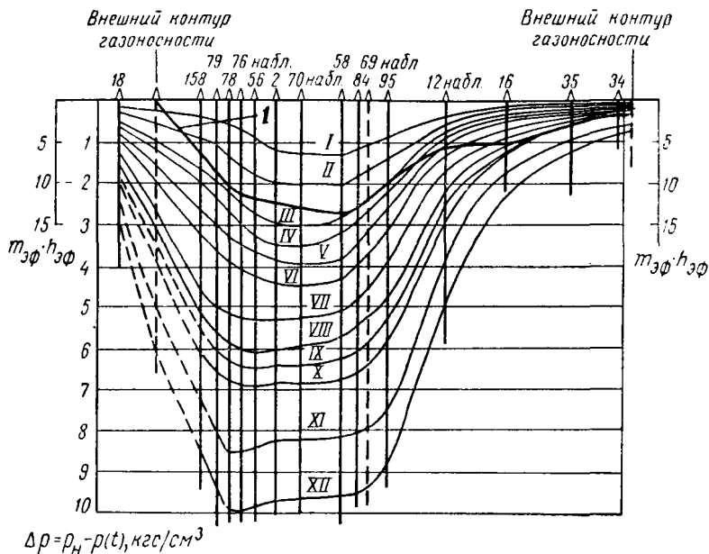
Рис. 45. Формирование общей депрессионной «воронки»:
