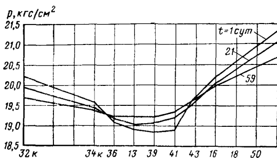
Рис. 2. Профили пластового давления по Султангуловскому месторождению на разные даты после закрытия эксплуатационных скважин (по оси абсцисс указаны номера эксплуатационных скважин)
