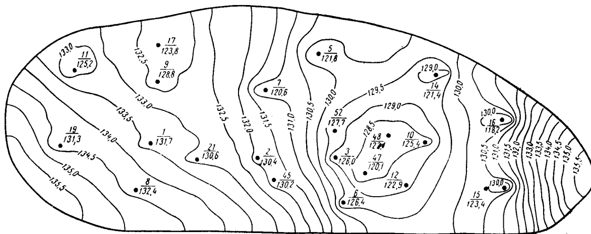
Рис. 51. Расчетная карта изобар месторождения Б после 10 лет разработки
