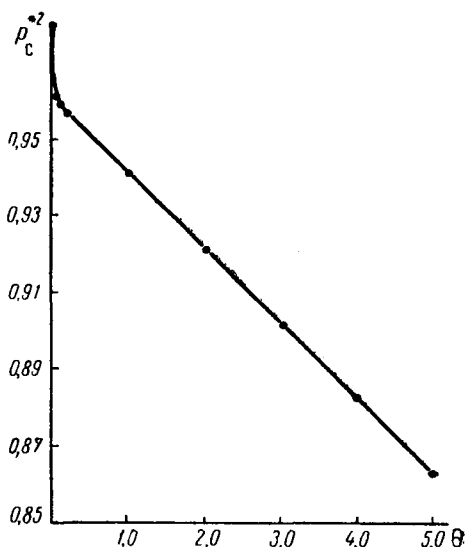
Рис. 39. Изменение квадрата безразмерного забойного давления в функции безразмерного времени
