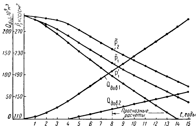
Рис. 71. Изменение во времени показателей разработки месторождения C в условиях газового режима и наличия слабопроницаемой перемычки между пластами
