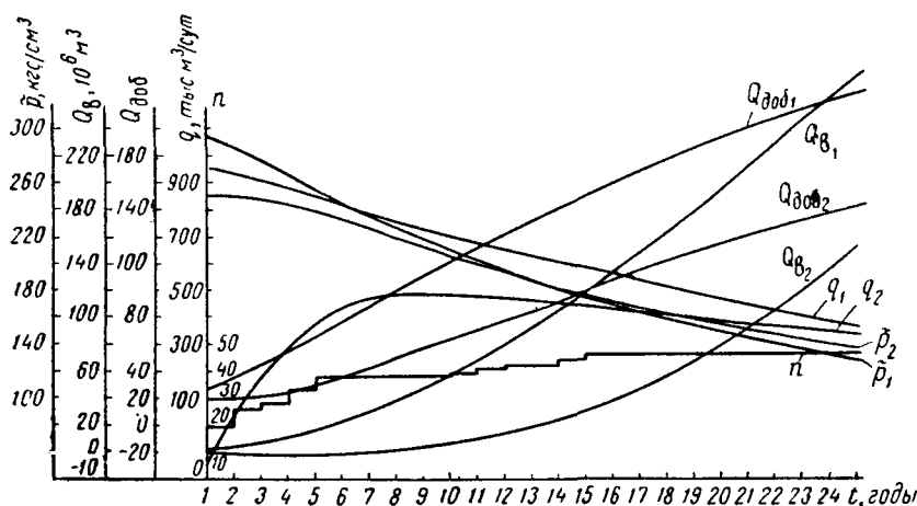
Рис. 67. Показатели разработки двухпластового месторождения C в условиях водонапорного режима (вариант с p_{н1} = 300 кгс/см 2 , p_{н2} = 250 кгс/см 2 )
