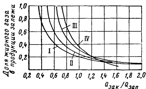
Рис. 85. Зависимость доли жирного газа в продукции (от начального содержания) от отношения количества закачанного сухого газа Q_{зак} к начальным запасам газа в пласте Q_{зап} [46]:
