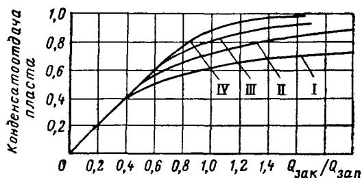
Рис. 86. Зависимость доли отобранного количества жирного газа (от начальных его запасов) от отношения количества закачанного сухого газа к начальным запасам газа в пласте [46].
