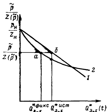
Рис. 7. Влияние неконтролируемых утечек газа на зависимость p/z(\tilde{p}) = f[Q_{доб}^*(t)]
