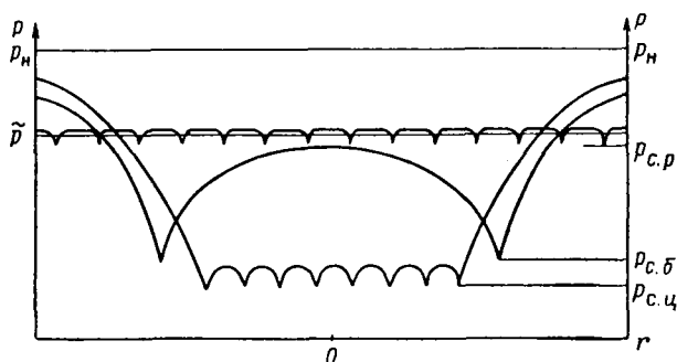
Рис. 26. Профили пластового давления для вариантов равномерного, батарейного и центрального размещения скважин на залежи, однородной по коллекторским свойствам (при одинаковом добытом количестве газа)
