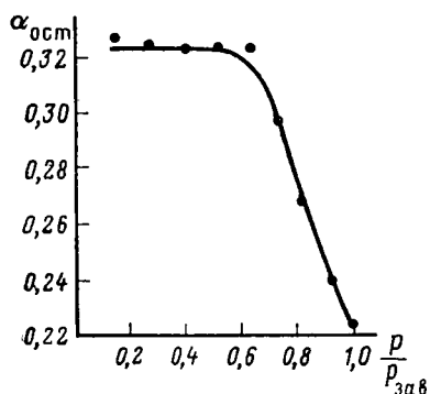
Рис. 11. Изменение коэффициента остаточной газонасыщенности при снижении давления p в обводненной модели. Модель № 1, коэффициент начальной газонасыщенности 0,74; p_{зав} — давление заводнения модели [71]
