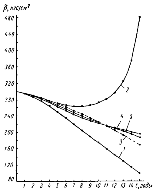
Рис. 57. Последовательные приближения при расчете поступления подопленной воды в месторождение А
