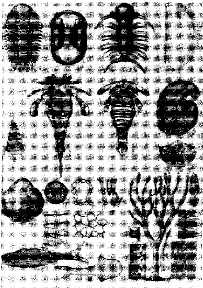
Рис. 11.1. Характерные представители силурийских организмов. Трилобиты: 1 — Cheirurus ; 2 — Illaenus ; 3 — Sciphoion . Граптолиты: 4 — Monograptus ; 5 — Rastrites ; 6 — Spiriograptus . Рафоскорпионы: 7 — Eurypterus ; 8 — Pterygotus . Брахиоподы: 9 — Conchidium ; 10 — Eospirifer ; 11 — Pentamerus . Кишечнополостные: 12 — Streptelasma ; 13 — Halysites ; 14 — Palaeofavosites . Двоякодышащие рыбы: 15 — Lamarkia ; 16 — Birkenia . Растения: 17 — Lepidodendron : а — реставрированное дерево; б и с — куски коры; d — кусок ствола с листьями; е — лист; f — плодовая шишка; g — два листа из шишки с плодами
