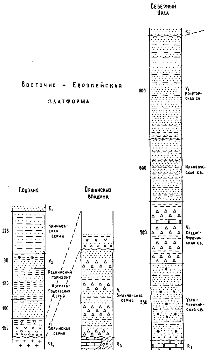
Рис. 8.1. Сопоставление разрезов вендской системы: 1 — конгломераты; 2 — тиллиты; 3 — пески и песчаники; 4 — алевролиты; 5 — глины; 6 — глины и глинистые сланцы; 7 — мергели и глинистые известняки; 8 — известняки; 9 — доломиты; 10 — угли; 11 — гипсы и ангидриты; 12 — соли; 13 — глинистые и кристаллические сланцы; 14 — складчатый фундамент; 15 — гранитоиды; 16 — основные эффузивы; 17 — кислые эффузивы; 18 — красноцветы; 19 — глаукониты; 20 — фосфориты
