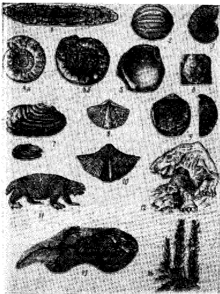
Рис. 14.1. Характерные представители пермских организмов. Простейшие: 1 — Pseudofusulina ( C_3 — P_1 ); 2 — Schwagerina ( P_1 ). Агонииатиты: 3 — Medlicottia . Гониатиты: 4a и 4b — Paragastrioceras ( P_1 ). Двустворчатые моллюски: 5 — Eurydesma ; 6 — Pseudomonotis speluncaria ; 7 — Allorisma komiensis . Брахиоподы: 8 — Licharewia ( P_2 ); 9 — Productus canerini ; 10 — Spirifer regularis . Пресмыкающиеся: 11 — Pareiasaurus ( P_2 ); 12 — Inostrancevia ( P_2 ). Земноводные: 13 — Eryops . Растения: 14 — Walchia ( C_3 — P_1 )
