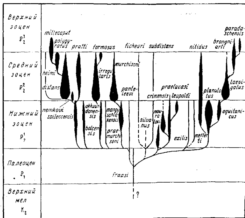
Рис. 2.4. Схема филогенетических взаимоотношений видов пуммулитов, подрод Nummulites (по Г. Н. Немкову)
