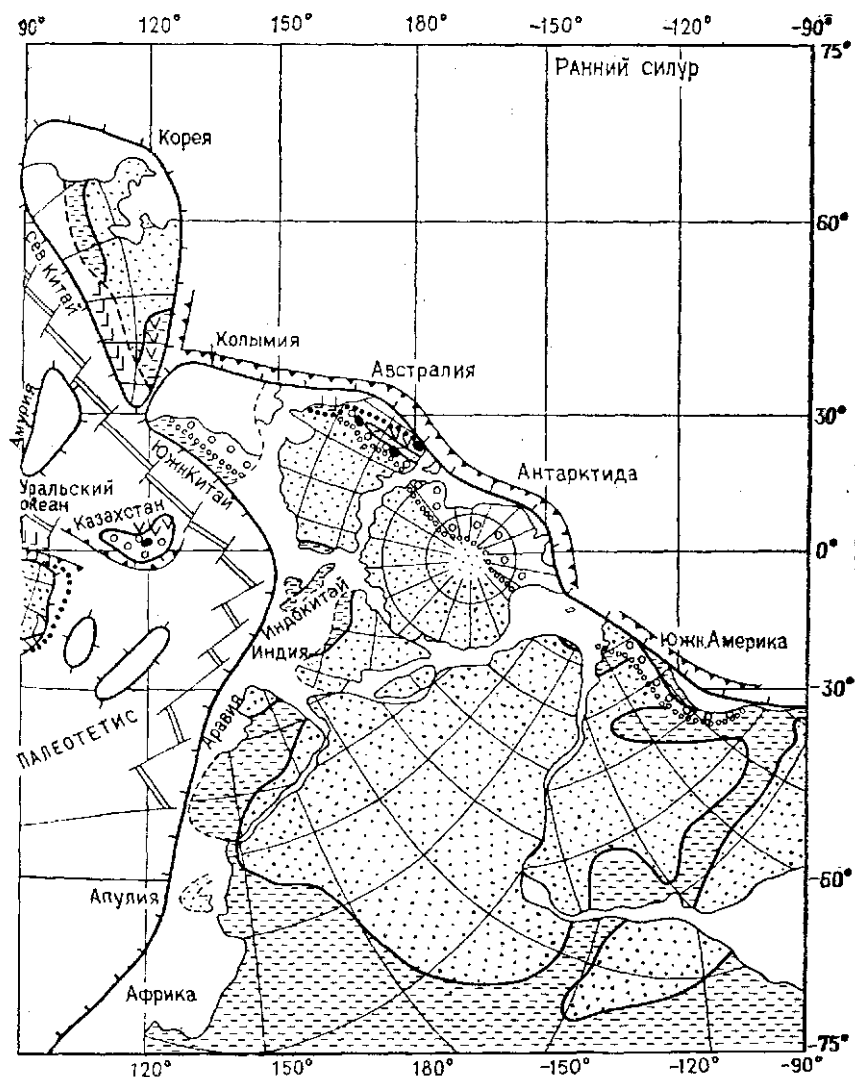
Меркатора с центром 0° с. ш. и 90° в. д.) (по В. Е. Ханну и К. Б. Сеславинско- см, на рис. 9.4
