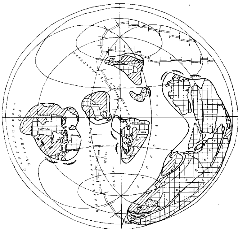
Рис. 10.3. Положение материков и океанов в раннем и среднем ордовике (по Л. П. Зонсшайну, с дополнениями). Условные обозначения см. на рис. 9.3
