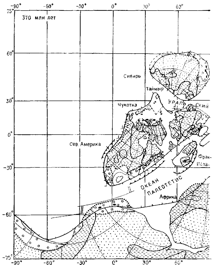
Рис. 12.4. Палеотектоническая реконструкция для позднего девона (проекция скому). Условные обозначения
