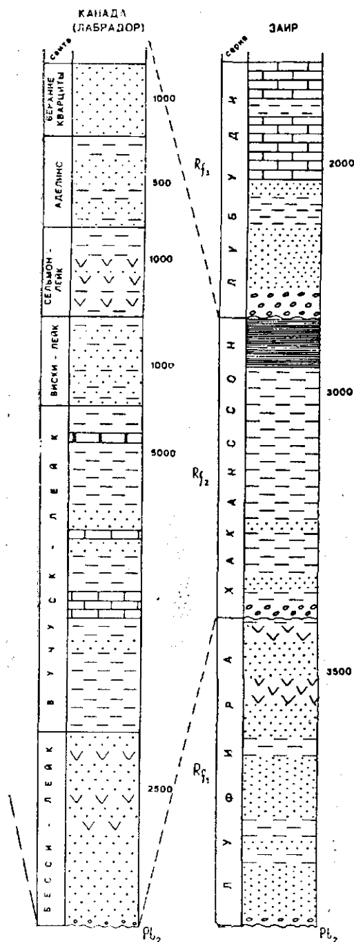
Рис. 7.1. Составление разрезов рифейской группы.
