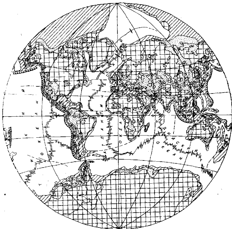
Рис. 19.3. Палеогеографическая реконструкция для плиоценовой эпохи (по В. Е. Ханну и А. Н. Балуховскому, с дополнениями). Условные обозначения см. на рис. 9.3
