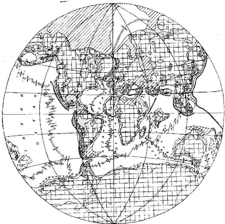
Рис. 18.4. Палеогеографическая реконструкция для палеоценовой эпохи (по В. Е. Ханну и А. Н. Балуховскому, с дополнениями). Условные обозначения см. на рис. 9.3
