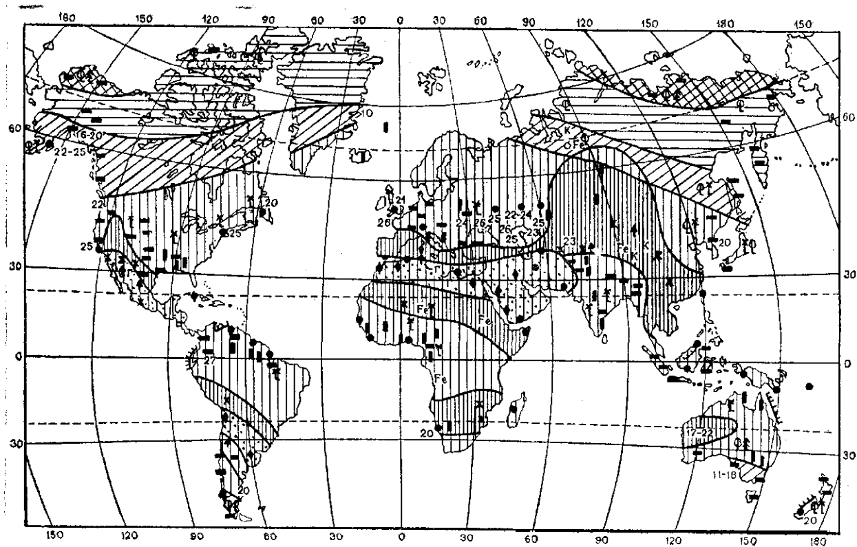
Рис. 18.7. Климатическая зональность материков в эоценовую эпоху (по Н. А. Ясаманову). Условные обозначения см. на рис. 9.5
