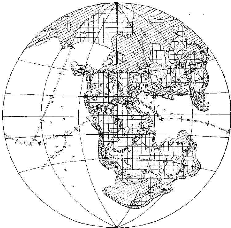
Рис. 16.4. Палеогеографическая реконструкция для среднеюрской эпохи (по В. Е. Ханну и А. Н. Балуховскому, с дополнениями и изменениями). Условные обозначения см. на рис. 9.3
