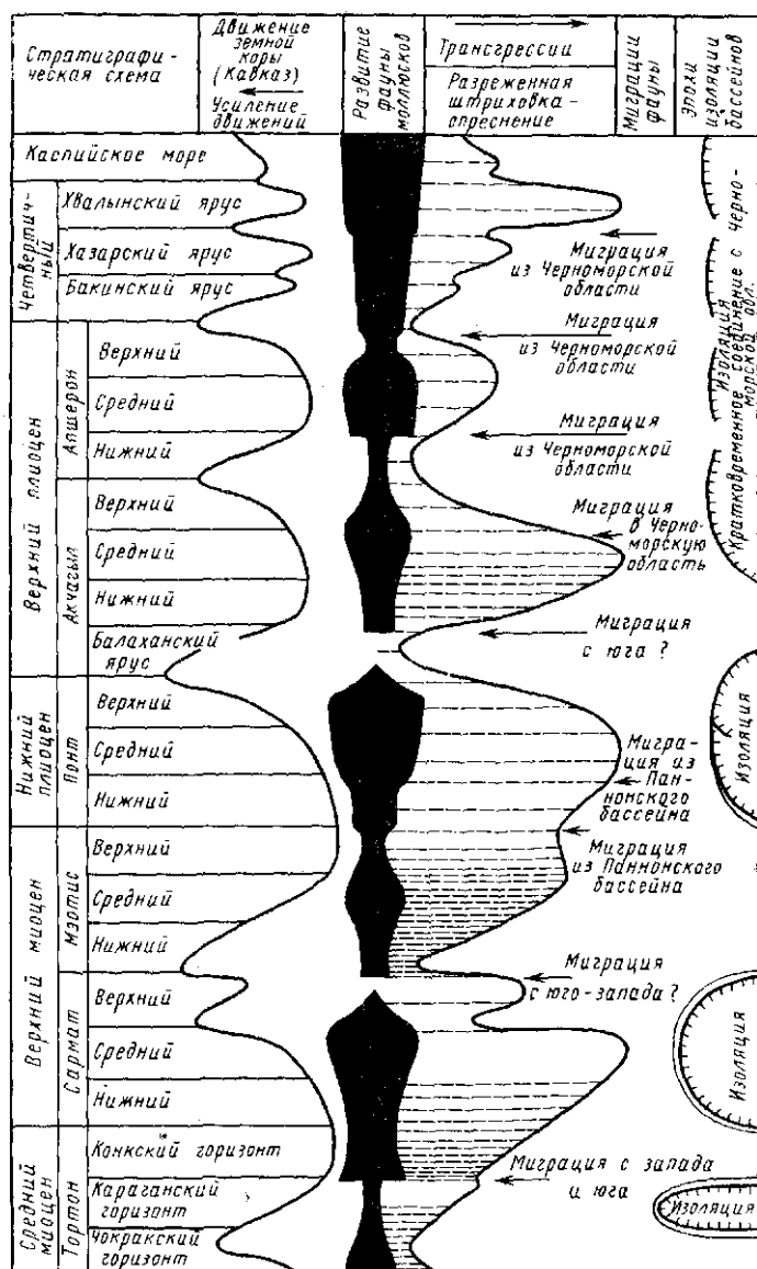
Рис. 2.6. Выделение циклов осадконакопления на примере геологического развития позднестретичных бассейнов Крымско-Кавказской области (по В. П. Колесникову)
