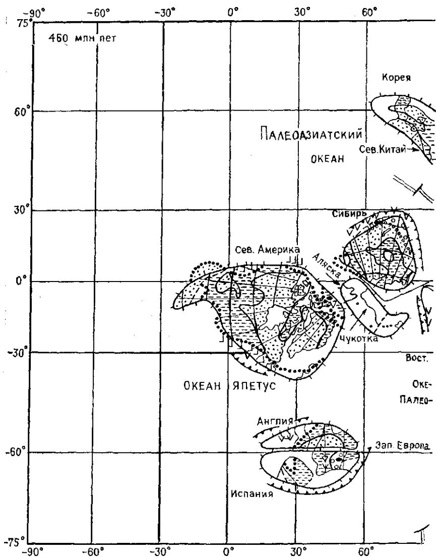
Рис. 10.6. Палеотектоническая реконструкция для среднего ордовика (проскния му). Условные обозначения
