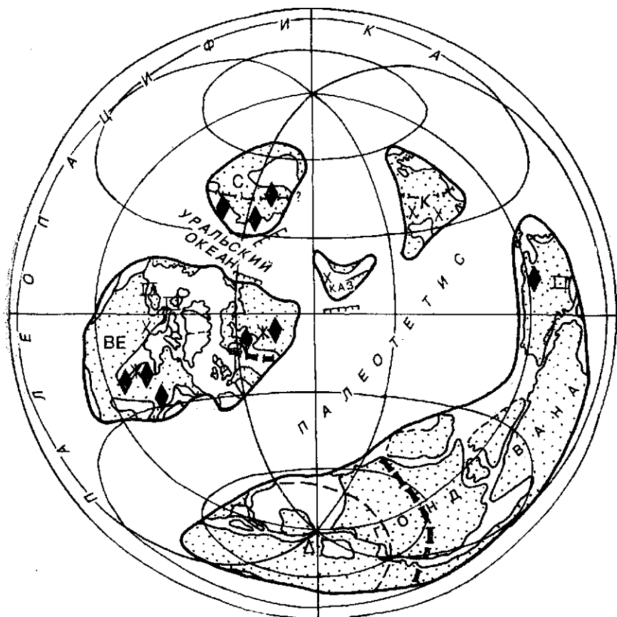
Рис. 11.5. Климатическая зональность силурийского периода на палинстратической основе. Условные обозначения см. на рис. 9.6
