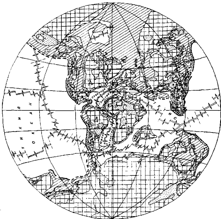
Рис. 17.4. Палеогеографическая реконструкция для раннего мела (по В. Е. Хан-ну и А. Н. Балуховскому, с дополнениями). Условные обозначения см. на рис. 9.3
