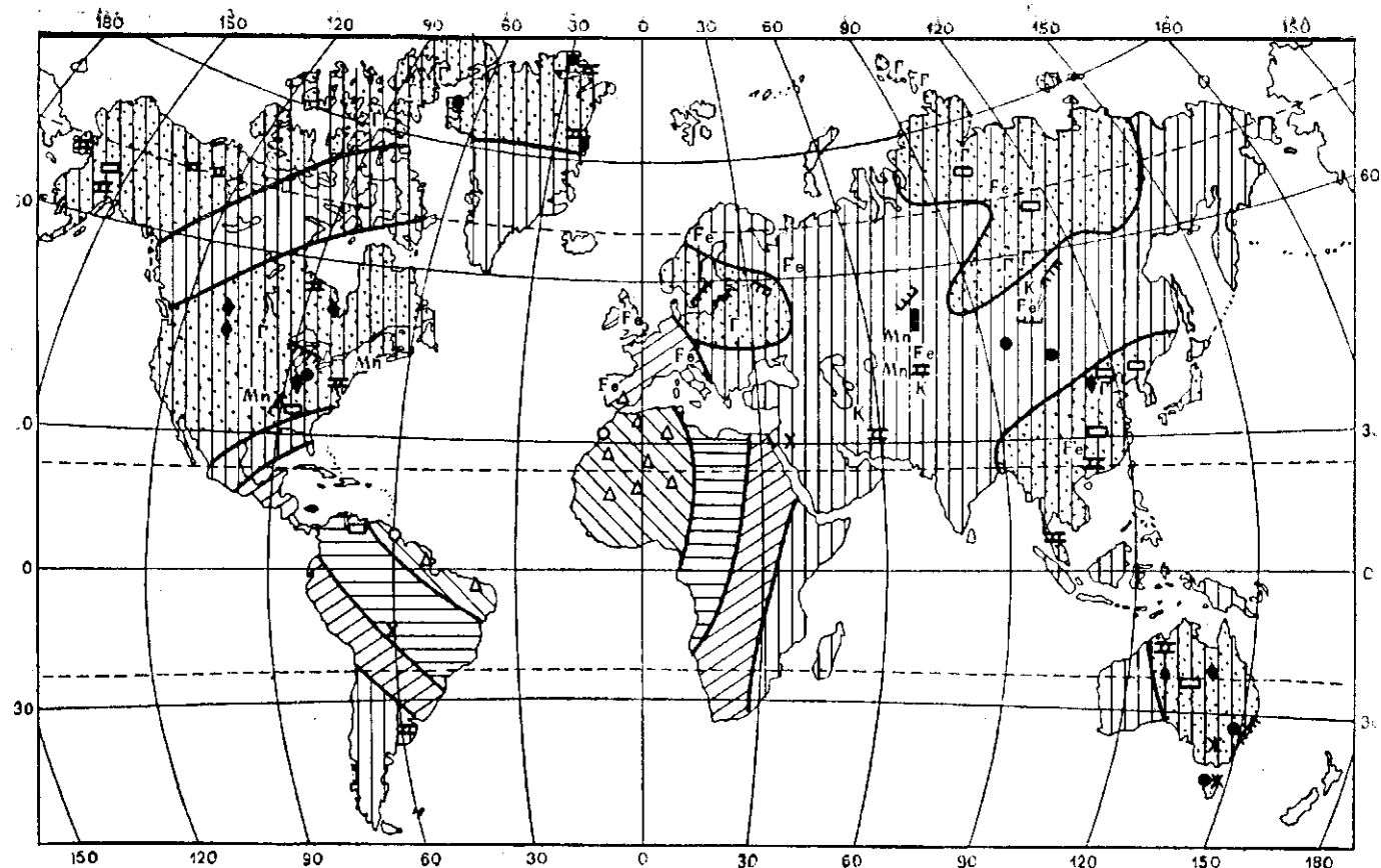
Рис. 10.7. Климатическая зональность материков в ордовикском периоде (по П. А. Ясаманову). Условные обозначения см. на рис. 9.5
