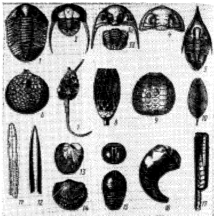
Рис. 10.2. Характерные представители ордовикских организмов. Трилобиты: 1 — Asaphus ; 2 — Onnia ; 3a и 3b — Chasmops ; 4 — Pterygomeridus ; 5 — Megalaspis . Иголкожие: 6 — Echinospaerites ; 7 — Pleurocystis ; 8 — Cyathocrinus ; 9 — Bothrioidaris . Граптолиты: 10 — Phyllograptus ; 11 — Didymograptus ; 12 — Diplograptus . Брахиоподы: 13 — Porambonites ; 14 — Orthis . Наутилоидеи: 15 — Gomphoceras ; 16 — Cyrtoceras ; 17 — Endoceras .
