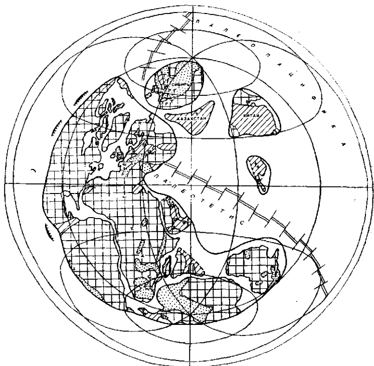
Рис. 14.4. Положение материков и океанов в поздней перми (по Л. П. Зоненшайну, с дополнениями). Условные обозначения см. на рис. 9.4
