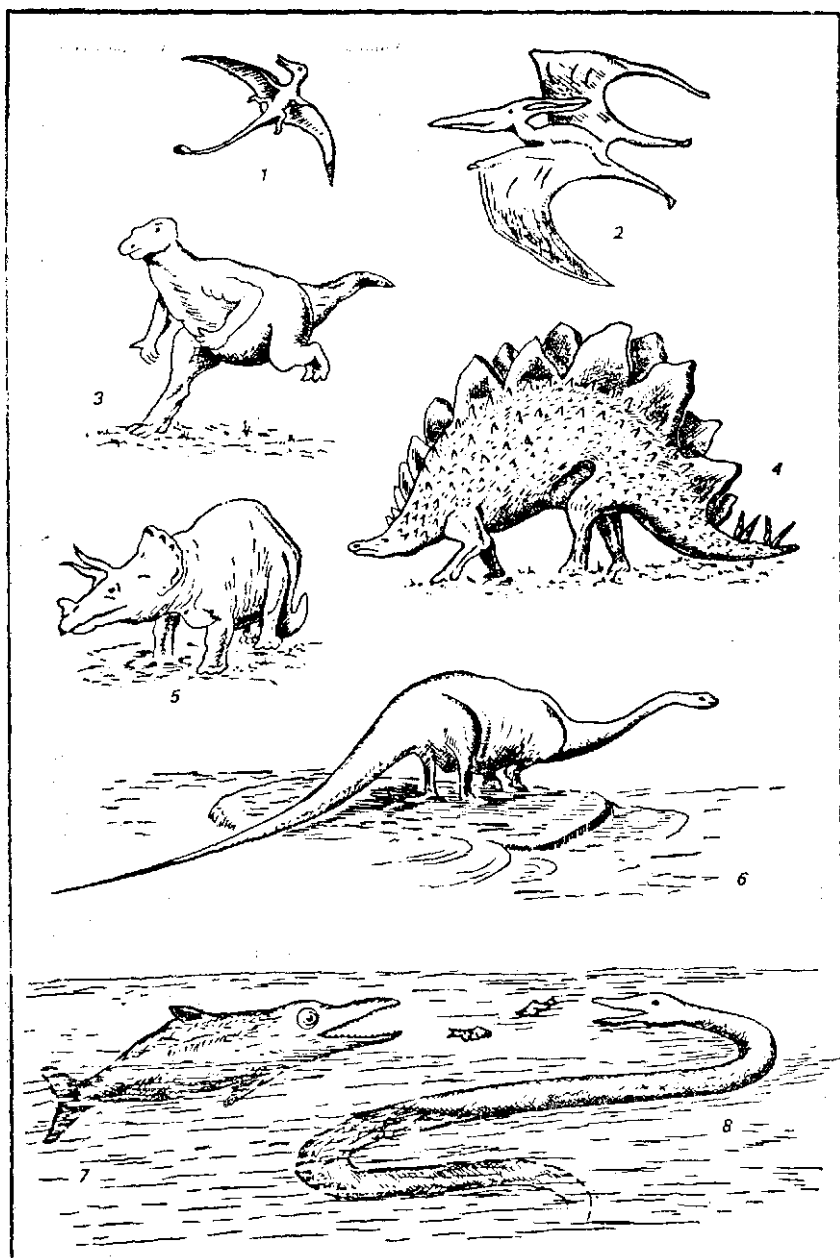
Рис. 17.3. Характерные представители мезозойских пресмыкающихся: 1 — Rhamphogynchus ( J_3 ); 2 — Pteranodon ( K_2 ); 3 — Iguanodon ( K_1 ); 4 — Stegosaurus ( J_3 — K_1 ); 5 — Triceratops ( K_2 ); 6 — Diplodocus ( J_3 ); 7 — Ichthyosaurus ( J_1 ); 8 — Mososaurus ( K_2 )
