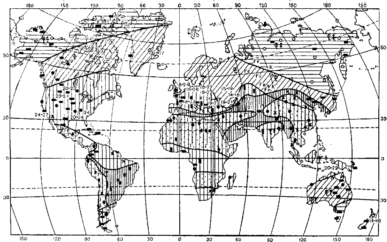
Рис. 17.7. Климатическая зональность материков в позднемеловую эпоху (по Н. А. Ясаманову). Условные обозначения см. на рис. 9.5
