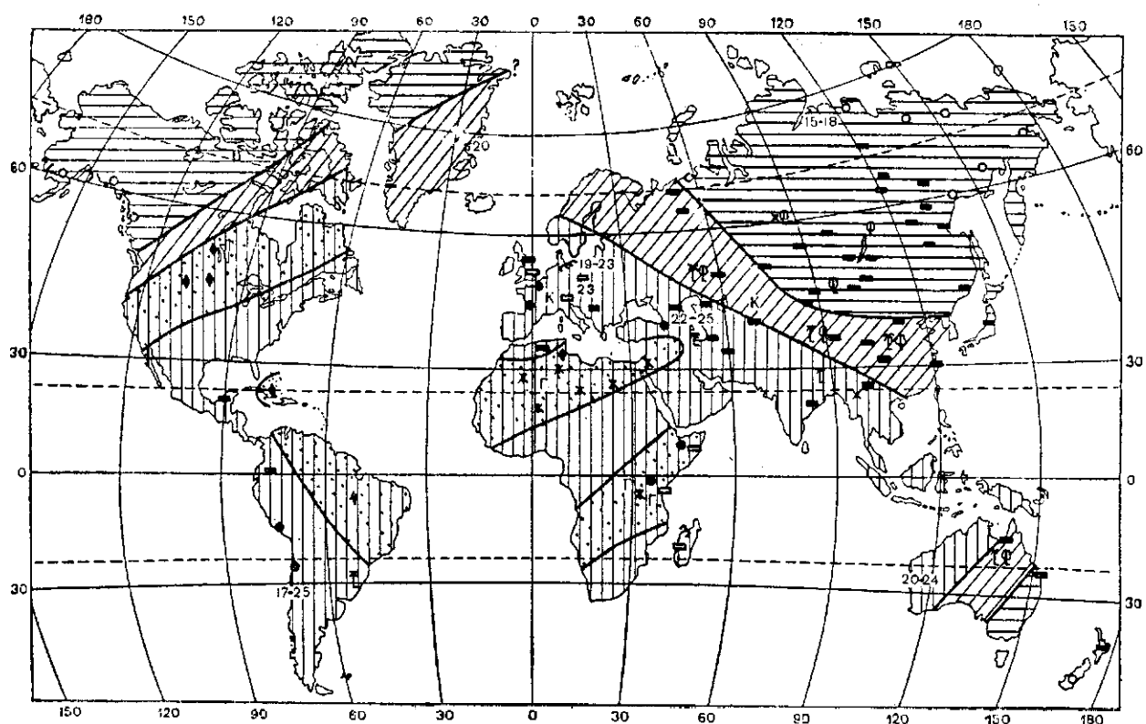
Рис. 16.7. Климатическая зональность в среднеюрскую эпоху (по Ц. А. Ясаманову). Условные обозначения см. на рис. 9.5
