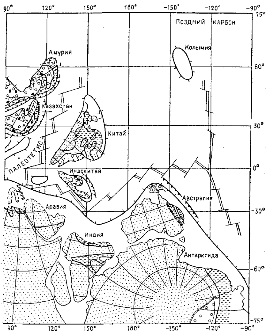
Меркатора с центром 0^{\circ} с. ш. и 90^{\circ} в. д.) (по В. Е. Хаину и К. Б. Сеславин- см. на рис. 9.4
