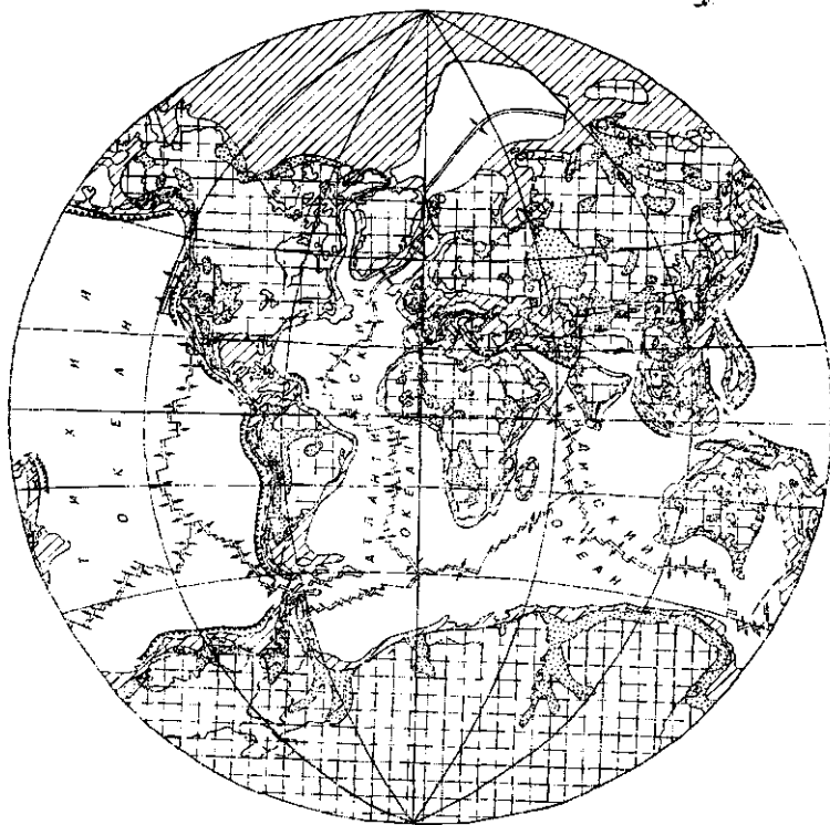
Рис. 18.6. Палеогеографическая реконструкция для олигоценовой эпохи (по В. Е. Ханну и А. И. Балухопскому). Условные обозначения см. на рис. 9.3
