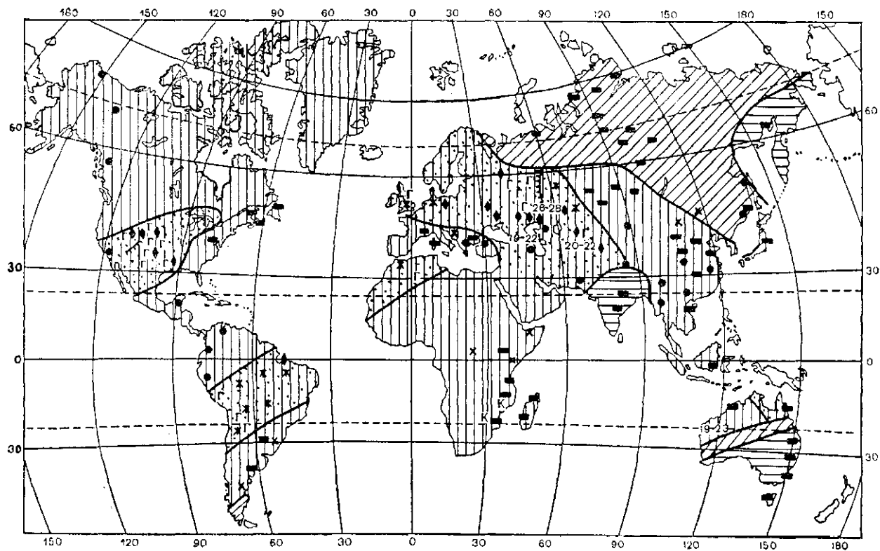
Рис. 14.6. Климатическая зональность материков в ранней перми (по Н. А. Ясмакову). Условные обозначения см. на рис. 9.5
