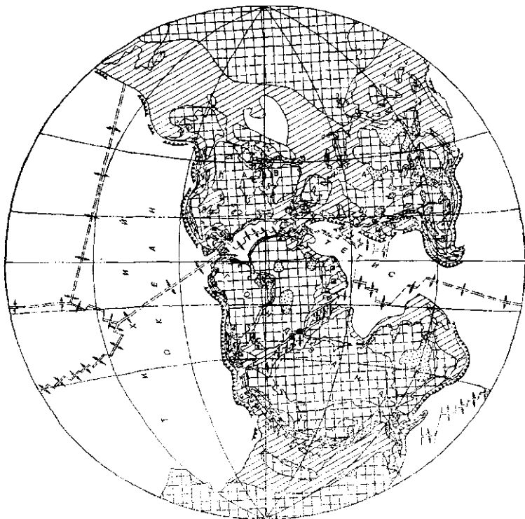
Рис. 16.5. Палеогеографическая реконструкция для позднеюрской эпохи (по В. Е. Ханну и А. Н. Балуховскому, с дополнениями и изменениями). Условные обозначения см. на рис. 9.3
