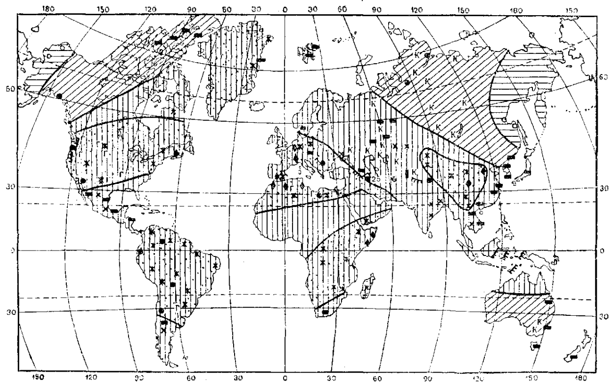
Рис. 15.4. Климатическая зональность материков в позднем триасе (по П. А. Ясаманову). Условные обозначения см. на рис. 9.5
