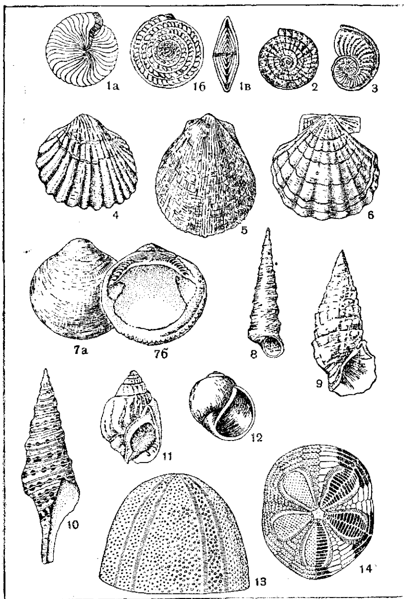
Рис. 18.2. Характерные ископаемые остатки палеогеновых организмов. Простейшие: 1а, 1б, 1в — Nummulites (P 2 ); 2 — Assilina (P 1-2 ); 3 — Operculina (K 2 —Q). Двустворчатые моллюски: 4 — Cardium (P—Q); 5 — Spondylus (KZ); 6 — Chlamys (T—Q); 7 — Glycymeris (KZ). Гастропоиды: 8 — Turritella (K—Q); 9 — Cerithium (K 2 —Q); 10 — Pleurotoma (P—Q); 11 — Nassarius (P 2 —Q); 12 — Natica (P—Q). Морские ежи: 13 — Conoclypeus (P 2 —N 1 ); 14 — Clypeaster (K 2 —Q)
