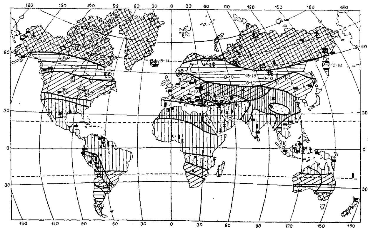
Рис. 19.5. Климатическая зональность материков в плистоценовую эпоху (по Н. А. Ясаманову). Условные обозначения см. на рис. 9.5
