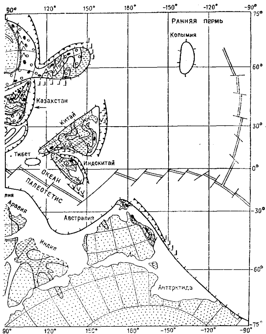
Меркатора с центром 0° с. ш. и 90° в. д.) (по В. Е. Хайну и К. Б. Сеславич-см. на рис. 9.4
