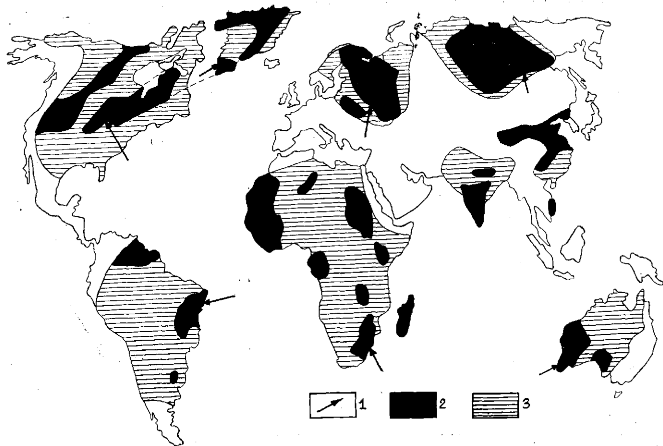
Рис. 5.1. Архейские протоплатформы и раннепротерозойские подвижные пояса в составе фундамента древних платформ (по В. Е. Хаину): 1 — стрелки показывают местонахождение «серых гнейсов» — древнейшей континентальной коры; 2 — архейские протоплатформы; 3 — раннепротерозойские подвижные пояса
