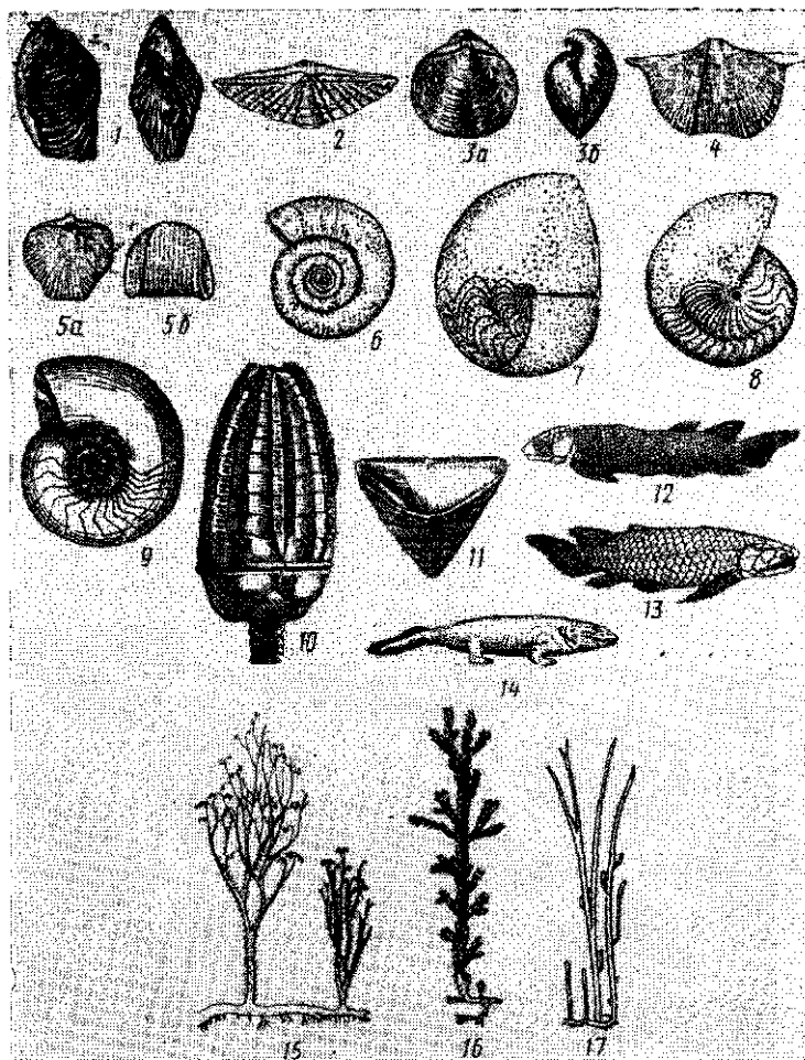
Рис. 12.1. Характерные представители девонских организмов: Брахиоподы: 1 — Karpinskia; 2 — Euryspirifer; 3a и 3б — Stringocephalus; 4 — Cyrtospirifer; 5a и 5б — Hypothyridina. Клименны: 6 — Cluymenia. Агониатиты: 7 — Timanites. Гониатиты: 8 — Tornoceras; 9 — Anarcestes. Кривоногие: 10 — Cypressocrinus. Кораллы: 11 — Calceola. Двоякодышащая рыба: 12 — Dipterus. Кистеперая рыба: 13 — Holoptychius. Земноводные: 14 — Ichthyostega. Риниофиты: 15 — Psilophyton; 16 — Asteroxylon; 17 — Rhynia
