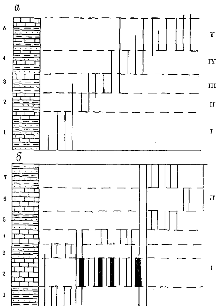
Рис. 2.3. Выделение разновозрастных палеонтологических комплексов. В однообразной толще a выделяют 5 палеонтологических комплексов. В толще б 7 пачек имеют собственный набор окаменелостей. Имеются повторения в пачках 1 и 3, 2 и 4, 5 и 7, связанные близостью фаций. В разрезе присутствуют 2 палеонтологических комплекса. I, II и I—V — палеонтологические сообщества
