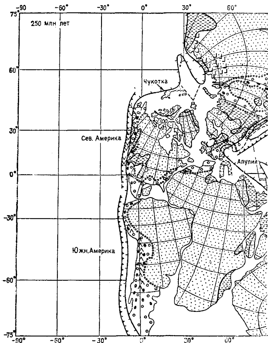
Рис. 14.5. Палеотектоническая реконструкция для поздней перми (проекции му). Условные обозначения
