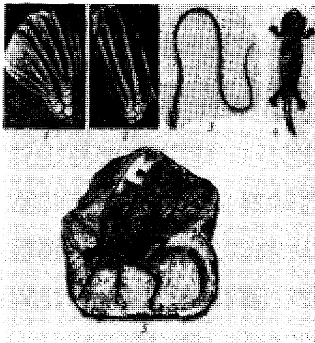
Рис. 13.3. Некоторые организмы каменноугольного периода. Морские лилии: 1 — Poteriocrinus multiplex , 2 — Cromocrinus ; панцирноголовые земноводные: 3 — Dolichosoma , 4 — Scineosaurus , 5 — Protophasma dumasii — гигантское насекомое карбона
