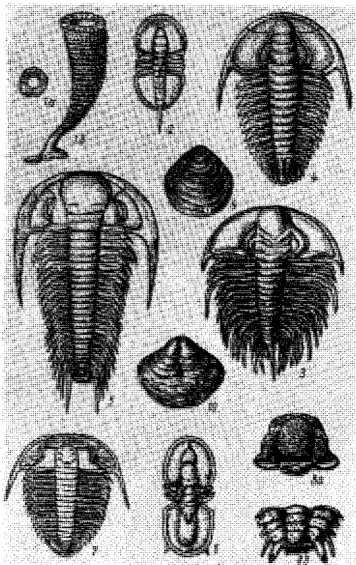
Рис. 9.2. Характерные представители кембрийских организмов: 1а, 1б — археоциаты (кембрий); 2—8 — трилобиты: 2 — Pagefia ( \epsilon_1 - \epsilon_2 ), 3 — Olenellus ( \epsilon_1 ), 4 — Redlichia ( \epsilon_1 ), 5 — Paradoxides ( \epsilon_2 ), 6 — Agnostus ( \epsilon_3 ), 7 — Olenus ( \epsilon_3 ), 8а, 8б — Dorypyge ( \epsilon_2 ); 9—10 — брахиоподы: 9 — Obolus ( \epsilon_2 - O_1 ), 10 — Kutorgina ( \epsilon_1 - \epsilon_2 )
