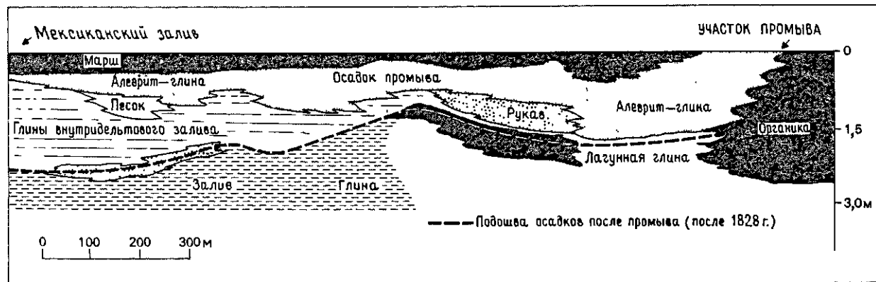
Рис. 6.7. Развитие субдельты в бухте Уэст-Бей, дельта Миссисипи, и ее фациальная модель [892]. а — условия открытого залива сразу после образования промоины;
