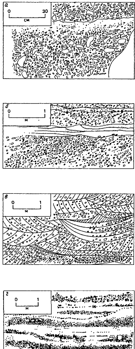
Рис. 3.32. Четыре конгломератовые фации, выделяемые в древнем красном песчанике аллювиальных конусов выноса, Ферт-оф-Клайд, Шотландия. А — параконгломераты с базальным цементом, интерпретируемые как отложения грязевых потоков; Б—Г — ортоконгломераты: Б — с прослоями мелкозернистых отложений и интерпретируемые как осадки плоскостного смыва, В и Г — отдельные примеры русловых речных отложений [253].
