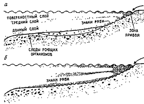
Рис. 9.16. Структура сезонной седиментации на континентальном шельфе Орегона. Турбидные слои показаны точками [1428]. Транспортировка турбидного слоя и образование знаков ряби происходят в течение зимы за счет высокого привноса осадка береговыми потоками и длительного периода образования волновых знаков ряби на дне в водах глубиной до 125 м. а — лето, низкий привнос осадка; б — зима, высокий привнос осадка.
