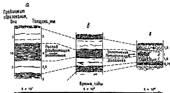
Рис.8.9. Схематическая диаграмма, иллюстрирующая возможную последовательность уплотнения нормальных накоплений водорослевых матов и их вероятный ископаемый аналог. а — разрез современного литорального водорослевого мата; б — разрез строматолита себхи; в — древний строматолит со слоистостью миллиметрового масштаба (d — микрит/микроспарит, обычно доломит, с — почти без исключения кальцит [1858]).
