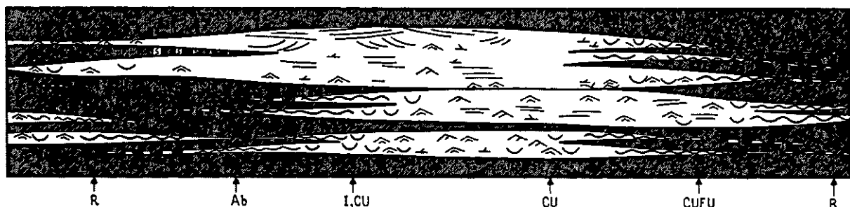
Рис. 9.52. Вертикальная последовательность отложений, связанных с тремя типами волновых песчаных баров: зарождающимися, погруженными и частично выступающими над водой. Основные типы переслаивания фаций: беспорядочное (R), резкое (Ab), прерывистое с
