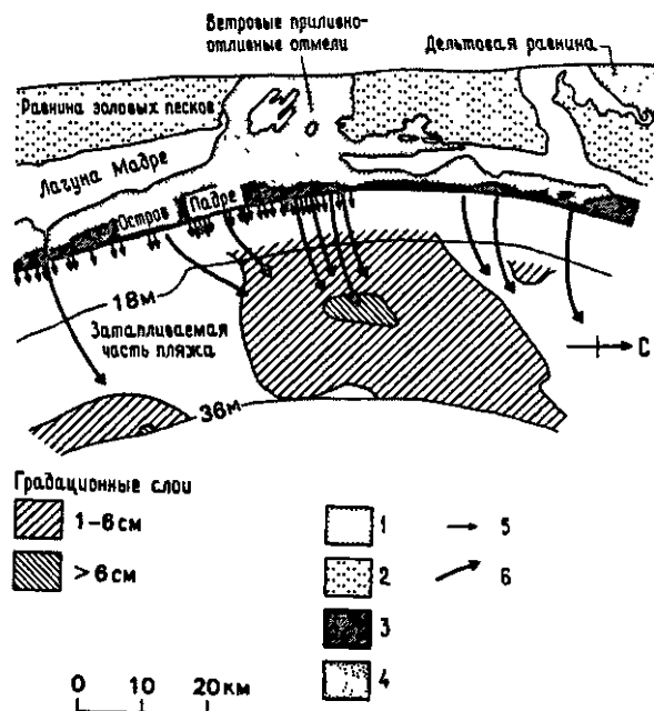
Рис. 7.8. Распределение слоев штормового происхождения, образованных ураганом Карла на пляже острова Падра, Мексиканский залив [1071, 1722]. Обстановки осадконакопления: 1 — ветровые приливо-отливные отмели; 2 — равнина золотых песков; 3 — дюны и окраинная низменная часть барьера, обращенная в сторону моря; 4 — дельтовая равнина; 5 — намывной канал; 6 — предполагаемые потоки.
