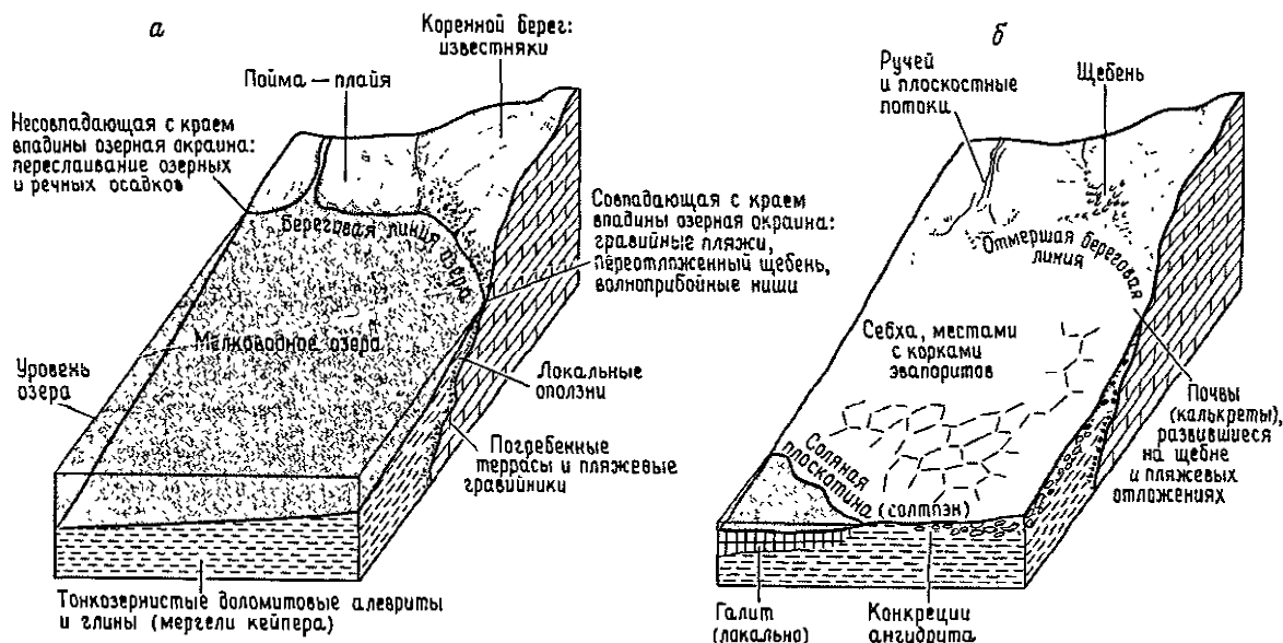
Рис. 4.31. Модель осадконакопления триасовых озерных отложений Южного Уэльса. а — стадия высокого стояния воды. На озерных окраинах, совпадающих с краем впадины, развиваются брекции прибрежных платформ и пляжей, на несовпадающих окраинах (края озера и края впадины) с озерными осадками переслаиваются речные отложения. Привнесенные реками але-
