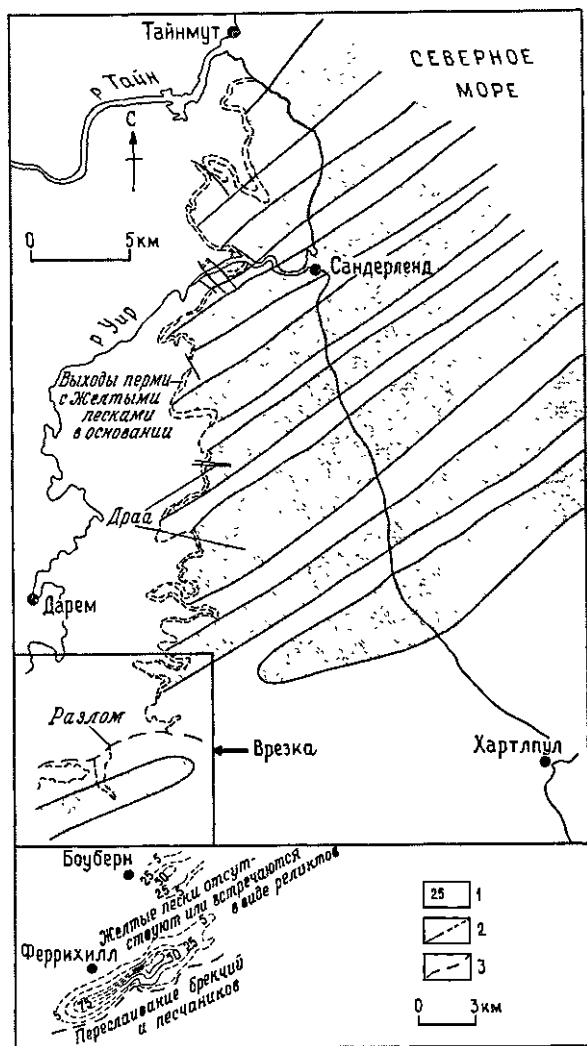
Рис. 5.11. Карта изопахит пермской песчаной залежи Желтых песков в форме крупной сейфовой драа, графство Дарем, Англия, и ее соотношение с соседними драа. Драа в основном погребены под более молодыми отложениями, и данные получены по результатам бурения и документации стволов шахт. Драа залегают на грубо плоской поверхности несогласия вестфальской угленосной свиты и ориентированы параллельно направлению палеоветра (мощности в футах) [2277, 2323]. 1 — мощность базальных отложений перми; 2 — изопахиты Желтых песков (установленные и предполагаемые); 3 — границы фаций песков и брекчий.
