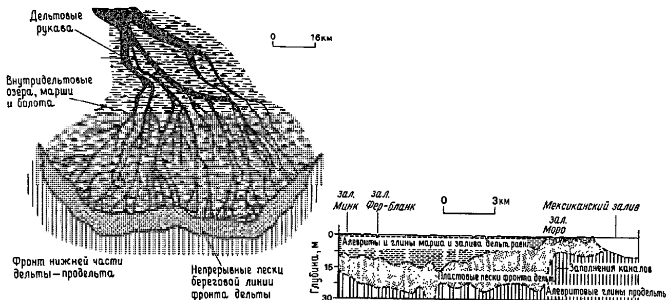
Рис. 6.36. Реконструкция отмершей мелководной лопасти Лафурш досовременной дельты Миссисипи и поперечный разрез через нее [798, 971].
