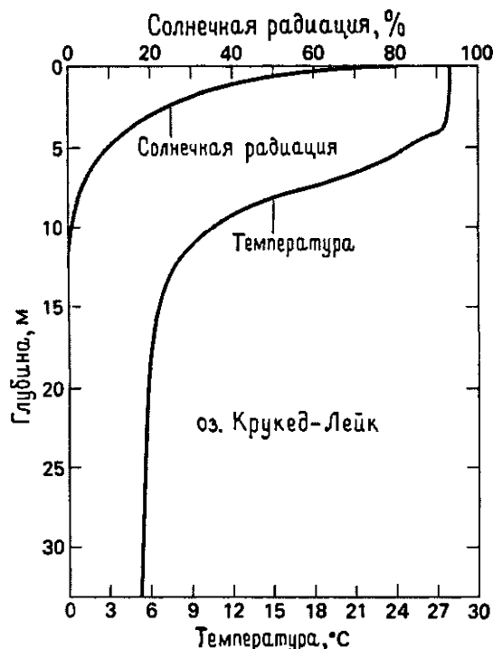
Рис. 4.3. Сравнение графиков проникающей солнечной радиации и температурного профиля озера Крукед-Лейк, шт. Индиана, США, на 18 июля 1964 г. [2595].
