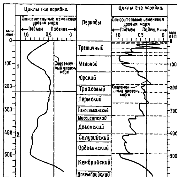
Рис. 2.12. Глобальные циклы относительных изменений уровня моря первого и второго порядка в фанерозое [2493].
