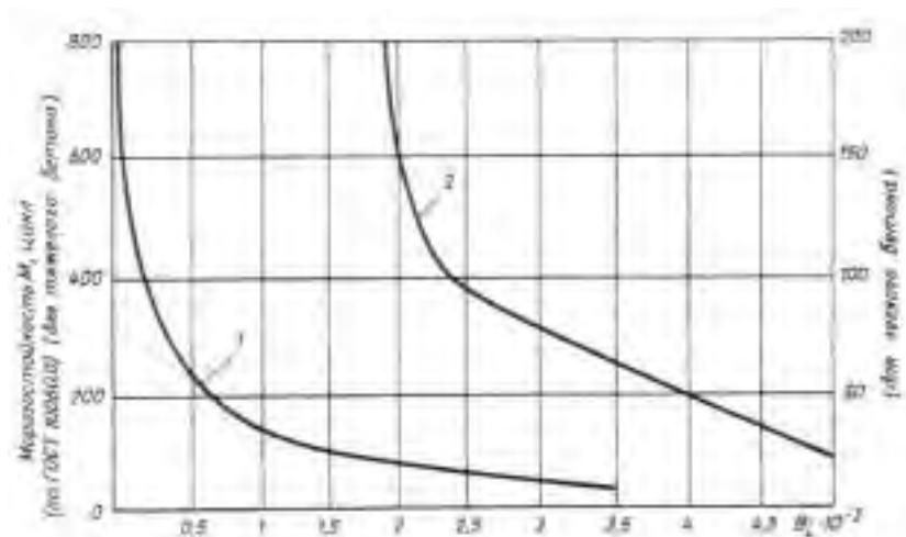
Рисунок 2 - График зависимости морозостойкости бетона от \theta_i - максимального относительного увеличения разности объемных деформаций бетонного и стандартного образцов при замораживании
