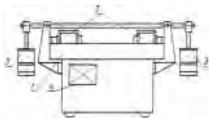
1 - истирающий диск; 2 - испытываемые образцы; 3 - нагружающее устройство; 4 - счетчик оборотов Черт. 1
