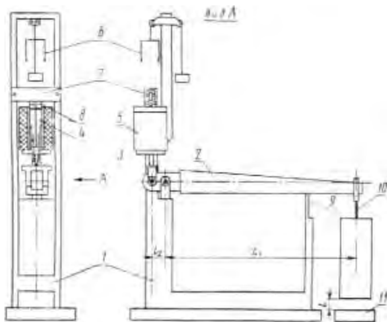
1 - металлическая рама; 2 - неравноплечий рычаг; 3 - опорный столик; 4 - образец; 5 - нагревательное устройство; 6 - приспособление для подъема нагревательного устройства; 7 - силовая балка; 8 - металлические оголовники; 9 - страховочная стойка; 10 - подвеска с грузами; 11 - страховочная опора.
