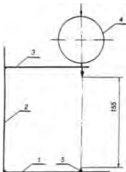
1 — основание; 2 — стойка; 3 — кронштейн; 4 — индикатор; 5 — шаровая опора
