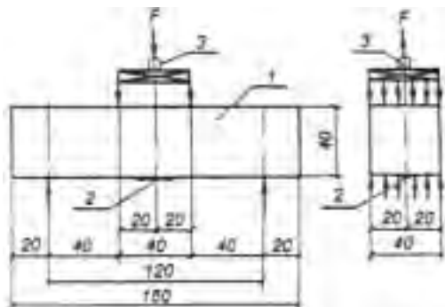
1 — опытный образец; 2 — тензорезистор базой 20 мм; 3 — электрический силоизмеритель
