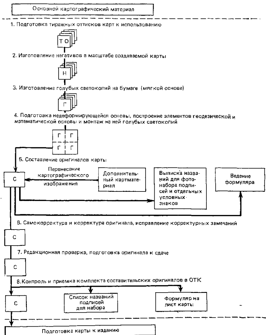
Рис. 67. Технологическая схема составления оригиналов топографических карт по одной голубой светокопии на непрозрачной (жесткой) основе
