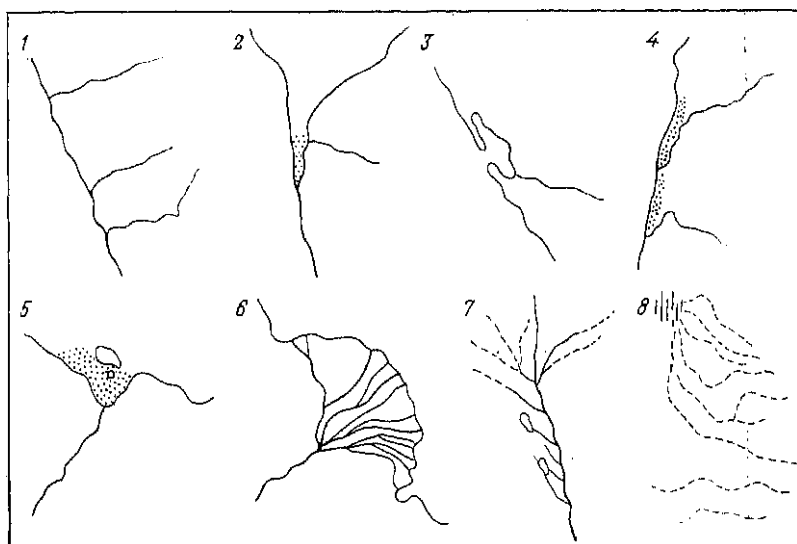
Рис. 53. Устья рек:
