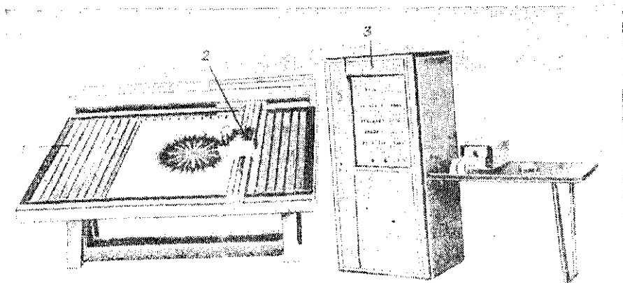
Рис. 43. Чертежный автомат Дигиграф (ЧССР)
