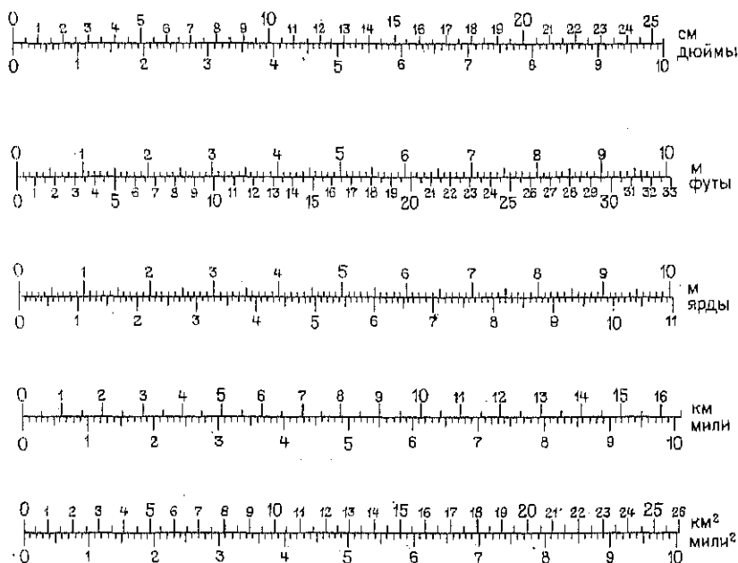
Рис. 19. Номограмма (двоенные шкалы) для перевода одних единиц измерения в другие
