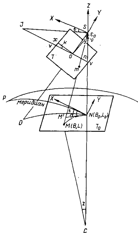
Рис. 79. Связь геодезических, сфероидических и прямоугольных координат точек поверхности эллипсоида и фотоснимков
