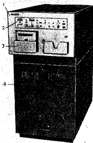
Рис. 22. Фотонаборная машина ФА-1000: 1 — фотонаборное устройство ФНУ; 2 — пульт управления и индикации; 3 — фотоот- сечивающее устройство; 4 — устройство управ- ления
