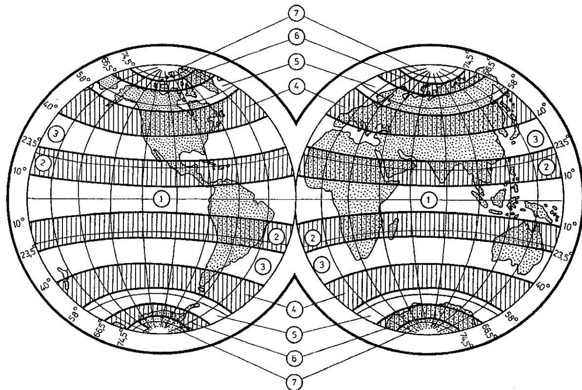
Рис. 8. Пояса освещенности Земли (Л. П. Шубаев, 1977):
