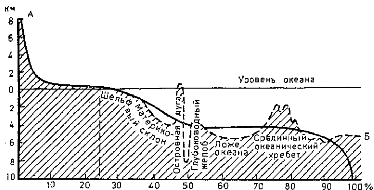
Рис. 11. Гипсографическая кривая Земли (А) и обобщенный профиль дна Океана (Б)
