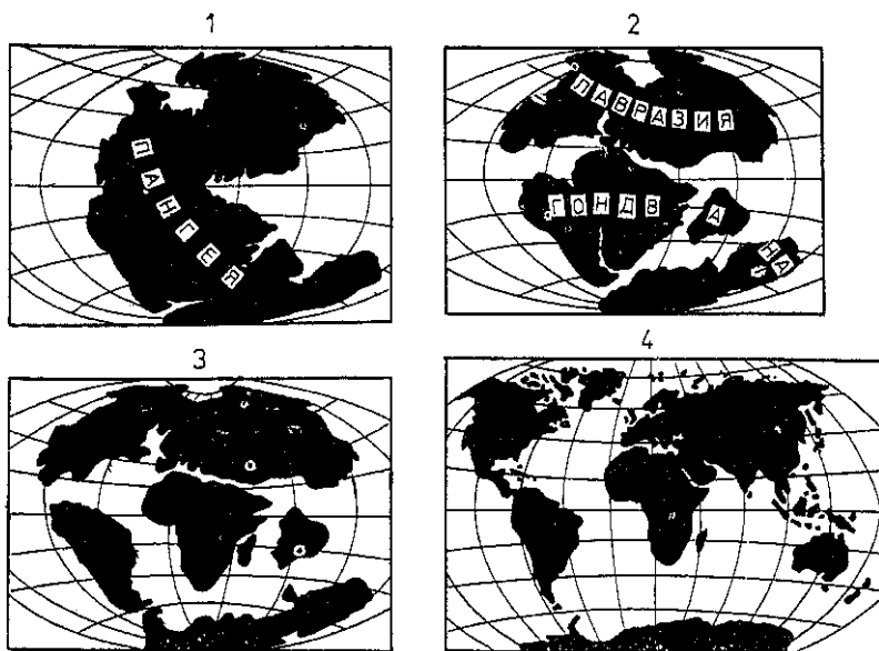
Рис. 20. Распад Пангеи и формирование современных материков (по Р. Дик и Дж. Холден, 1974):
