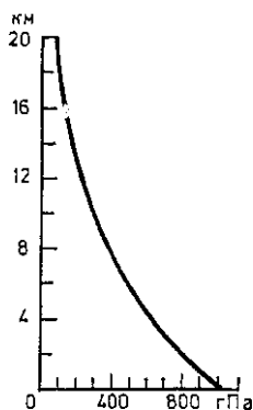
Рис. 22. Изменение атмосферного давления с высотой (по С. П. Хромову, 1933)
