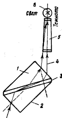
Рис. 52. Оптическая схема рефрактометра Аббе:
