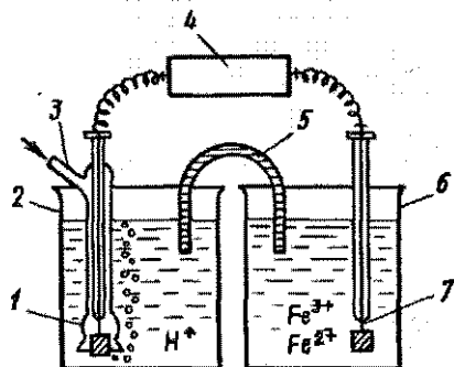
Рис. 17. Схема прибора для определения стандартного окислительно-восстановительного потенциала пары \text{Fe}^{3+}/\text{Fe}^{2+} :
