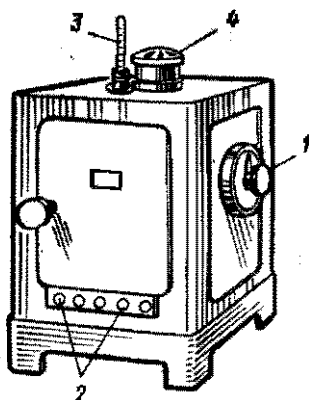
Рис. 29. Сушильный шкаф с электрическим обогревом:
