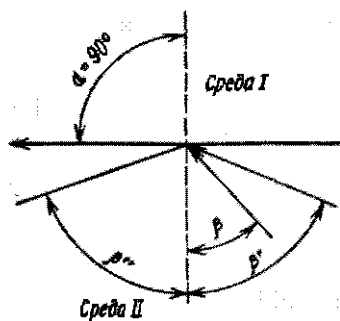
Рис. 51. Оптическая схема полного внутреннего отражения
