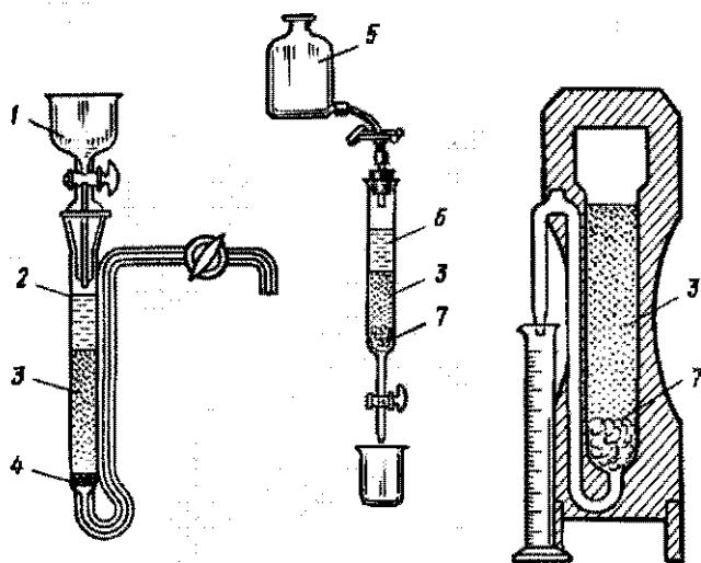
Рис. 39. Адсорбционные колонки:
