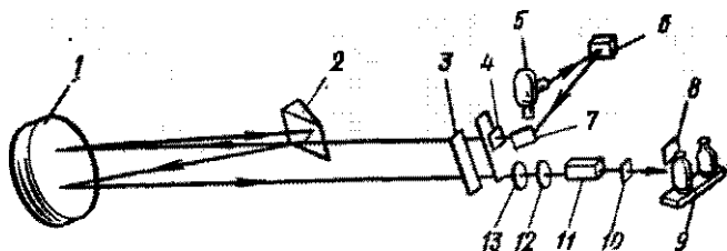
Рис. 43. Оптическая схема спектрофотометра СФ-4:
