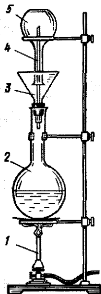
Рис. 25. Очистка колбы водяным паром:
