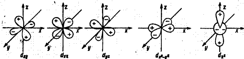
Рис. 3. d -Орбитали
