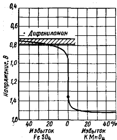
Рис. 38. Кривая титрования раствора \text{FeSO}_4 перманганатом (при [\text{H}^+] = 1 моль/л)
