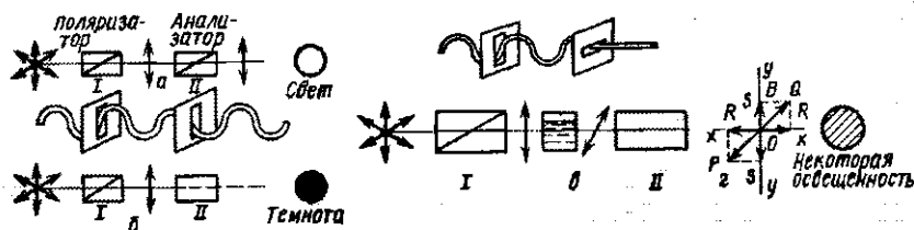
Рис. 46. Схема поляриметрического исследования
