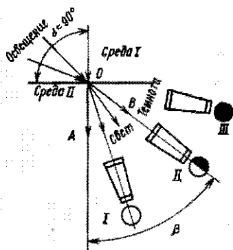
Рис. 50. Оптическая схема измерения предельного угла преломления
