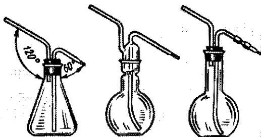
Рис. 27. Промывалки
