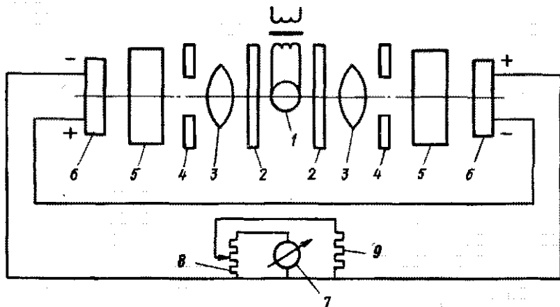
Рис. 42. Схема фотоколориметра ФЭК-М:
