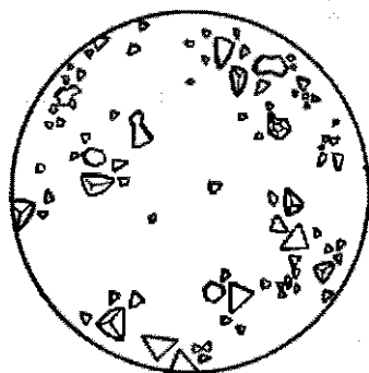
Рис. 15. Кристаллы \text{NaUO}_2(\text{CH}_3\text{COO})_3
