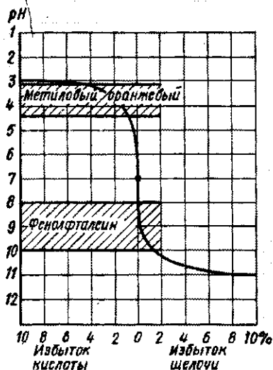
Рис. 36. Кривая титрования 0,1 М раствора \text{CH}_3\text{COOH} 0,1 М раствором \text{NaOH}
