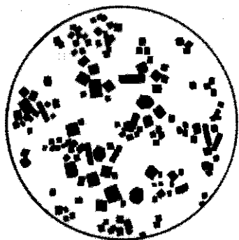
Рис. 14. Кристаллы K_2Pb[Cu(NO_2)_6]
