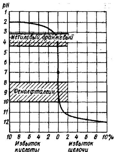
Рис. 35. Кривая титрования 0,01 М раствора \text{HCl} 0,01 М раствором \text{NaOH}
