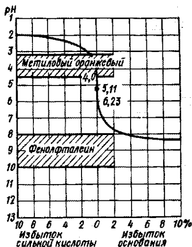
Рис. 37. Кривая титрования 0,1 М раствора аммиака 0,1 М раствором \text{HCl}
