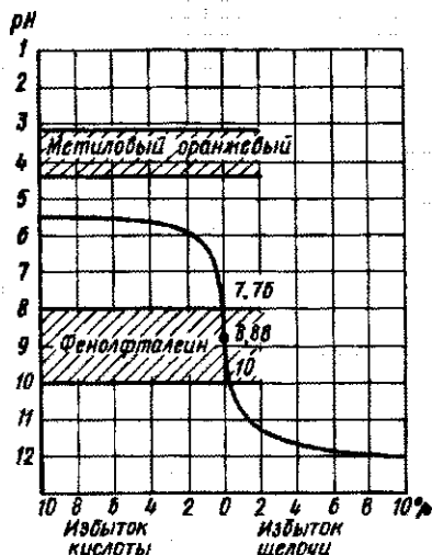
Рис. 34. Кривая титрования 0,1 М раствора \text{HCl} 0,1 М раствором \text{NaOH}
