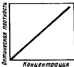
Рис. 40. Зависимость оптической плотности раствора от концентрации (градуировочная кривая)
