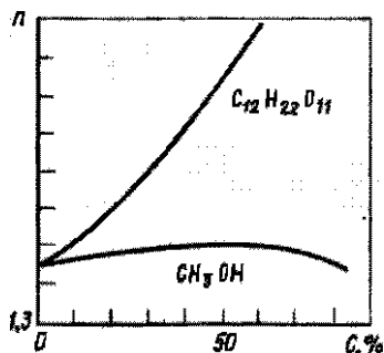
Рис. 48. Градуировочный график для рефрактометрических определений сахара C_{12}H_{22}O_{11} и метанола CH_3OH
