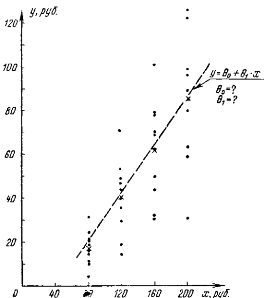
Рис. В.2. Графическое представление результатов обследования 40 семей по их среднему доходу ( x_i ) и среднему денежному сбережениям ( y_i )
