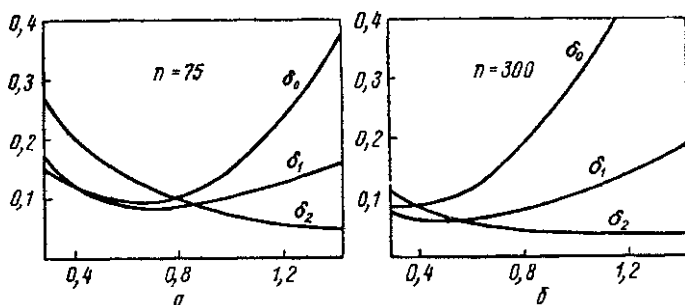
Рис. 10.1. Зависимость погрешности локальной параболлической аппроксимации от величины b для выборки объема: а) n=75 ; б) n=300
