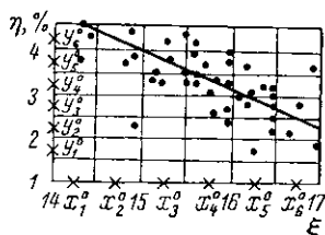
Рис. В.6. Графическое представление данных по связи вакуума в печи для обжига стекла ( \xi ) и процента брака в стекольном производстве ( \eta )
