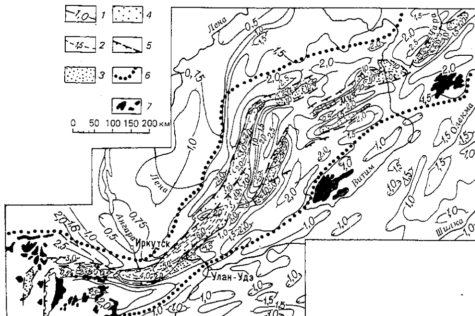
Рис. 41. Схема неотектонических деформаций Байкальского рифтового пояса (по материалам Ю. А. Зорина и др.): 1 — изогипсы позднемеловой — палеогеновой денудационной поверхности, деформированной новейшими движениями, км; 2 — изогипсы поверхности фундамента впадин, км; 3 — кайнозойские отложения во впадинах; 4 — то же, на дне Байкала; 5 — крупные кайнозойские разломы сбросового и сбросо-сдвигового типов; 6 — граница Байкальского рифтового пояса; 7 — неоген-четвертичные базальты
