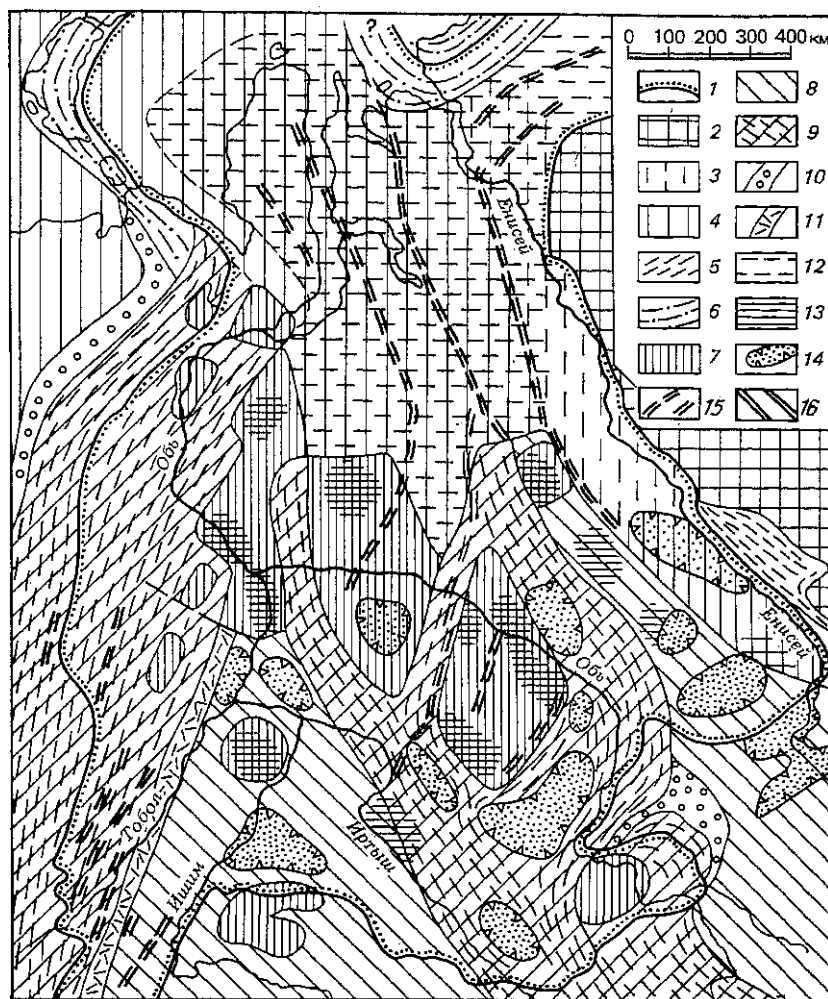
Рис. 55. Гипотетическая схема строения докембрийского основания и доплитных комплексов чехла Западно-Сибирской плиты (сост. с использованием данных М. Я. Рудкевича, 1986, и других авторов):
