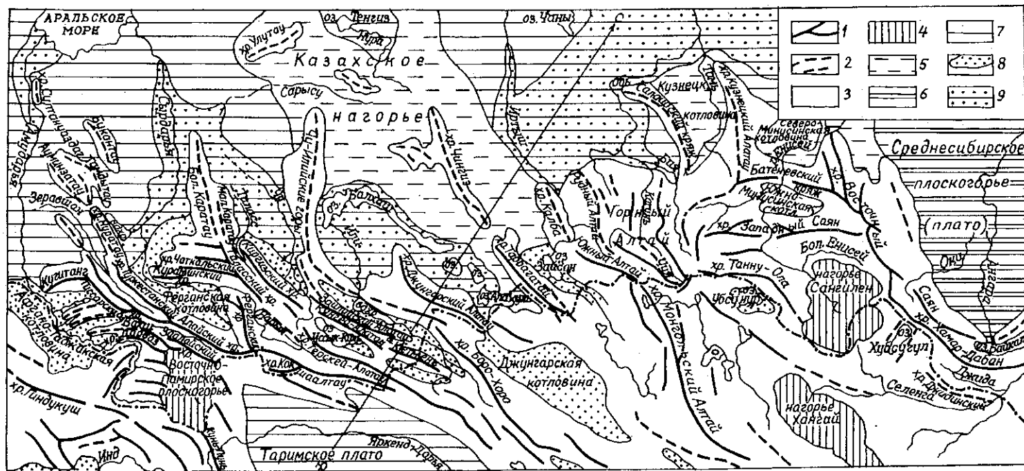
Рис. 50. Схема орографии и неотектоники Тянь-Шаньской, Алтае-Саянской областей и сопредельных территорий:
