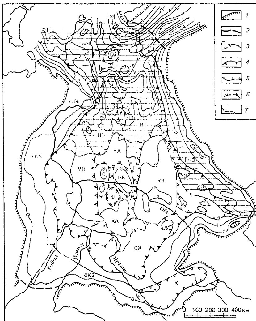
Рис. 56. Структурная схема и районирование чехла Западно-Сибирской плиты по подложке юрско-кайнозойского плитного комплекса (по И. И. Нестерову и др., 1984, с изменениями и дополнениями):
