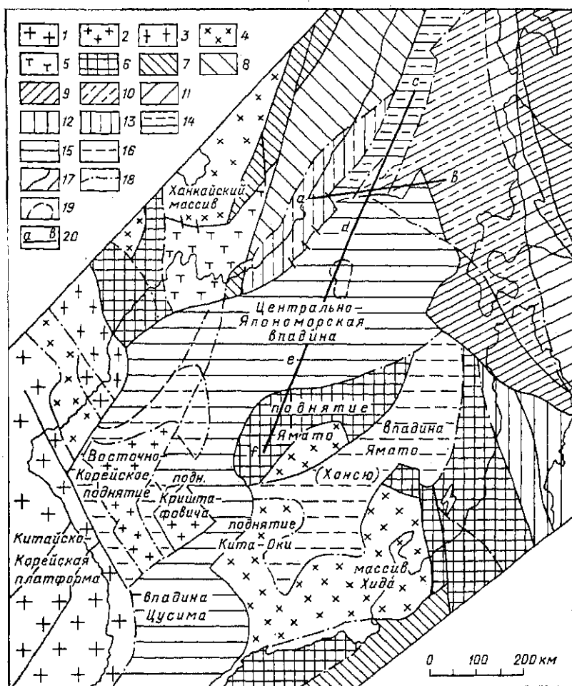
Рис. 90. Схема тектонического строения дна Японского моря и его обрамления (по И. И. Берсеневу и В. Л. Безверхнему, 1988, с изменениями).
