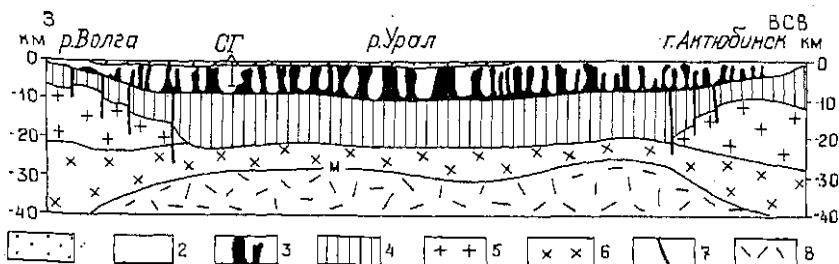
Рис. 7. Глубинный геолого-геофизический профиль через Прикаспийскую впадину. Из «Тектоники Европы» (1978).
