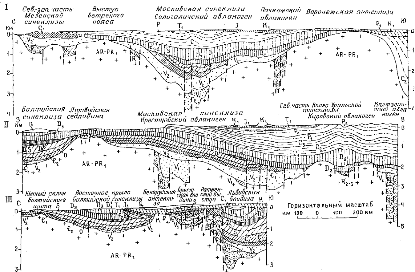
Рис. 4. Меридиональные (I—I и III—III) и широтный (II—II) геологические профили Русской плиты (по Н. С. Игolkной, с упрощениями). Положение профилей показано на рис. 3. Соотношение масштабов 1:100
