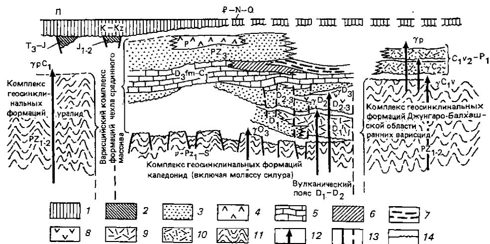
Рис. 49. Соотношения вариссийского комплекса формаций с каледонским в разных тектонических зонах Казахского нагорья (по О. А. Мазаровичу, 1976, с упрощениями и изменениями).
