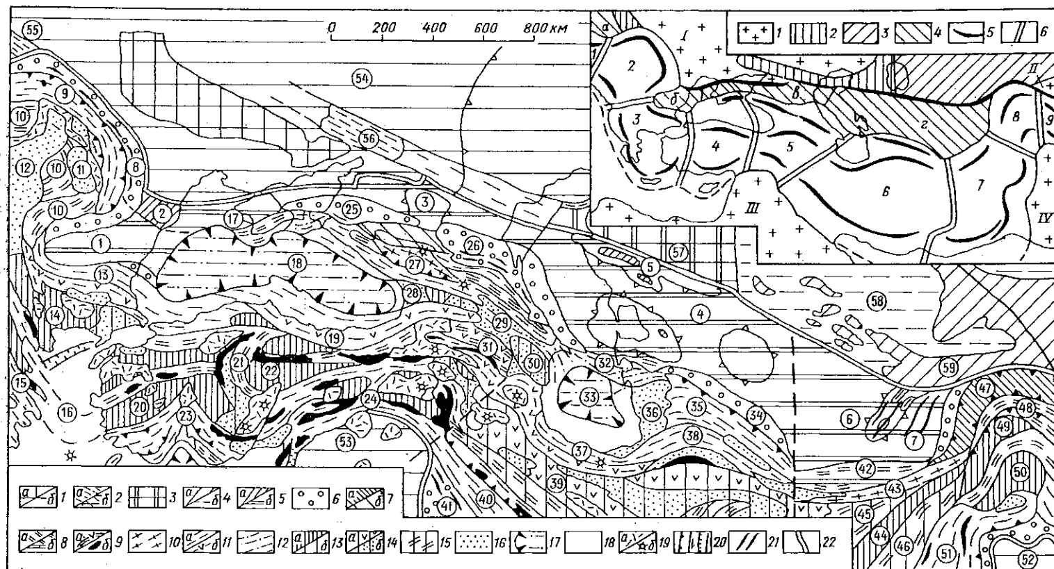
Рис. 62. Схема тектонического строения средней части Средиземноморского подвижного пояса:
