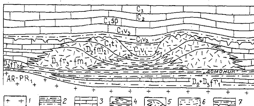
Рис. 15. Принципиальная схема строения депрессионных зон («некомпенсированных прогибов») Камско-Кинельской системы в поперечном субширотном разрезе.
