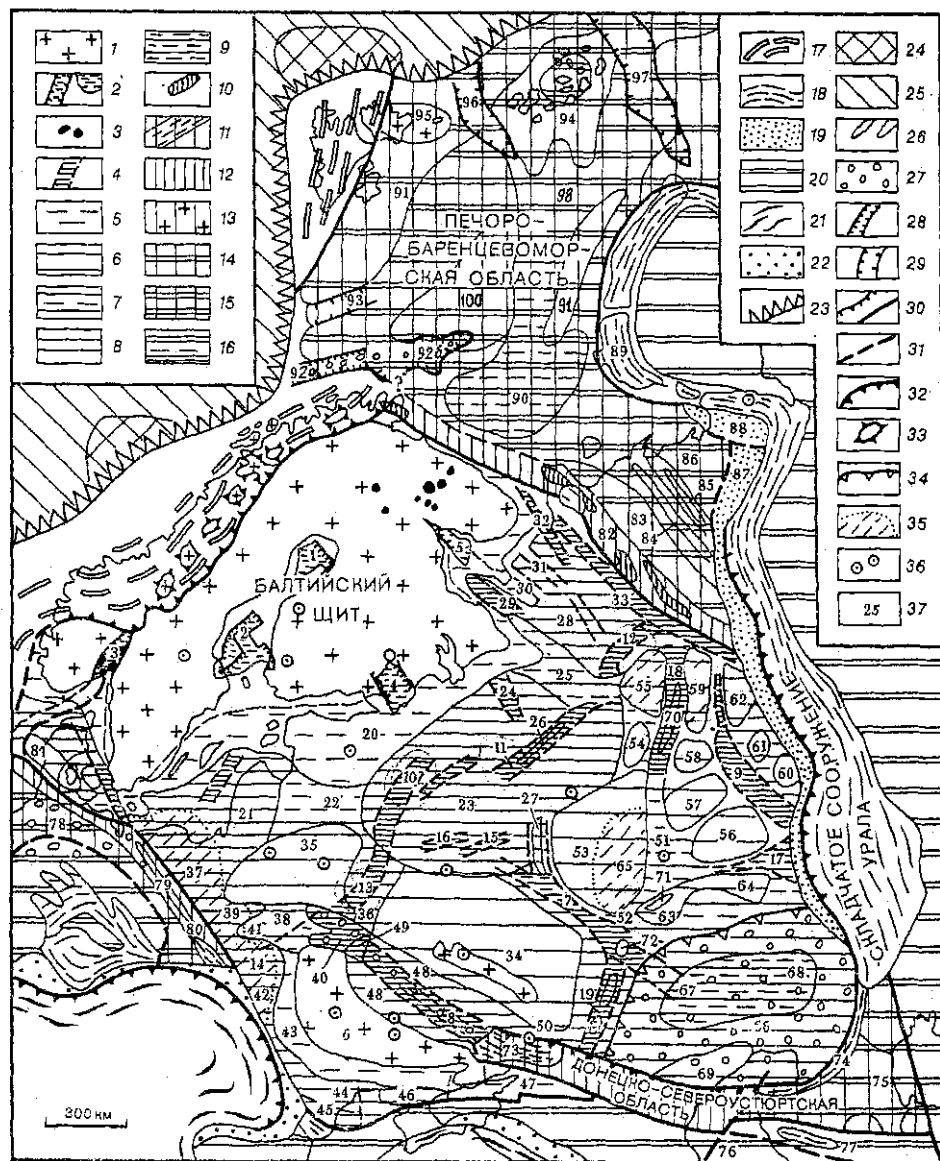
Рис. 2. Схема тектонического районирования Восточно-Европейской платформы и смежных метакратонных областей.
