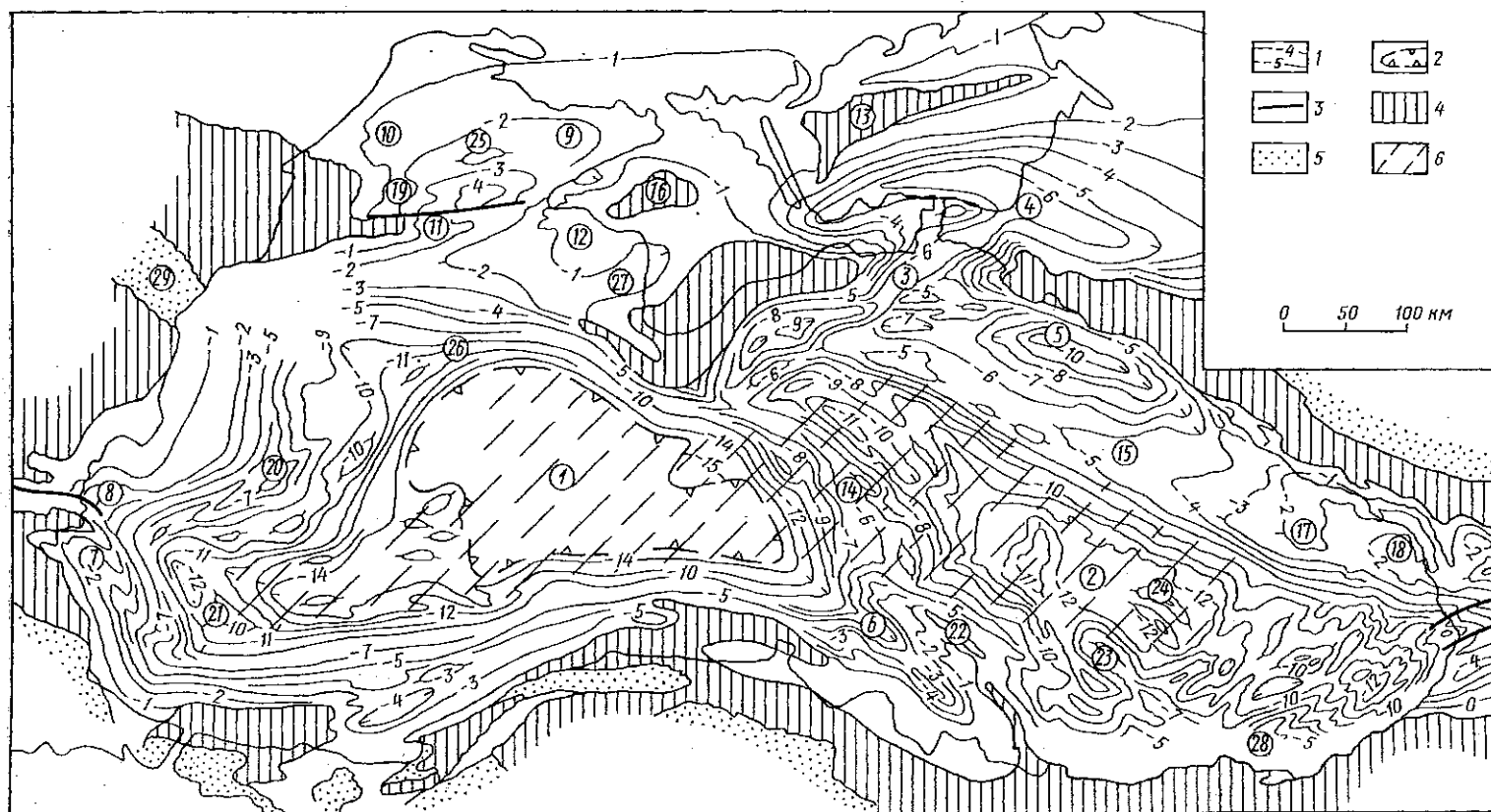
Рис. 71. Структурная карта Черного моря по поверхности мезозоя (отражающий горизонт III-N) (по Д. А. Туголесову и др., 1985) и область предполагаемого отсутствия геофизического «гранитного слоя», согласно альтернативным представлениям Ю. П. Непрочнова и других исследователей:
