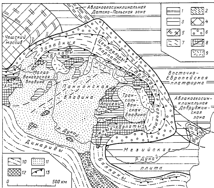
Рис. 66. Тектоническое положение и районирование Карпатской складчатой области: 1 — Восточно-Европейская древняя платформа; 2—3 — метаплатформенные области; 2 — авлакогесинклинальные складчатые зоны, 3 — плитный чехол; 4—13 — Средиземноморский подвижный пояс: 4—5 — Западно-Европейская палеозойская складчатая область; 4 — Чешский срединный массив, 5 — палеозойские складчатые зоны; 6—13 — области альпийской складчатости: 6 — Предкарпатский и Предальпийский краевые прогибы, 7 — Внешняя (флишевая) мегазона Карпат и Альп, 8 — Внутренняя мегазона Карпат и Альп: докембрий и палеозой (а), мезозой (б), 9 — неогеновые вулканические зоны на поверхности и под чехлом внутренних впадин, 10 — складчатые сооружения Балкан и Динарид, 11 — внутренние впадины, выполненные неогеном и антропогеном, 12 — выступы основания внутренних впадин, 13 — фронтальные линии крупных альпийских надвигов и покровов
