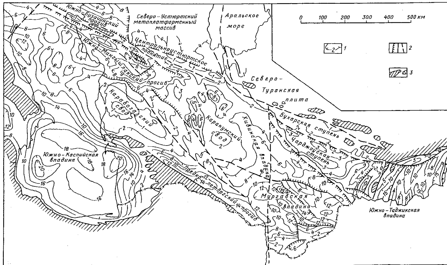
Рис. 65. Структурная схема подошвы верхнепалеозойско-мезокайнозойского чехла Южно-Туранской плиты и подошвы осадочной толщи дна Среднего и Южного Каспия (по картам, составленным под ред. В. В. Семеновича и др. и И. С. Грамберга):
