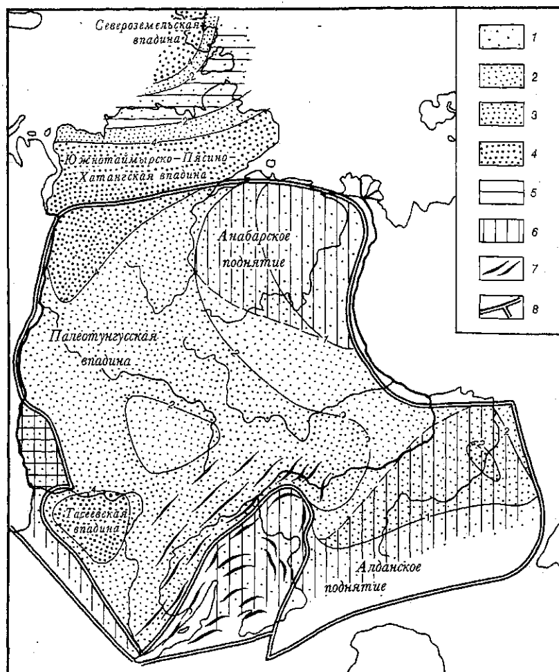
Рис. 30. Палеотектоническая схема Сибирской платформы и смежных метаплаформенных областей для синкаледонского этапа развития (кембрий — начало девона).
