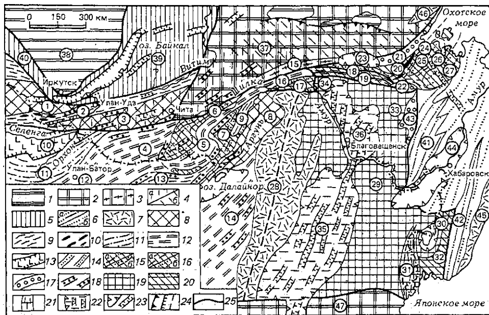
Рис. 60. Схема тектонического строения Забайкальско-Охотской складчатой области и Бурейно-Дунбэйской метаплатформенной области. 1—3 — древние платформы: 1 — плиты, 2 — щиты, 3 — южная зона Алдано-Станового щита; 4 — участки щитов и срединных массивов, подвергавшиеся тектономагматической активизации в палеозое (а) и мезозое (б); 5 — Присяжно-Енисейская
