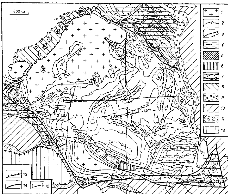
Рис. 3. Схематическая карта рельефа поверхности фундамента Восточно-Европейской платформы и смежных метаплаформенных областей. Сост. по тектонической карте Европы масштаба 1:10 000 и другим материалам.
