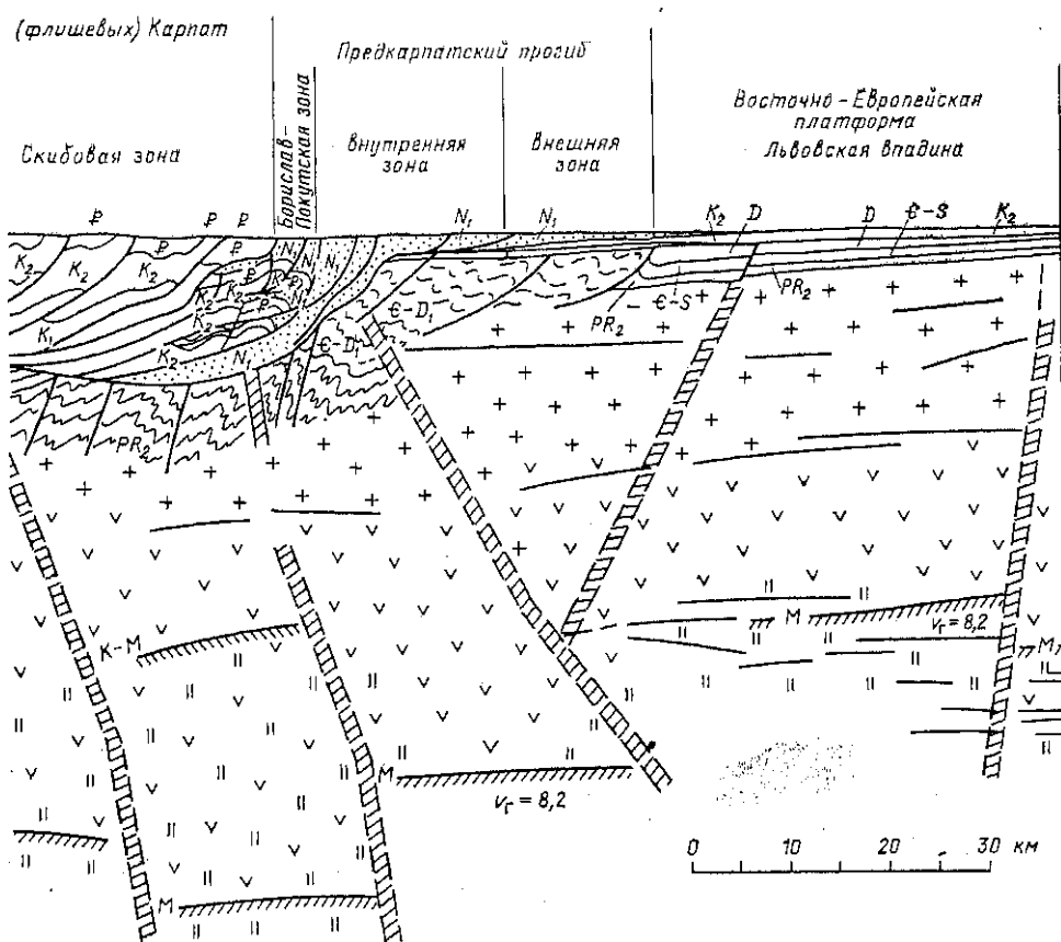
В. В. Глушко и др., с упрощениями): 1 — палеозойское основание флишевых Карпат; 2 — мел- ный со своего основания; 3 — базальтовый слой; 4 — «базальтовый» слой; 5 — базальтовый слой; 6 — коро-мантийный комплекс; 7 — верхняя мантия; 8 — нижняя мантия; 9 — граница коро-мантийного комплекса; 10 — раздел Мохо; 11 — отражающие границы
