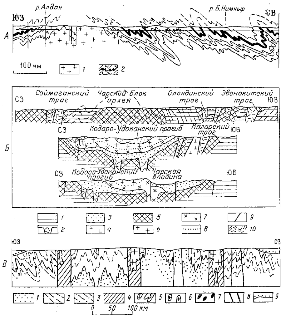
Рис. 28. Геологические разрезы докембрия Алдано-Станового щита и Анабарского массива.
