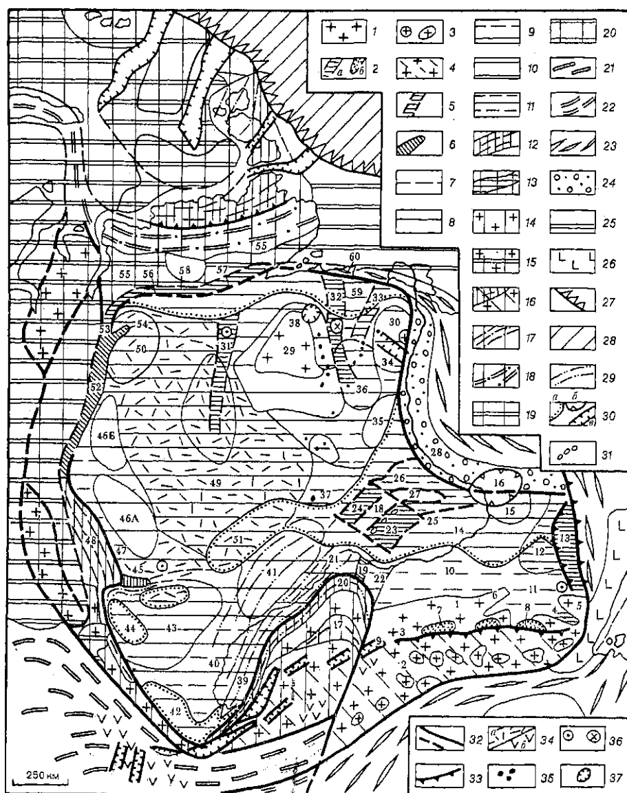
Рис. 24. Схема тектонического районирования Сибирской платформы и смежных метаплаформенных областей.
