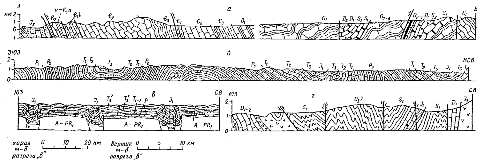
Рис. 81. Геологические разрезы Верхояно-Чукотской складчатой области: а — через Сетта-Дабанский антиклинорий; б — через Сартагский синклиниорий (восточное крыло северной части Верхоянского мегасинклиниория); в — через Эльгийский район пологих дислокаций в Яно-Индиговском мегасинклиниории; г — через северо-восточное крыло Омудевского горст-антиклинория (а, б, г — по Г. С. Гусеву, 1979; в — по С. И. Гаврикову)
