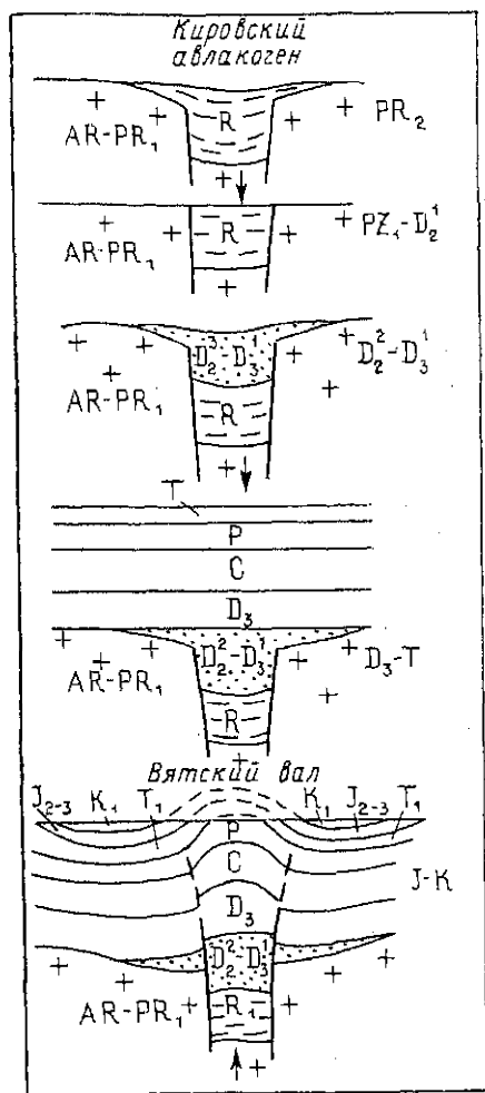
Рис. 6. Этапы развития Кировского авлакогена
