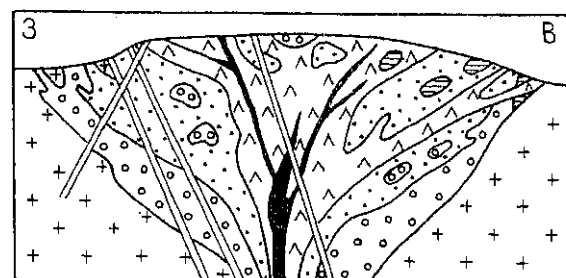
Рис. 16. Строение Хибинского и Ловозерского щелочных массивов (по Е. А. Каменеву, И. В. Буссену, А. С. Сахарову, Е. В. Свешниковой, с упрощениями и изменениями).
