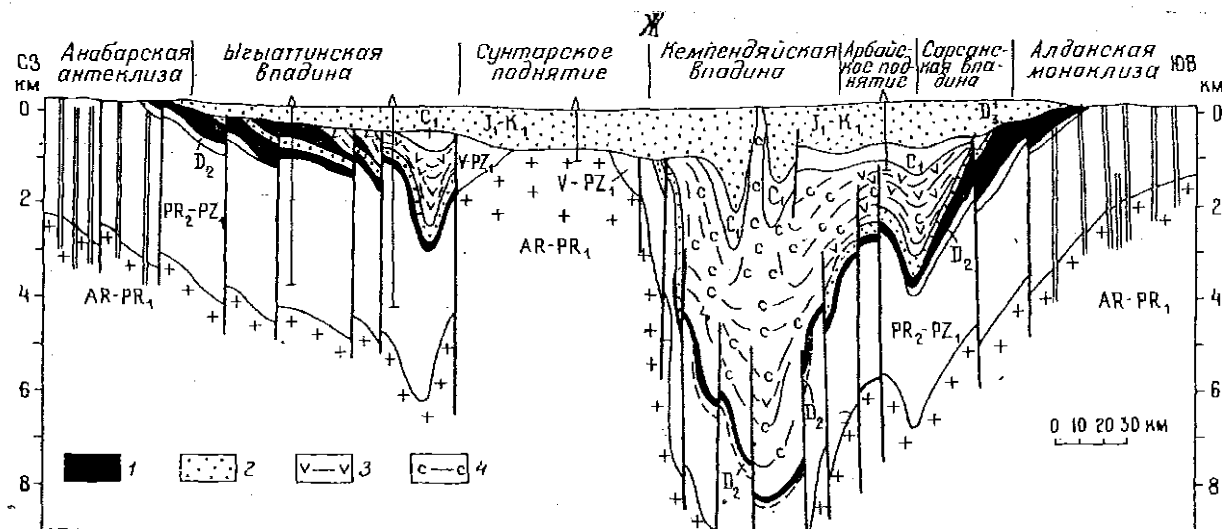
Рис. 26. Геологические профили через разные районы Сибирской платформы: А — средняя часть Тунгусской синеклизы (по А. Э. Конторовичу и В. С. Старосельцеву); Б — Иркийский авлакоген (по О. А. Вотаху и Б. В. Шибистову); В — Ангаро-Ленская ступень и Прибайкальский прогиб (по В. Е. Ханну); Г — Вилуйская синеклиза (по В. Е. Бакину и Д. П. Сидорову); Д — Урянский авлакоген (по Н. М. Чумакову); Е — Чульманская впадина (по П. В. Данкевичу); Ж — Патомско-Вилуйская система, погребенная под юрско-меловым чехлом Вилуйской синеклизы (по В. В. Гайдуку, 1985). 1 — толщи базальтов; 2 — толщи песчаников; 3 — вулканогенно-осадочные толщи; 4 — соленосные толщи верхнего девона
