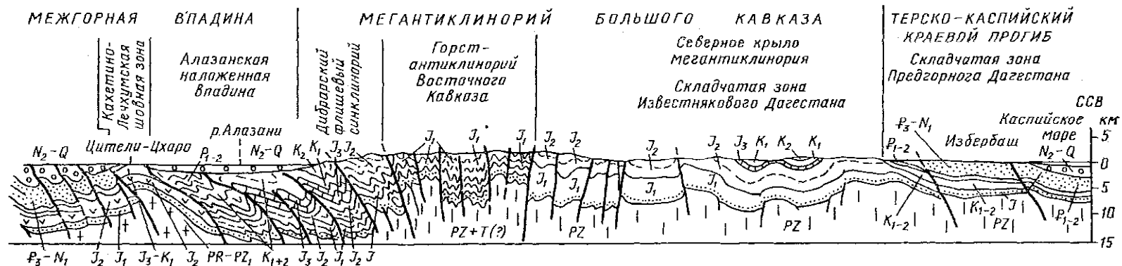
Рис. 74. Геологические разрезы через Центральный Кавказ (А), Западную (Б) и Восточную (В) части Восточного Кавказа
