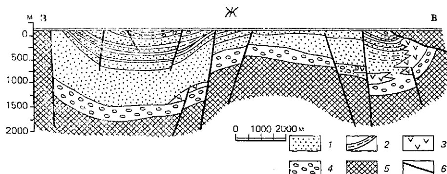
Рис. 44. Геологические разрезы разных зон Уральского складчатого сооружения: А — Верхнеисерская и Б — Бельская впадины Предуральяского краевого прогиба (по Ю. В. Казанцеву и М. А. Камалетдинову); В — Кракинский гипербазитовый аллохтон (по М. А. Камалетдинову и Т. Т. Казанцевой); Г — Западно-Мугоджарский синклиниорий (вдоль р. Шульдак) (по В. Г. Корниевскому, 1984); Д 2 mg — толстые подушечные лавы мугоджарского комплекса, прорванные параллельными долеритовыми дайками, δD 2 — перматитовые амфиболитизированные габбро; Д 2 kg — силлы и потоки долеритов, яшмовидные алевриты куркудукского комплекса, δD 2 — кварцевые диориты, Д 2 nl — подушечные лавы андезитобазальтов, туфы андезитов и туф-фитты мугоджарского комплекса с субвулканическими телами кислого и среднего состава, Д 2 sh — кремни и яшмы шульдакского горизонта, Д 2 gv — вулканогенно-осадочные породы алабасского комплекса, Д 2 gt — конгломераты, известняки и песчаники, Д 2 ln — известняковая толща, С 1 l — известняки, алевриты, песчаники и гравелисты, С 1 z — угленосная терригенно-карбонатная толща; Д — разрез через западный склон Северного Урала (по В. В. Юдину); Е — принципиальный разрез через Полярный Урал (по А. В. Нейве и др., 1977): 1 — верхнепалеозойские молассы, 2 — сланцевый палеозой многоосинклиналиной зоны, 3 — доордовикское основание, 4 — силур-девонская эвгеосинклиналиная серия, 5 — плагнограниты, 6 — габброиды и амфиболиты, 7 — гипербазиты, 8 — главные надвиги; Ж — Челябинская раннемезозойская грабенообразная впадина (по В. С. Бочкареву, 1973): 1 — угленосные отложения челябинской серии (Т 3 ), 2 — пласты углей, 3 — базальты и 4 — конгломераты туринской серии (Т 1-2 ), 5 — палеозойский складчатый фундамент, 6 — разломы
