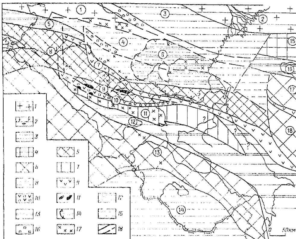
Рис. 75. Схема тектонического строения доальпийского (доюрского) основания Кавказской области (по материалам А. А. Белова и А. И. Летагина) с упрощениями и изменениями, без палинеастических реконструкций).
