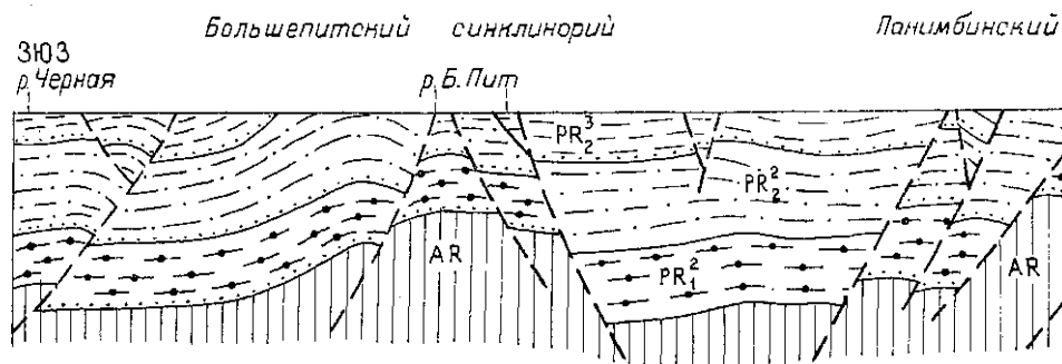
Рис. 38. Схематический геологический профиль через среднюю часть сооружения Енисейского края. PR^3 — тунгусикская и осянская серии, PR^2 — сухонитская серия, PR^1 — тейская
