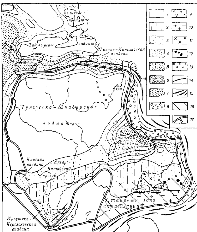
Рис. 34. Палеотектоническая схема Сибирской платформы и смежных метаплатформенных областей для синпозднекимерийского этапа развития (юра — мел):
