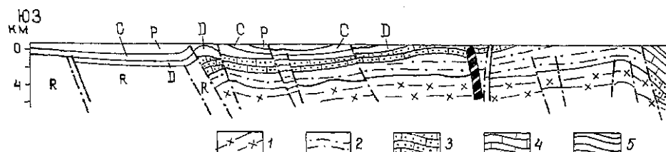
Рис. 21. Геологический профиль через Средний Тиман (Четласский камень) (по 1 — средний рифей (светлинская свита); 2—5 — верхний рифей (четлаская, джежимская, нижне- и верхнебыстринская свиты); 6 — терминальный рифей (кислоручей-
