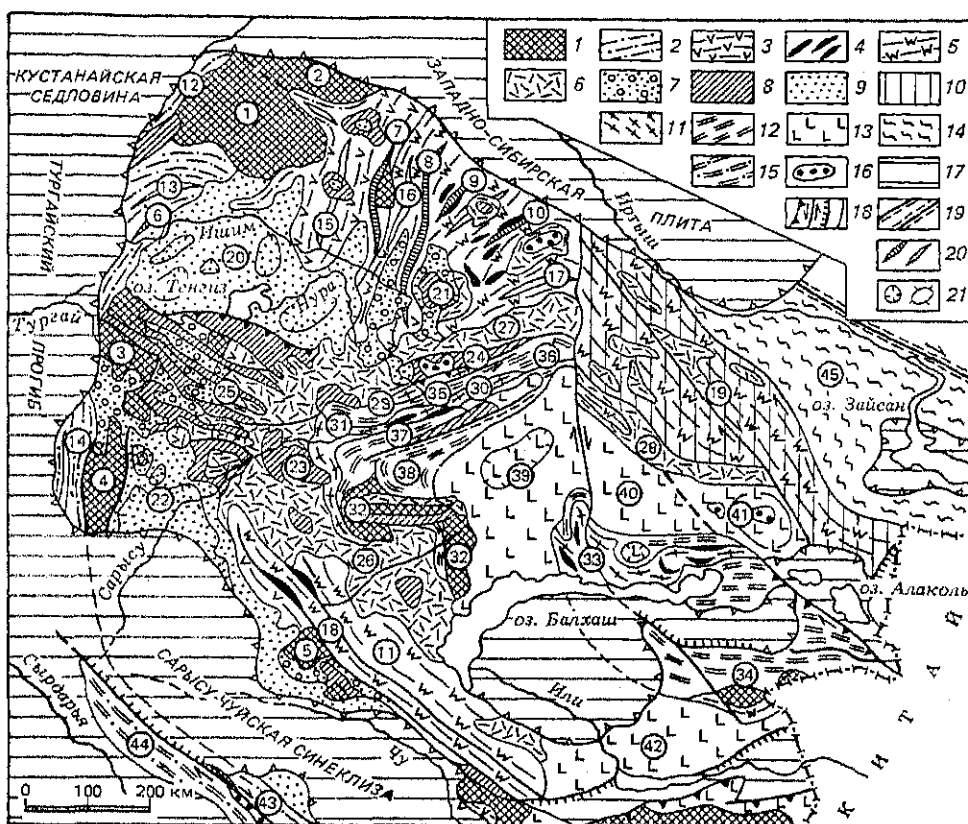
Рис. 46. Схема тектонического строения складчатой области Казахского нагорья. 1—13 — палеозойская складчатая область Казахского нагорья: 1 — выступы архейско-нижнепротерозойского и частично нижне-среднерифейского метаморфического фундамента; 2—10 — каледонская Казахстанско-Северотяньшанская складчатая система; 2 — позднепериферийско-ордовикский складчатый комплекс в мезогесинклинальной зоне ранних каледонид, 3 — то же, в эвгесинклинальной зоне, 4 — кембро(?)раннеордовикский офиолитовый комплекс (в каледонидах и герцинидах), 5 — кембро-нижнесилурийский складчатый комплекс в эвгесинклинальных зонах поздних герцинид, 6 — нижнедевонско-франский наземно-вулканогенный комплекс в девонском вулканическом поясе и частью вне его, 7 — среднедевонско-франский молассовый пологоскладчатый комплекс, 8 — фаменско-визейский карбонатный комплекс, 9 — среднекаменноугольно-пермский молассовый комплекс в наложенных впадинах, 10 — раннегерцинская регенерация каледонского складчатого основания Чунгизской зоны; 11—13 — герцинская Джунгаро-Балхашская складчатая система: 11 — кемброордовикский эвгесинклинальный комплекс в ядрах антиклинорий, 12 — силурийско-нижнекаменноугольный мезогесинклинальный комплекс на крыльях антиклинорий и в синклинориях, 13 — среднекаменноугольно-пермский наземно-вулканогенный комплекс Балхаш-Илийского вулканического пояса; 14 — позднегерцинская Иртыш-Зайсанская складчатая система; 15 — каледоно-герцинская Срединно-Тяньшанская складчатая система; 16 — раннемезозойские впадины, выполненные континентальной угленосной юрой; 17 — позднемезозойско-кайнозойский чехол Западно-Сибирской, Северо-Туранской плит и параплатов; 18 — разломы типа надвигов и взбросов, сдвигов, сбросов и без расчленения; 19 — палеозойские зоны смятия и расщепления; 20 — оси палеозойских антиклинорий и синклинорий; 21 — брахиморфные структуры в позднепалеозойских впадинах.
