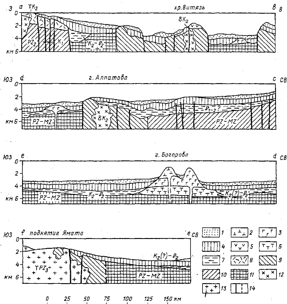
Рис. 91. Сейсмологические разрезы дна Японского моря по линиям а—в и с—d—e—f (см. рис. 90) (по И. И. Берсеневу и В. Л. Безверхнему, 1988):
