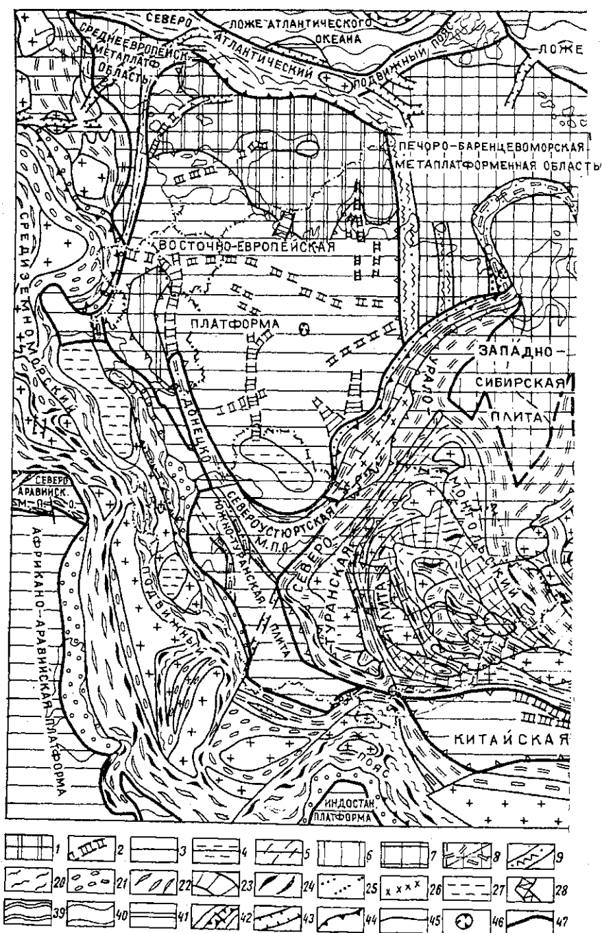
Рис. 1. Схема тектонического 1—5 — древние платформы: 1 — выступы дорифейского фундамента (щиты); 2 — плитным чехлом); 3 — области, покрытые вендско-фанерозойским чехлом (древние тисинеклизы); 5 — каледонские складчатые зоны в плитном чехле. 6—14 — метапласти нерасчлененные, без чехла, 7 — то же, с фанерозойским чехлом (молодые плитном чехле; 9—14 — авлакогеосинклинальные складчатые зоны: 9 — байкальские позднекайменские, 14 — альпийские. 15—38 — подвижные пояса: 15 — остаток
