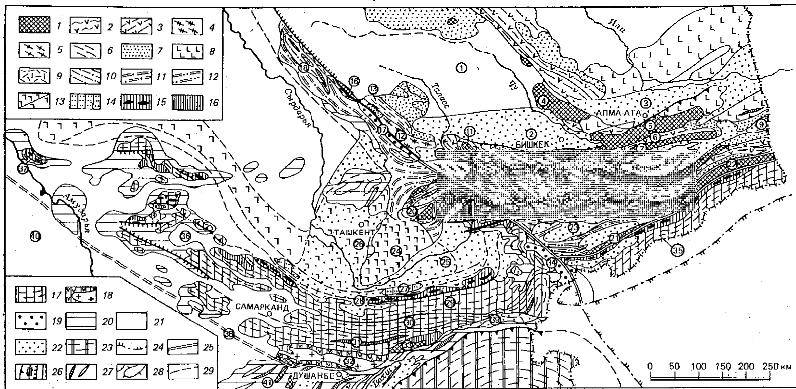
Рис. 51. Схема тектонического строения Тянь-Шаня.
