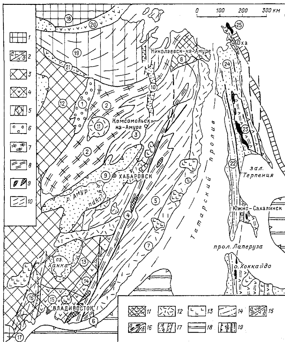
Рис. 88. Схема тектонического строения Сихотэ-Алинской и Сахалинской областей: 1 — щиты древних платформ; 2 — герцинско-позднекеммерийские складчатые зоны (а) и краевые прогибы (б) Амуро-Охотского сегмента Урало-Монгольского подвижного пояса; 3—5 — Бурейно-Дунбэйская метаплатформенная область: 3 — приподнятые метаплатформенные массивы, 4 — краевые участки Ханкайского массива, подвергшиеся опусканиям и тектономагматической переработке в палеозое и мезозое, 5 — Западно-Приморская авлакогеосинклинальная палеозойская складчатая зона; 6—18 — Тихоокеанский подвижный пояс: 6—13 — Сихотэ-Алинская позднемезозойская складчатая область: 6 — Бурейнский краевой прогиб, 7 — Хингано-Бурейнский мегантиклинорий, сложенный протерозойскими, палеозойскими и нижнемезозойскими отложениями, 8 — Сихотэ-Алинский и Прибрежный антиклинории, сложенные верхнепалеозойскими и нижнемезозойскими отложениями, 9 — блоки метаморфического фундамента в зоне Сихотэ-Алинского антиклинория, 10 — синклинорий, в основном выполненные юрскими и меловыми отложениями, 11 — гипотетический Тахтинский массив с мезозойским пологоскладчатым чехлом, 12 — сеонско-палеогеновый Восточно-Сихотэалинский вулканический пояс и синхронные ему наложенные вулканические
