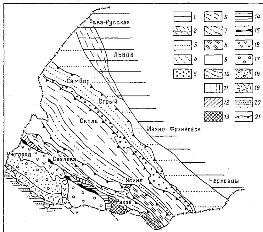
Рис. 67. Схема тектонической зональности Украинских Карпат (по С. С. Круглову и др., с изменениями):
