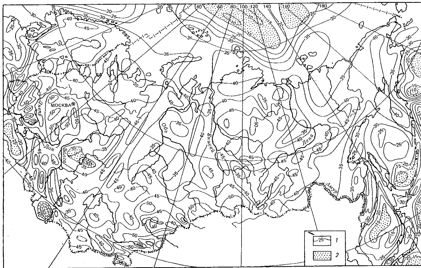
Рис. 8. Схема глубинного строения земной коры в пределах территории России, близлежащих стран и ложа прилегающих морей. Сост. по разным материалам.
