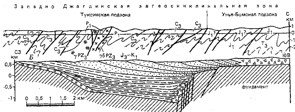
А — Гусиноозерская впадина в Западном Забайкалье (по В. А. Соловьеву); Б — ву); В — Джагинская складчатая система (по Г. Л. Кирилловой, М. Г. Турбину,
