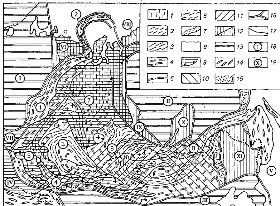
Рис. 42. Тектоническое положение и районирование Урало-Монгольского подвижного пояса.
