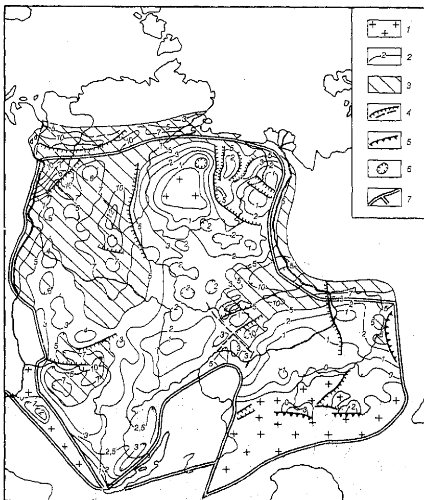
Рис. 25. Схематическая карта рельефа фундамента Сибирской платформы. Сост. с использованием карт Н. В. Неволлина и др., Г. С. Гусева, Г. С. Фрадкина и др.
