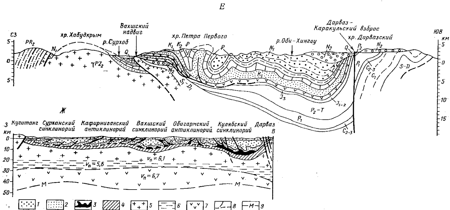
Рис. 63. Геологические разрезы Скифской, Южно-Туранской плит и Южно-Таджикской впадины: А — Западное Предкавказье (по А. Н. Шарданову и др.); Б — Восточное Предкавказье (по А. И. Летавину и др.); В — западная часть Южно-Туранской плиты (по В. И. Попкову), черным показаны залежи нефти; Г — Бухаро-Хивинская ступенчатая зона (по М. Б. Гохбергу, Е. А. Рогожину и др.); Д — Южно-Таджикская впадина (по А. Ю. Мессиневой и др.); Е — Памиро-Алайская (Дарваз-Заалайская) зона в районе Гармского полигона (по Т. В. Гусевой и др.); Ж — геолого-геофизический разрез земной коры через Южно-Таджикскую впадину (по Я. А. Беккеру и др. 1983, с упрощениями): 1 — неоген — антропоген; 2 — мел — палеоген; 3 — соленосная верхняя юра; 4 — подсолевая юра — триас (?); 5 — герцинский комплекс — «гранитный» слой; 6 — волновод в средней части коры; 7 — «базальтовый» слой; 8 — надвиги и тектонические покровы; 9 — граница Мохо
