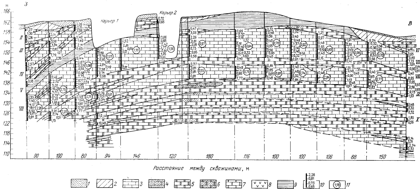
Рис. 14. Геолого-литологический разрез Храповицкого месторождения (Воробьева Гора). По Е. А. Кононовой.
