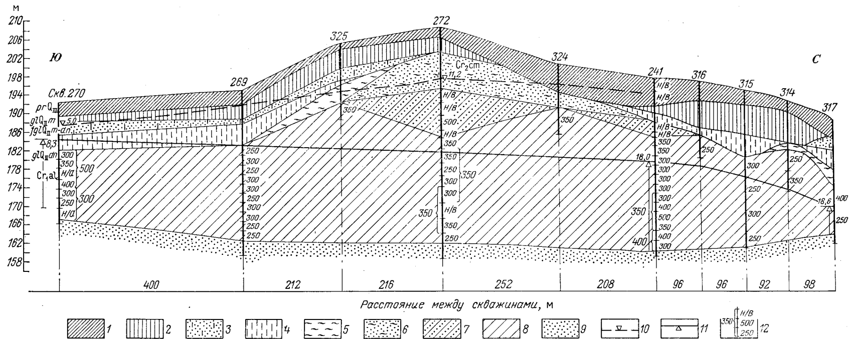
Рис. 27. Геолого-литологический разрез Ельדיгинского месторождения. По М. А. Гроховской.
