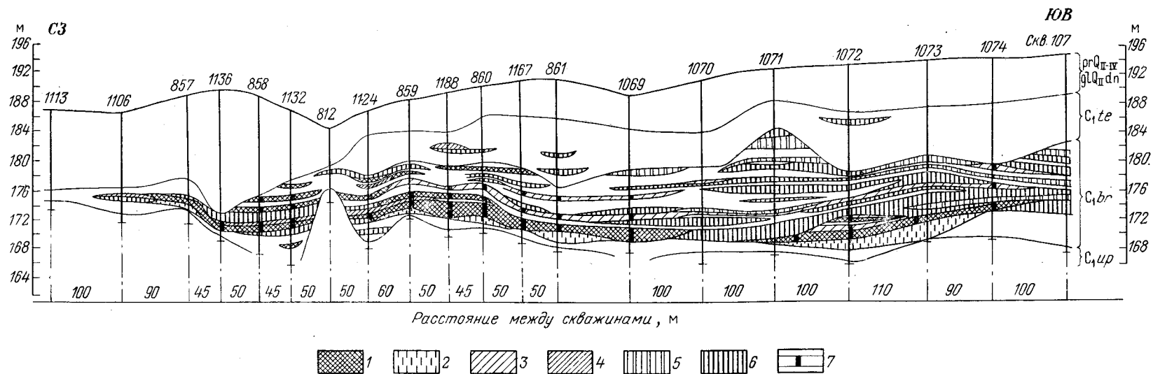
Рис. 24. Геолого-литологический разрез продуктивной толщи Безово-Березовского участка Суворовского месторождения. По Н. Ф. Кузовлеву.
