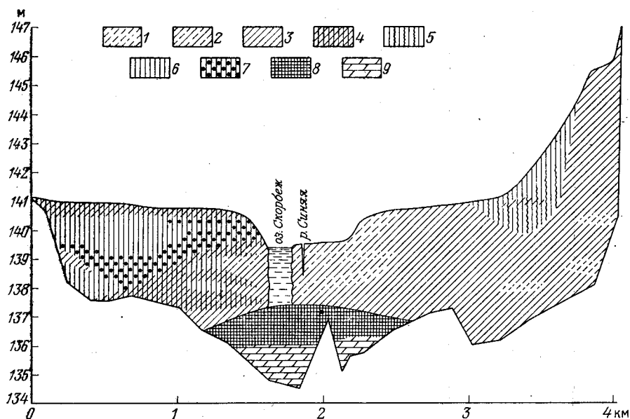
Рис. 7. Разрез торфяной залежи месторождения Сачинского (Калининская область).
