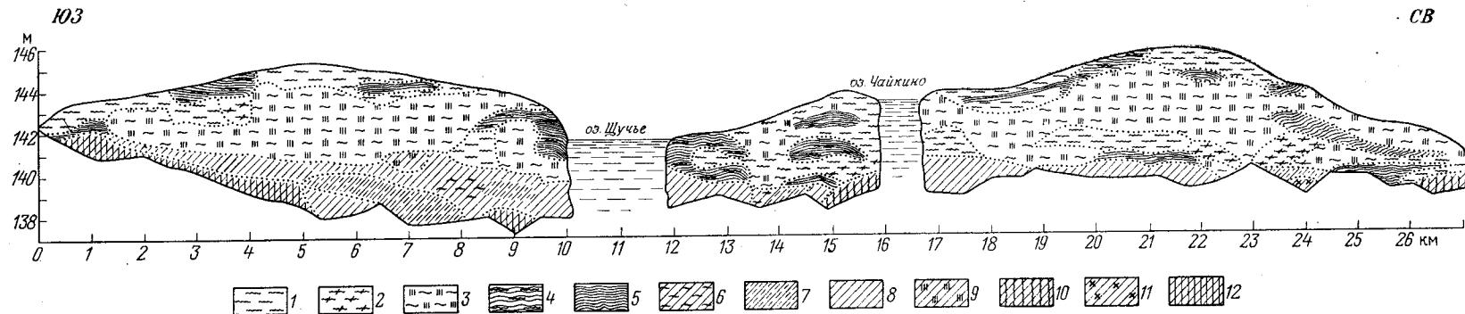
Рис. 5. Разрез торфяной залежи месторождения Оршинский Мох (Калининская область). Торф: 1 — медиум; 2 — фускум; 3 — шейхцериево-сфагновый верховой; 4 — пушицево-сфагновый верховой; 5 — пушицевый верховой; 6 — осоково-сфагновый низинный; 7 — осоково-гипновый низинный; 8 — осоковый низинный; 9 — шейхцериевый низинный; 10 — осоковый тростниковый низинный; 11 — осоково-хвощевый низинный; 12 — древесно-осоковый низинный
