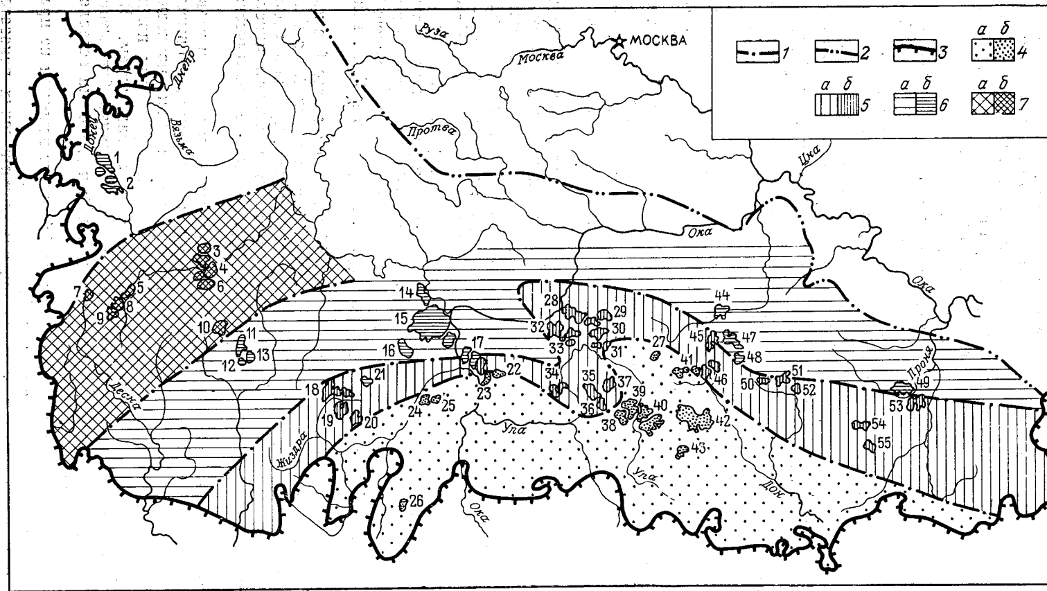
Рис. 1. Схема районирования месторождений угля Подмосковского бассейна по условиям осушения. Составлена М. И. Чельцовым (Гипроцветмет).
