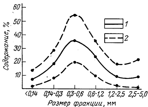
Рис. 21. Средний гранулометрический состав песчаного и мелкогравийного материала аллювиальных месторождений.
