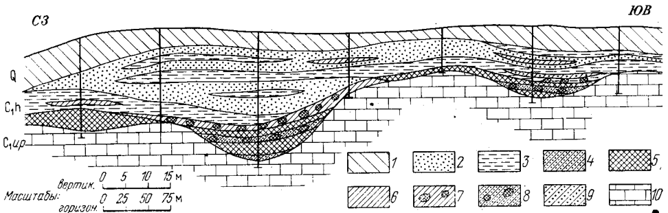
Рис. 11. Разрез Шенуровского месторождения.
