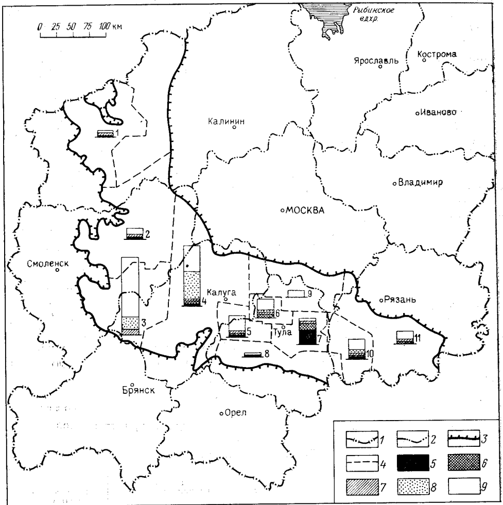
Рис. 2. Схематическая карта угленосных районов Подмосковского бассейна с указанием степени промышленного освоения балансовых запасов угля. По А. К. Борисевич.
