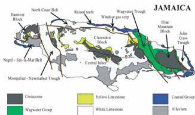
Рисунок 1. Упрощенное геологическое строение Ямайки, демонстрирующее положение Central Inlier и других районов, представляющих интерес.
