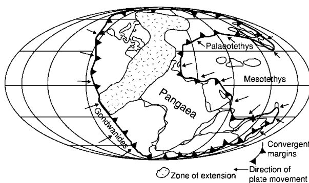
Figure 3 Triassic Pangaea, showing major tectonic elements. After Lucas (2000) The epicontinental Triassic, an overview. Zentralblatt für Geologie und Paläontologie Teil I 7-8: 475–496.
