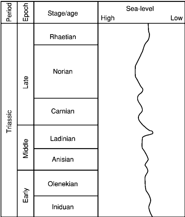
Figure 4 Triassic sea-level curve. After Lucas (2000) The epicontinental Triassic, an overview. Zentralblatt für Geologie und Paläontologie Teil I 7-8: 475–496.
