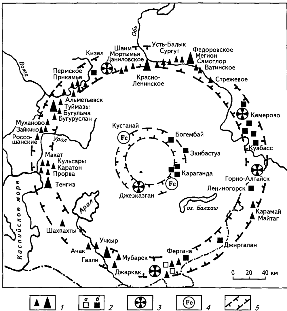
Рис. 22. Распределение месторождений полезных ископаемых в деформационных зонах Ишимской планетарной геосистемы (по О.Л.Кузнецову и др., 1994)
