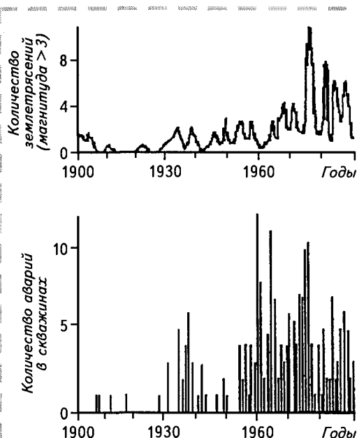
Рис. 23. Сопоставление временного хода распределения сильных землетрясений и аварий в скважинах в пределах Терско-Сунженской нефтегазоносной зоны (по Н.А.Касьяновой, 1996)
