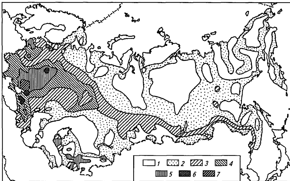
Рис. 29. Схема распределения техногенного геохимического воздействия (по М.А.Глазовой и др., 1995)
