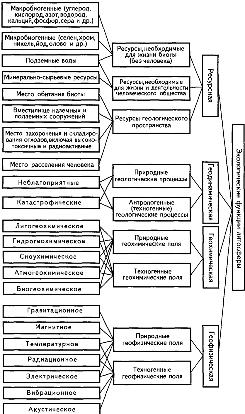
Рис. 3. Систематика экологических функций литосферы (по В.Т.Трофимову и Д.Г.Зинину)
