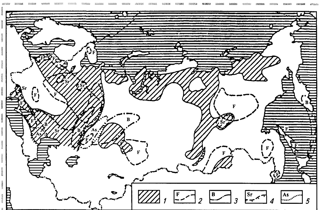
Рис. 26. Гидрогеохимические провинции подземных вод с повышенными содержаниями \text{SO}_4^{2-} и \text{Cl} (1), F (2), B (3), Sr (4), As (5) на территории бывшего СССР (по С.Р.Крайнову, В.П.Закутину, 1994). Республики Средней Азии и Кавказа не показаны
